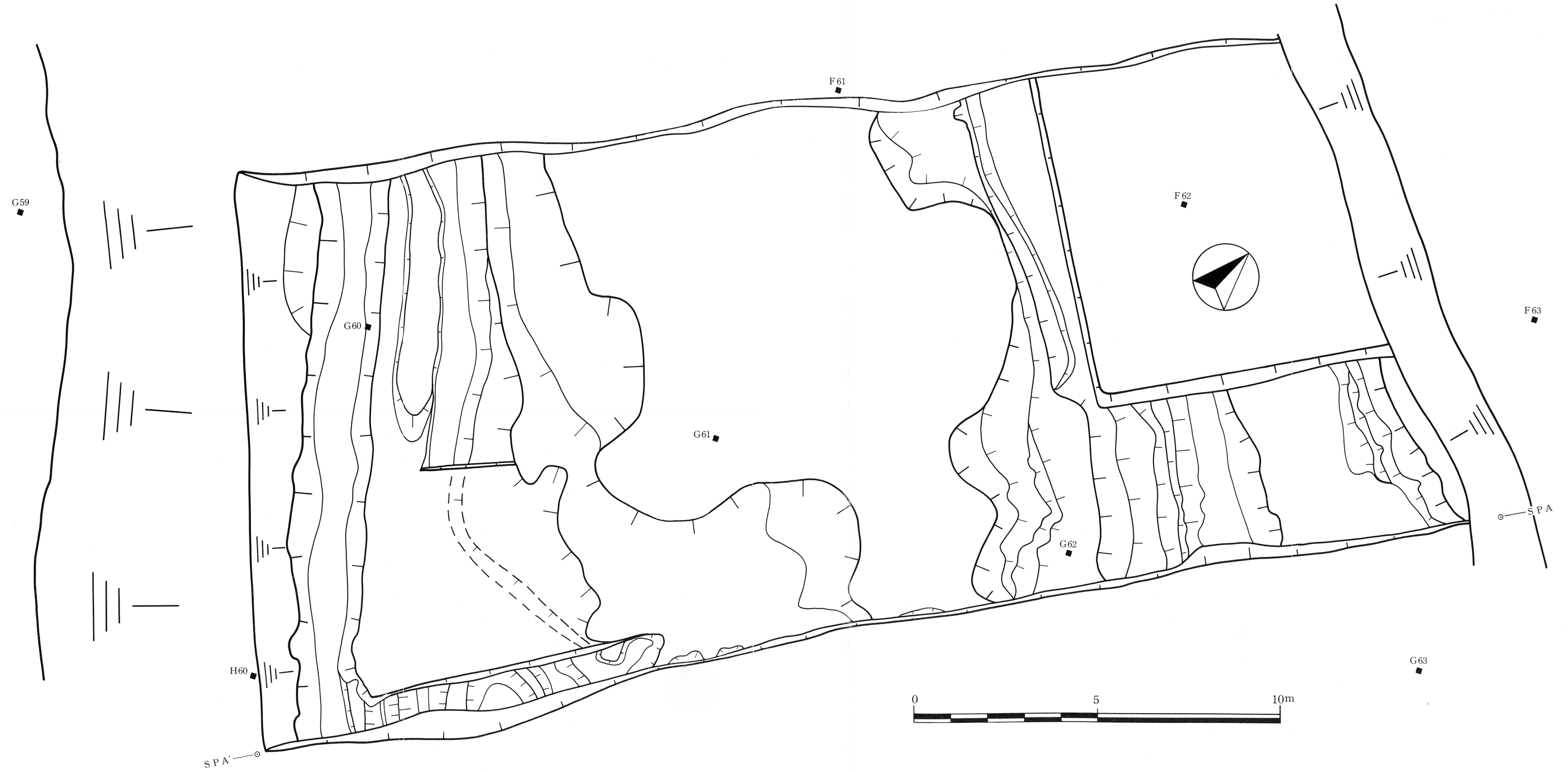
Fig. 3 調査区平面実測図
