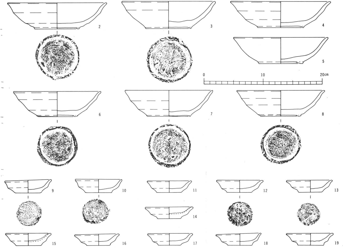
大根古窯出土遺物実測図
