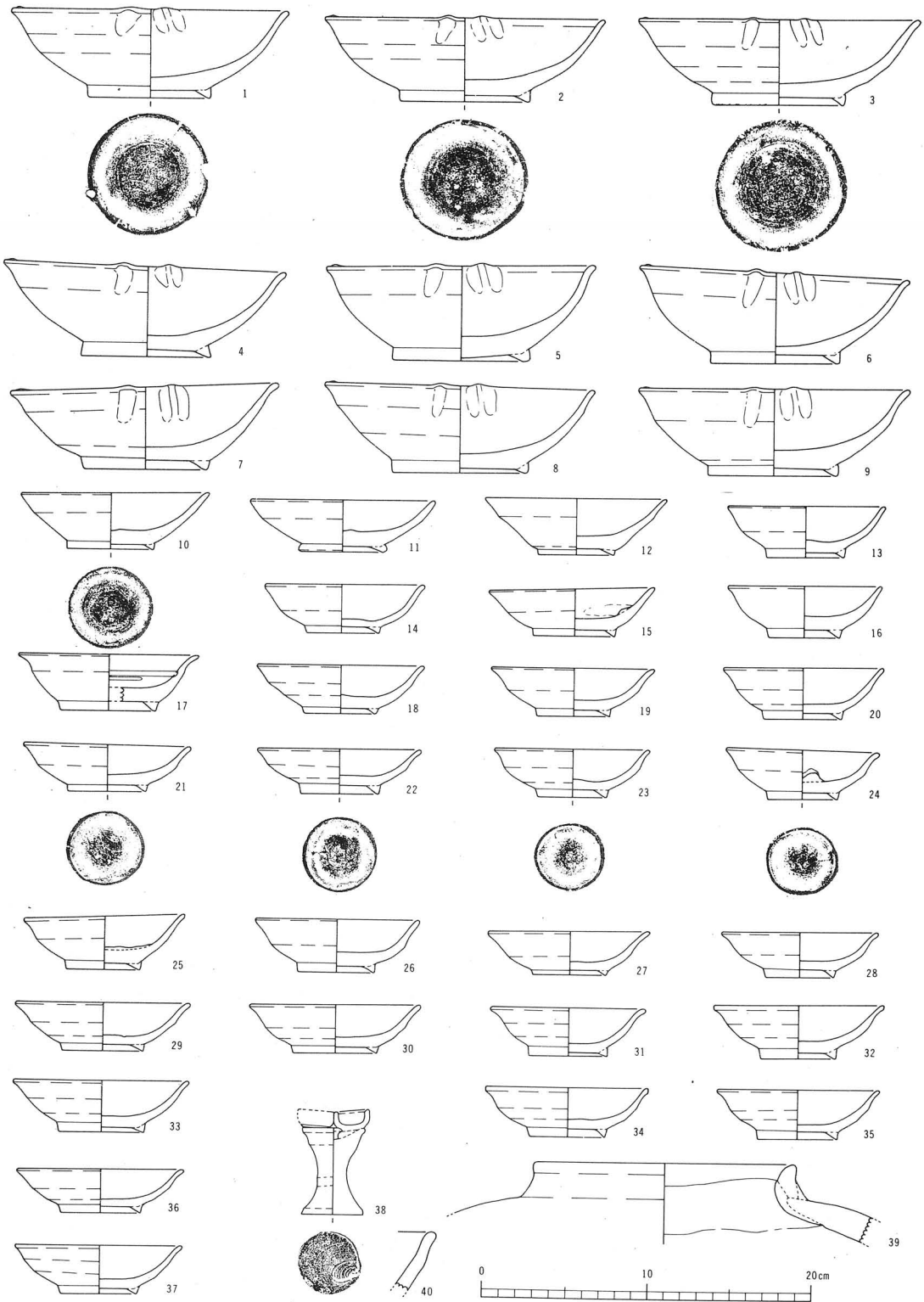
法秀古窯出土遺物実測図 1
