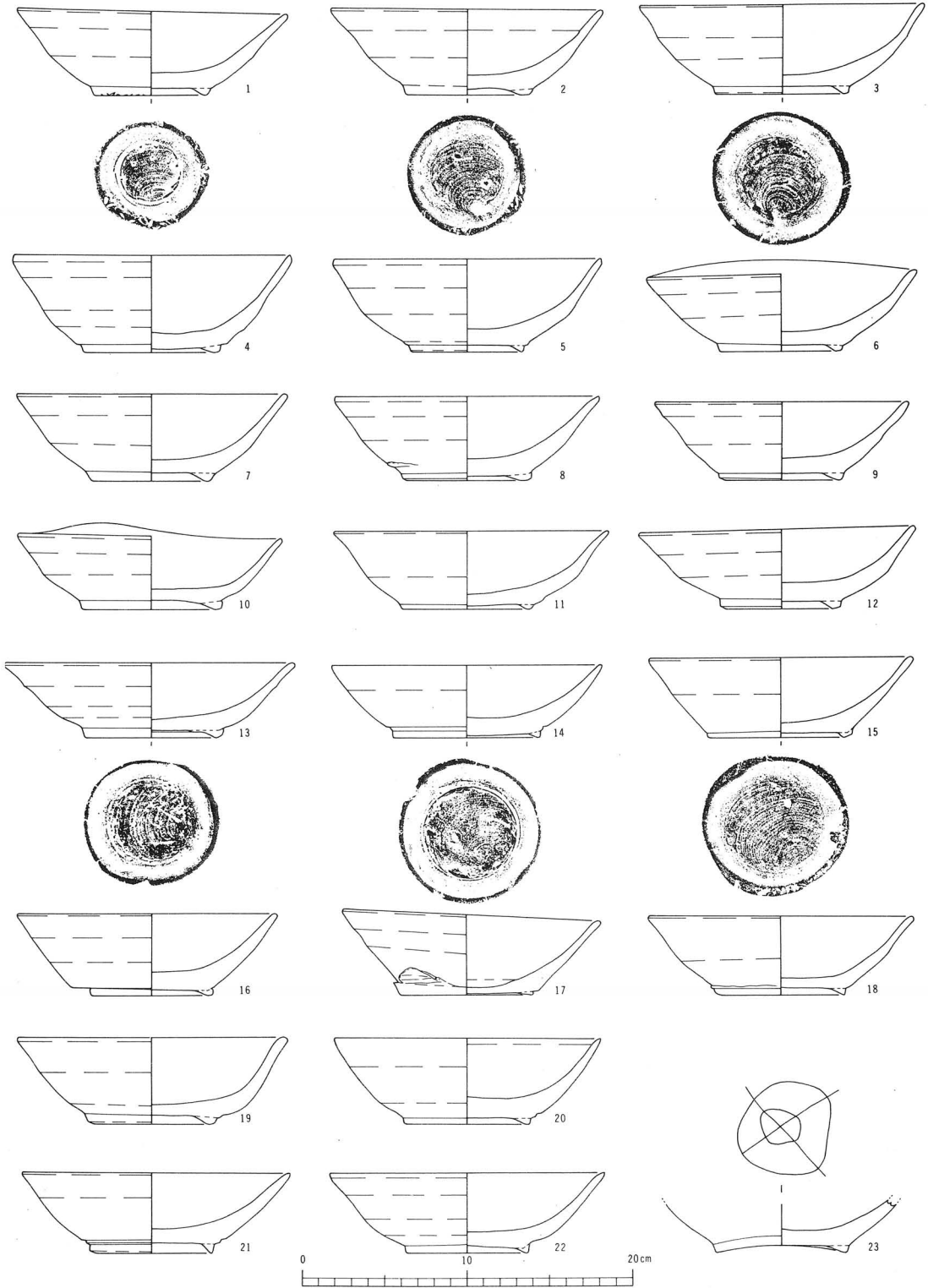
法秀古窯出土遺物実測図 4
