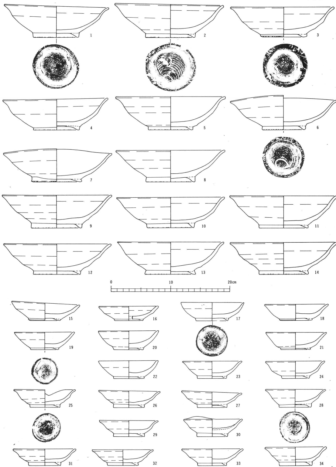
法秀古窯出土遺物実測図 6
