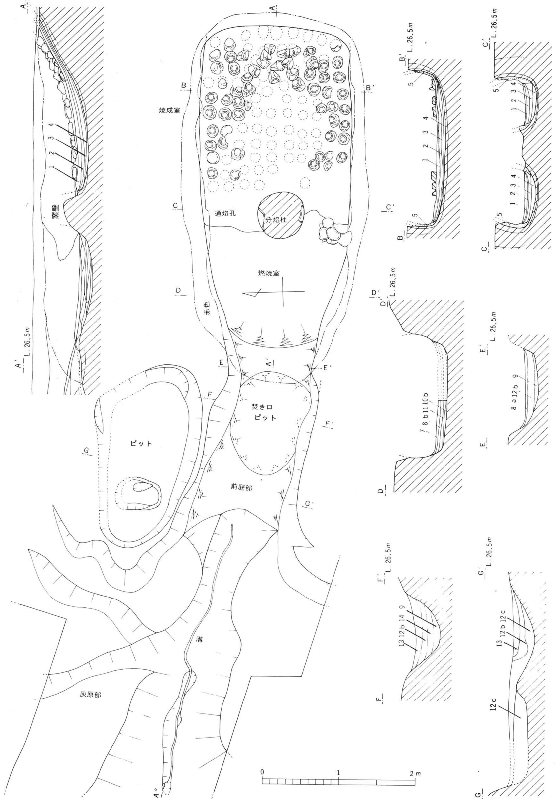
法秀古窯窯体実測図
