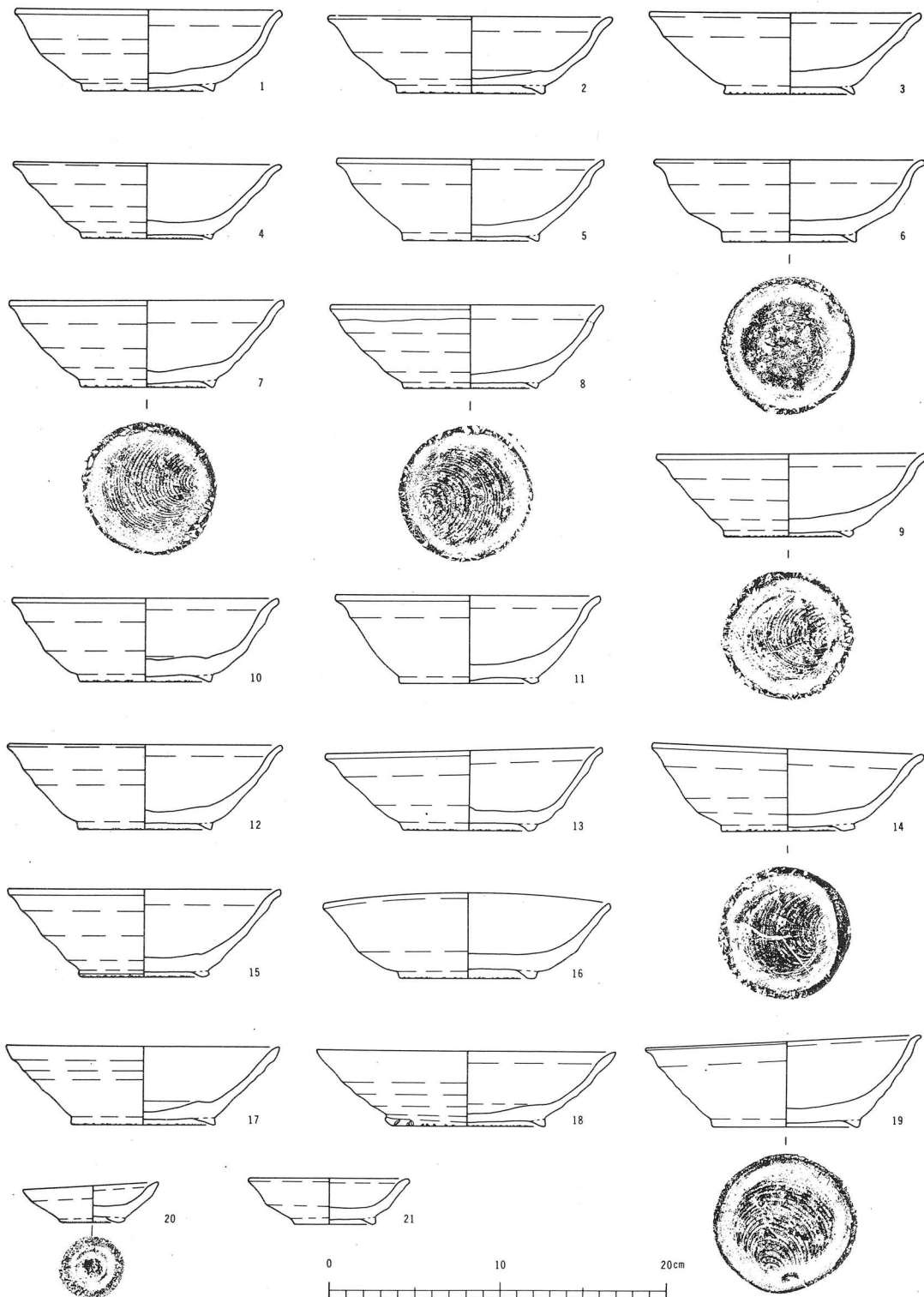
寺の前古窯出土遺物実測図 1
