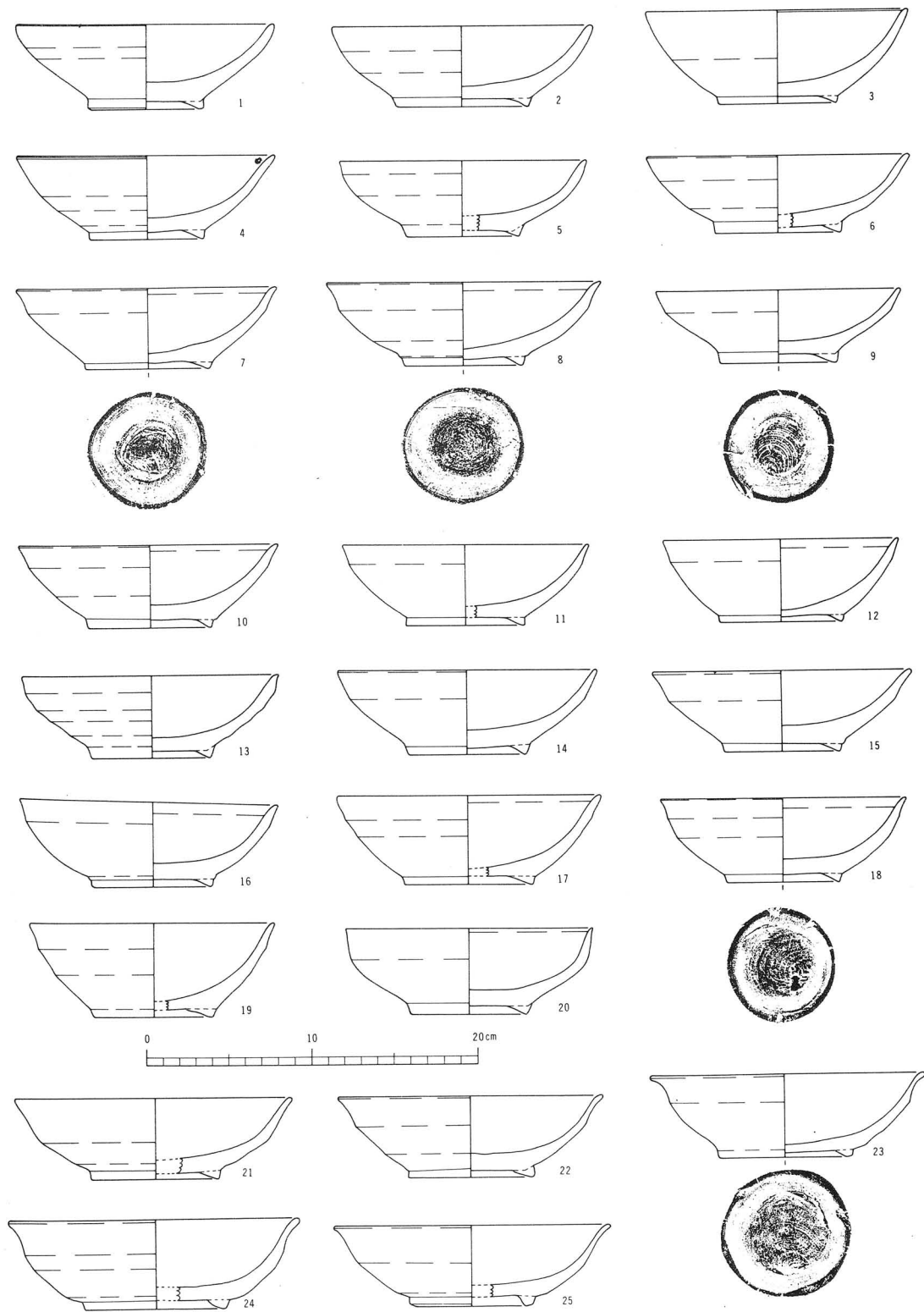
法秀古窯出土遺物実測図 2
