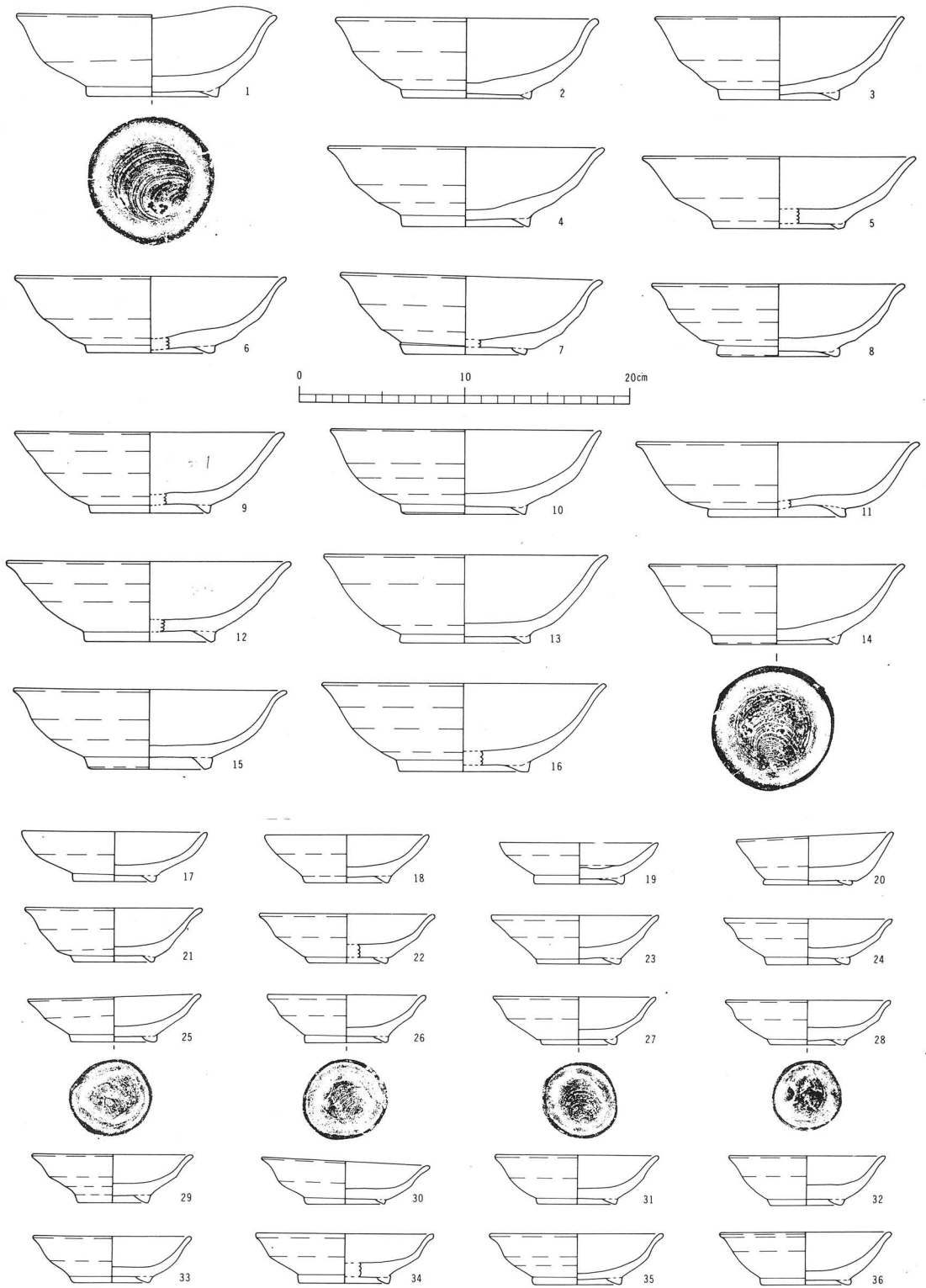
法秀古窯出土遺物実測図 3
