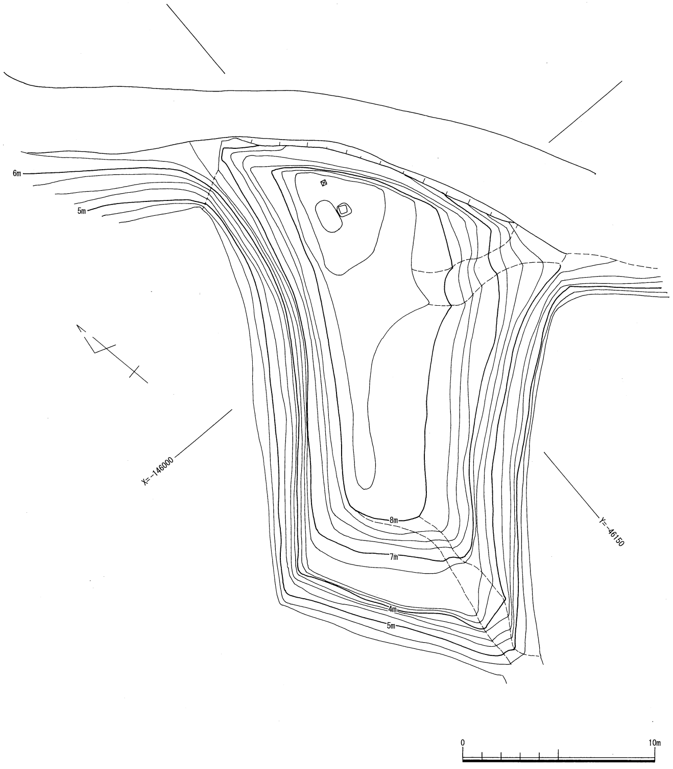
图 23 築堤残存部実測図
