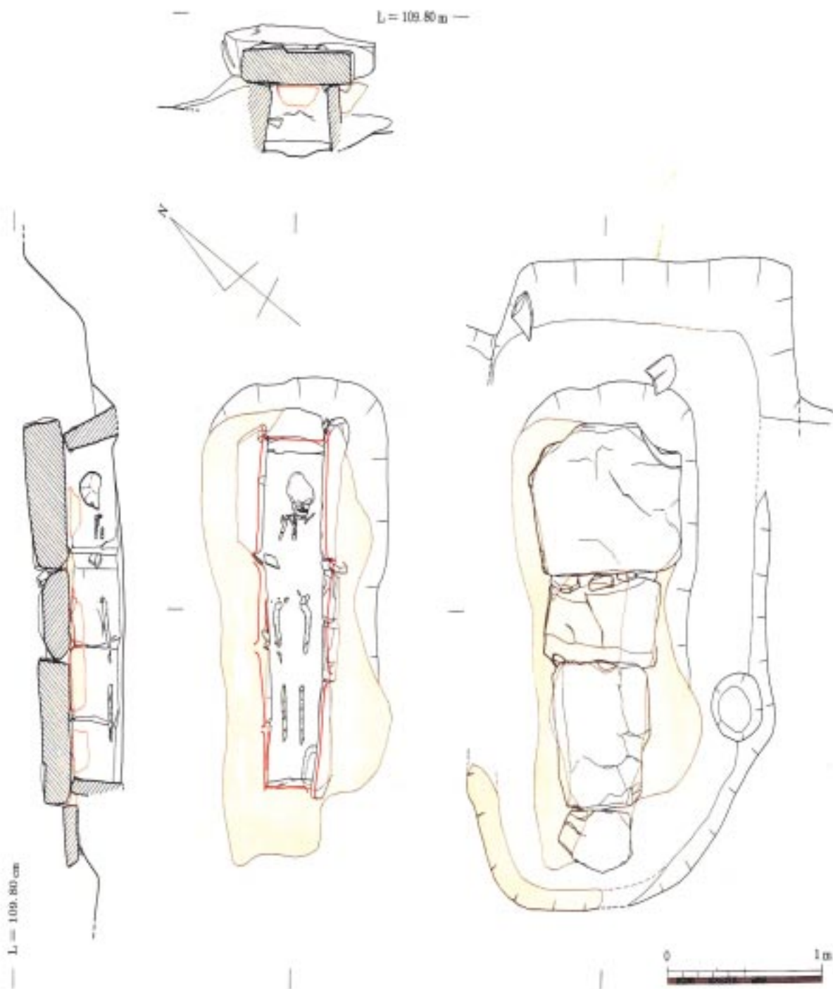
第84図 芳ヶ谷3号古墳第1主体部実測図
