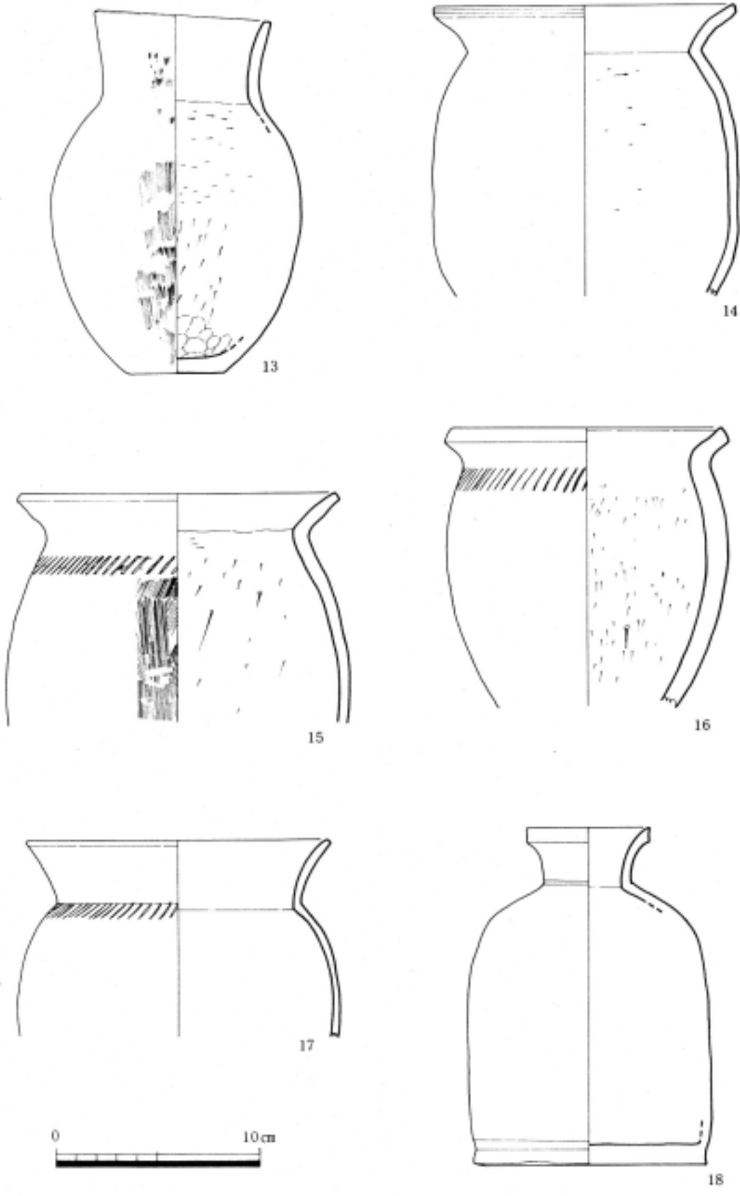
第 87 図 大谷遺跡 A 地点出土土器実測図(2)
