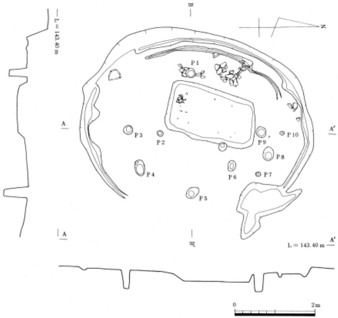
第76图 大谷遺跡A地点第1号住居跡実測図
