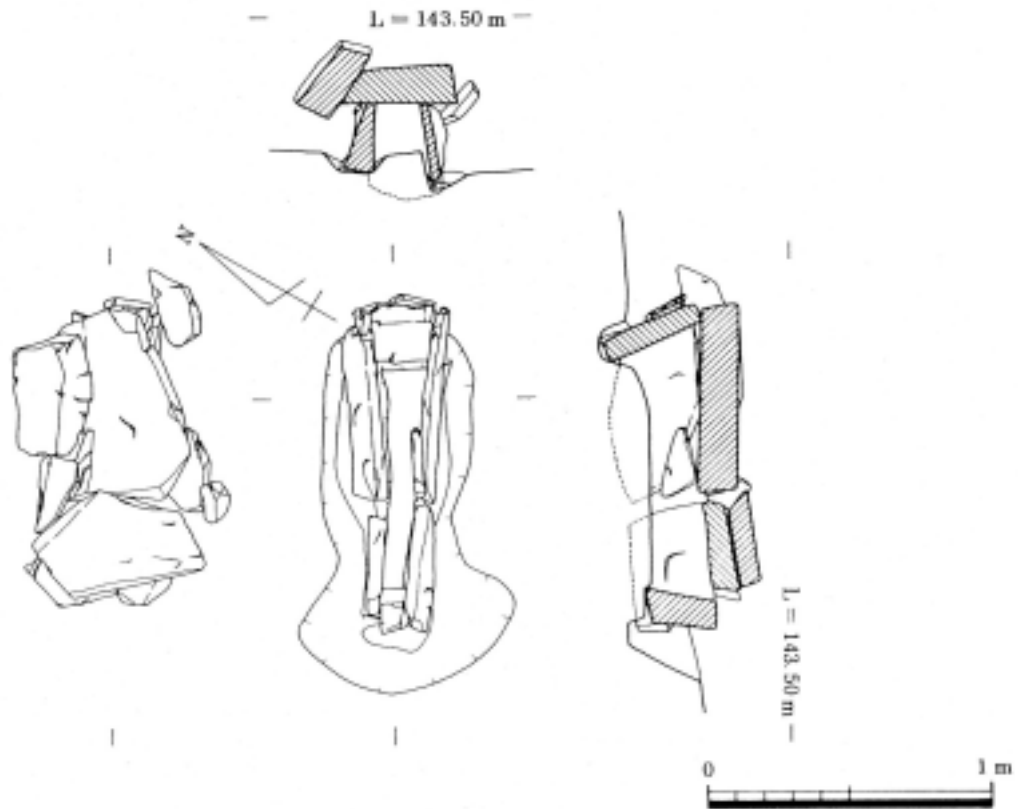
第83図 芳カ谷2号古墳主体部実測図
