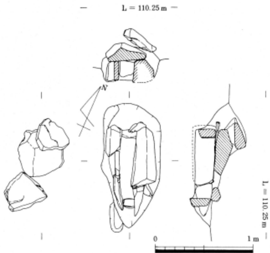
第85図 芳カ谷3号古墳第2主体部実測図
