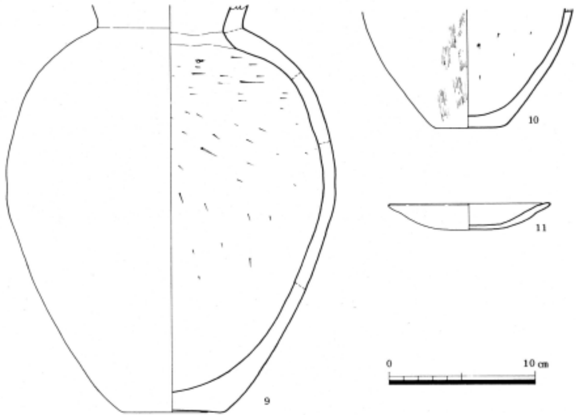
第 89 图 大谷遺跡 B 地点出土土器実測図(2)
