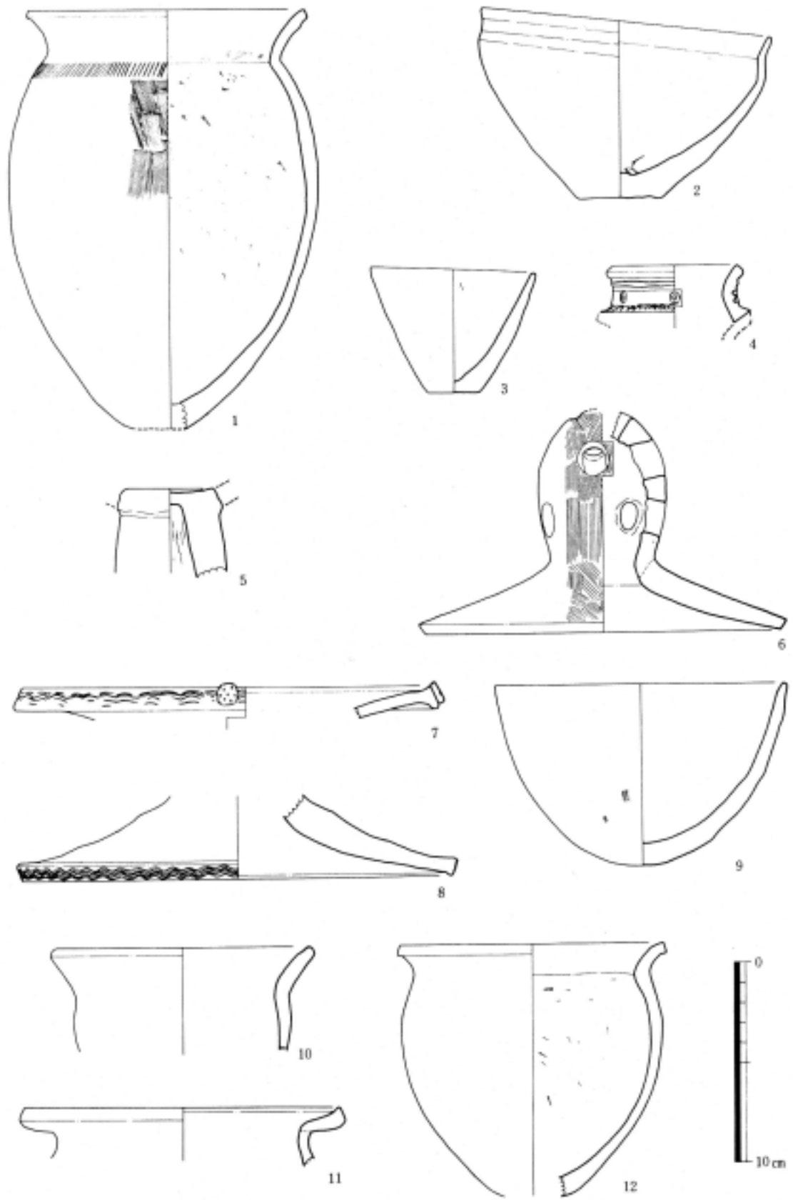
第 86 図 大谷遺跡 A 地点出土土器実測図(1)
