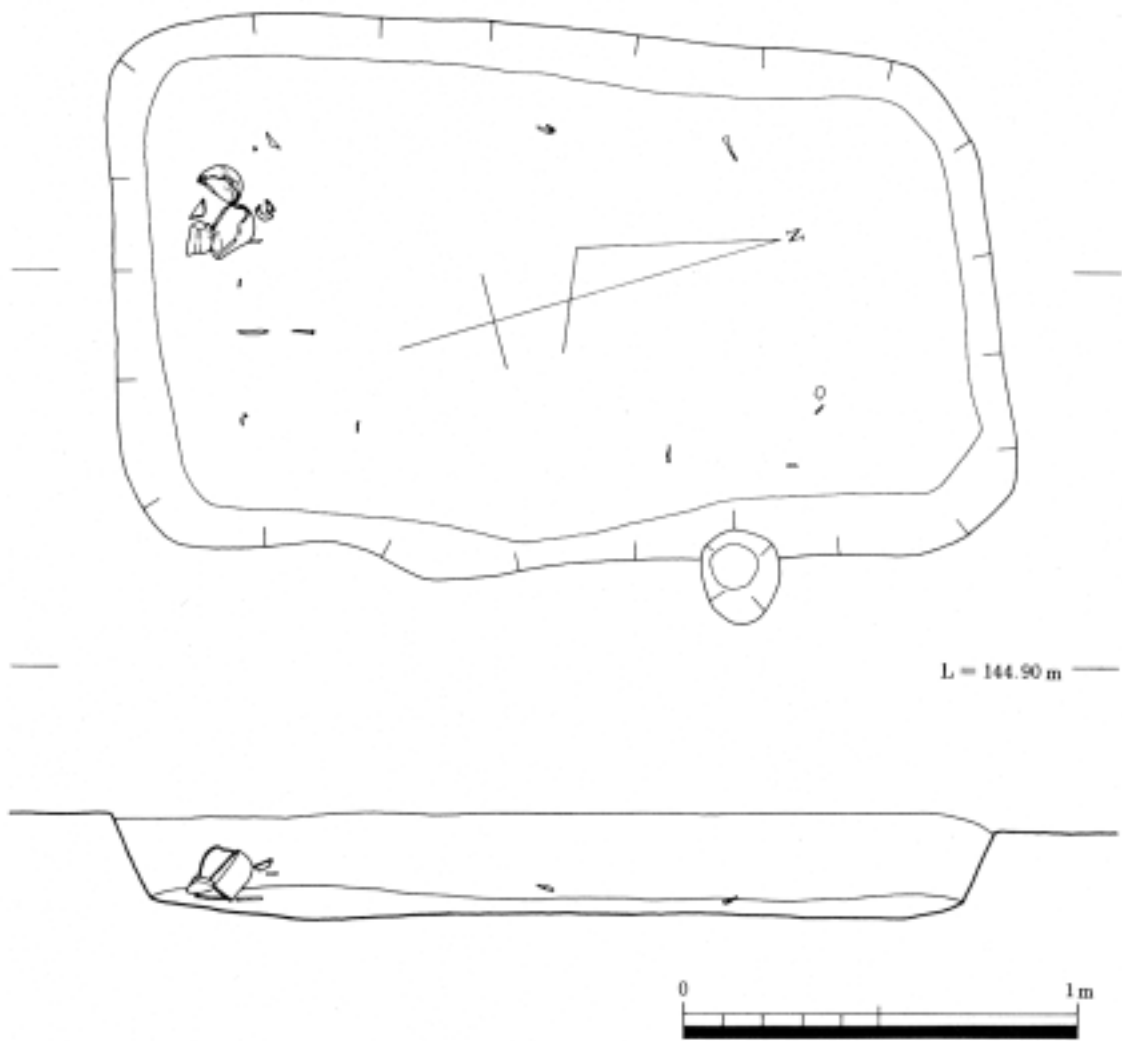
第79図 大谷古墓実測図
