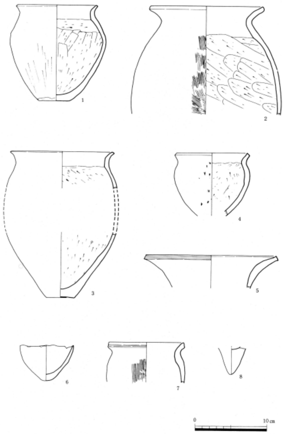
第 88 図 大谷遺跡 B 地点出土土器実測図(1)
