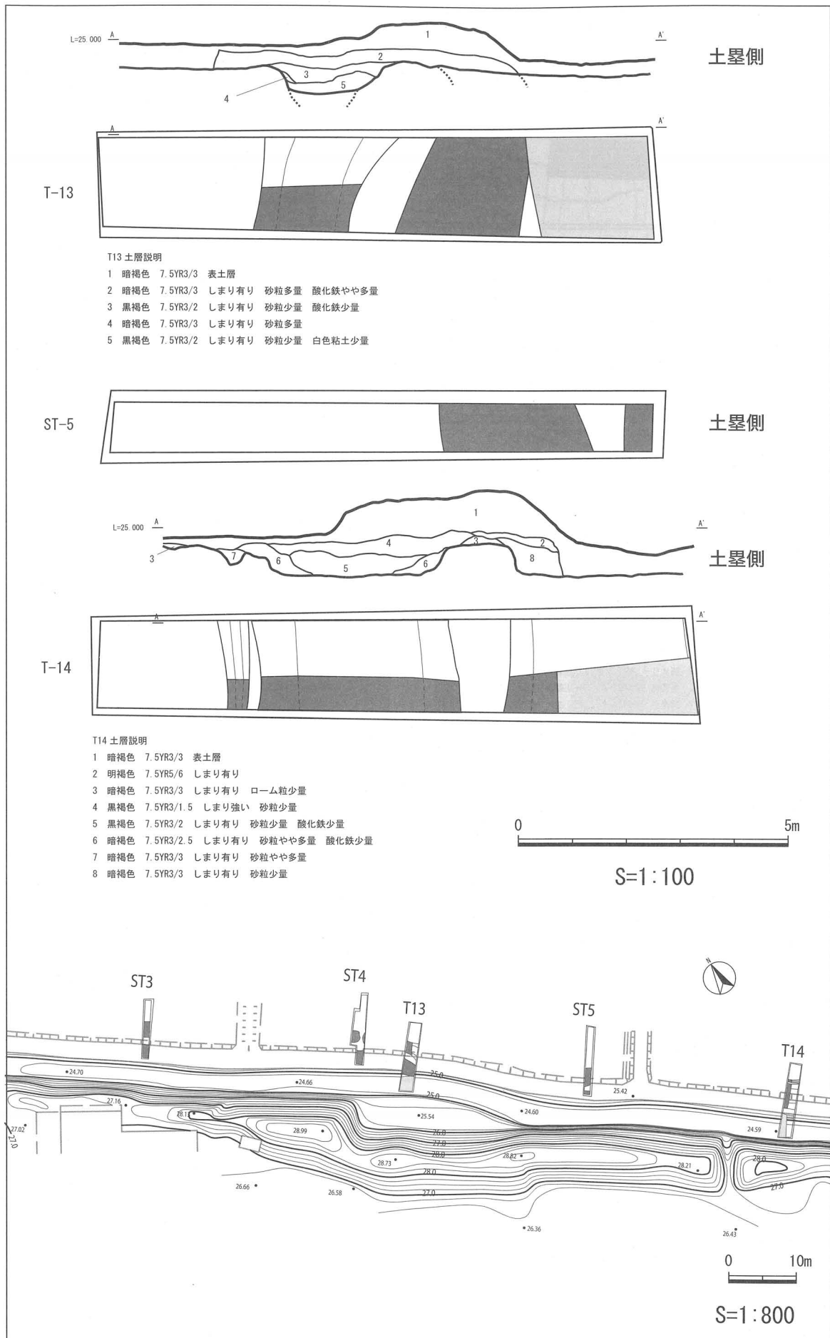
図11 トレンチ13, 14平面及び断面図
