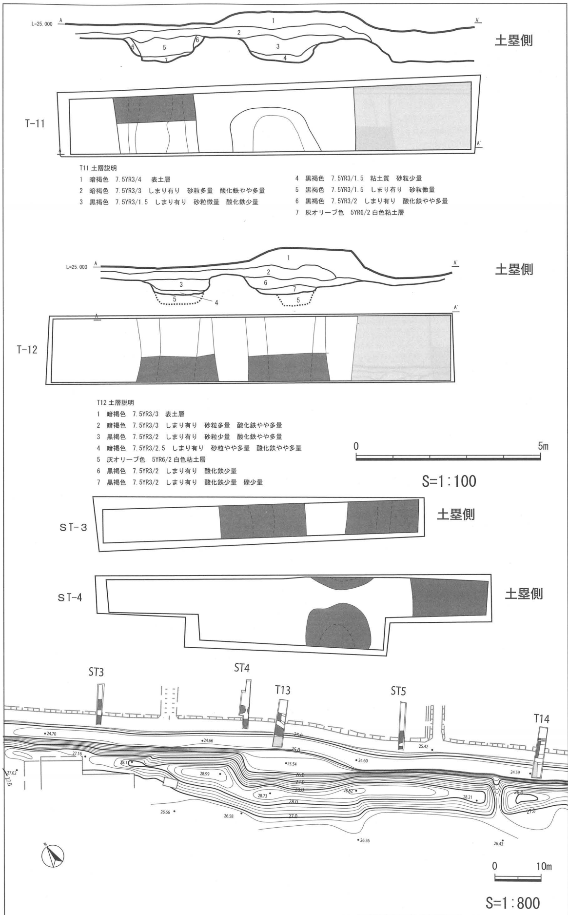
図10 トレンチ11, 12平面及び断面図
