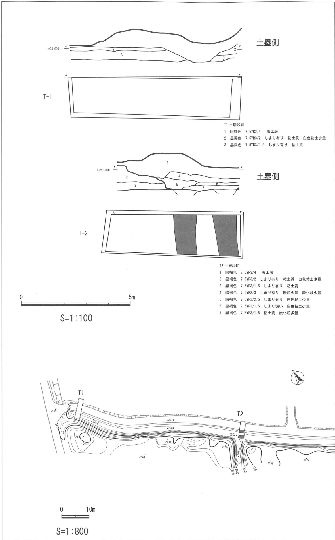
図5 トレンチ1,2平面及び断面図
