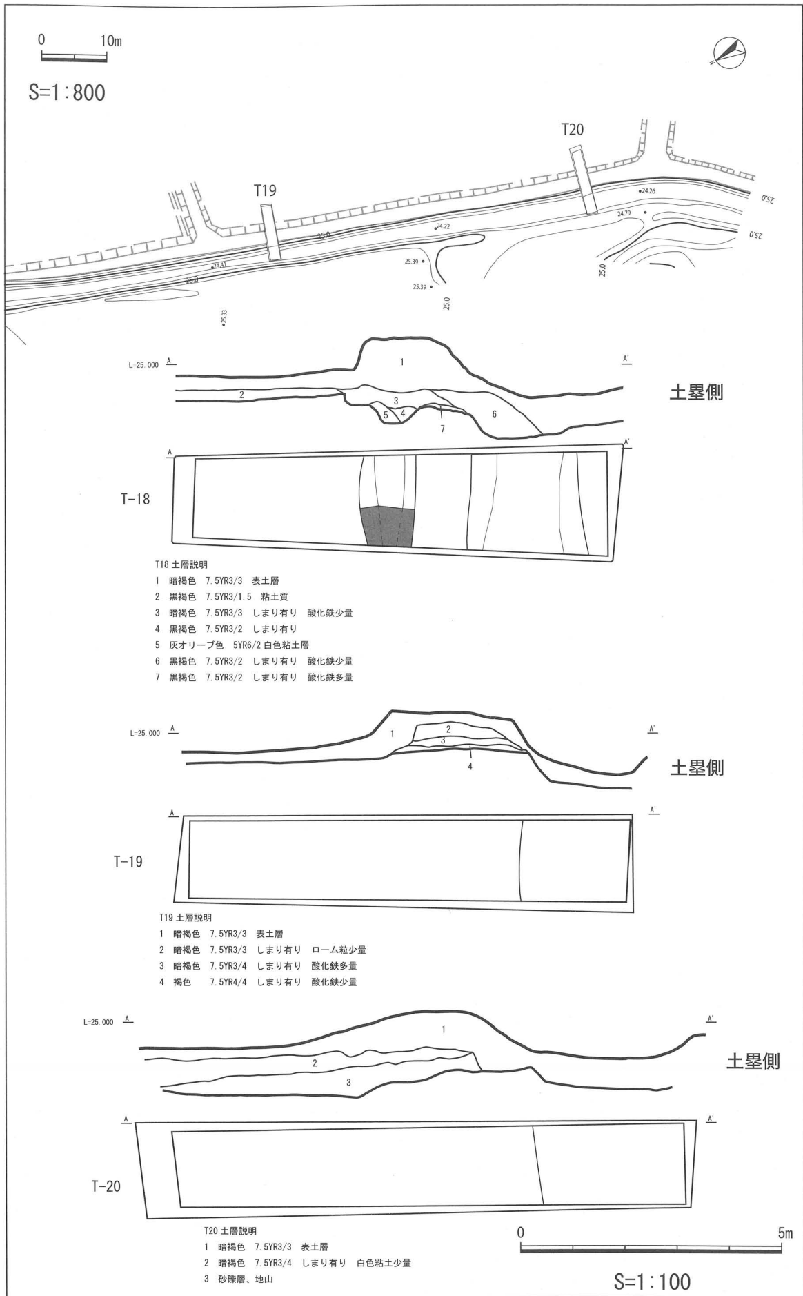
図14 トレンチ18, 19, 20平面及び断面図
