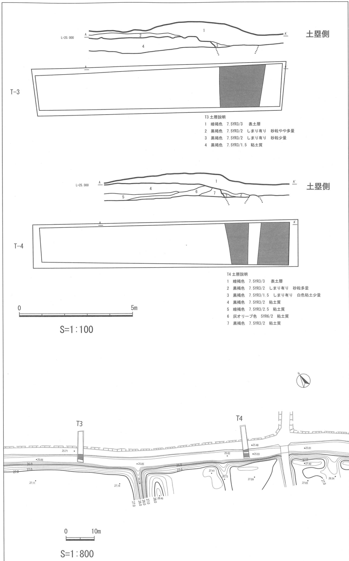
図6 トレンチ3,4平面及び断面図
