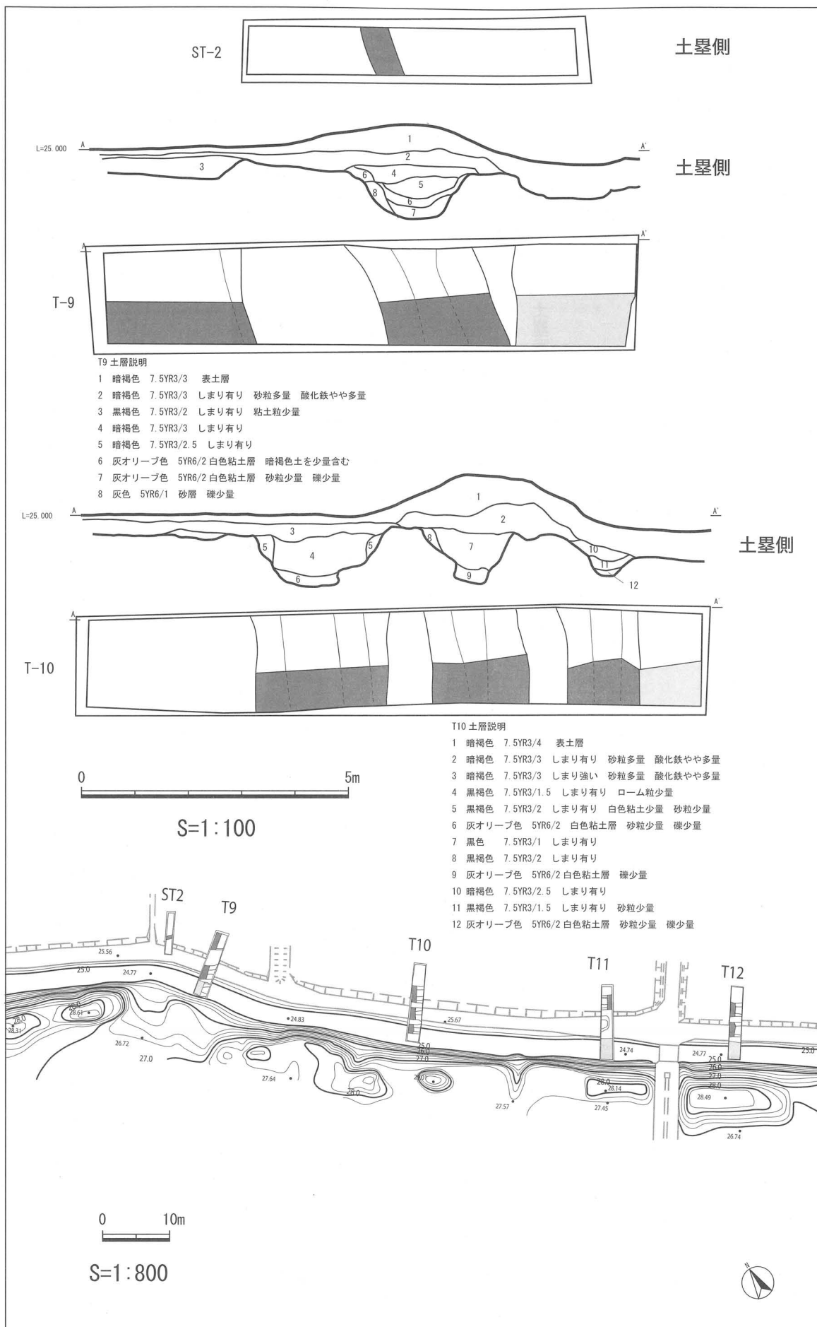
図9 トレンチ9, 10平面及び断面図
