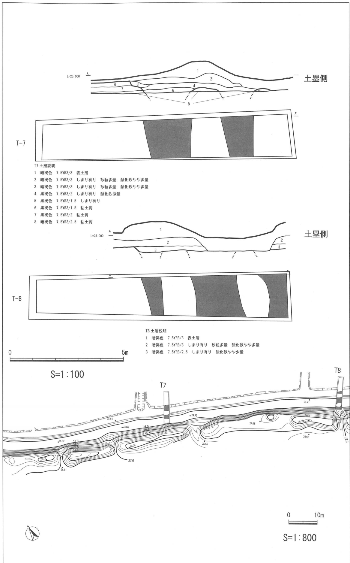
図8 トレンチ7, 8平面及び断面図
