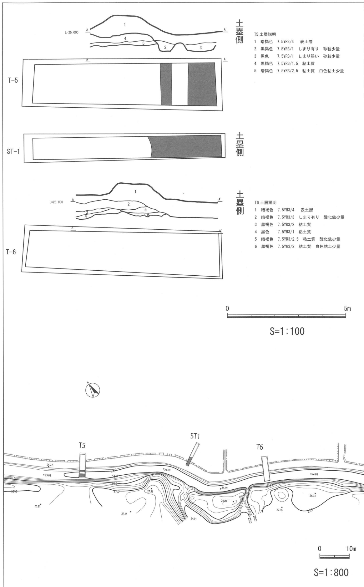
図7 トレンチ5,6平面及び断面図
