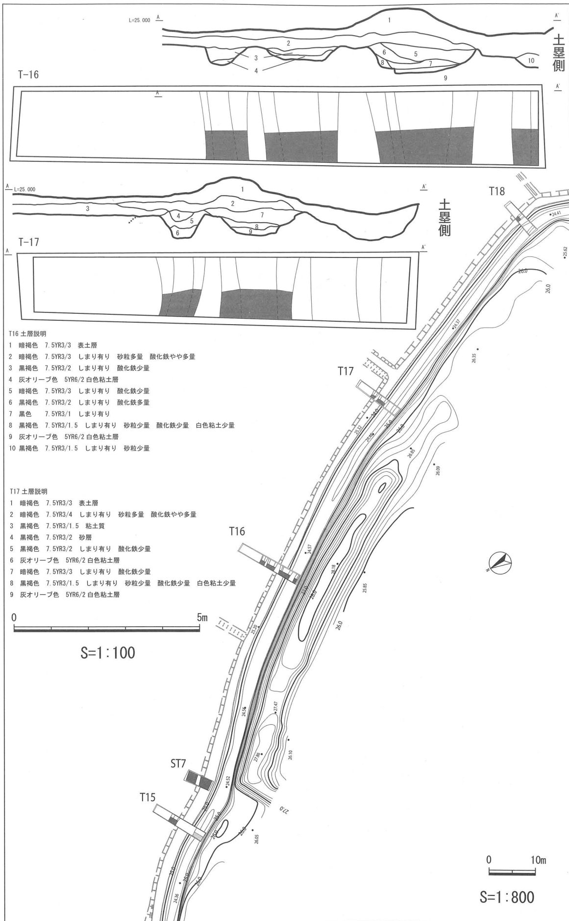
図13 トレンチ16, 17平面及び断面図
