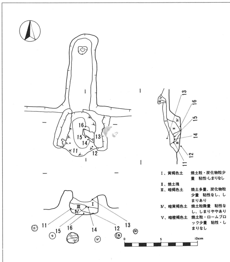
Fig 6 1号住居址カマド完掘状況
