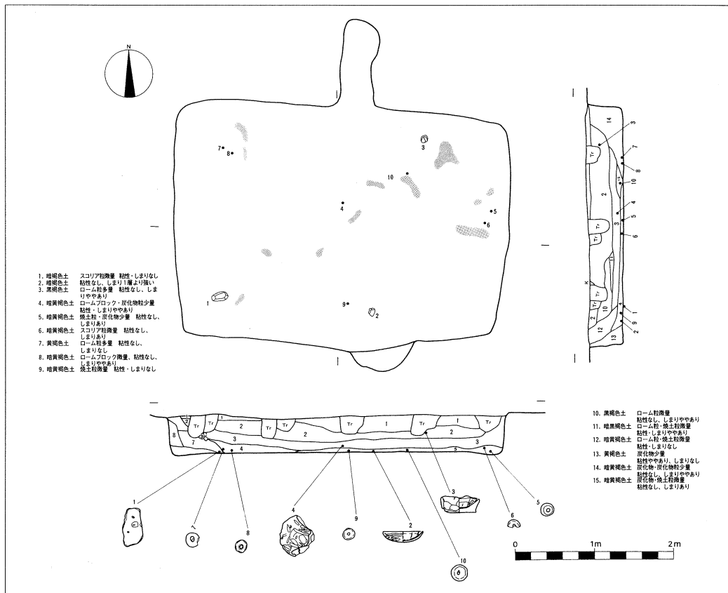
Fig 4 1号住居址遺物出土状況
