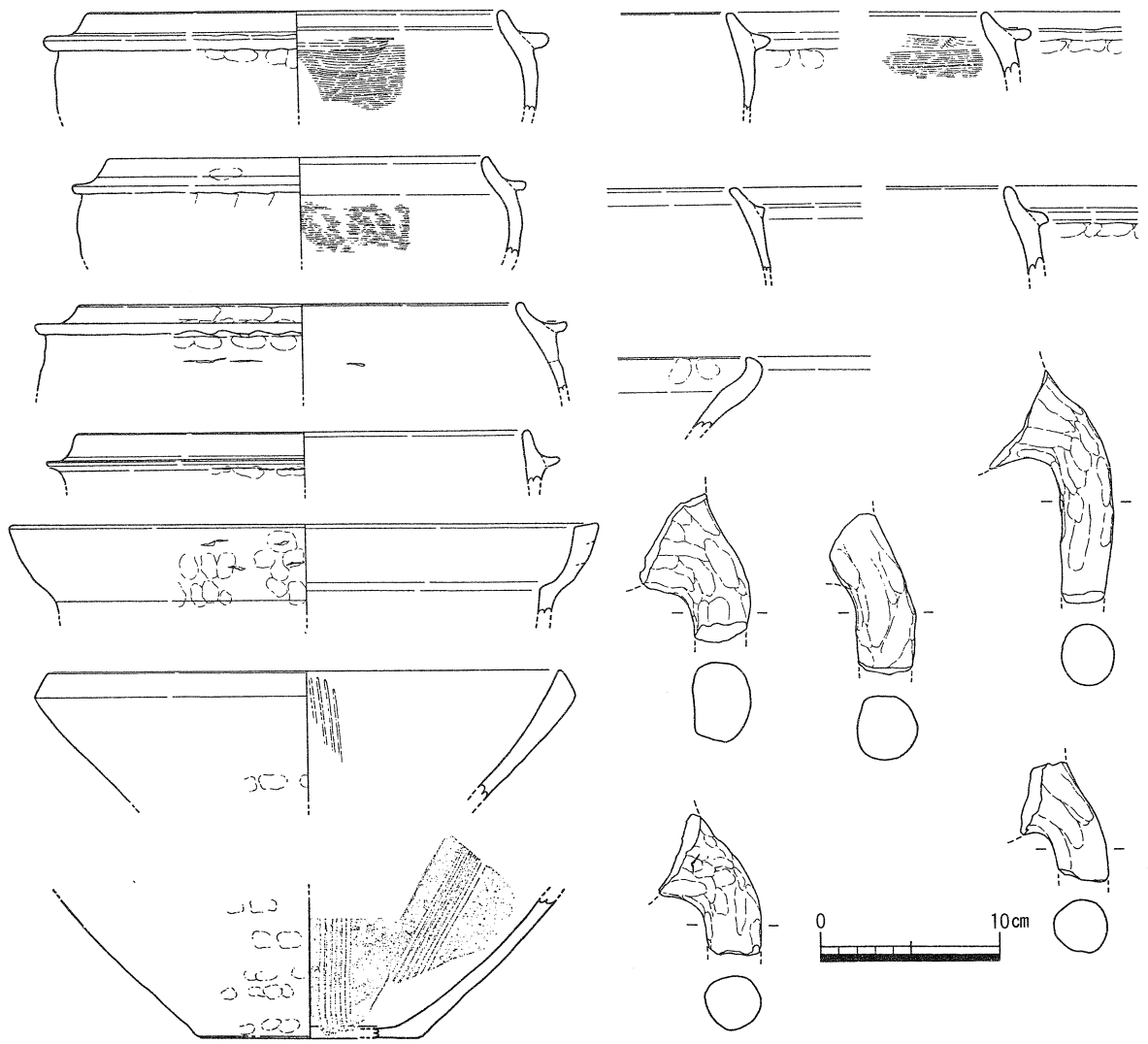
第32图 B区SX 02出土遺物実測図
