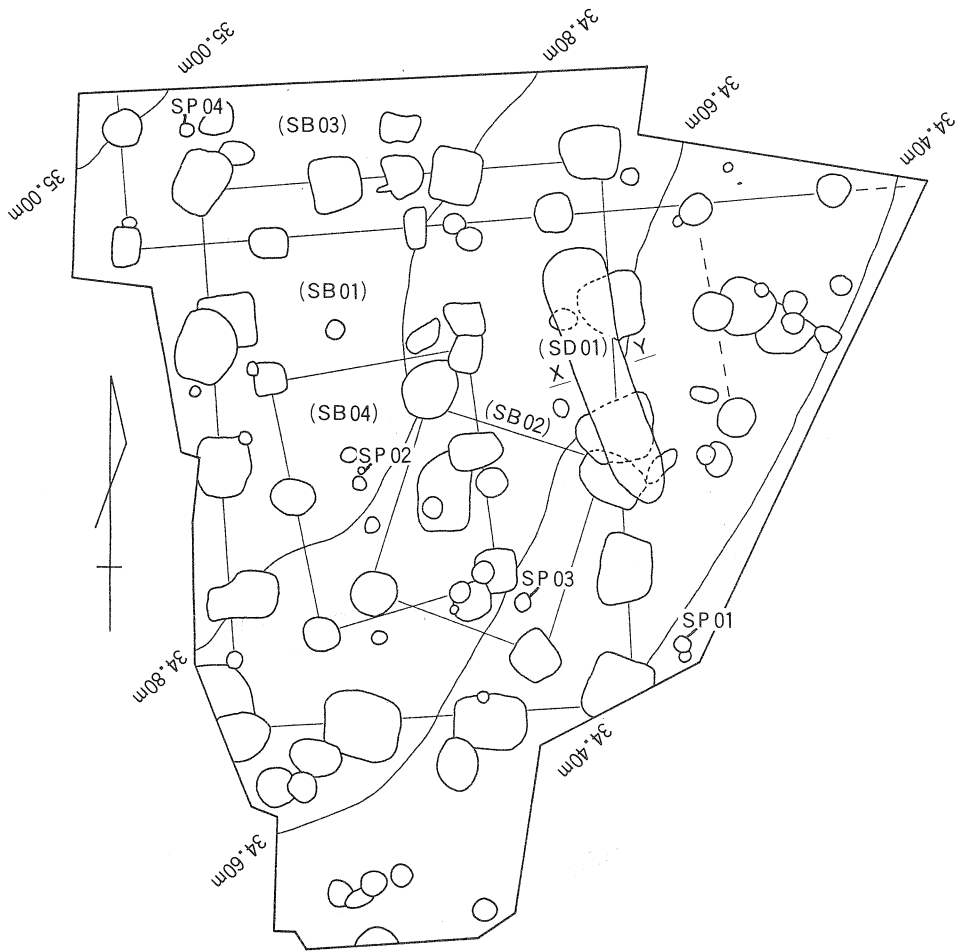
第34図 C区遺構配置図(S=1/100)
