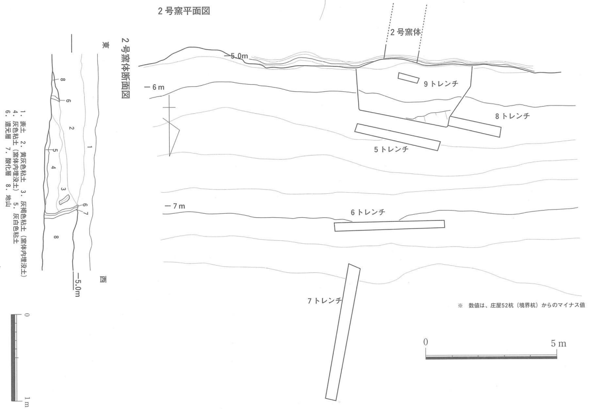
図28 1号窯及び2号窯平・断面図
