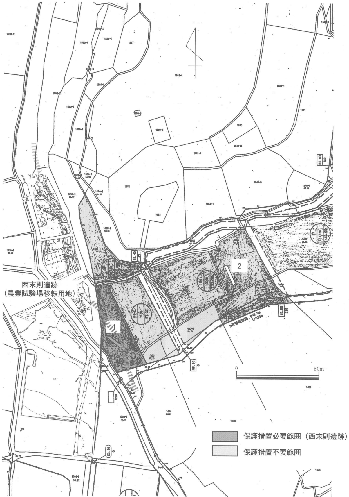
図33 トレンチ配置図 (山田地区)
