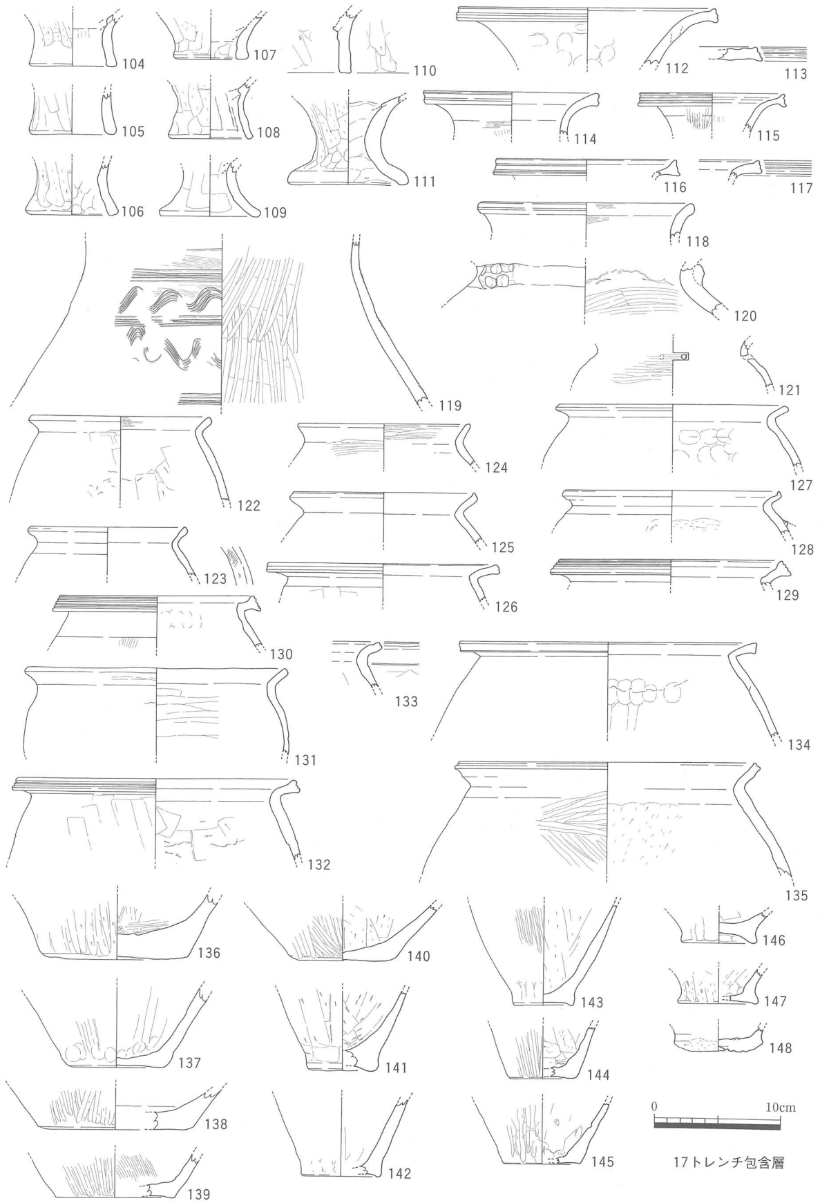
図22 出土遺物 その3
