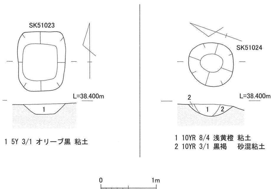
第21図 第1遺構面検出土坑平・断面図③
