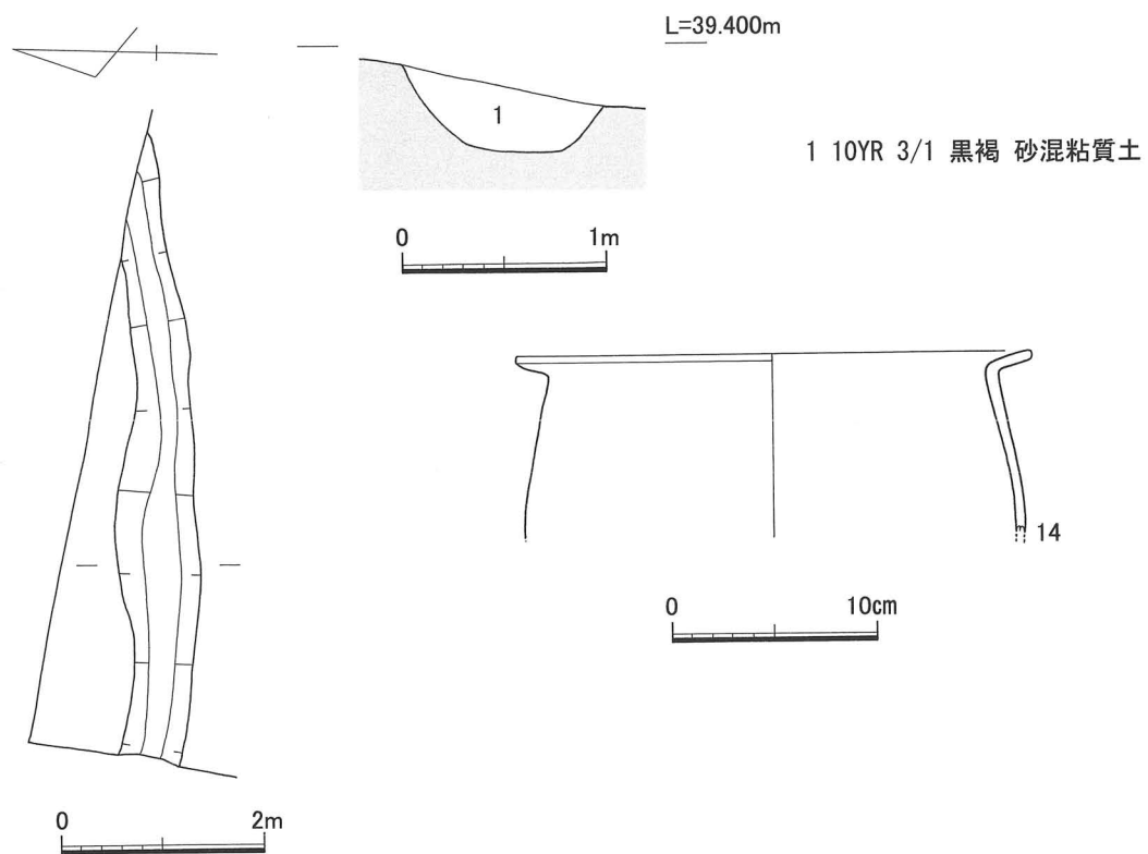
第12図 SD52003平・断面図及び出土遺物実測図
