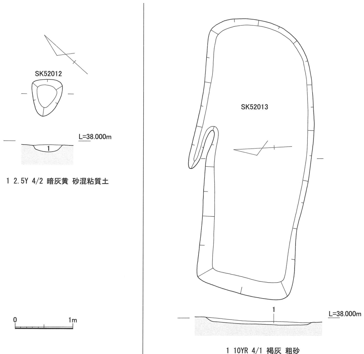
第10図 第2遺構面検出土坑平・断面図②
