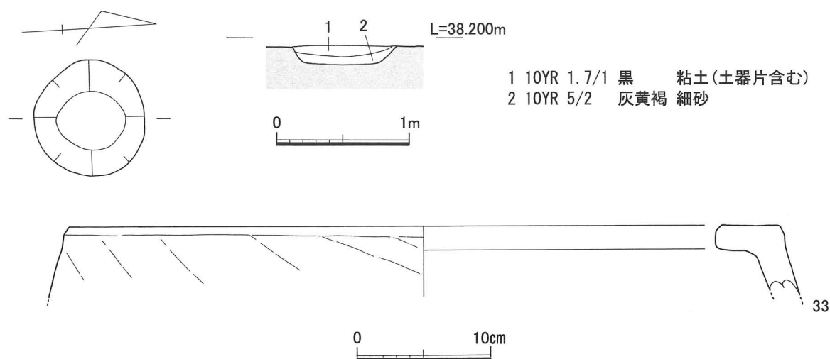
第20図 SK51019平・断面図及び出土遺物実測図
