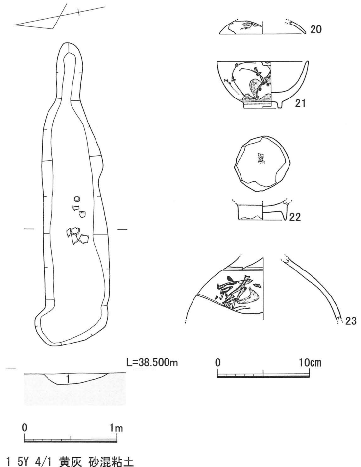
第16図 SK51014平・断面図及び出土遺物実測図
