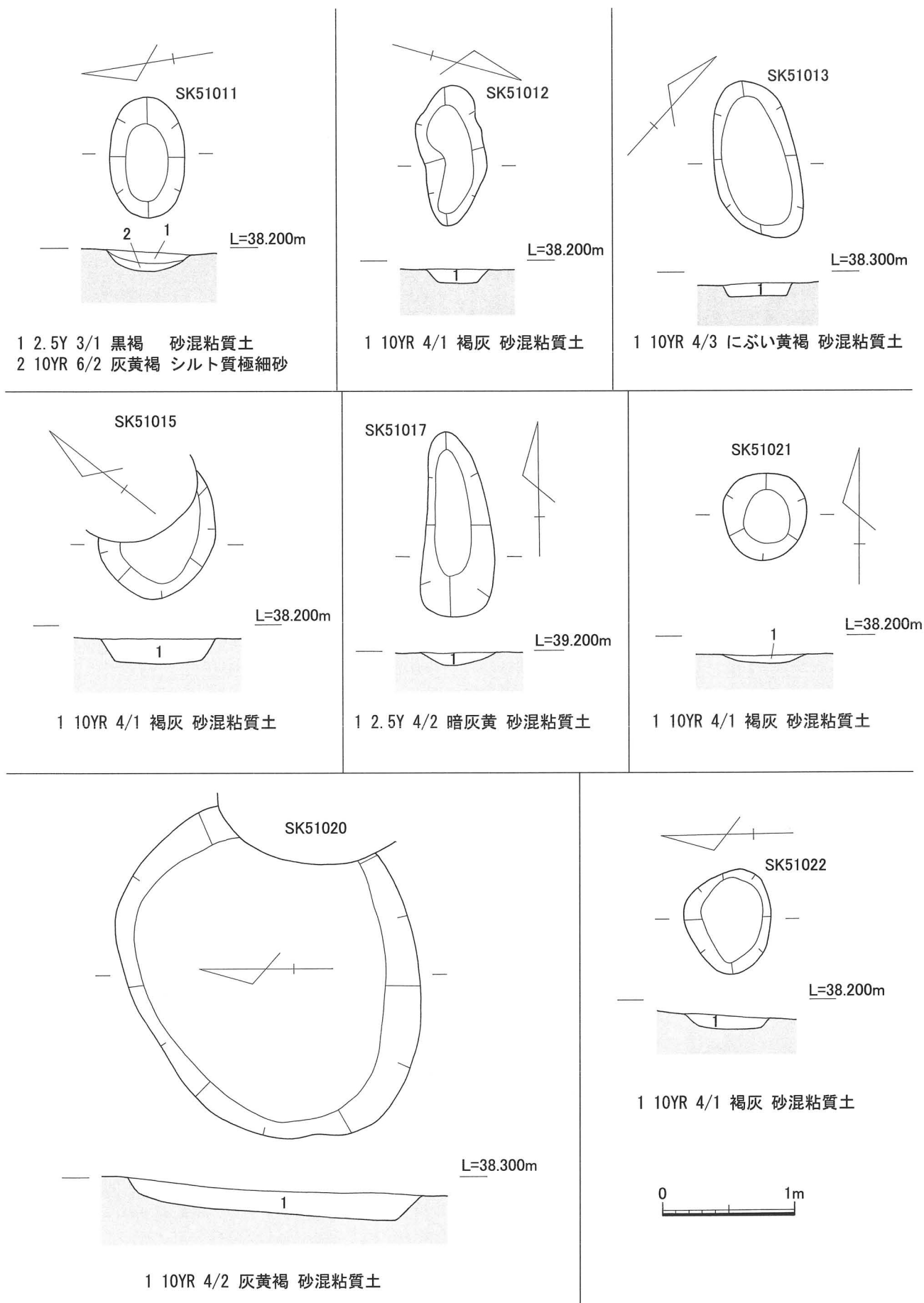
第15図 第1遺構面検出土坑平・断面図②
