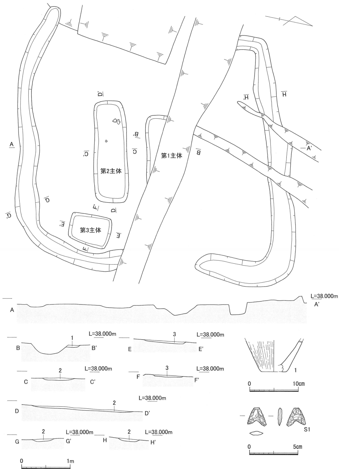
第6図 ST52001平・断面図及び出土遺物実測図
