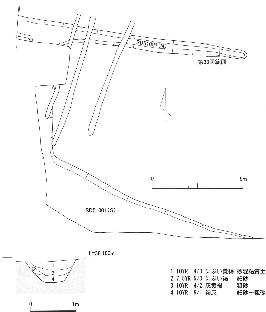
第28図 SD51001平・断面図
