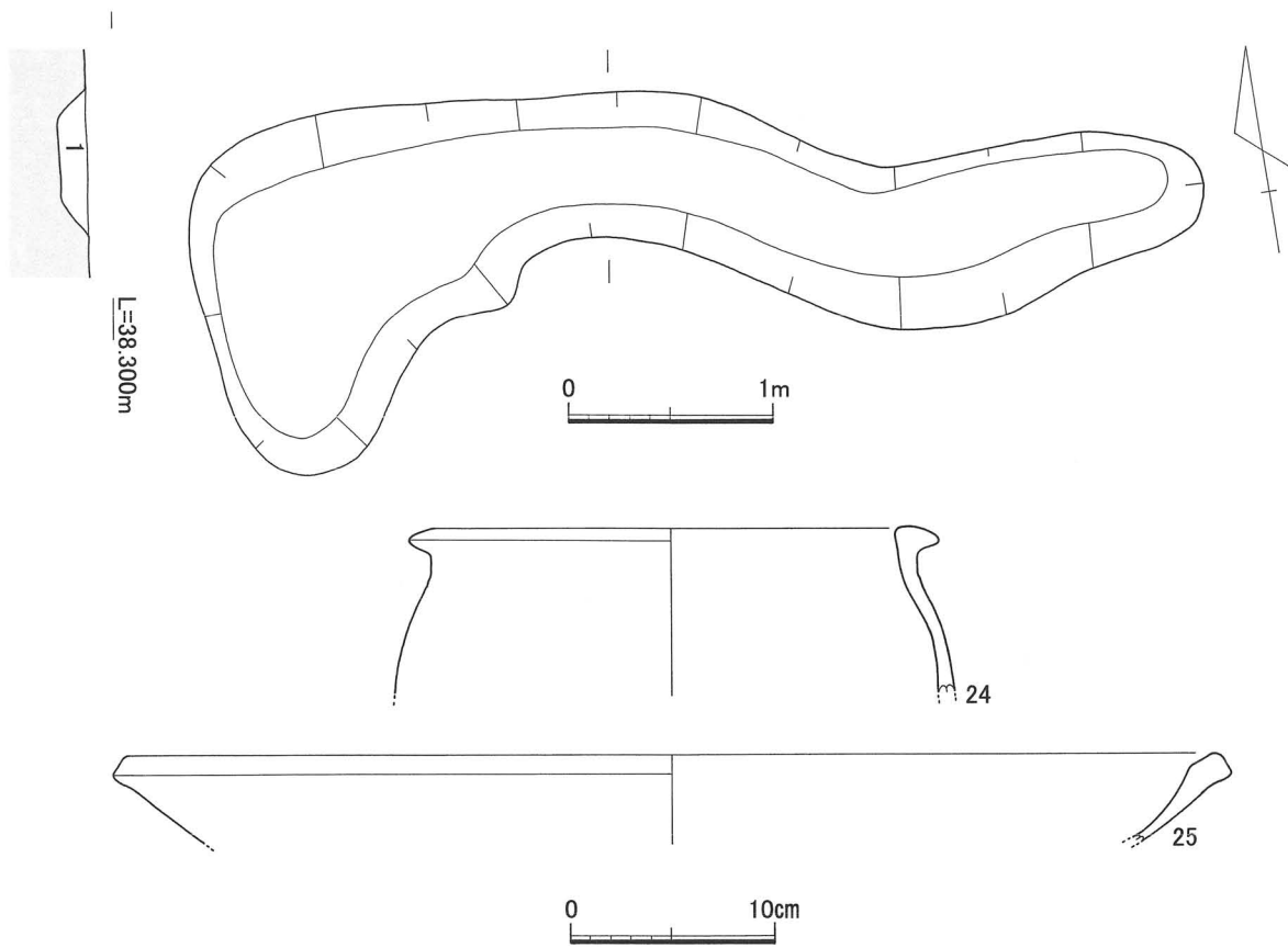
第17図 SK51016平・断面図及び出土遺物実測図
