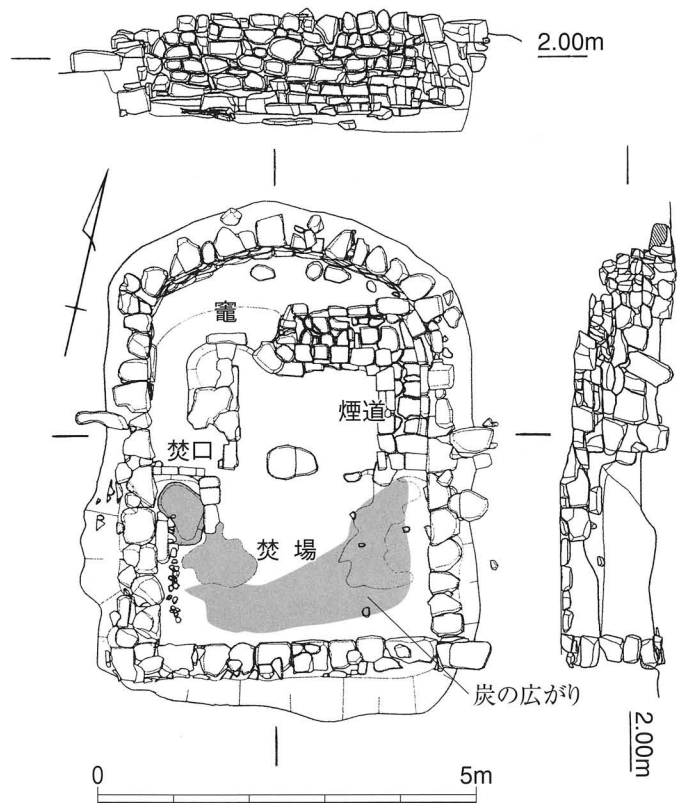
釜場Ⅱ平・立面図
