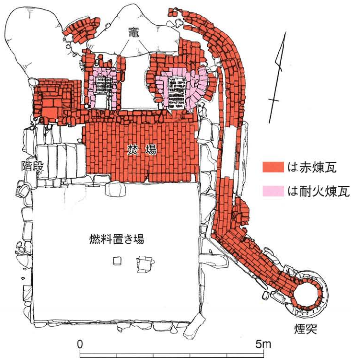
釜場Ⅰ平面図
