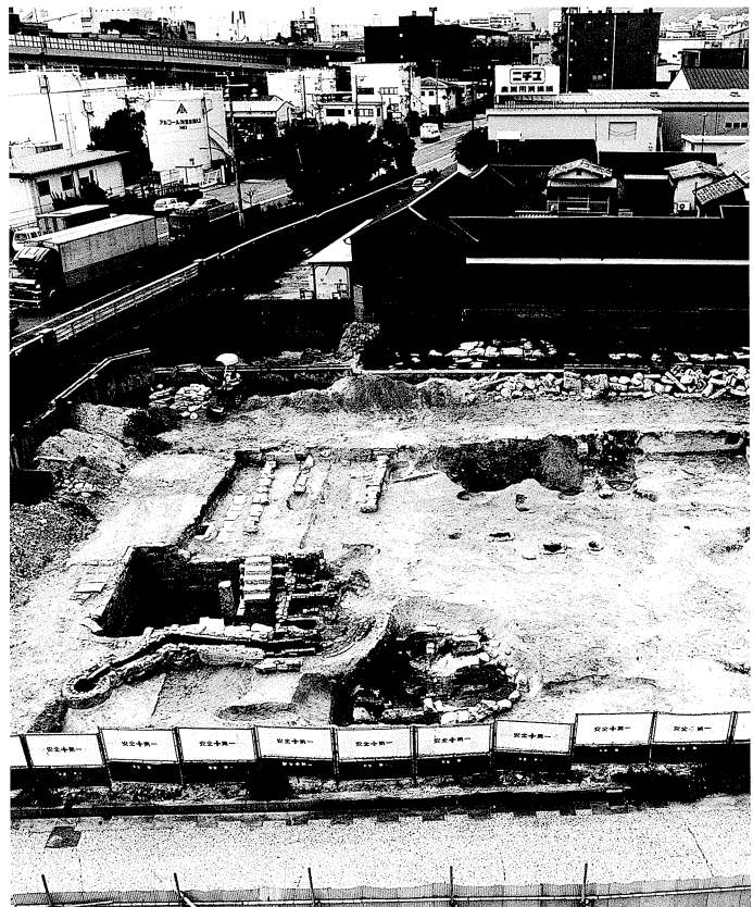
石屋乙蔵空中写真(東から)
