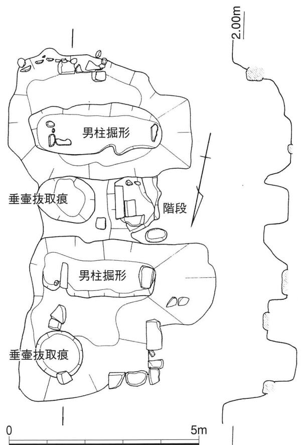
釜場Ⅲ平面図と断面図
