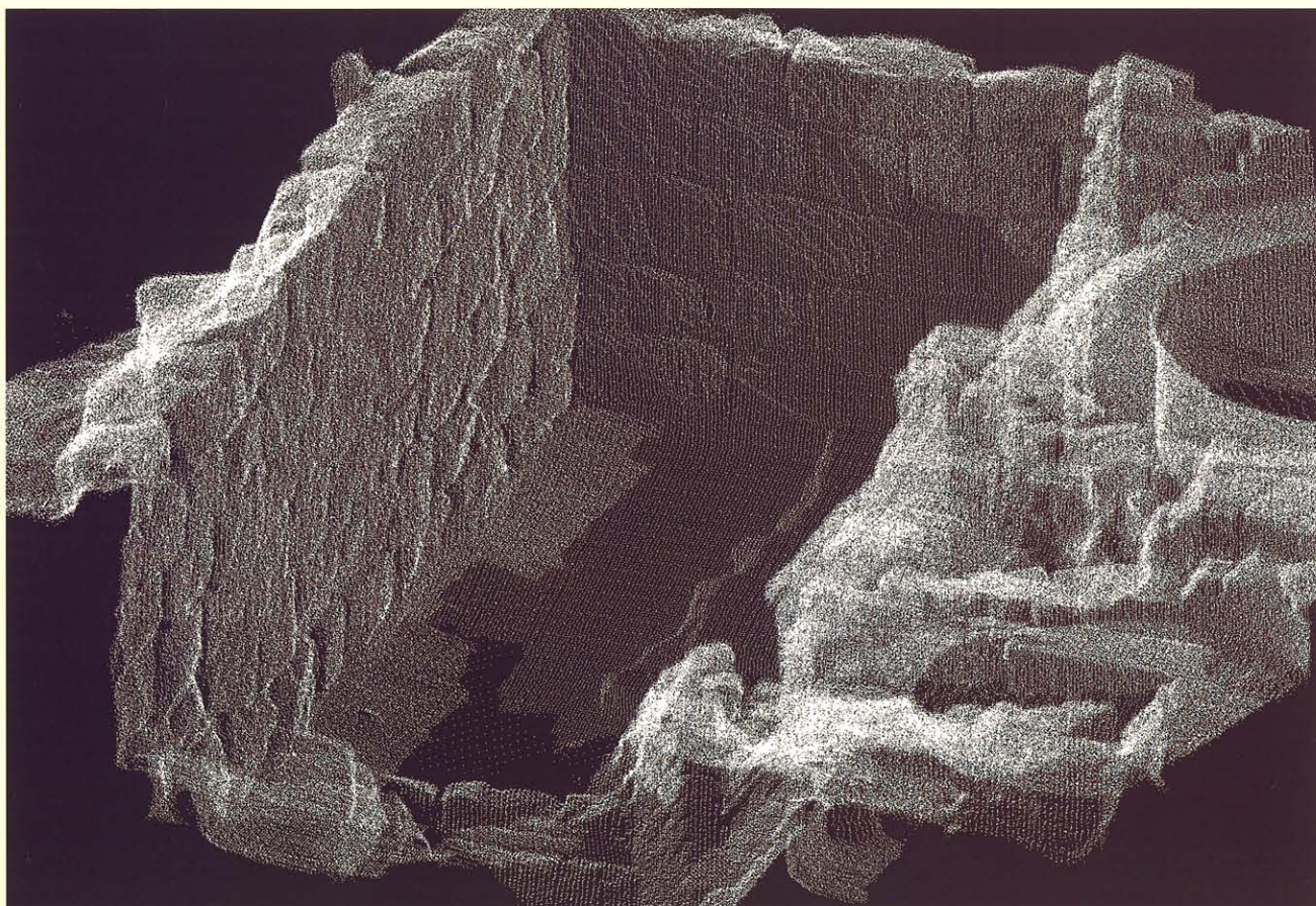
石屋甲蔵・釜場Ⅰの点群表現
