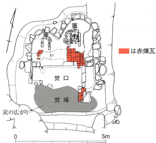
釜場Ⅱ平面図
