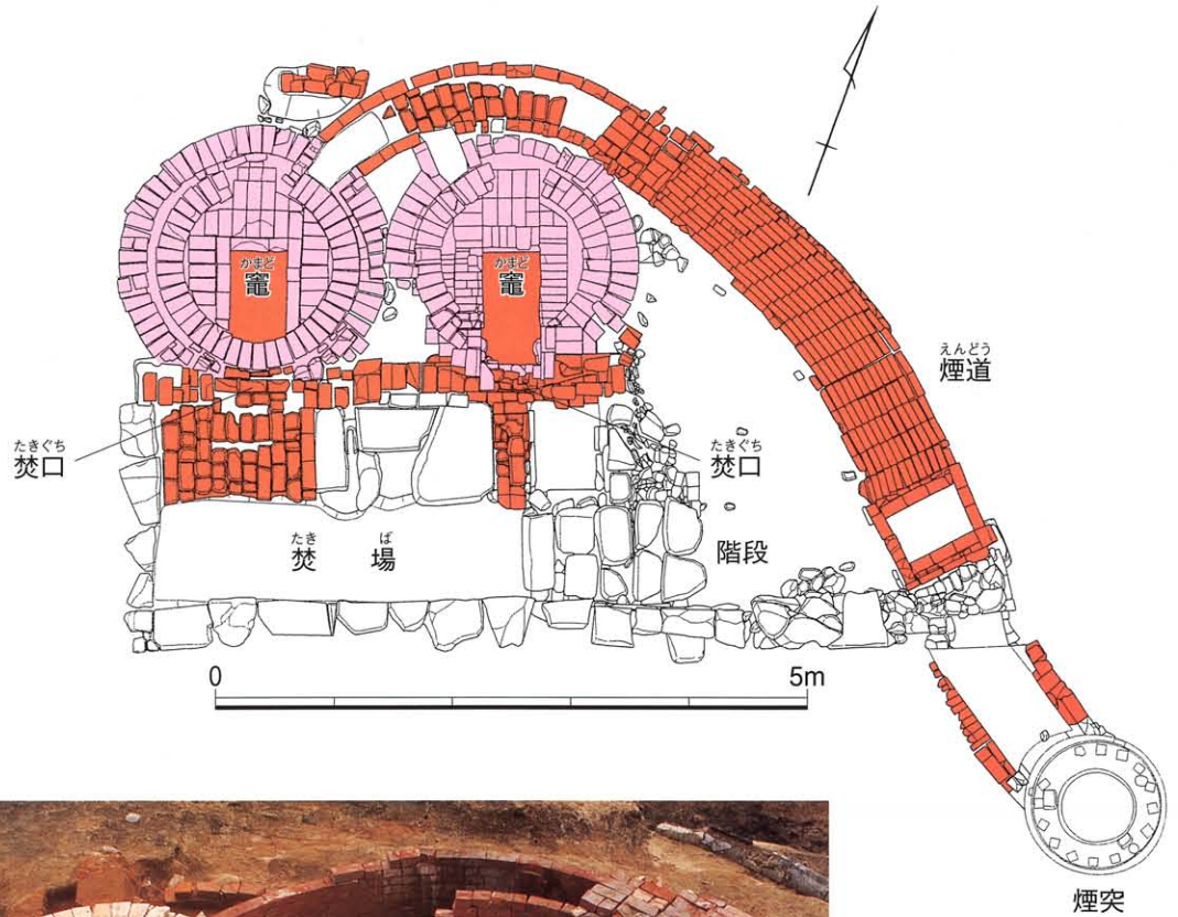
釜場 I 平面図
