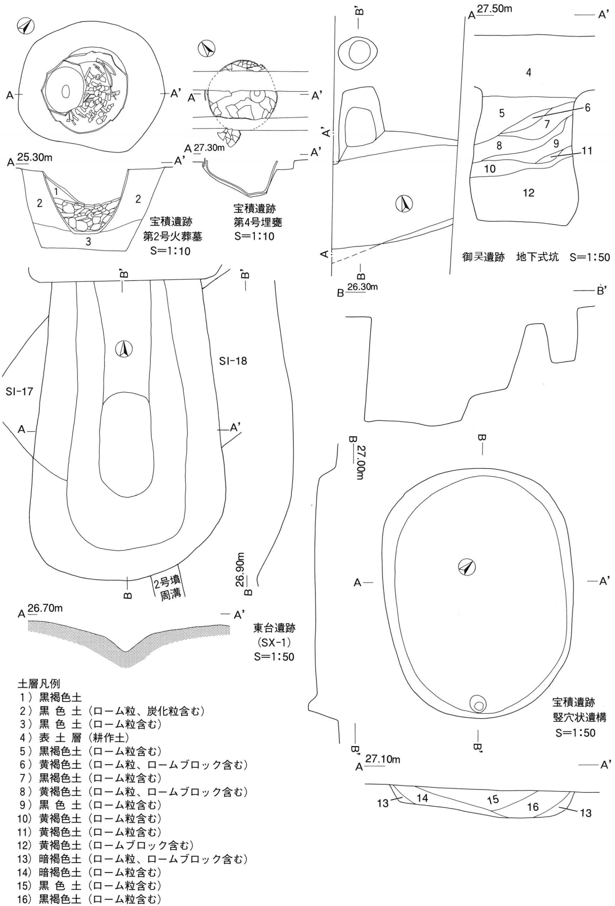
第143図 御灵遺跡遺構実測図2. 東台遺跡遺構実測図2. 宝積遺跡遺構実測図
