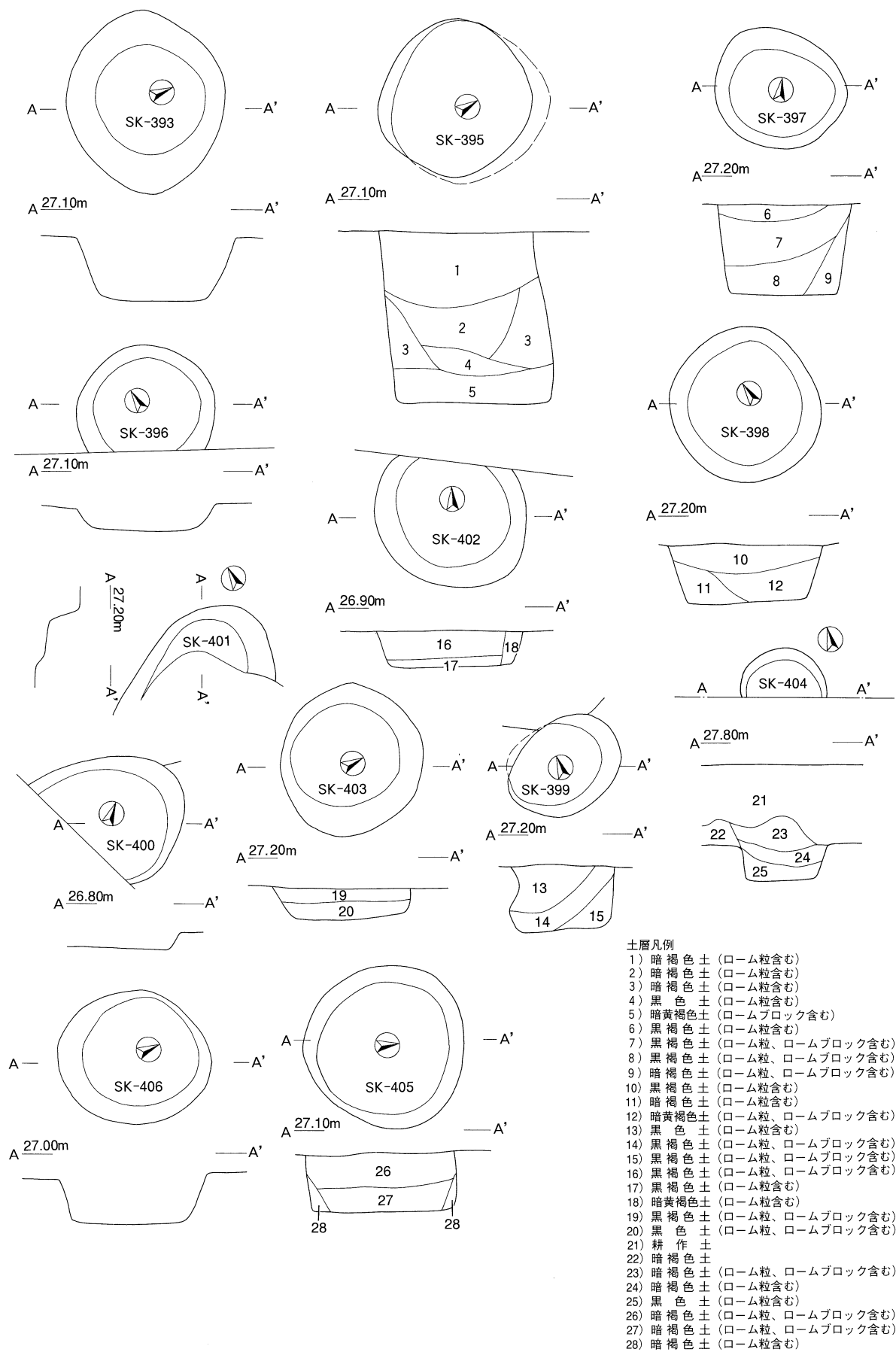
第164図 御霊遺跡土坑実測図13 (SK-393・394・395・396・397・398・399・400・401・402・403・404・405・406, S=1:50)
