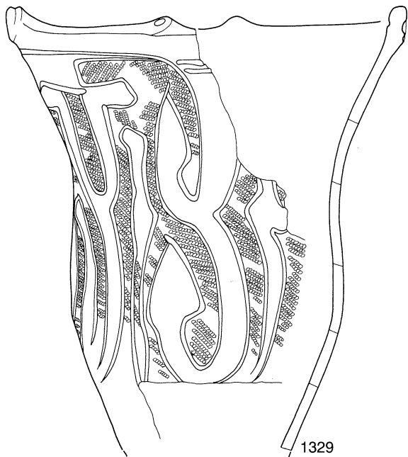
第240図 御霊遺跡住居跡・土坑出土遺物実測図1
