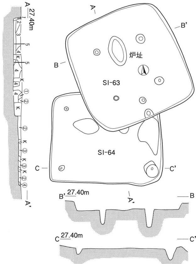
第63号・64号住居跡 (SI-63・64) 実測図
