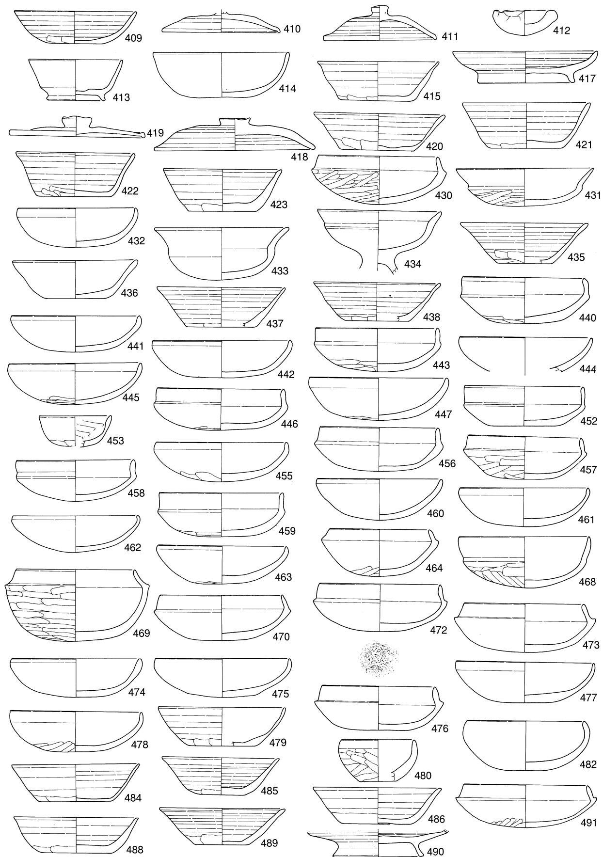
第190図 粉買場遺跡出土遺物実測図15 (No.409~491, S=1:4)
