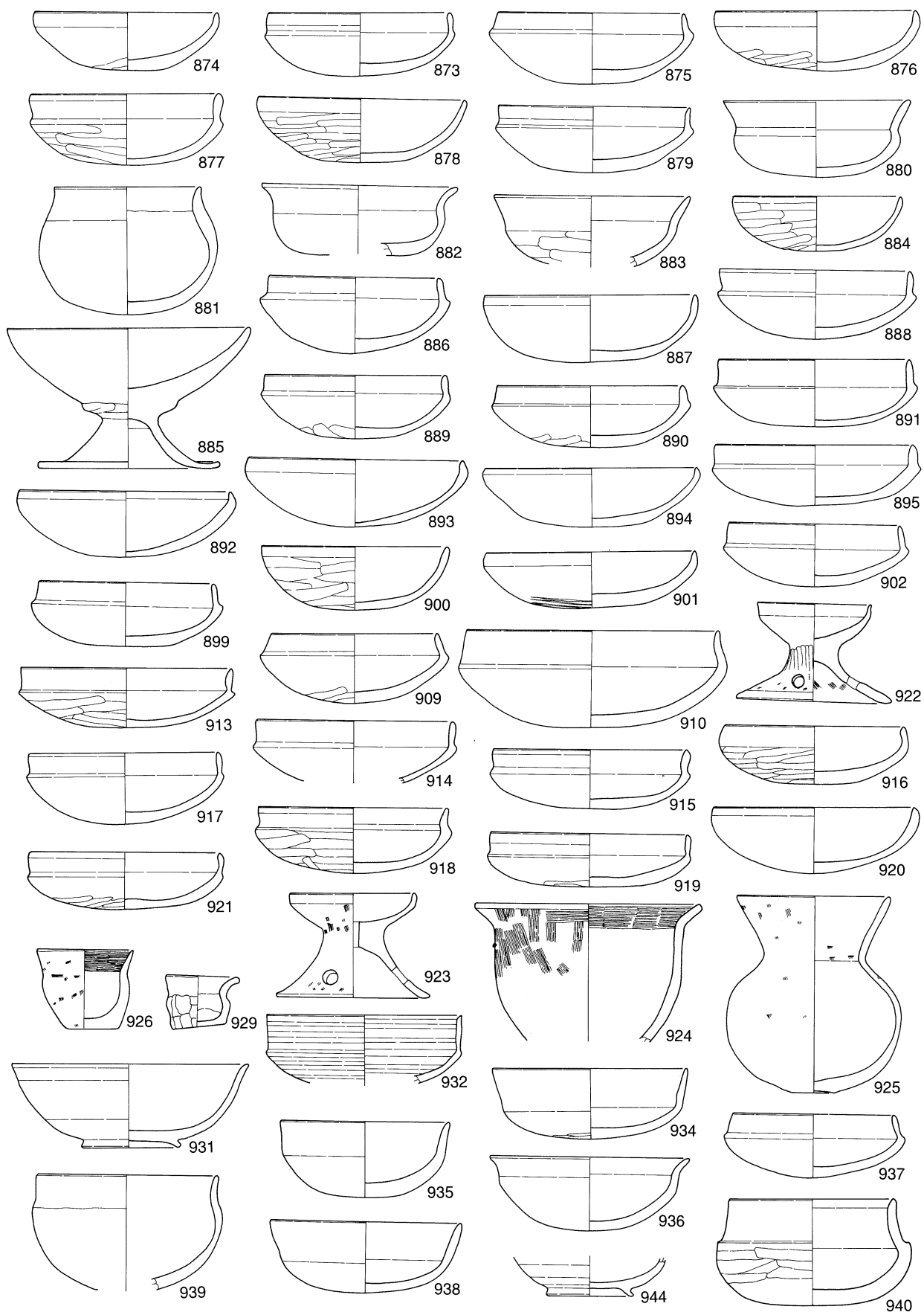
第 209 図 御灵遺跡出土遺物実測図 7 (No. 873 ~ 944, S = 1 : 4)
