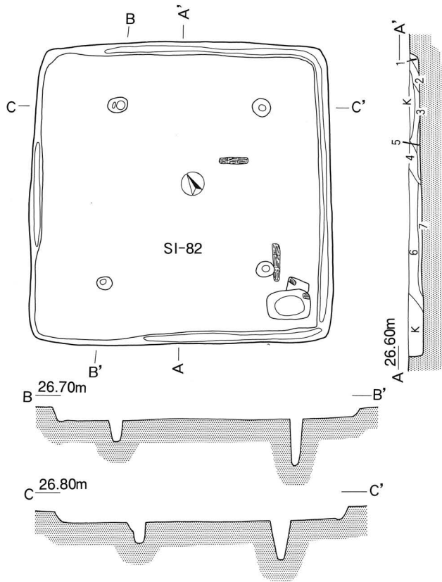
第82号住居跡 (SI-82) 実測図
