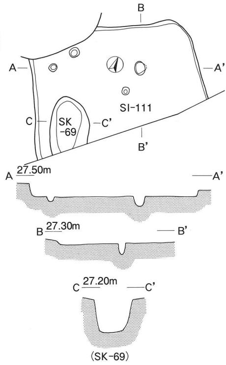
第111号住居跡, 第69号土坑 (SI-111, SK-69) 実測図
