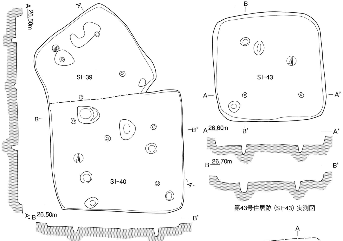
第39号・40号住居跡 (SI-39・40) 実測図
