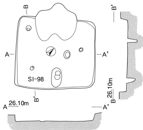
第98号住居跡 (SI-98) 実測図
