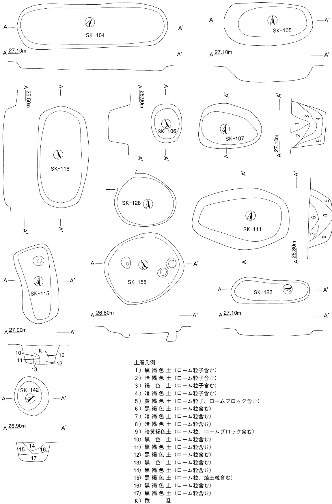
第169図 東台遺跡土坑実測図4 (SK-104・105・106・107・111・115・116・123・128・142・155, S=1:50)
