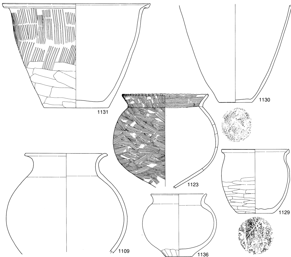
第220图 宝積遺跡出土遺物実測図6 (No.1109~1136, S=1:4)
