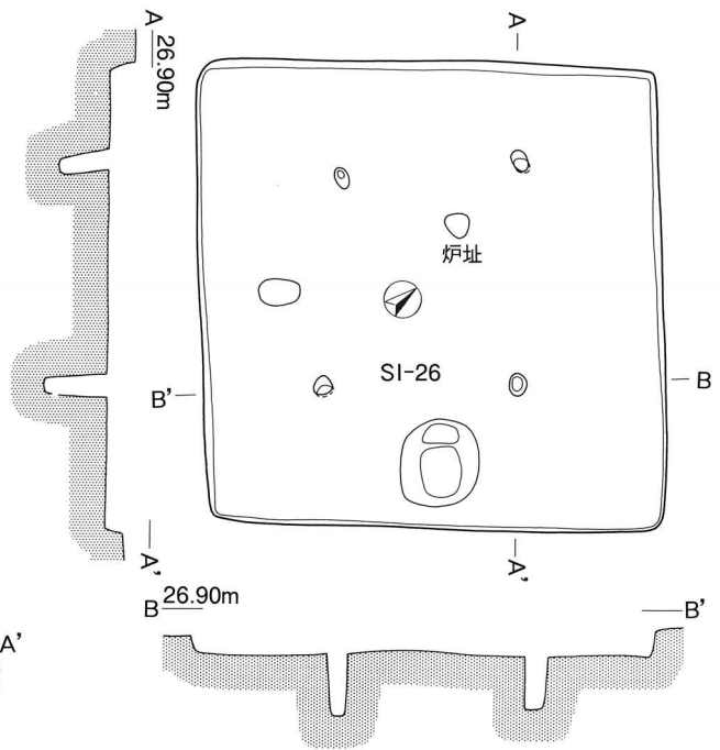
第26号住居跡 (SI-26) 実測図
