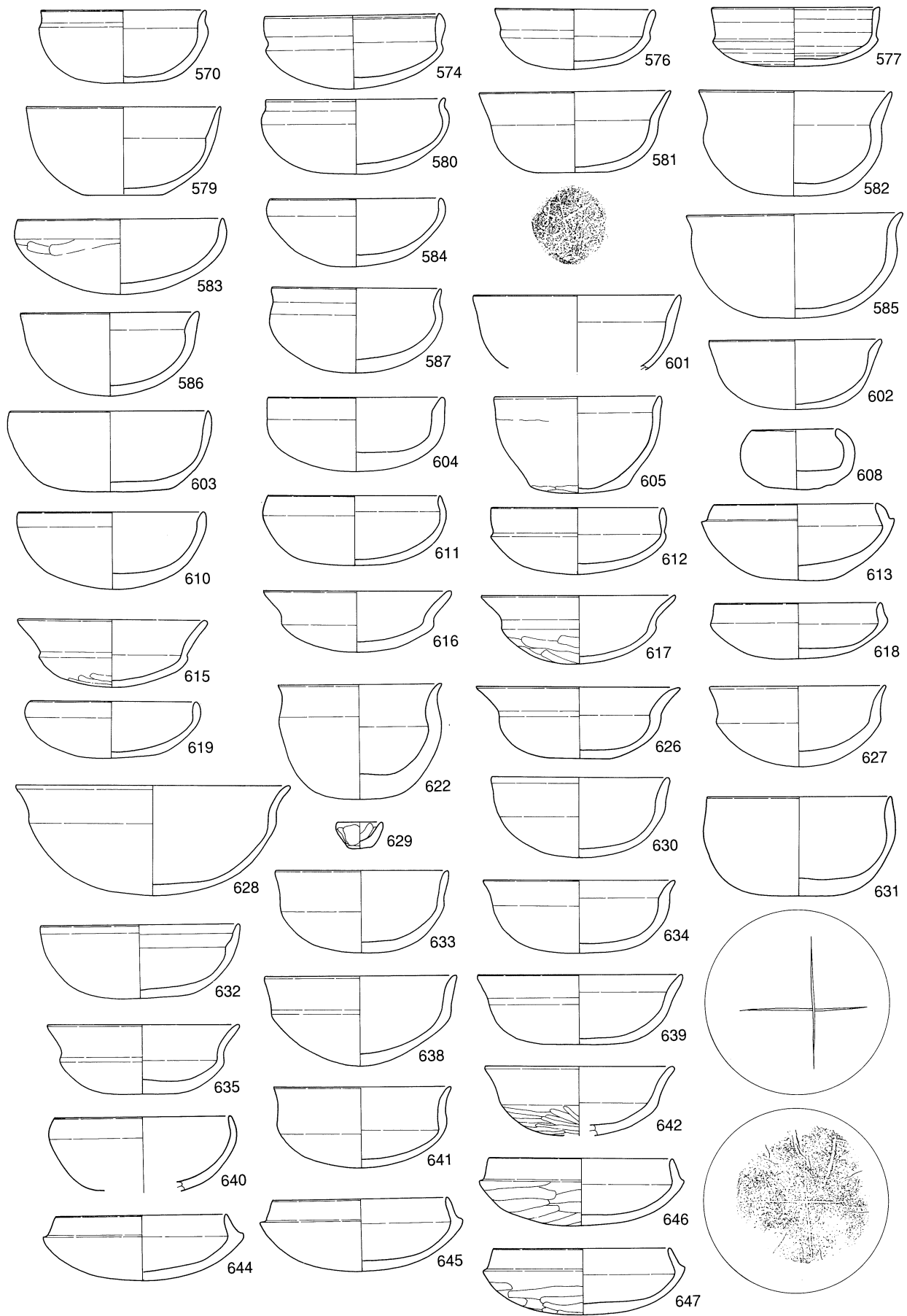
第 196 図 粉買場遺跡出土遺物実測図 21 (No. 570 ~ 647, S = 1 : 4)
