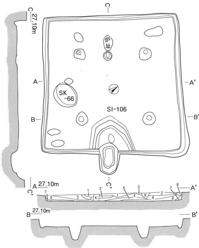
第106号住居跡 (SI-106) 実測図
