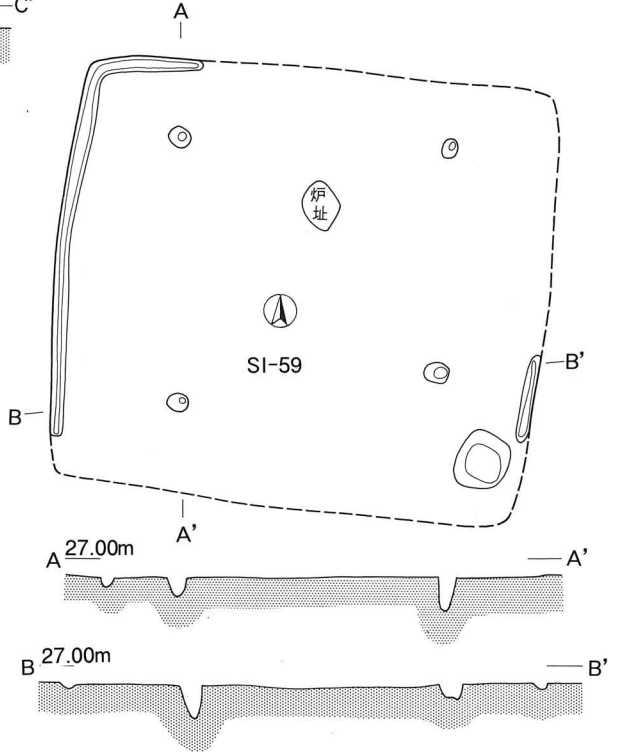
第59号住居跡 (SI-59) 実測図
