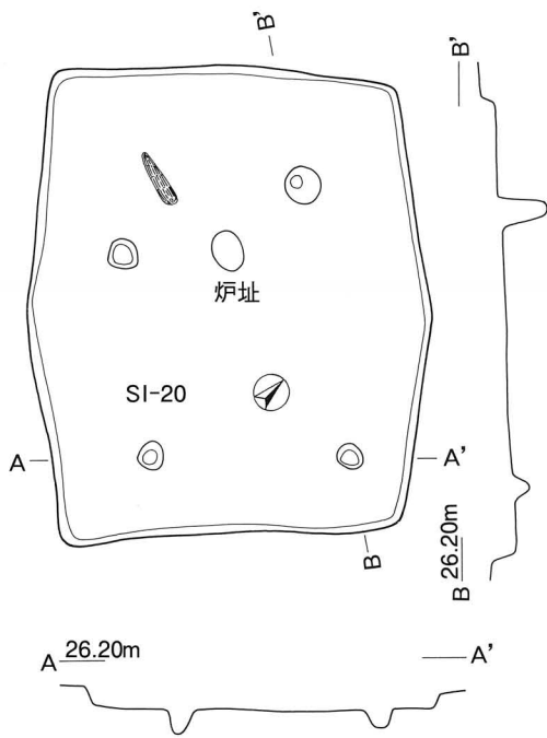
第20号住居跡 (SI-20) 実測図
