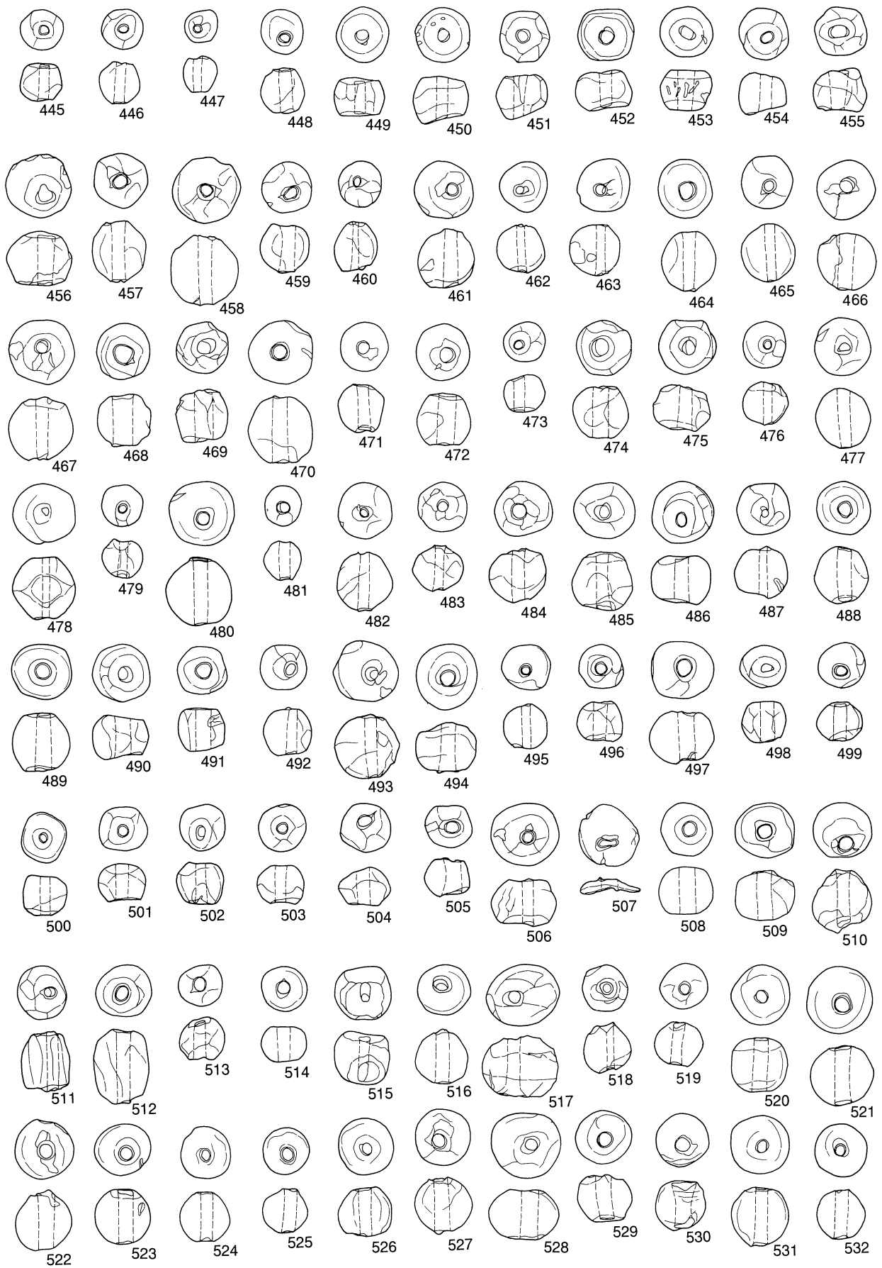
第 233 图 木田余台遺跡群出土土玉実測図 5 (S = 1 : 3)
