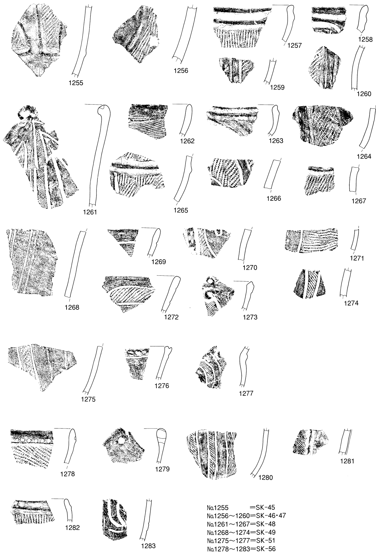
第 237 図 粉買場遺跡土坑出土遺物実測図 2 (S = 1 : 4)
