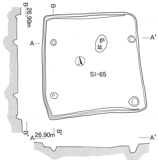
第65号住居跡 (SI-65) 実測図
