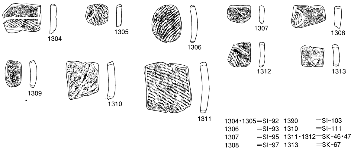
第 239 図 粉買場遺跡出土土器片錘実測図 (S = 1 : 4)
