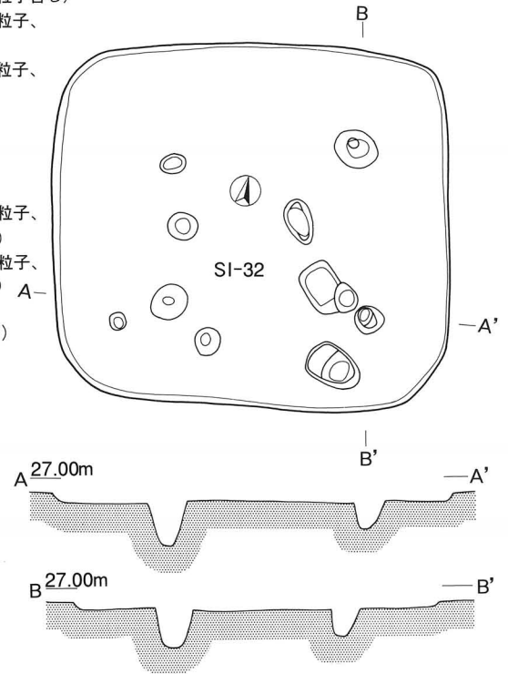
第32号住居跡 (SI-32) 実測図
