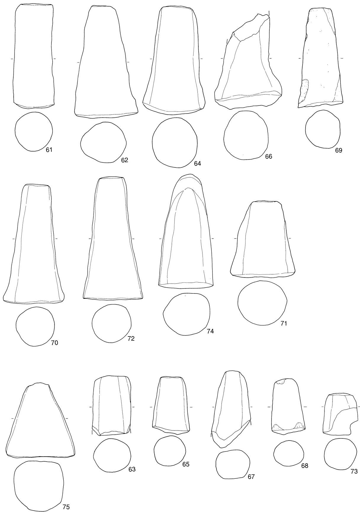
第228图 木田余台遺跡群出土遺物実測図5 (No.61~75, S=1:4)
