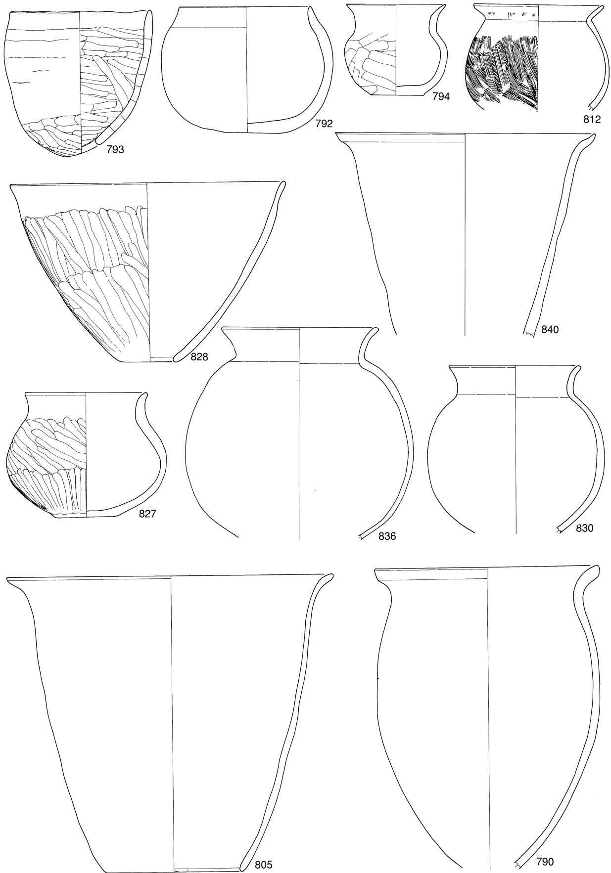
第205図 御灵遺跡出土遺物実測図3 (No.790~840, S=1:4)
