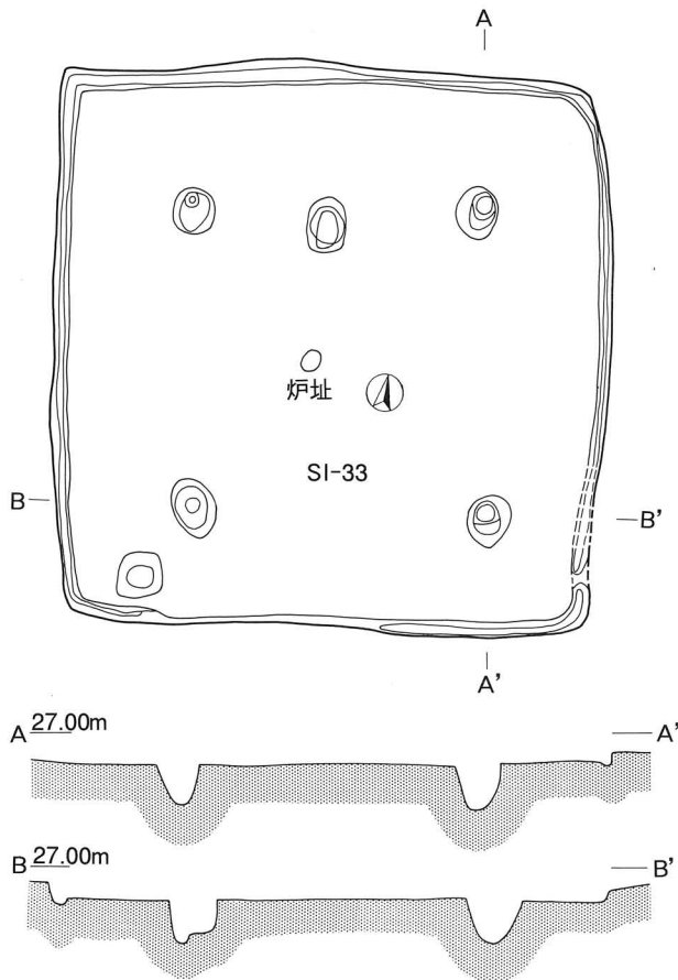
第33号住居跡 (SI-33) 実測図
