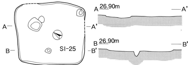
第25号住居跡 (SI-25) 実測図
