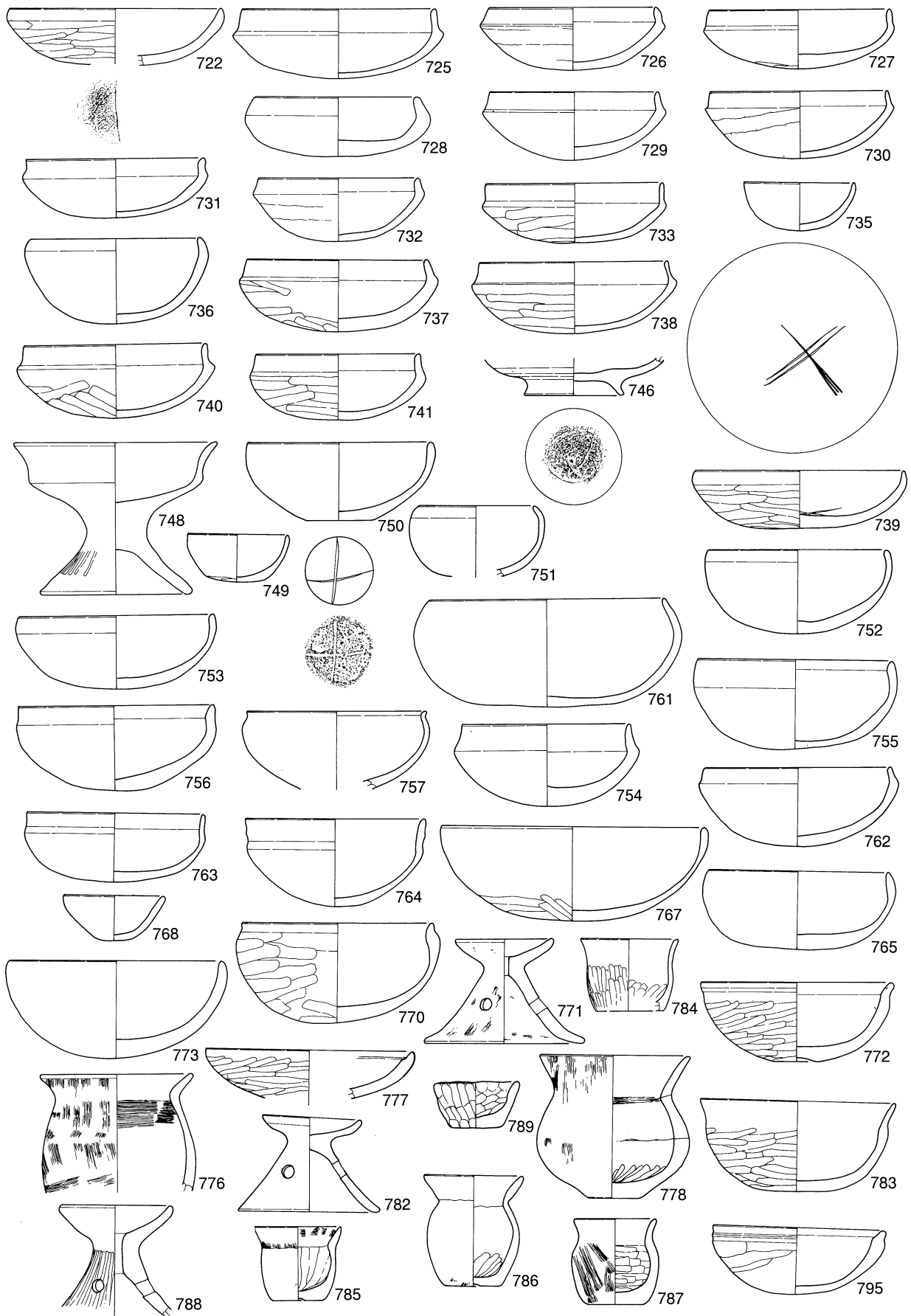
第 203 図 粉買場遺跡出土遺物実測図 28 (No.722 ~ 768, S = 1 : 4). 御灵遺跡出土遺物実測図 1 (No.770 ~ 789, S = 1 : 4)
