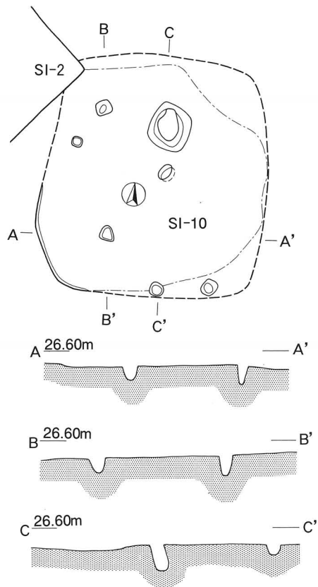
第10号住居跡 (SI-10) 実測図
