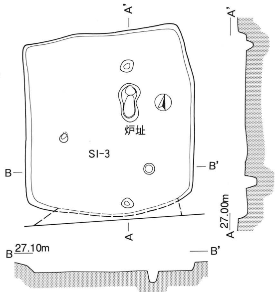
第3号住居跡 (SI-3) 実測図
