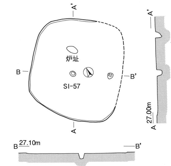
第57号住居跡 (SI-57) 実測図
