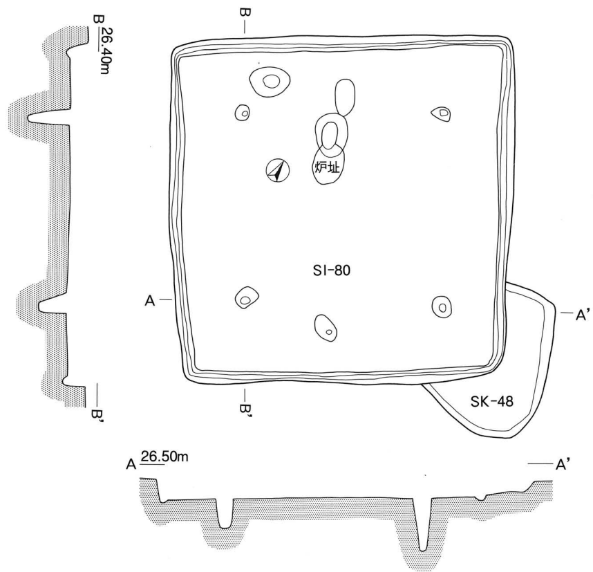
第80号住居跡, 第48号土坑 (SI-80, SK-48) 実測図
