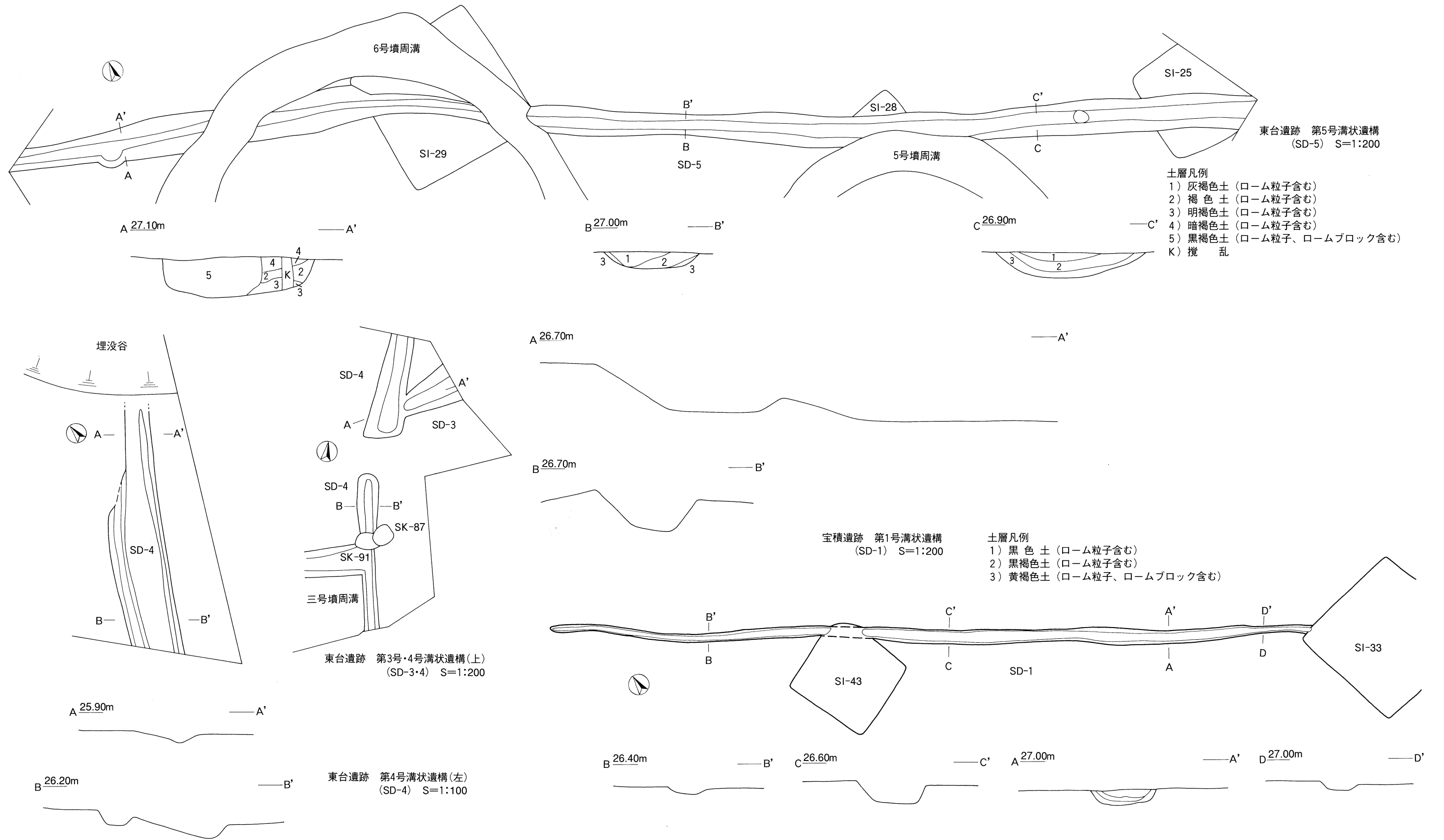
第140図 東台・宝積遺跡溝状遺構実測図 (S.L., E.L. S=1:40)
