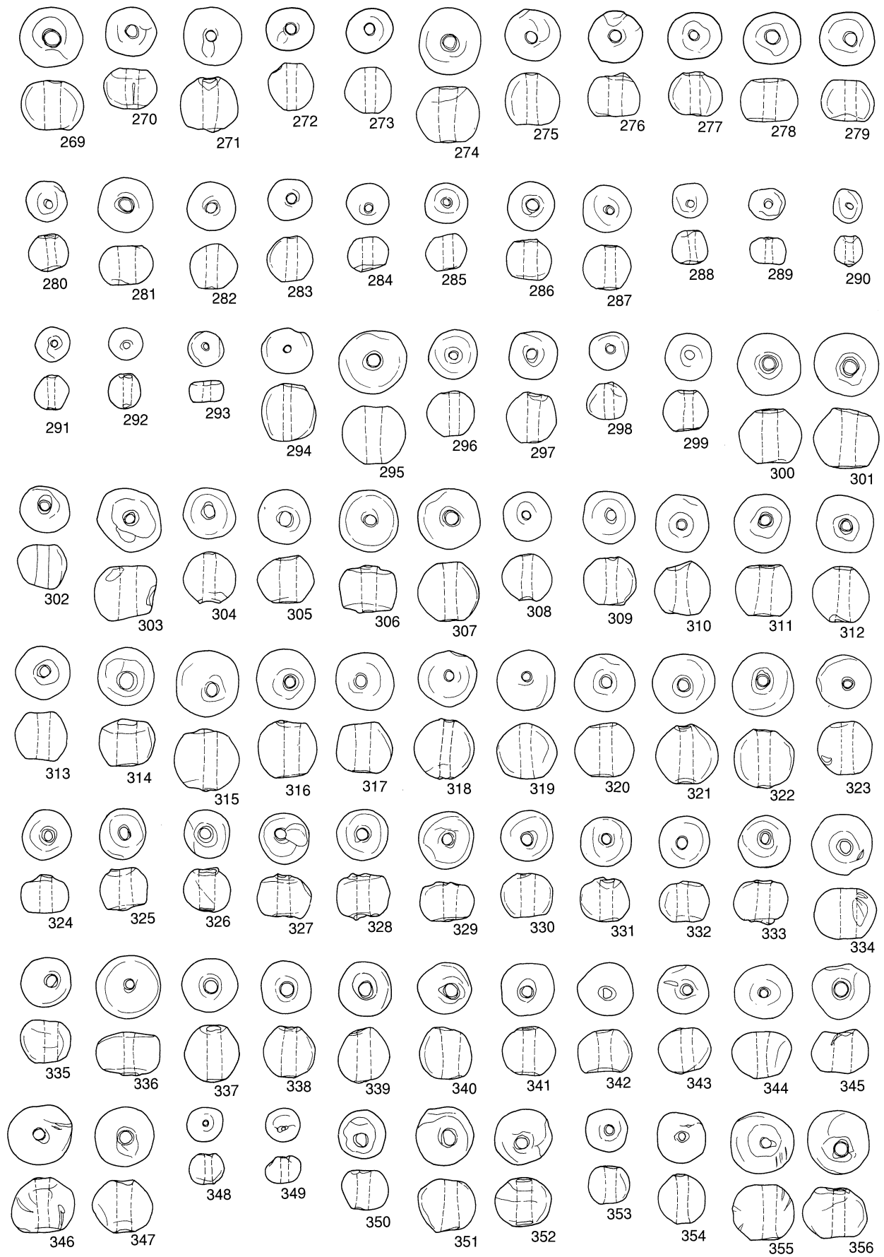
第 231 図 木田余台遺跡群出土土玉実測図 3 (S = 1 : 3)
