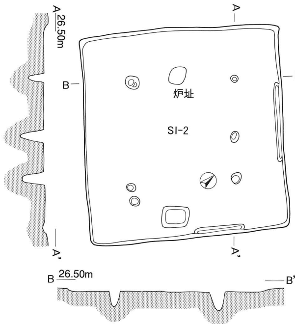
第2号住居跡 (SI-2) 実測図
