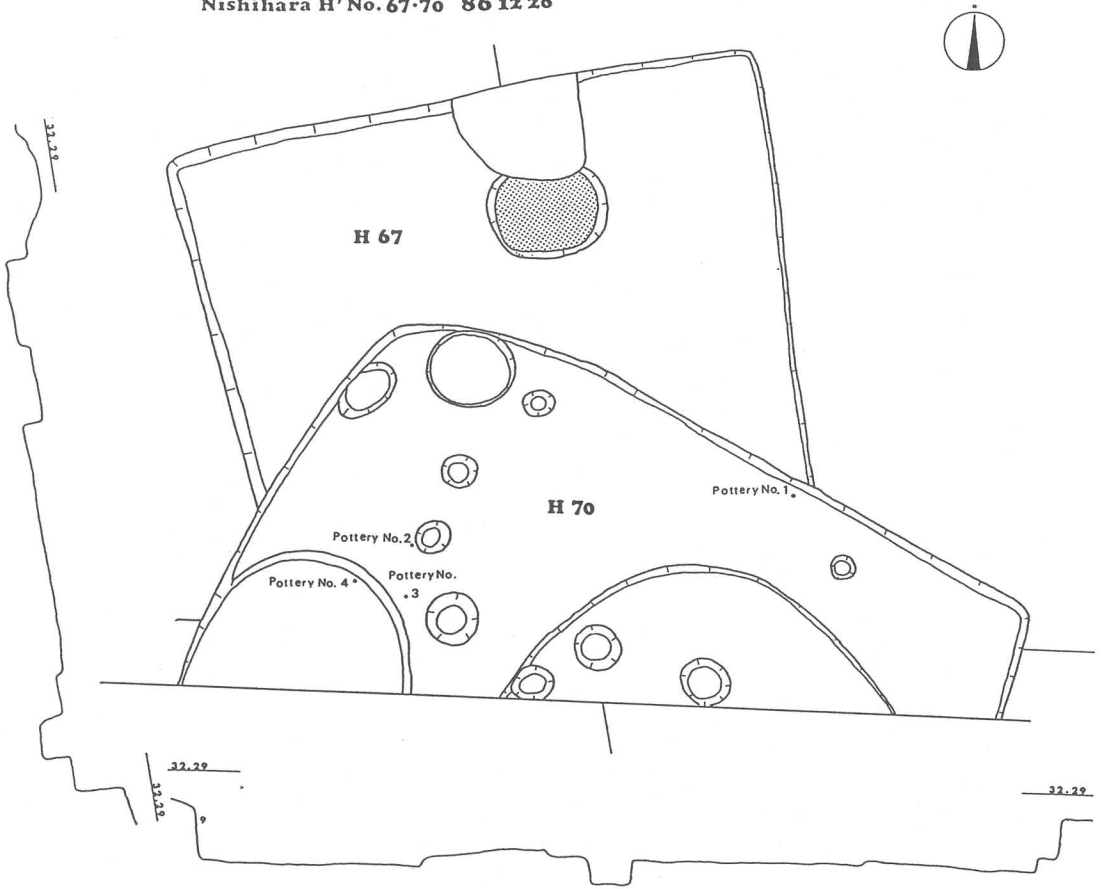
第24図 第67号住居実測図
