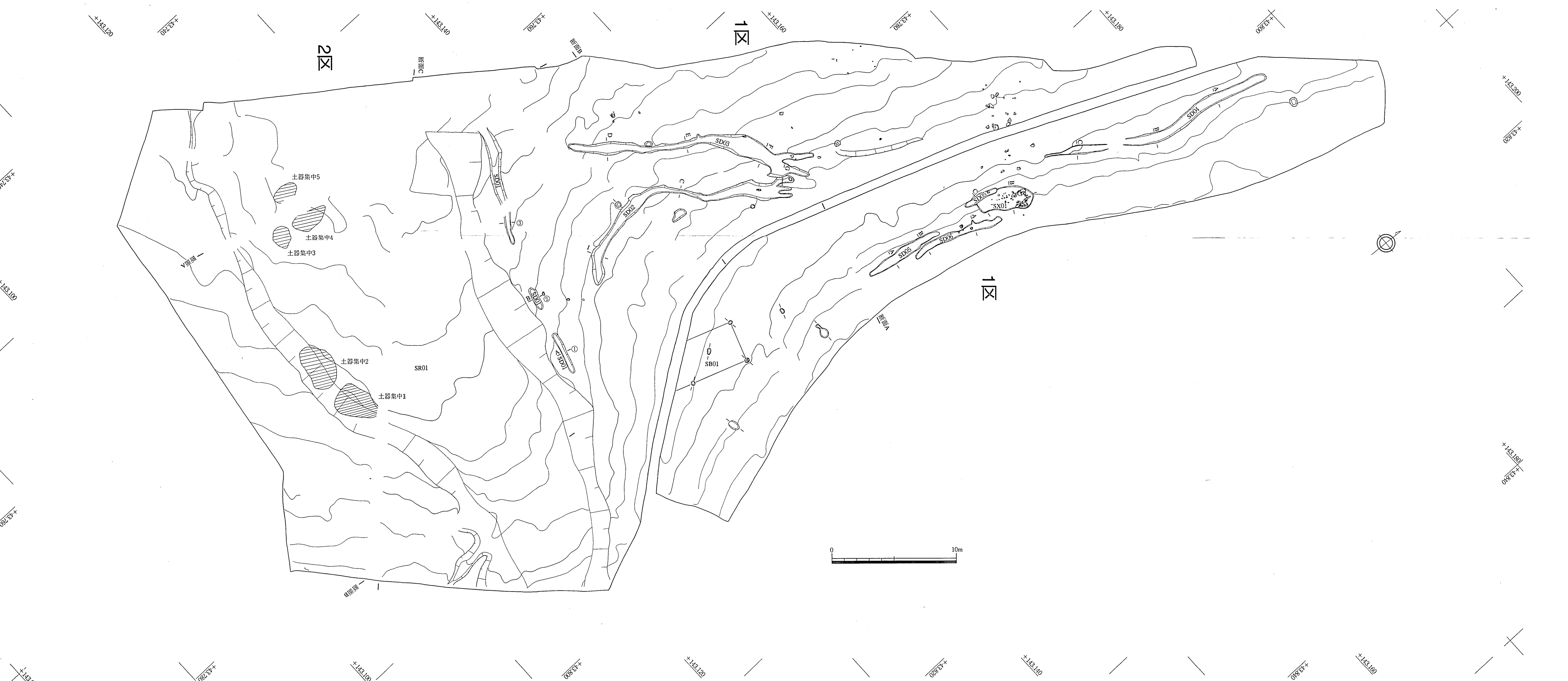
付図1 国分寺六ツ目遺跡・遺構配置図(1) (1/200)
