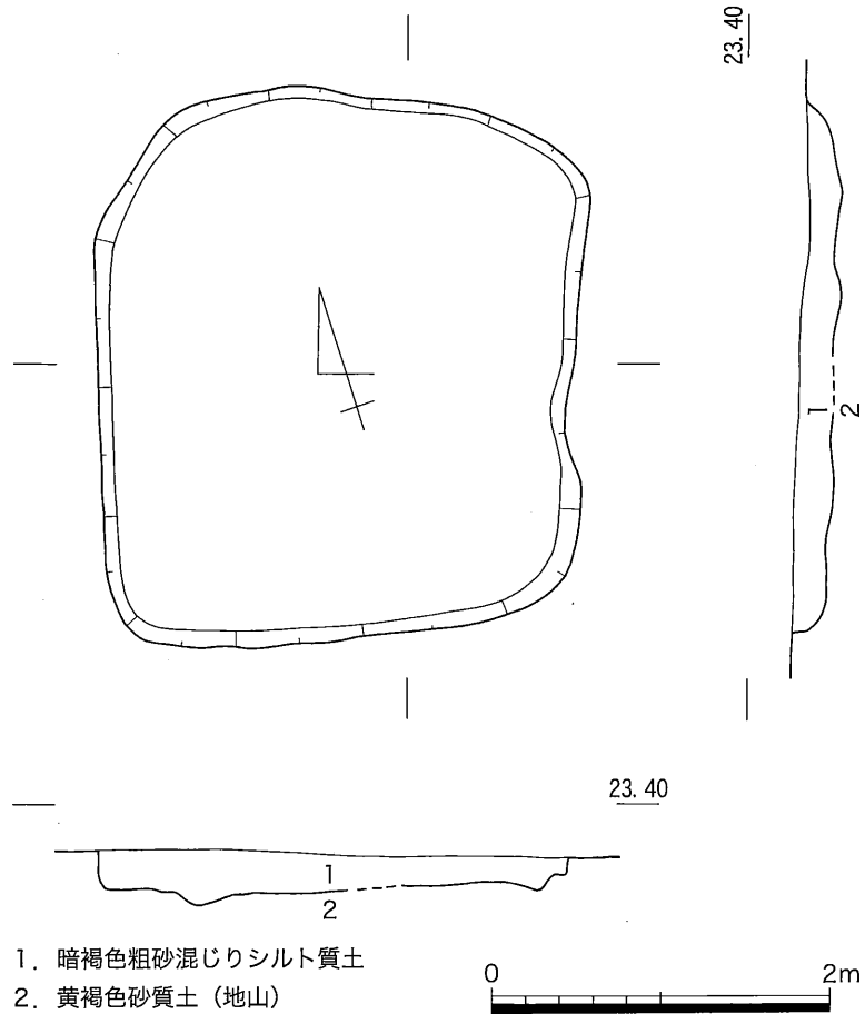
第16図 SH02 平・断面図 (1/50)
