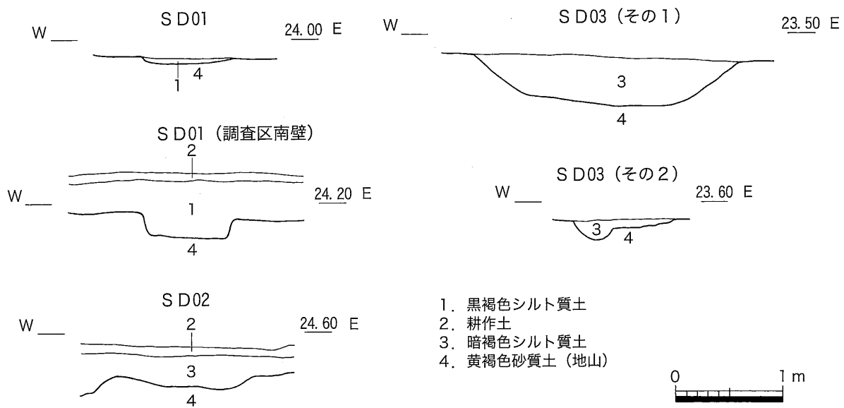
第63図 S D01~03 断面図 (1/50)
