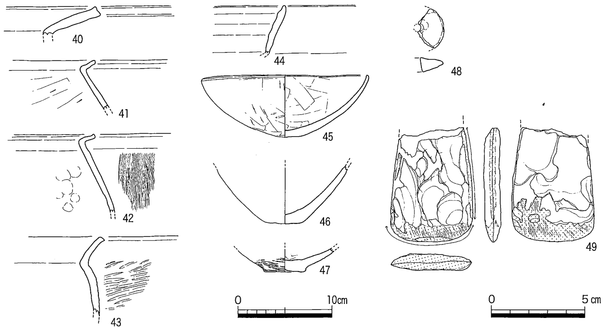
第17図 SH02 出土遺物実測図
