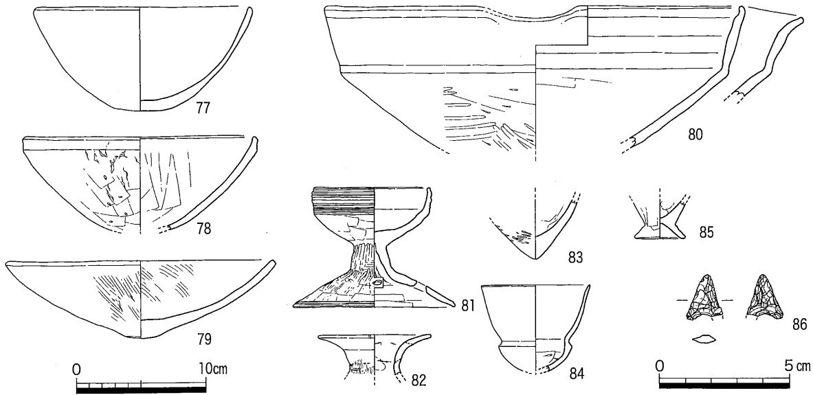
第23図 S H05 出土遺物実測図 (2)
