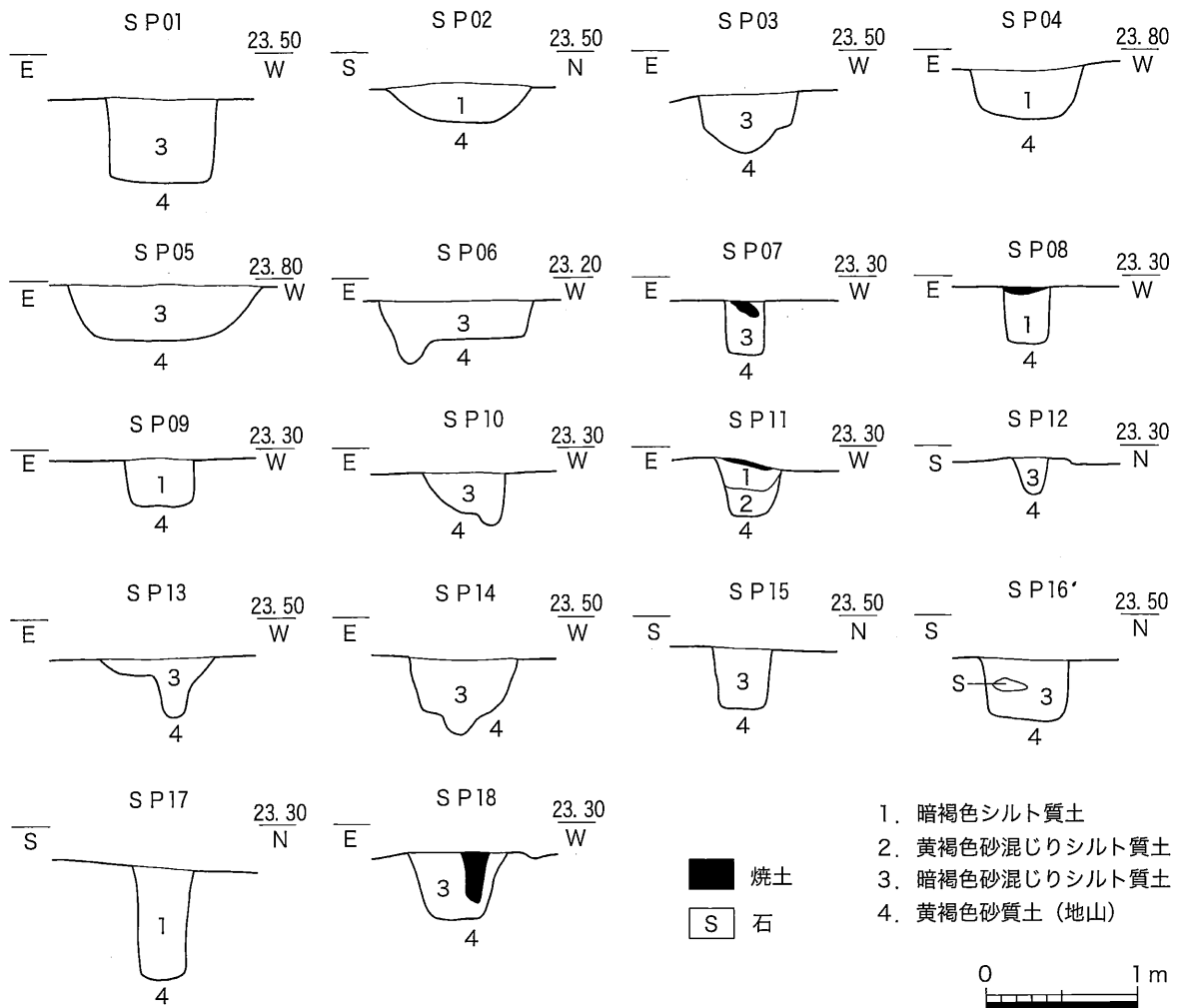
第35図 東段丘地区 SP 断面図 (1/50)
