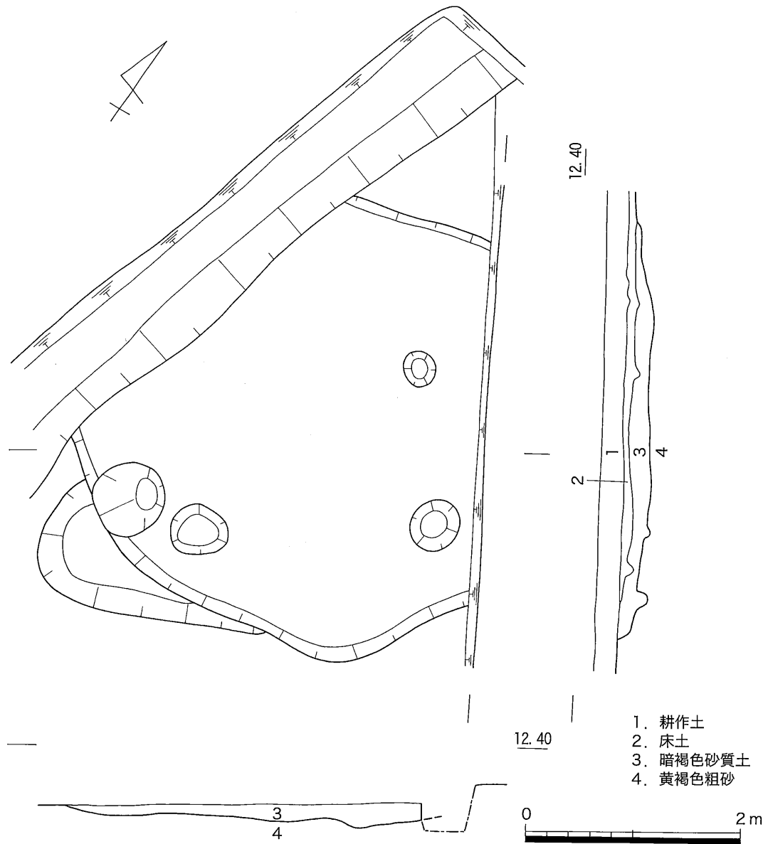
第69図 SX02 平・断面図 (1/50)
