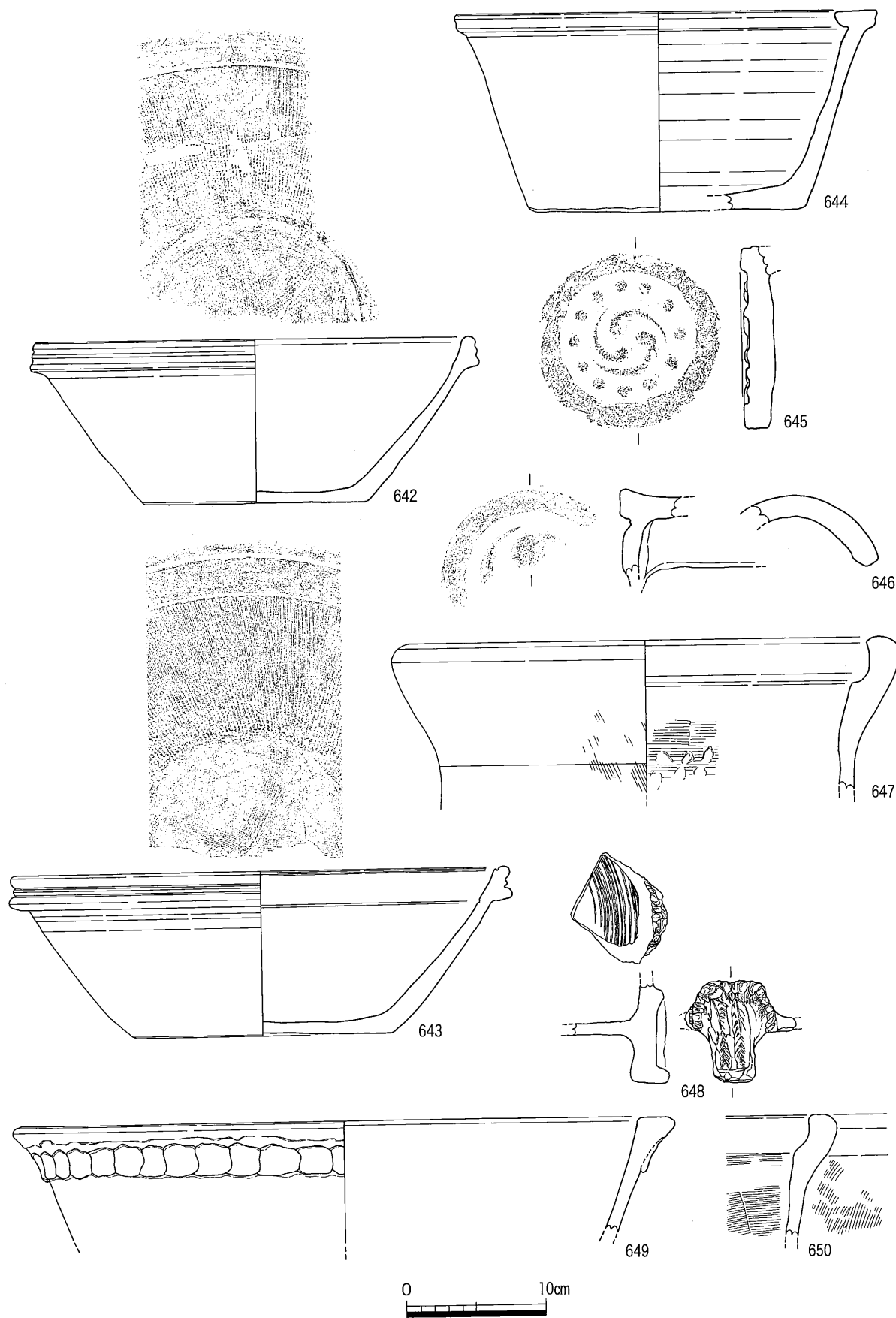
第68図 S D04、05 出土遺物実測図
