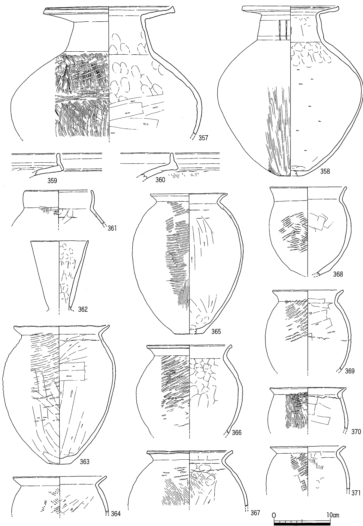
第48図 S R01 出土遺物実測図 (10)
