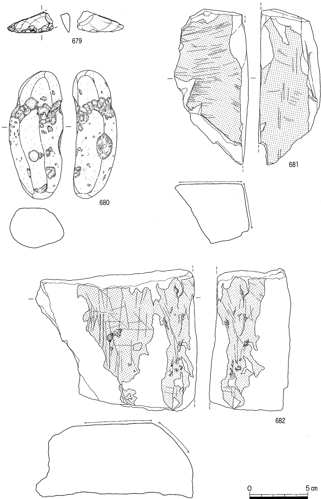
第74図 包含層遺物実測図
