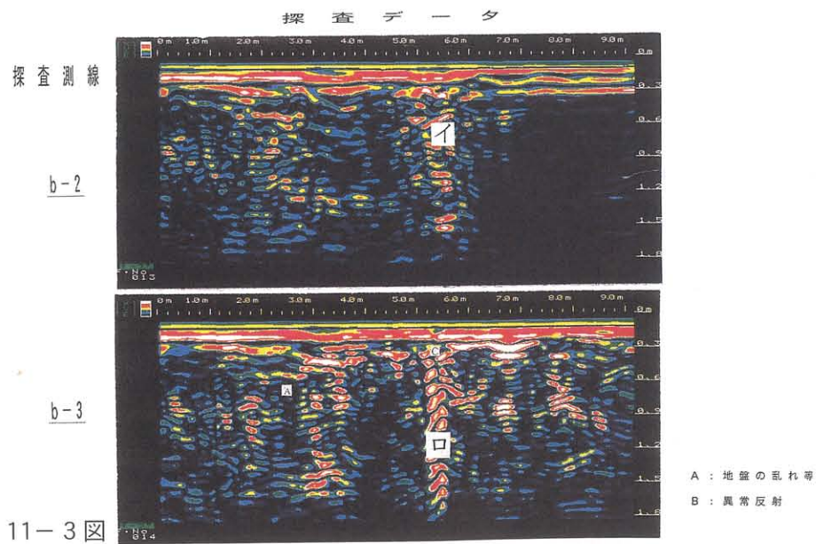
第11図 地中探査成果図 (1)
