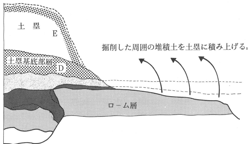
第16図 堆積土層と遺構変遷図
