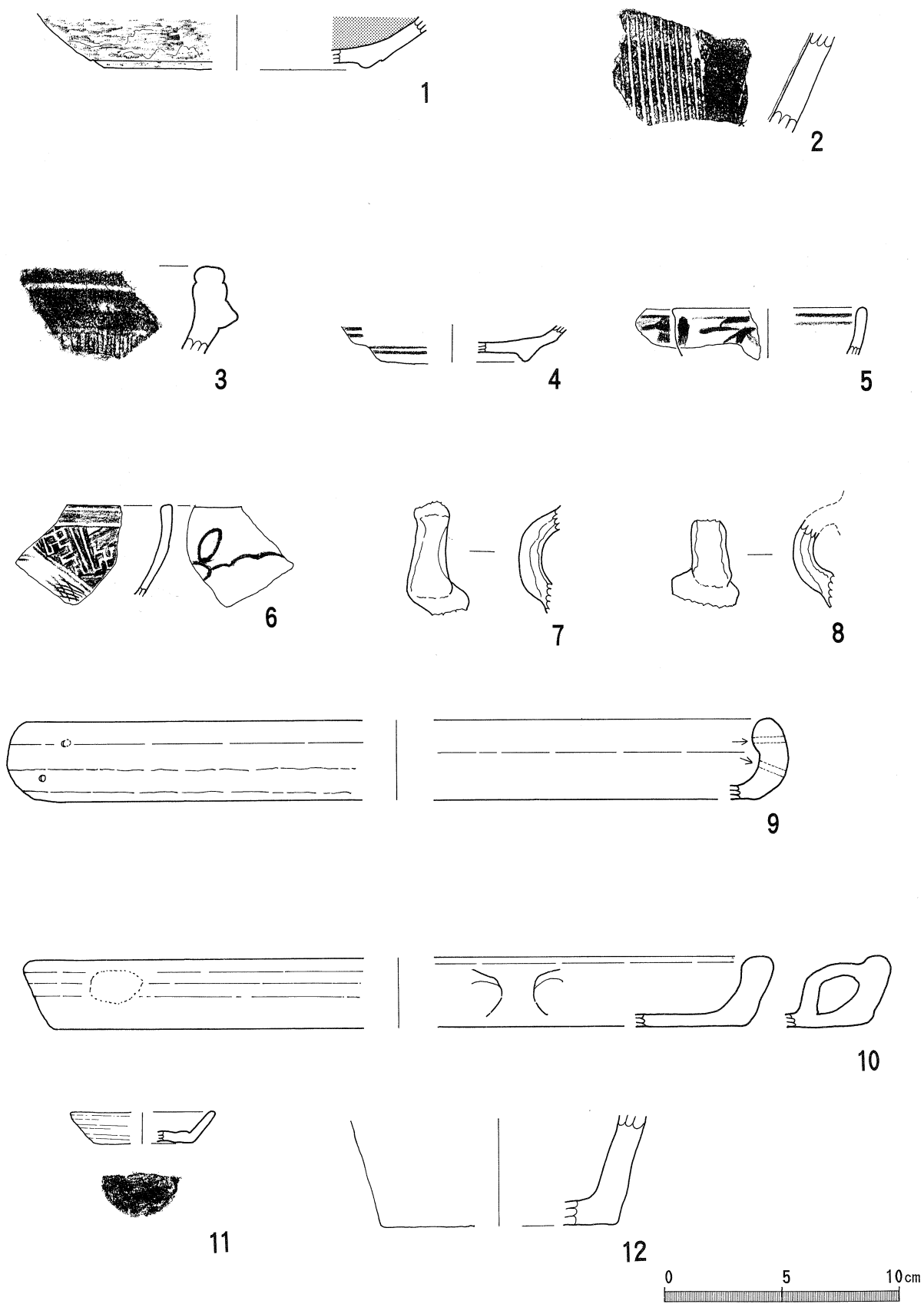
第8图 第1号地下式坑出土遺物実測図
