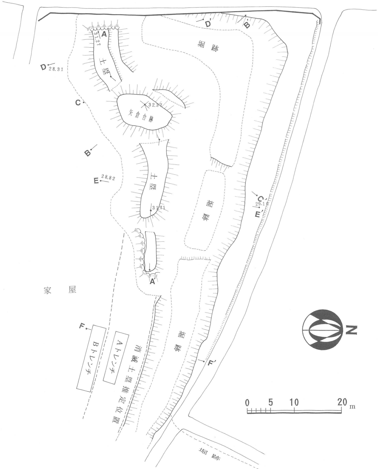
第3図 関城跡現存土塁実測図 (平面図)
