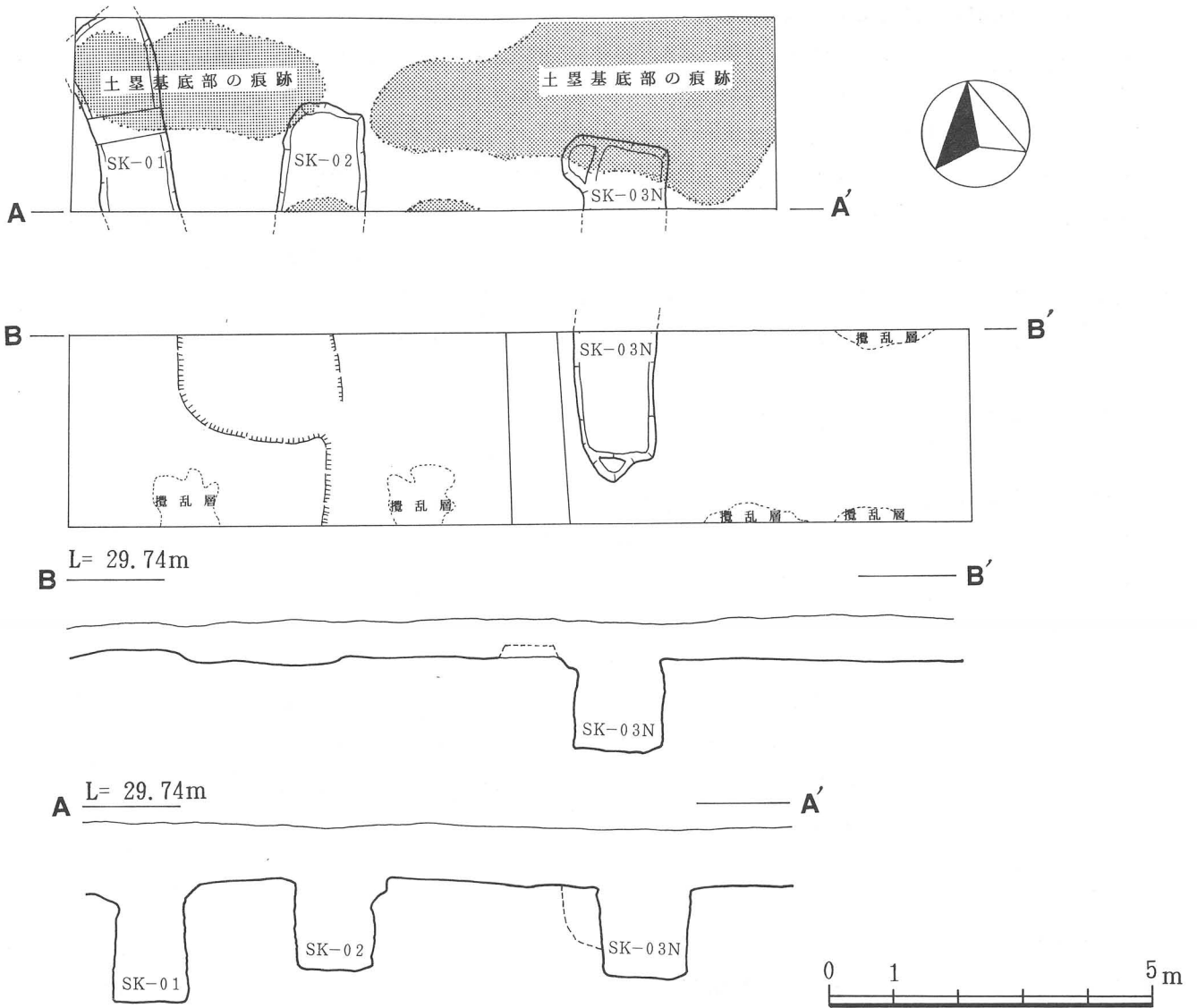
第5図 発掘遺構全体図
