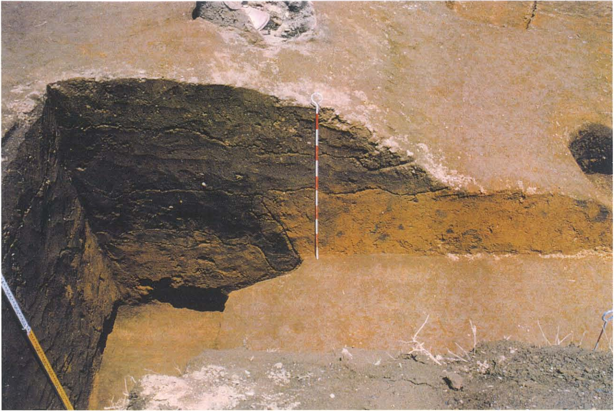
テストトレンチ北側面に確認した土壘基底部と地下式坑竪坑部（SK-01）
