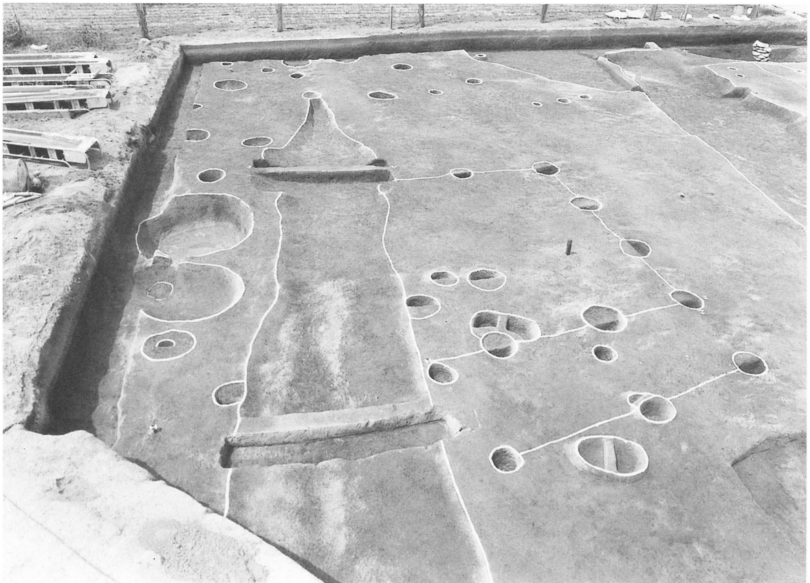
SD12全景 (南より)
