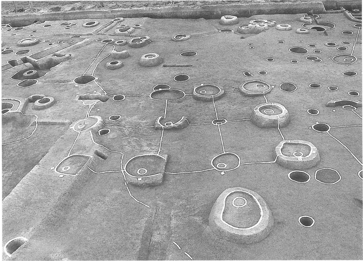
SB25全景（南より）
