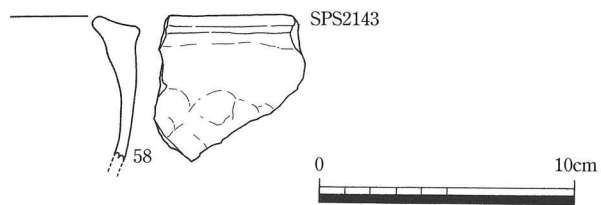
第16図 SKS2001・2002・2010平・断面図 (1/40), 出土遺物 (1/3), SPS2110・2143出土遺物 (1/3)
