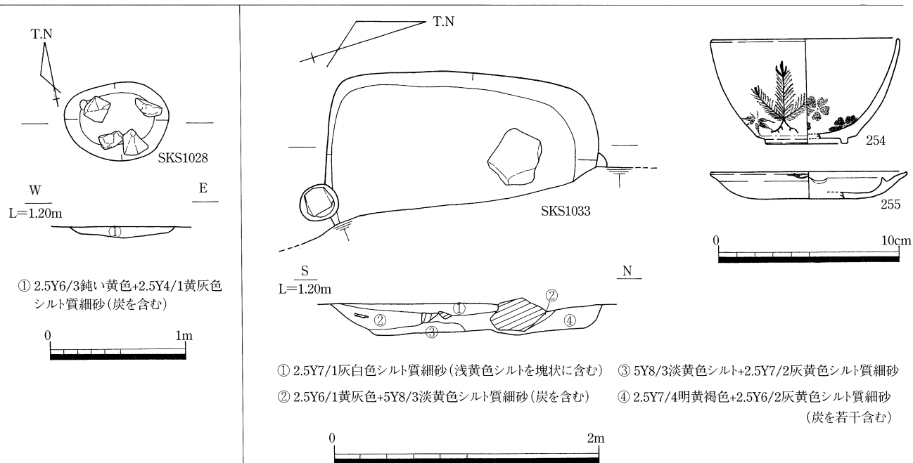
第46図 SKS1027・1028・1033平・断面図 (1/40), SKS1027・1033出土遺物 (1/3, 1/4)
