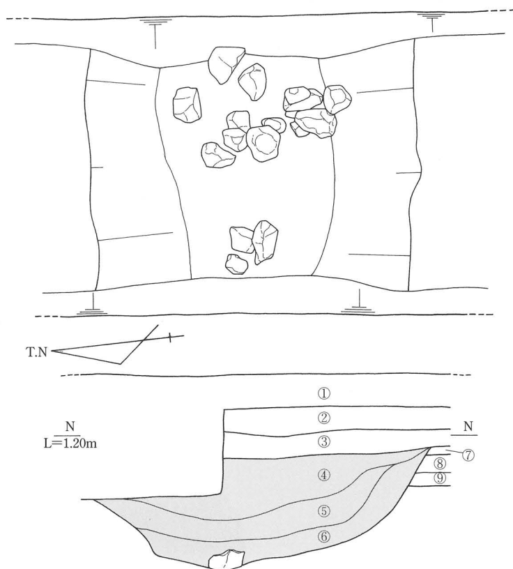
第2トレンチ東壁土層図
