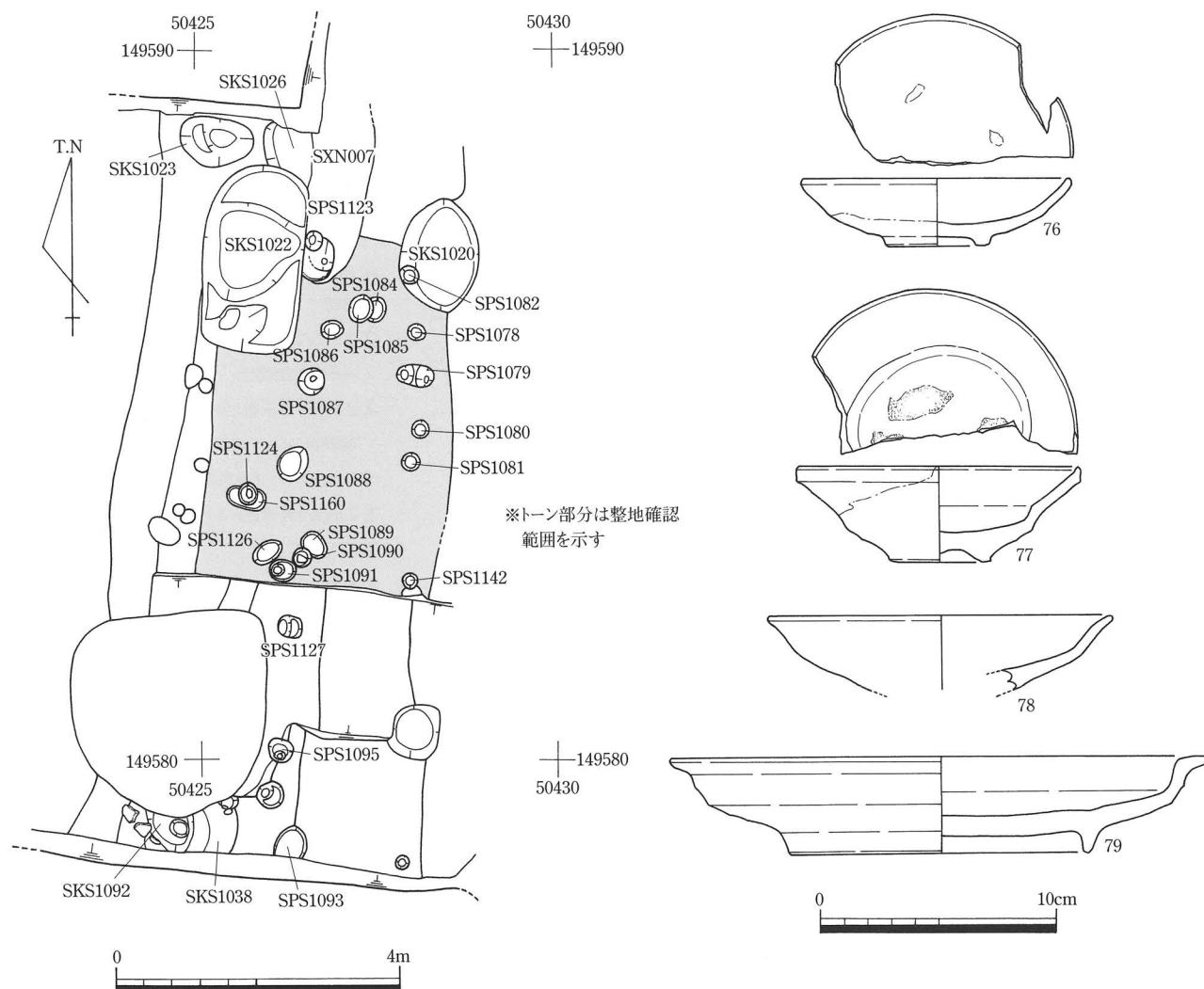
第22図 南調査区中央部平面図（1/100），出土遺物（1/3）
