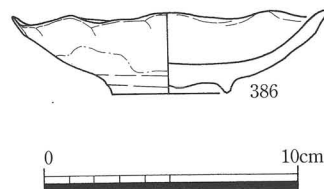
第68図 SKN014・021・025平・断面図 (1/40), SKN025出土遺物 (1/3)
