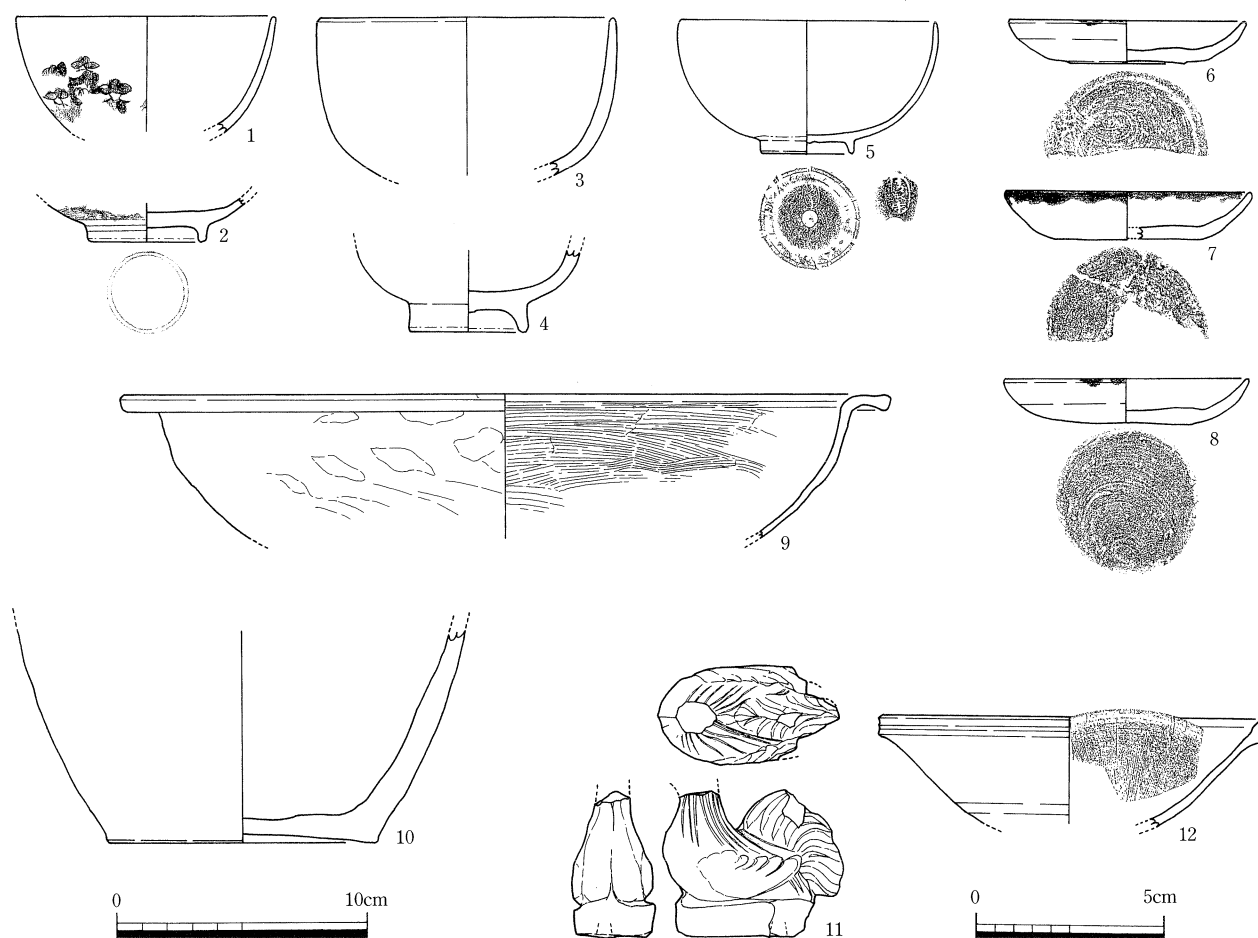
第5図 試掘調査第1トレンチS1出土遺物（1/3，1/2）
