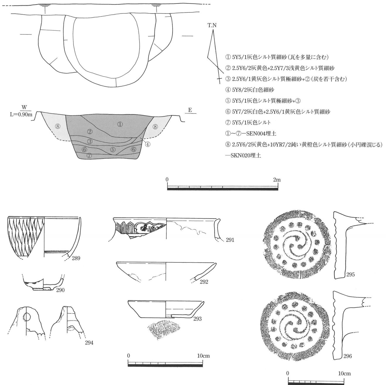
第53図 SEN004, SKN020平・断面図 (1/40), SEN004出土遺物 (1/3, 1/4)
