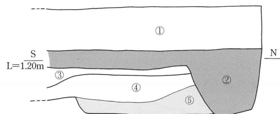
第2トレンチ西壁土層図
