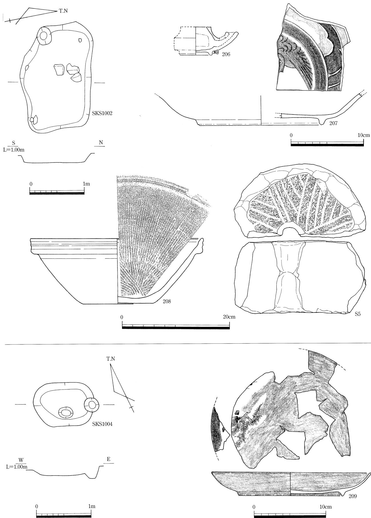
第39図 SKS1002・1004平・断面図 (1/40), 出土遺物 (1/3, 1/4)
