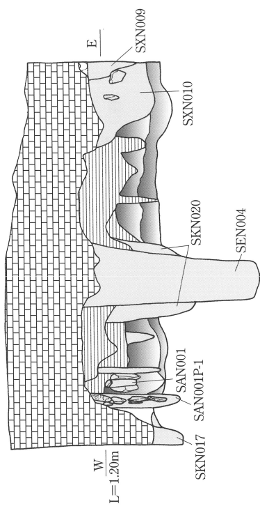
第5トレンチ北壁
