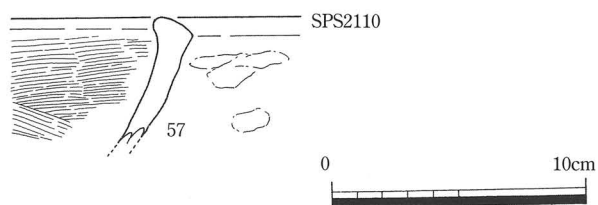
第16図 SKS2001・2002・2010平・断面図 (1/40), 出土遺物 (1/3), SPS2110・2143出土遺物 (1/3)
