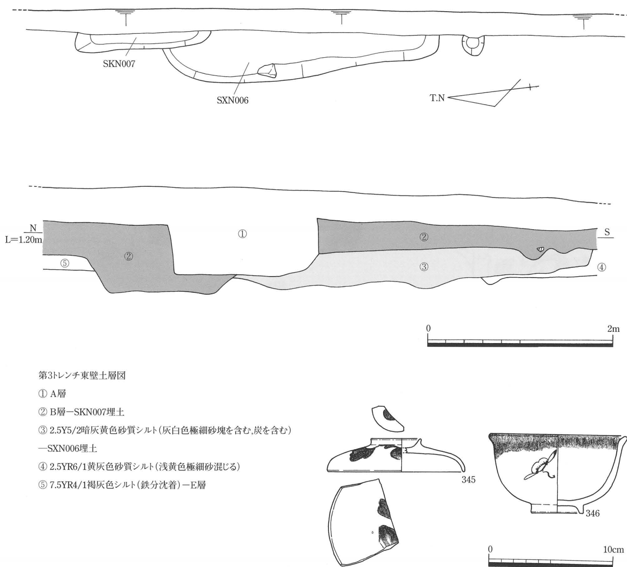
第59図 SXN006・SKN007平・断面図 (1/40), SKN007出土遺物 (1/3)
