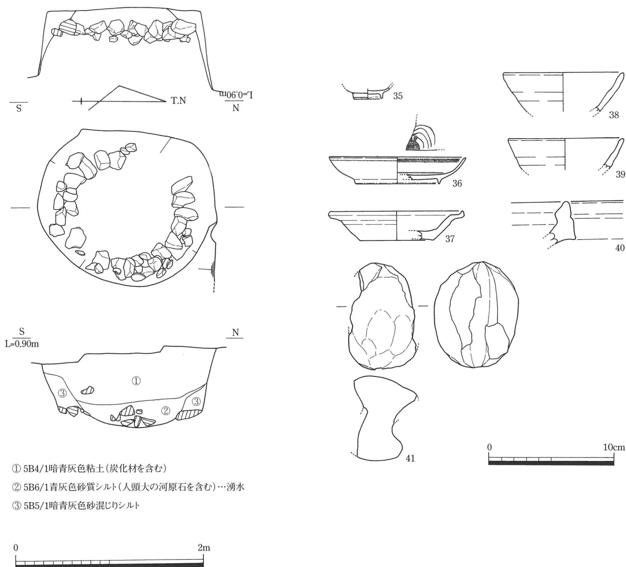
第13図 SES2001平・断面図（1/40）、出土遺物（1/3）
