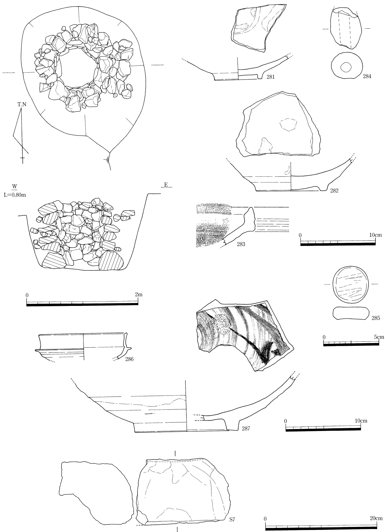
第51図 SEN001平・断面図 (1/40), 出土遺物 (1/3, 1/2, 1/4)
