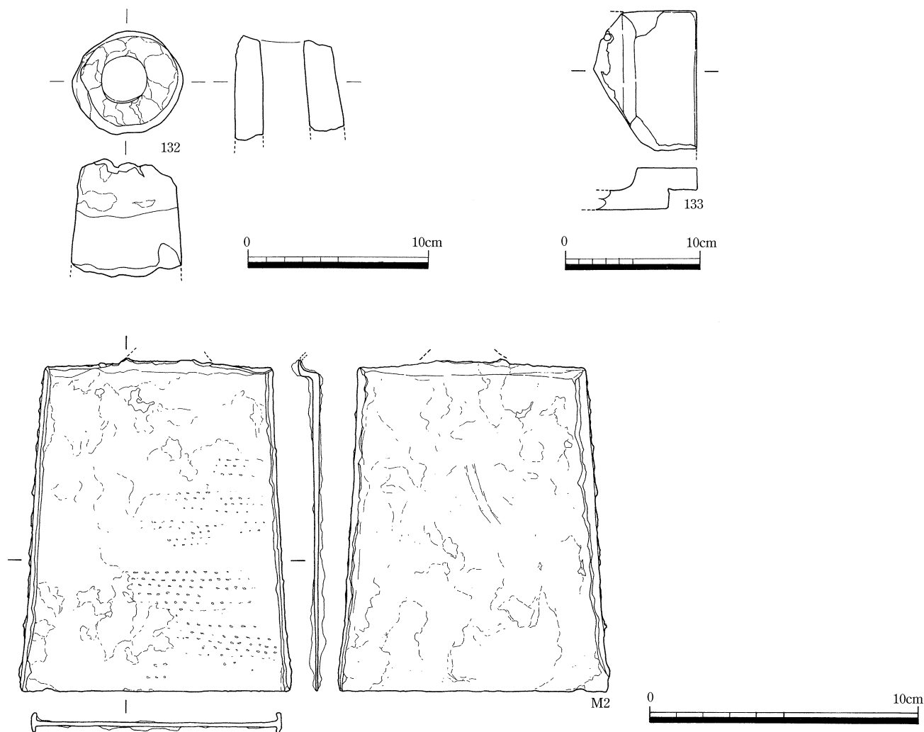
第30図 SXS1001上層出土遺物 (1/3, 1/4, 1/2)
