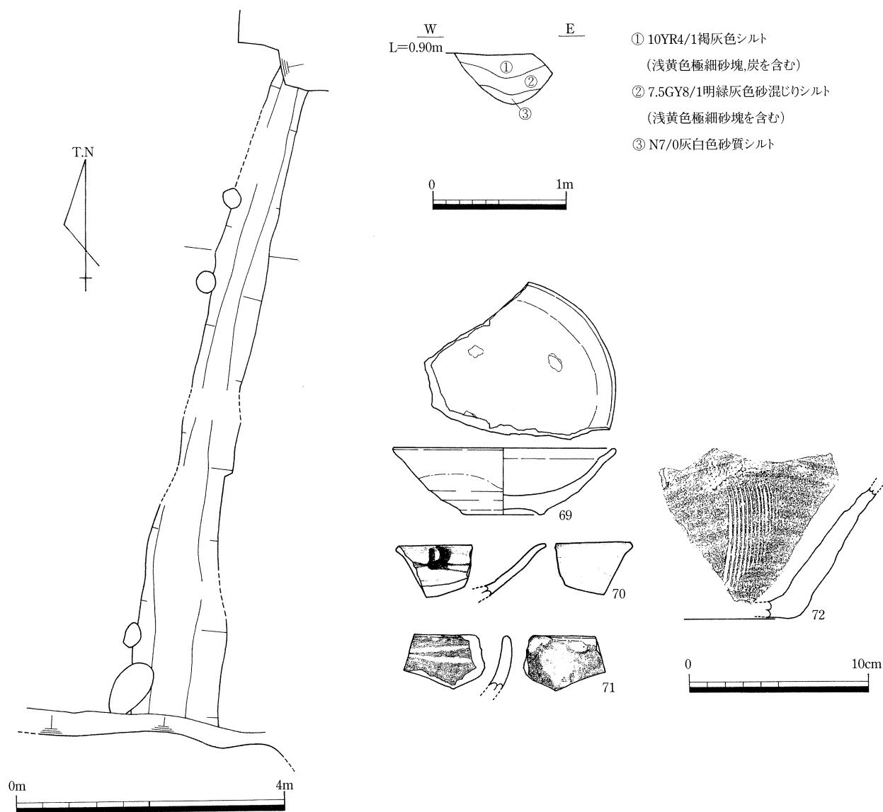
第20図 SDS2002平・断面図 (1/80, 1/40), 出土遺物 (1/3)
