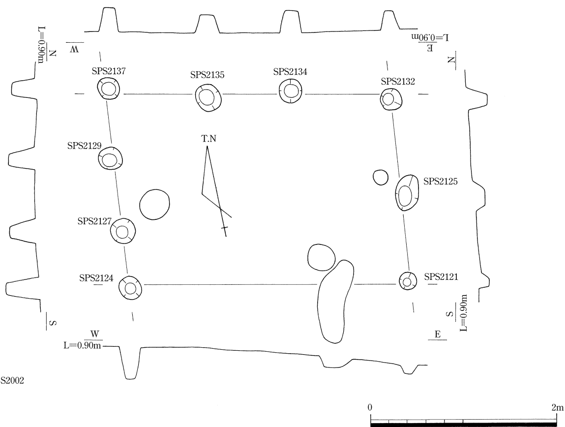
第17図 SBS2001・2002平・断面図 (1/40)
