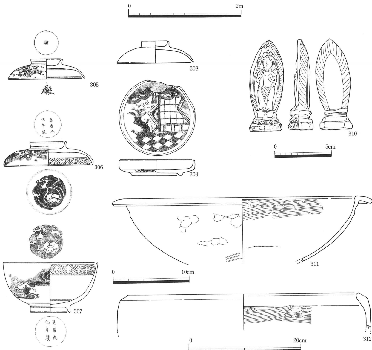
第55図 SXN002, SKN001平・断面図 (1/40), SKN001出土遺物 (1/3, 1/4, 1/2)
