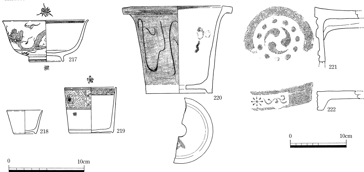
第40図 SKS1005・1006平・断面図 (1/40), 出土遺物 (1/3, 1/4)
