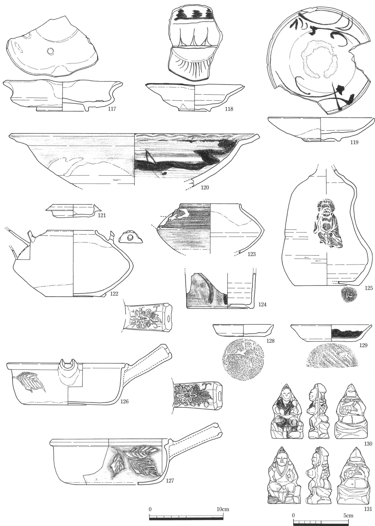
第29図 SXS1001上層出土遺物 (1/3, 1/2)
