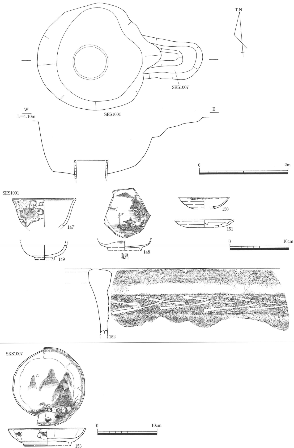
第32図 SES1001, SKS1007平・断面図 (1/40), 出土遺物 (1/3)
