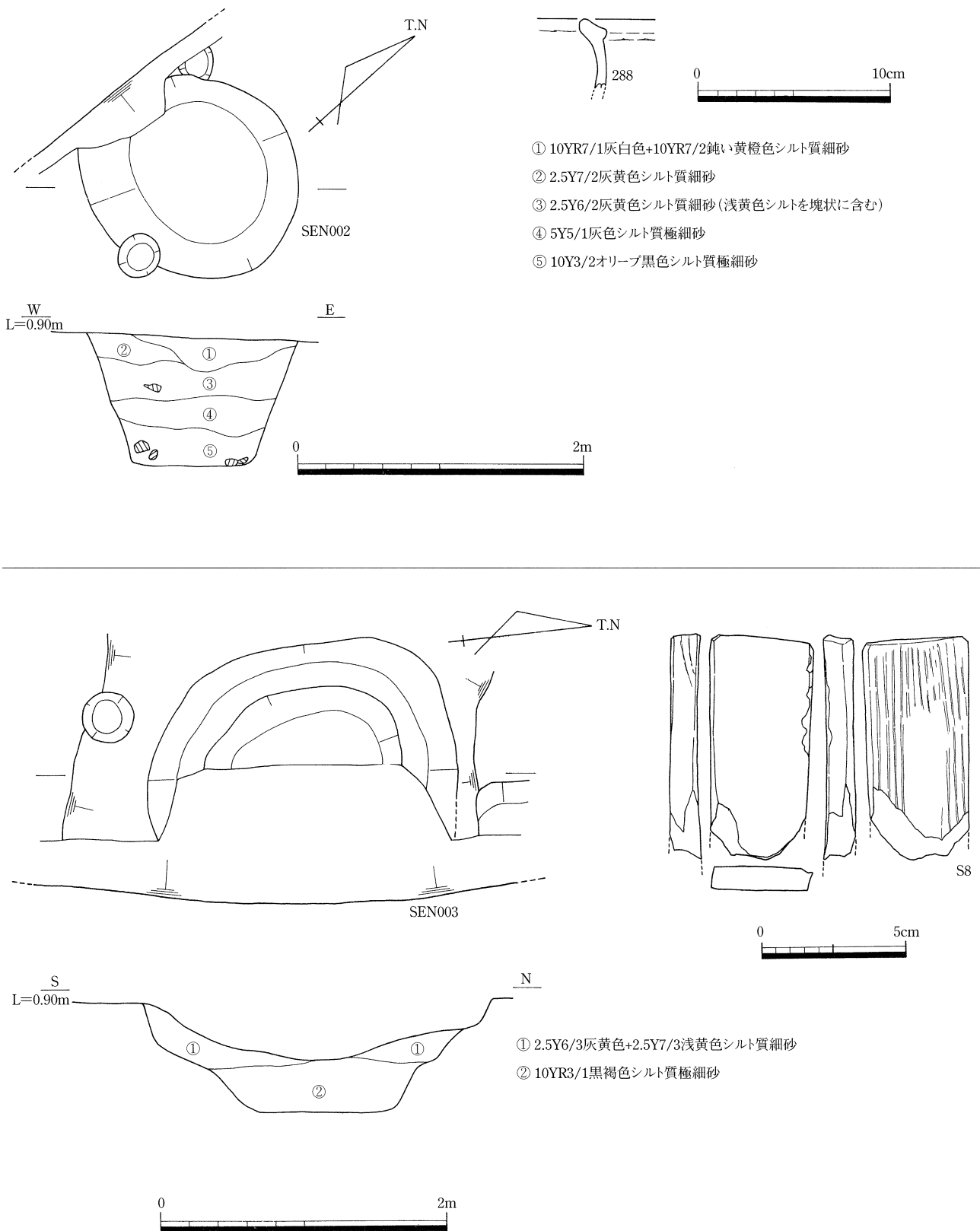
第52図 SEN002・003平・断面図 (1/40), 出土遺物 (1/3, 1/2)
