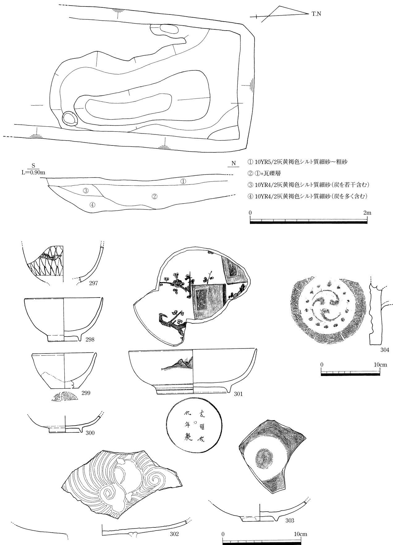
第54図 SXN001平・断面図 (1/40), 出土遺物 (1/3, 1/4)
