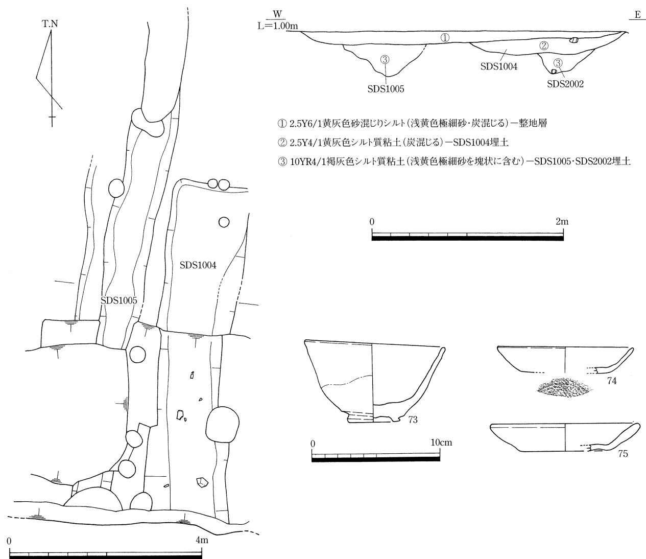
第21図 SDS1004・1005平・断面図（1/80，1/40），SDS1004出土遺物（1/3）
