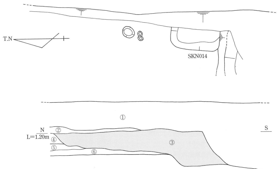
第4トレンチ東壁土層図
