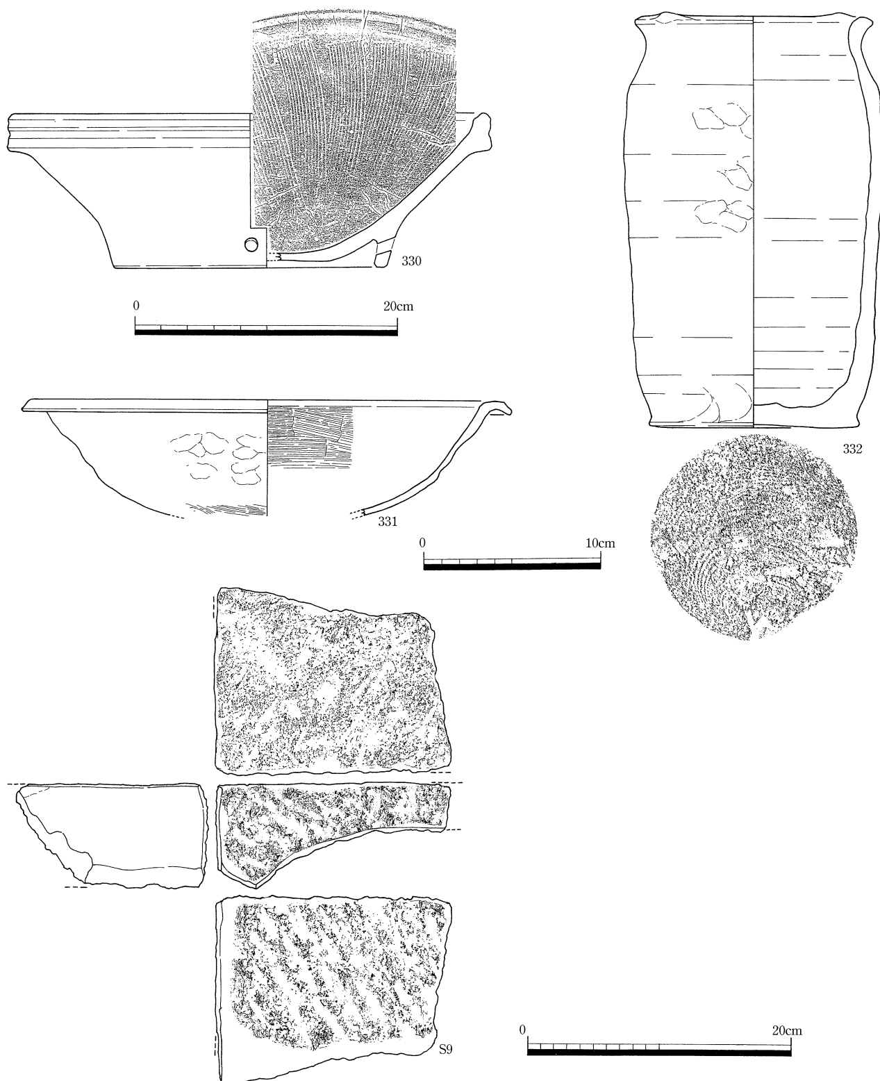
第57図 SXN003出土遺物 (1/3, 1/4)
