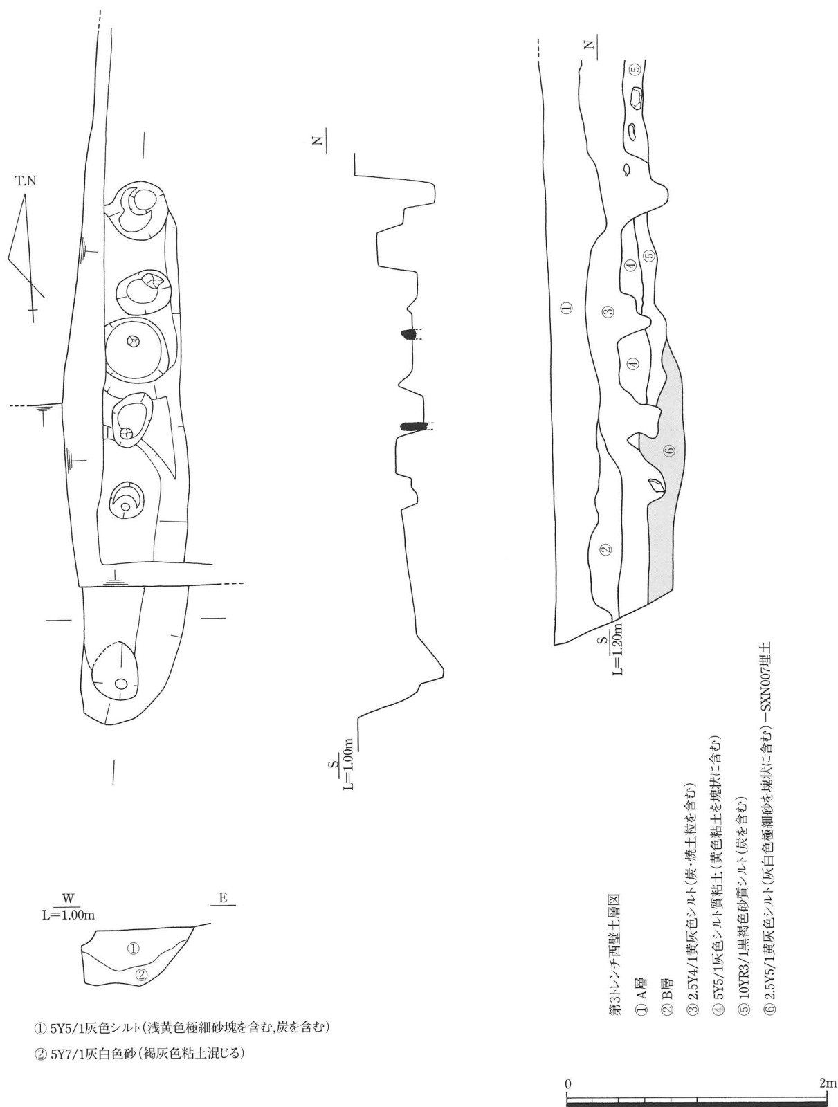
第61図 SXN007平・断面図 (1/40)
