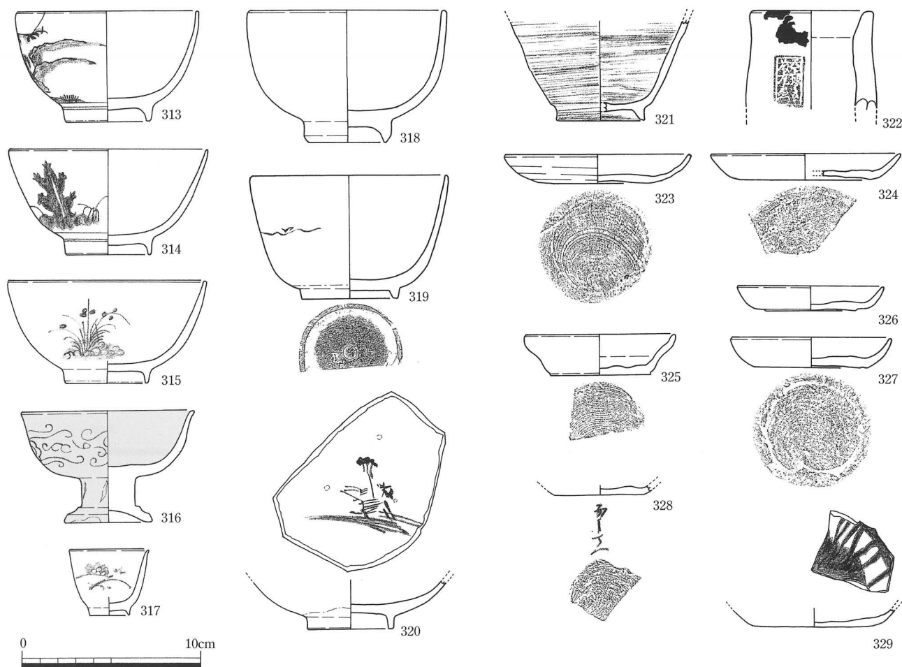
第56図 SXN003平・断面図 (1/40), 出土遺物 (1/3)
