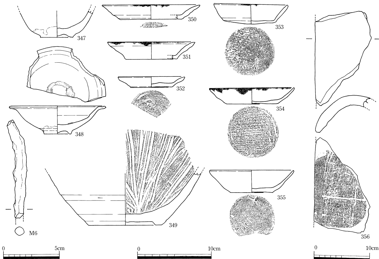
第63図 SXN008平・断面図 (1/40), 出土遺物 (1/3, 1/4, 1/2)
