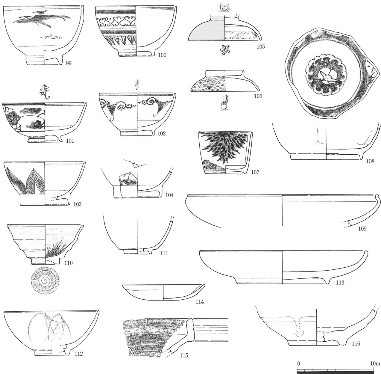
第28図 SXS1001中層・上層出土遺物 (1/3)
