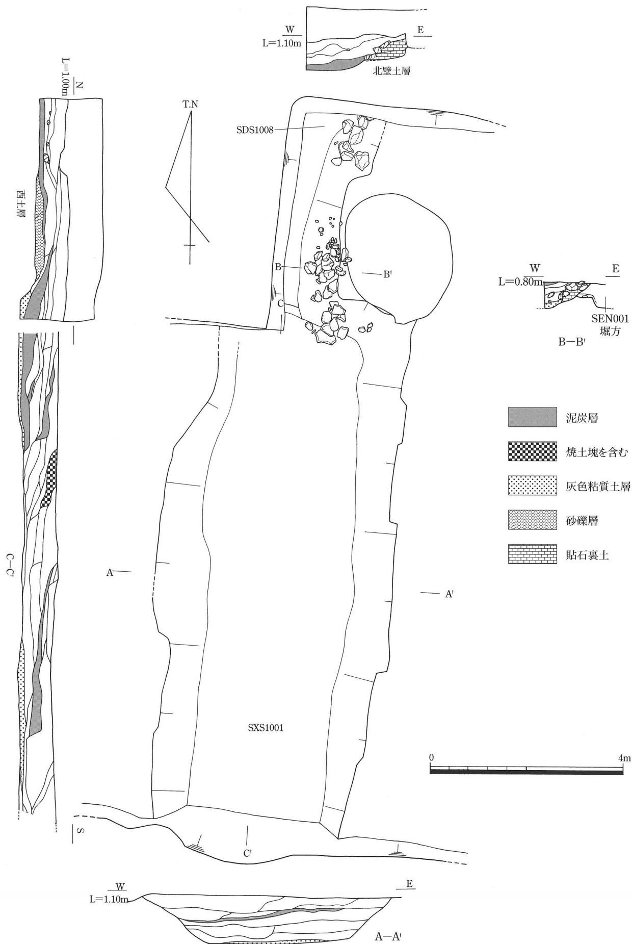
第26図 SXS1001, SDS1008平・断面図 (1/80)
