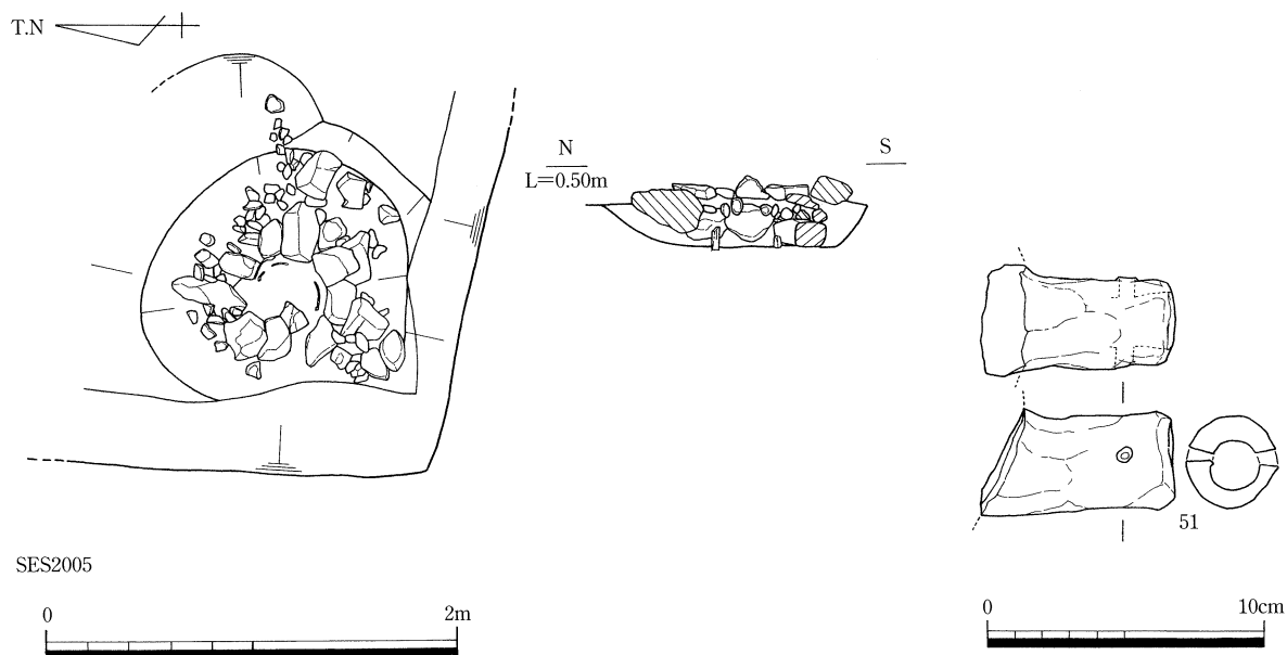
第15図 SES2004・2005平・断面図 (1/40), 出土遺物 (1/3, 1/4)
