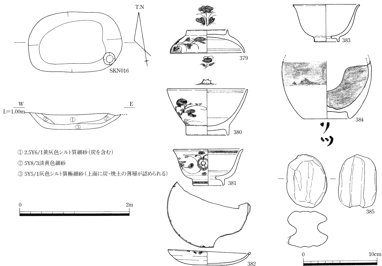
第67図 SKN013・016平・断面図 (1/40), 出土遺物 (1/3, 1/2)
