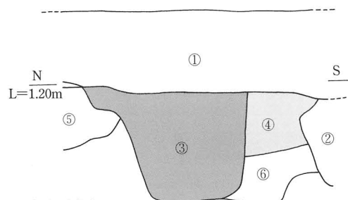
第4トレンチ東壁土層図
