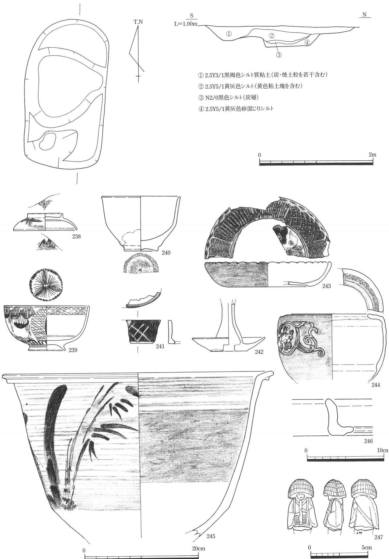
第44図 SKS1022平・断面図 (1/40), 出土遺物 (1/3, 1/4, 1/2)
