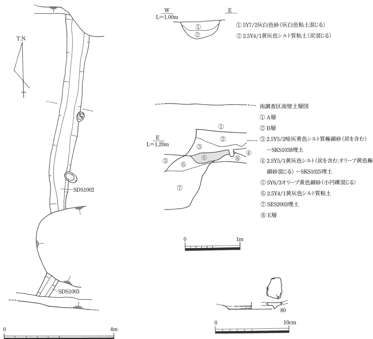
第23図 SDS1002・1003平・断面図（1/80, 1/40）, SDS1003出土遺物（1/3）
