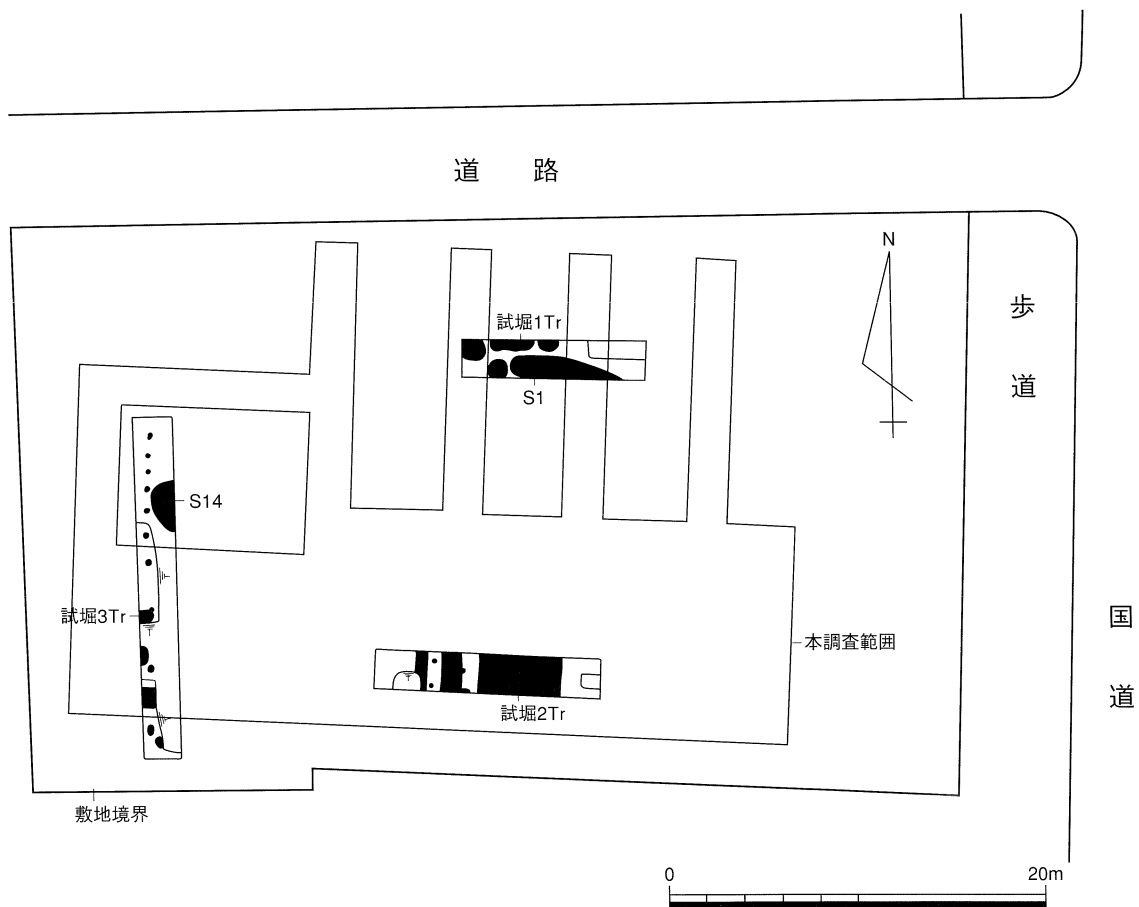
第4図 試掘調査トレンチ・遺構配置図（1/400）
