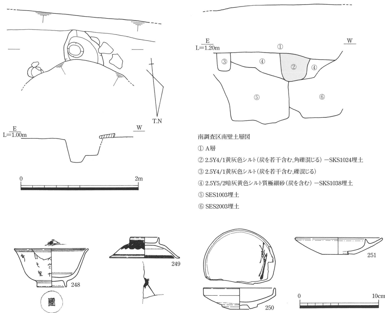
第45図 SKS1024平・断面図 (1/40)，出土遺物 (1/3)
