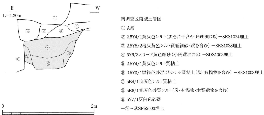
第14図 SES2002・2003平・断面図 (1/40), 出土遺物 (1/3, 1/4)
