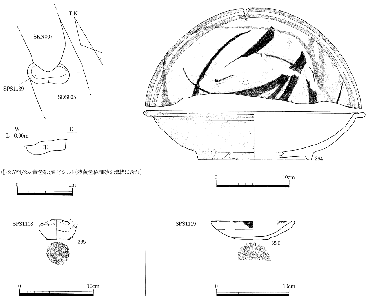
第48図 SPS1139平・断面図（1/40），SPS1139・1108・1119出土遺物（1/3）
