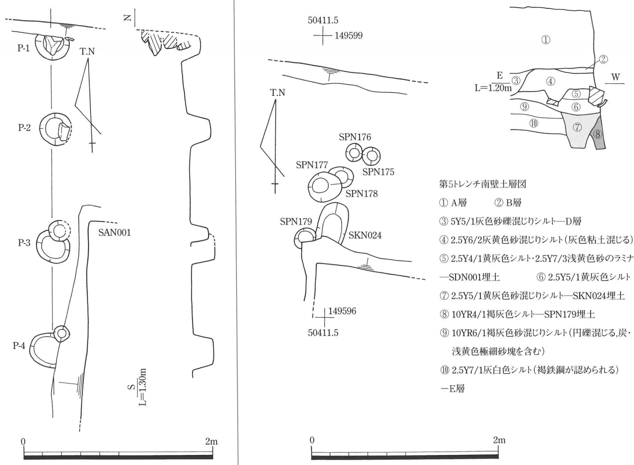
第69図 SDN001, SAN001, SDN001下層検出遺構平・断面図 (1/40), SDN001出土遺物 (1/3)
