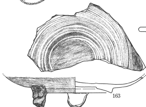
第33図 SES1002平・断面図 (1/40), 出土遺物 (1/3)
