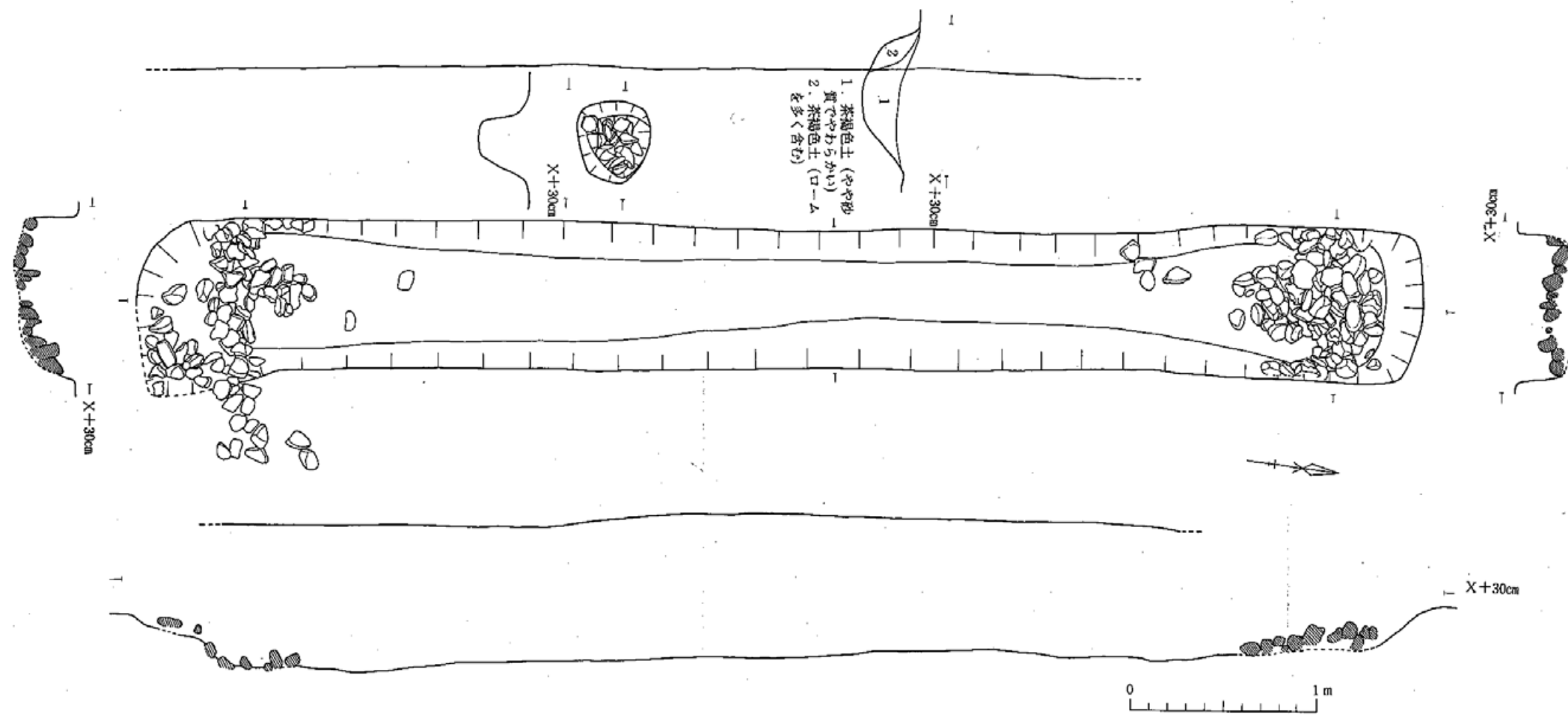
第7図 主体部実測図
