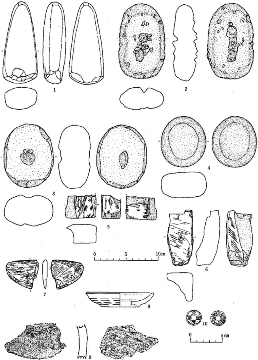
第14図 出土遺物
