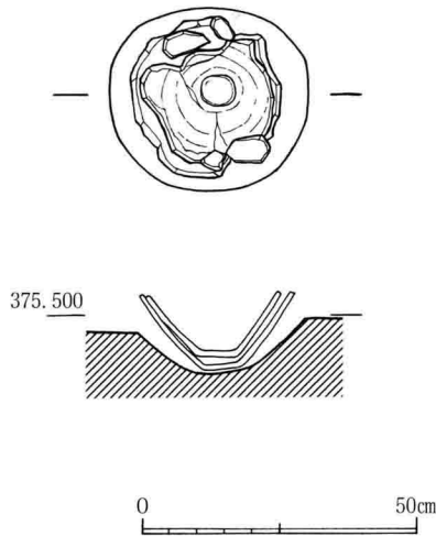
図16 E区SB6実測図 (S=1:15)
