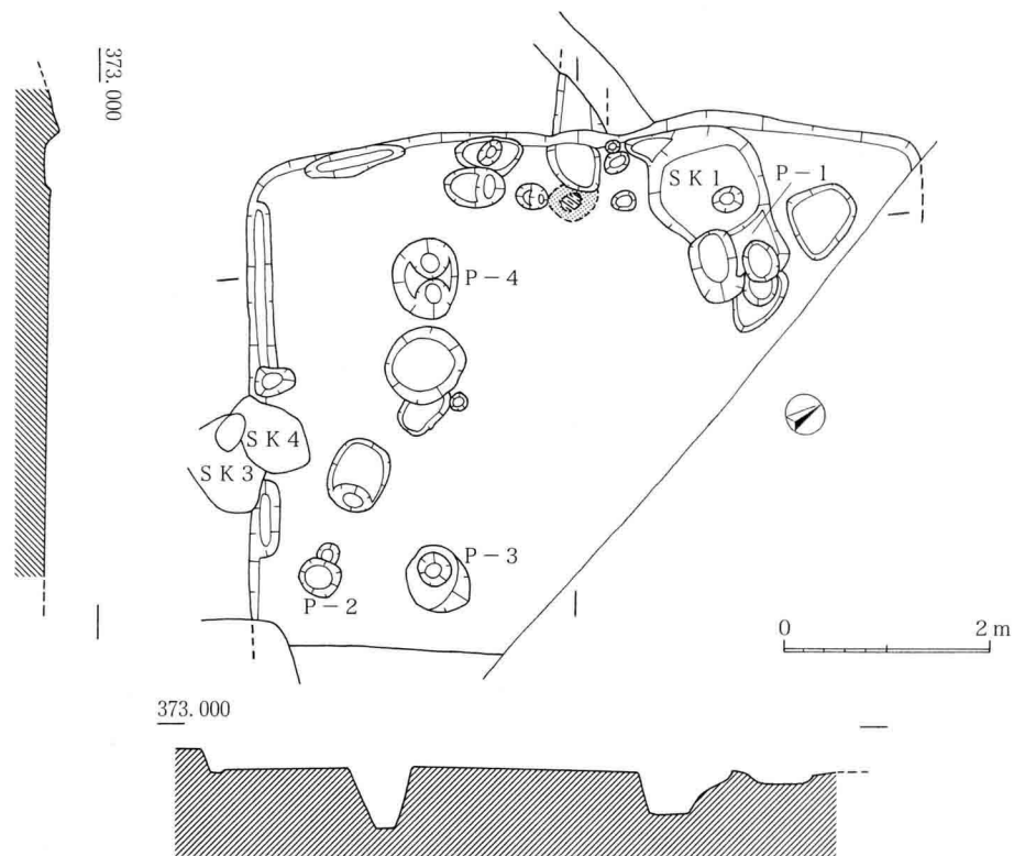
図19 AB区SB3実測図（S=1:80）
