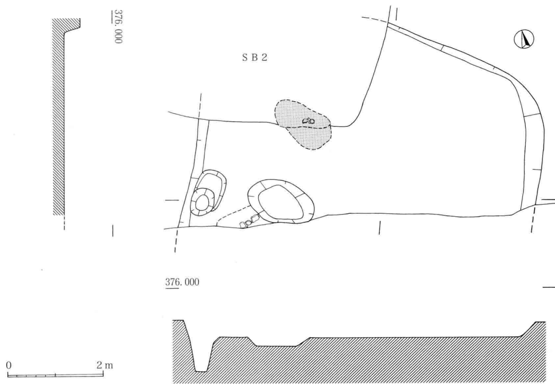
図52 G区SB 3実測図 (S = 1 : 80)
