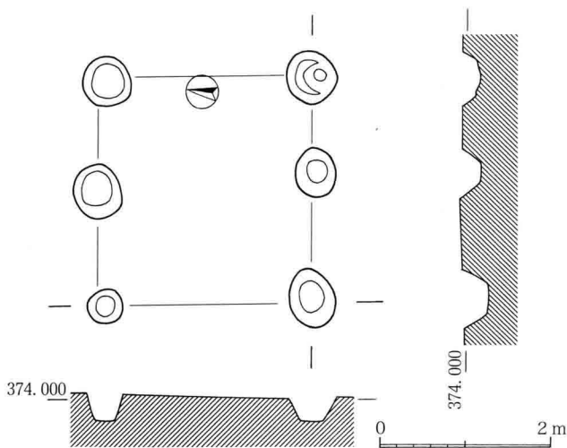
図60 H区ST1実測図 (S=1:80)
