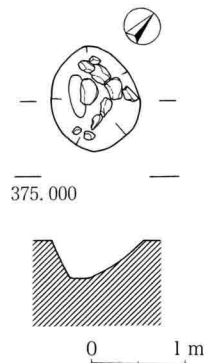
図63 J区SK1 実測図 (S = 1 : 80)
