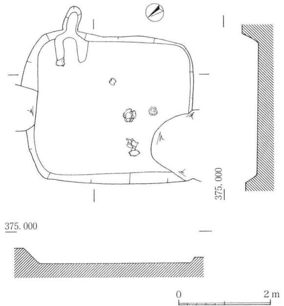
図26 I区SB4実測図 (S=1:80)
