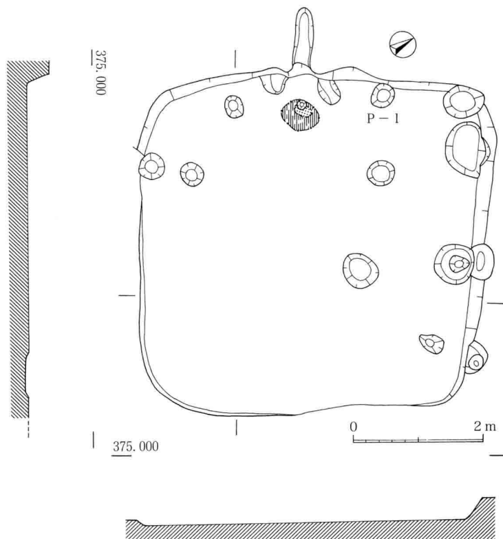
図30 J区SB2実測図（S=1:80）
