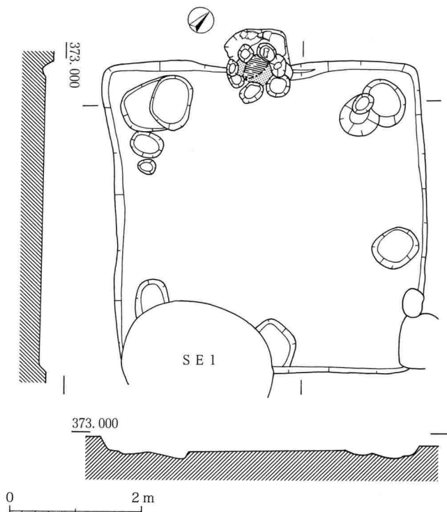
図32 AB区SB2実測図（S=1:80）
