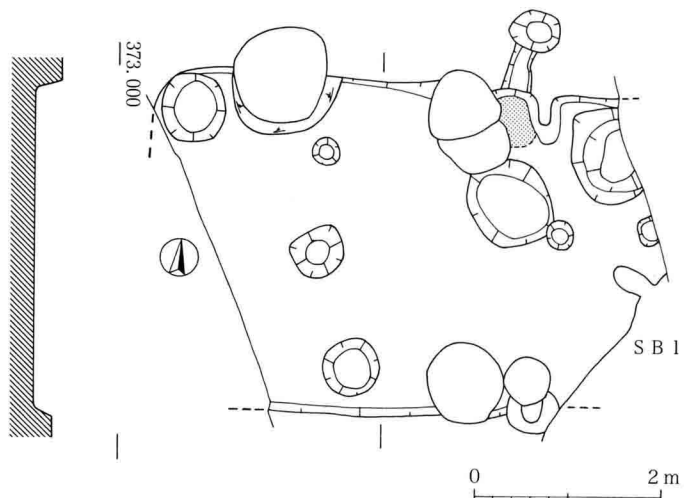
図49 F区SB4実測図 (S=1:80)
