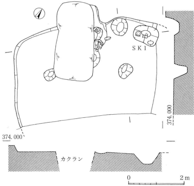
図25 H区SB2実測図(S=1:80)
