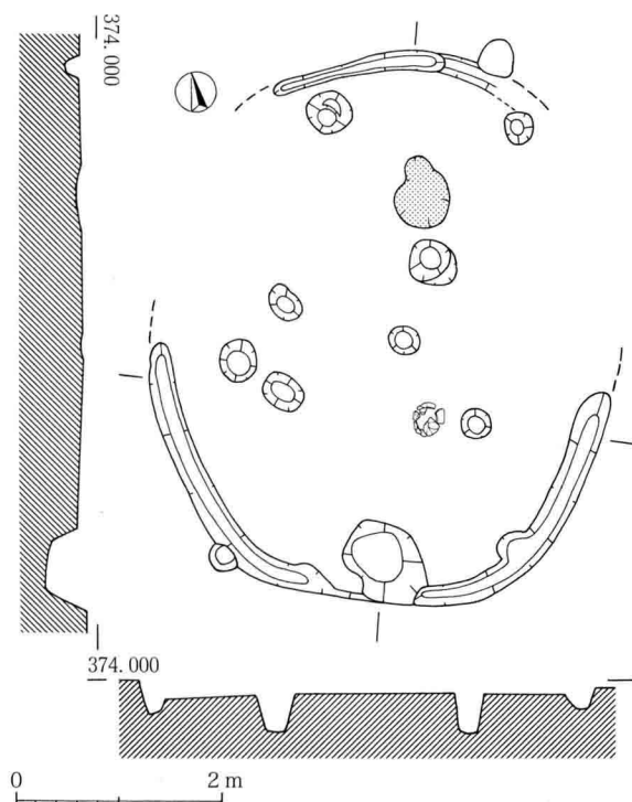
図12 H区SB3実測図 (S=1:80)
