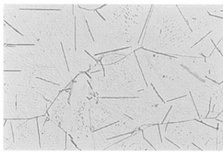
北之脇遺跡 鍛造剥片 NO.1-4 ×800
