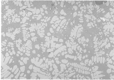
北之脇遺跡 鍛造剥片 NO.1-2 ×800
