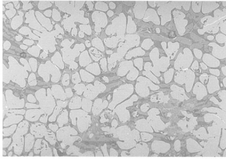
北之脇遺跡 鍛造剥片 NO.1-1 ×800
