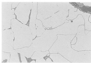
前山田遺跡鉄塊 (資料NO.2) ×800
