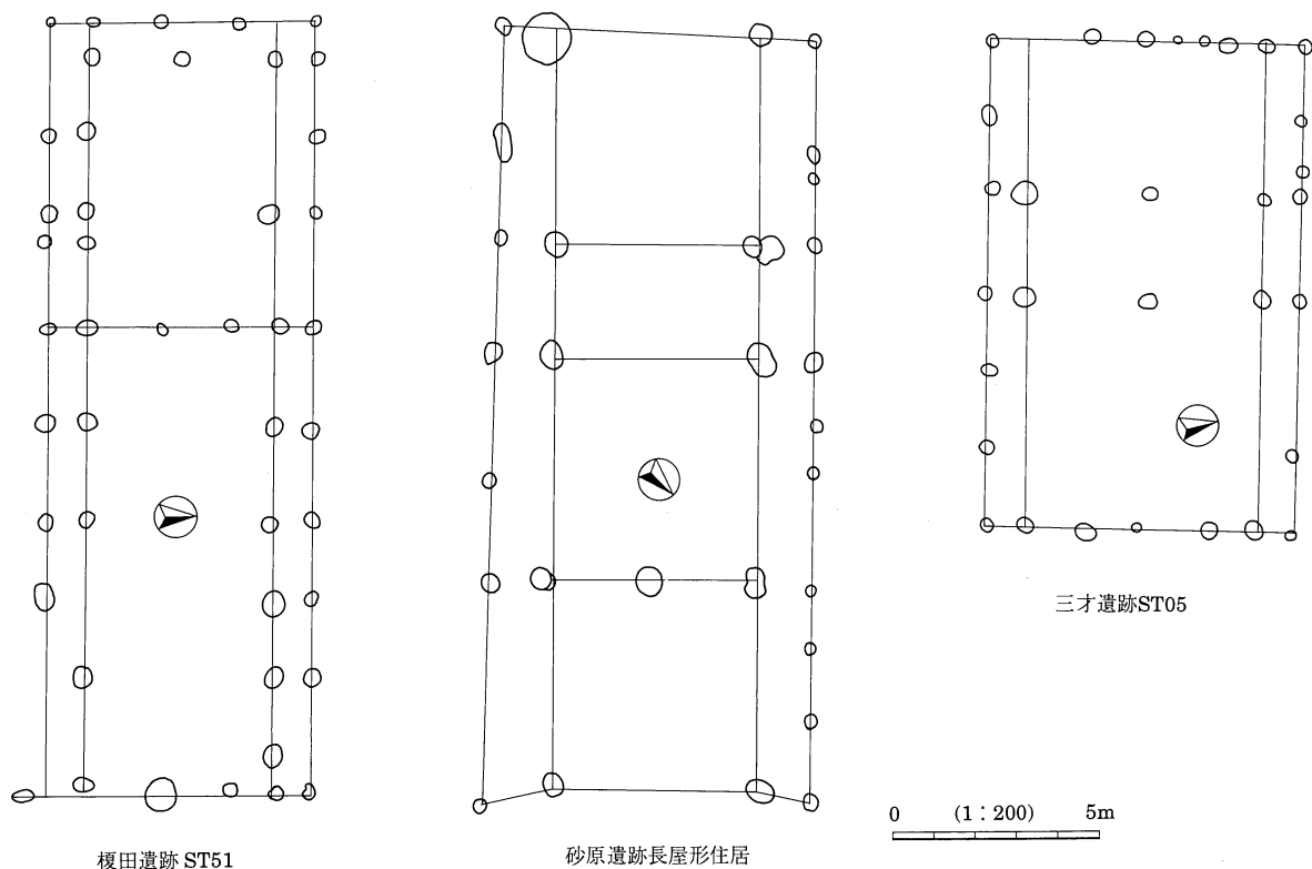
第315図 庇状柱列を持つ掘立柱建物跡(各報告書より加除筆 再トレース)
