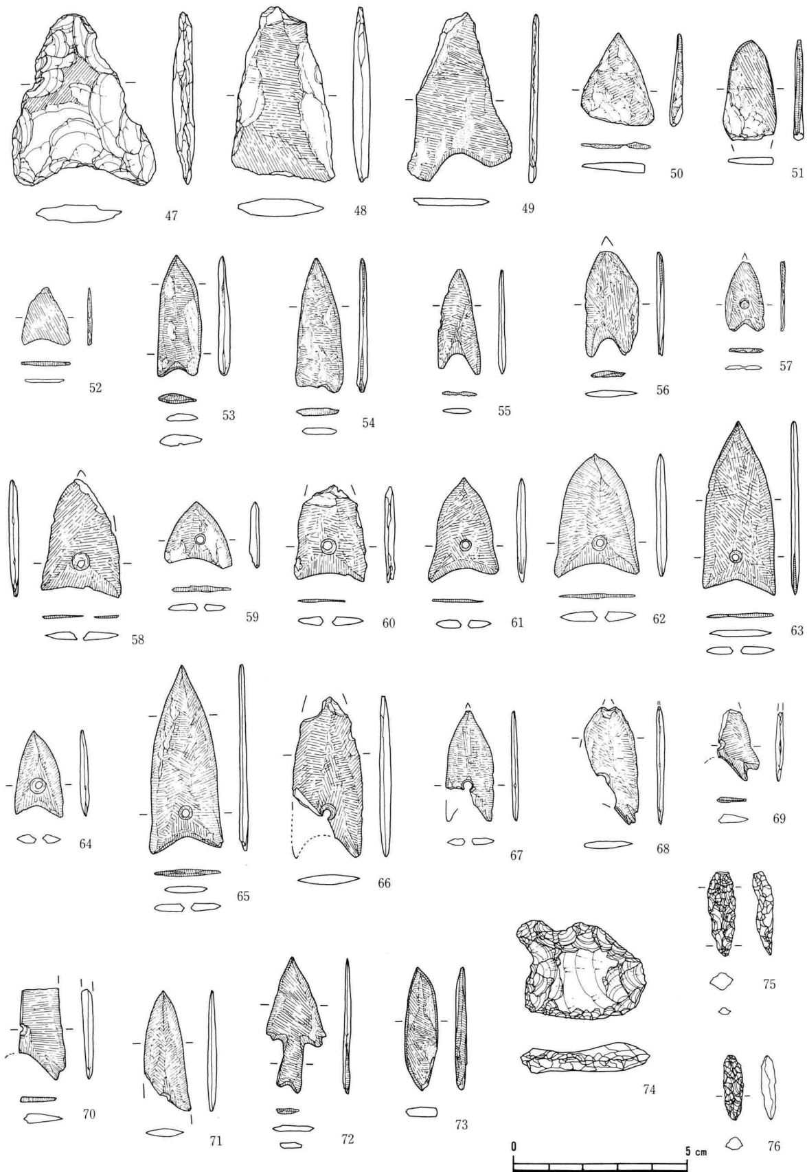
図62 石器（磨製石鏃・石匙・石錐）実測図（2：3）
