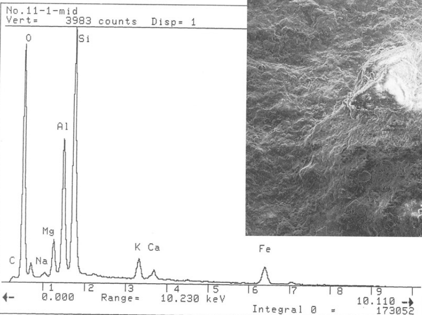
刃部 (B-3) EDX分析チャート
