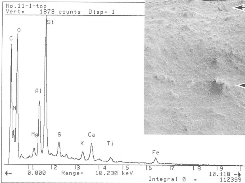
刃部 (B-1) EDX分析チャート
