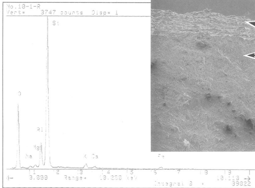
刃部 (C-2) EDX分析チャート
