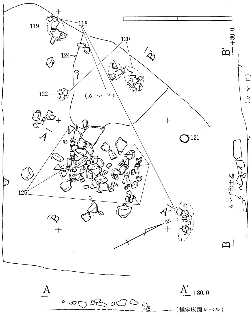
第 28 図 千鹿頭社遺跡 5 区 50 号住居跡遺物分布図・1 号集石平面図・エレベーション図 (S=1/40)
