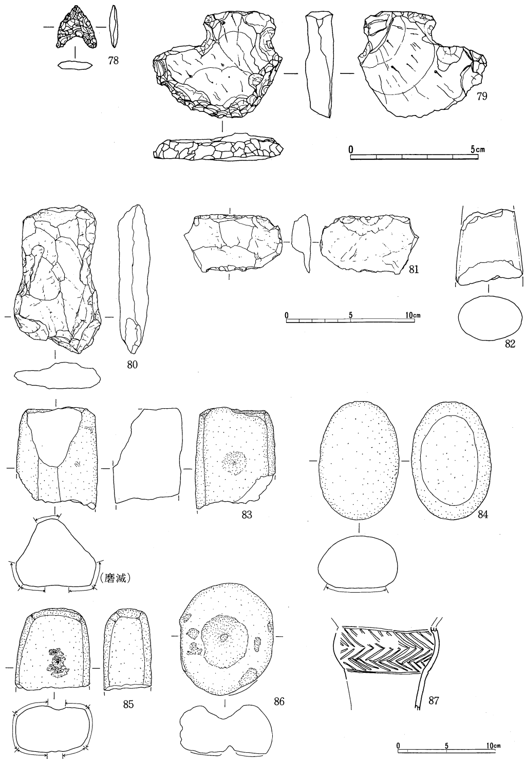
第 22 図 千鹿頭社遺跡 5 区遺構外出土遺物(1) (78・79… S = 2/3、80~86… S = 1/3、87… S = 1/4)
