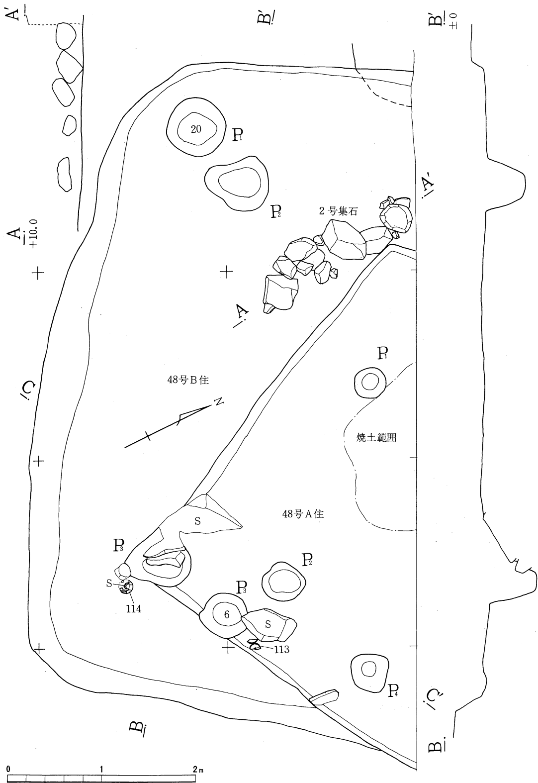
第25図 千鹿頭社遺跡5区48号A・B住居跡・2号集石平面図・エレベーション図 (S=1/40)
