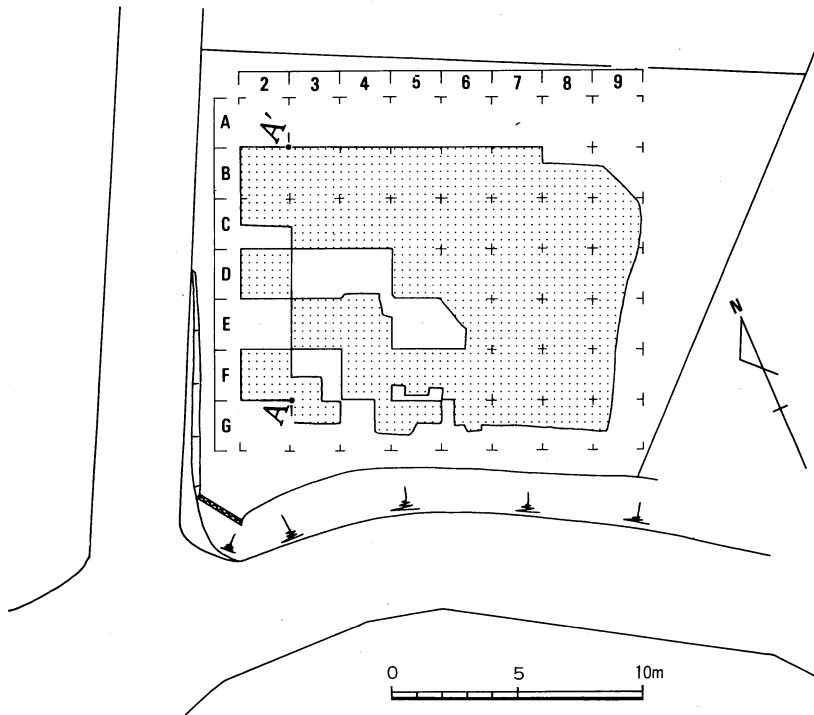
第4図 千鹿頭社遺跡5区全体図 (S=1/300)
