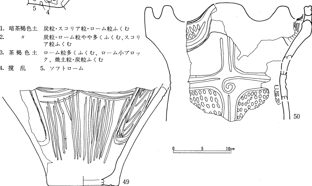
第16図 千鹿頭社遺跡5区53号住居跡平面図・エレベーション図 (S=1/40) 53号住居跡出土遺物 (S=1/4)
