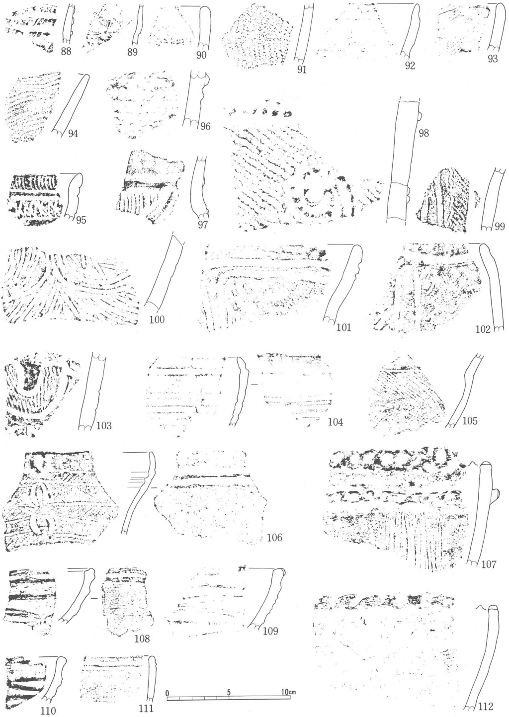
第23図 千鹿頭社遺跡5区遺構外出土遺物(2) (S=1/3)
