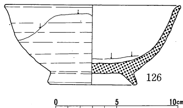
第32図 千鹿頭社遺跡5区遺構外 出土遺物3 (S=1/3)
