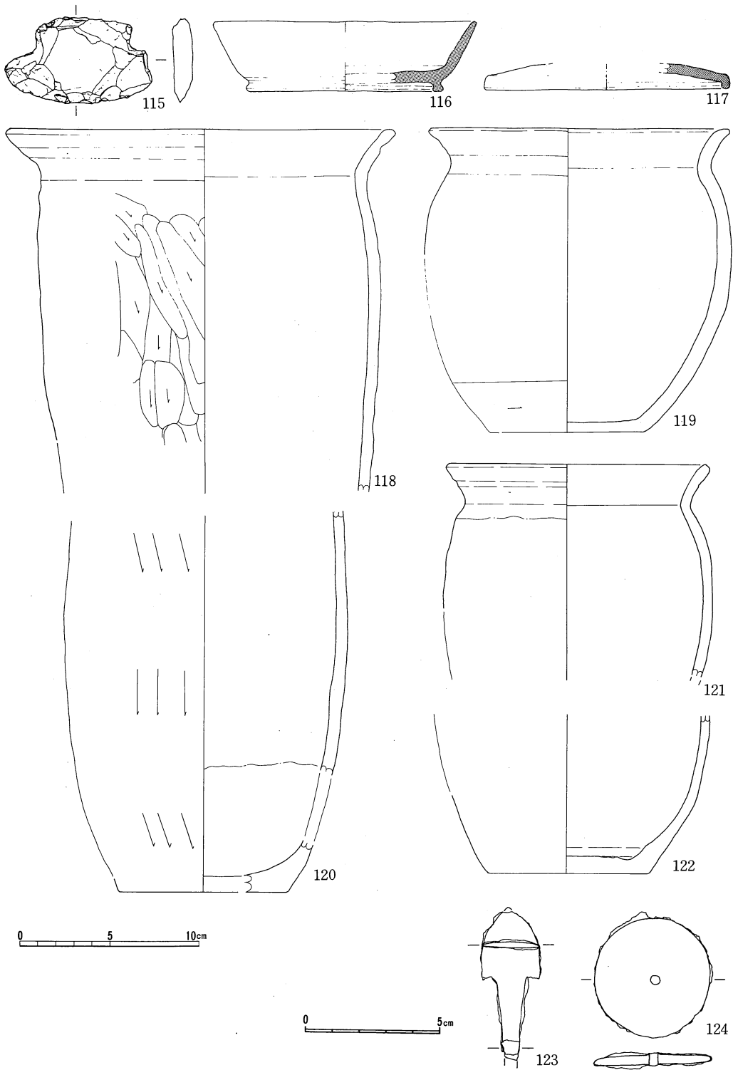
第 29 図 千鹿頭社遺跡 5 区 50 号住居跡出土遺物 1 ( S = 1/3、123・124 のみ S = 1/2 )
