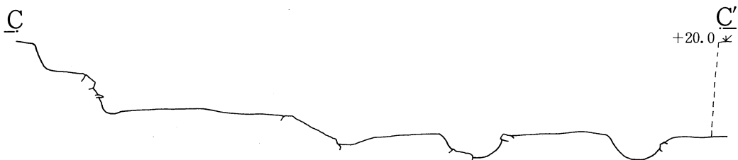
第26図 千鹿頭社遺跡5区48号A・B住居跡・エレベーション図（S=1/40）
