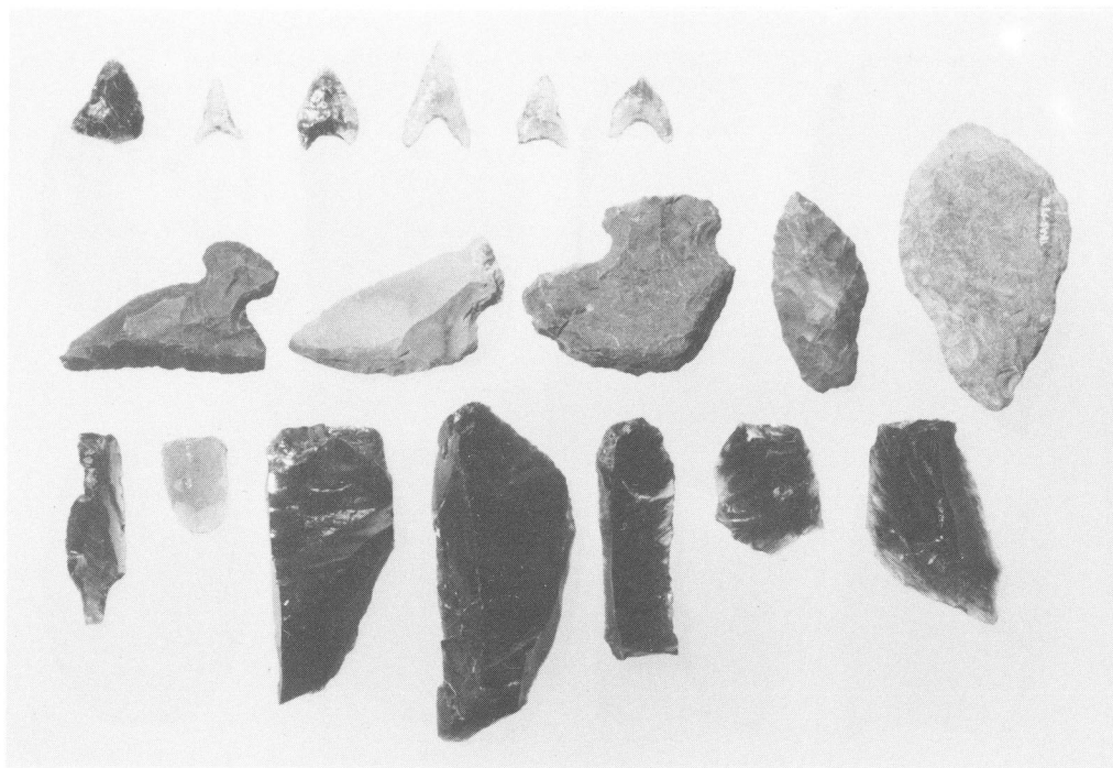
出土石器その1 (約1/2)
