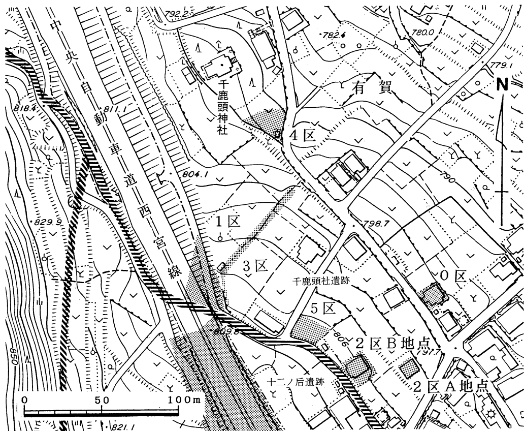
第3図 発掘区の位置 (S=1/2500)
