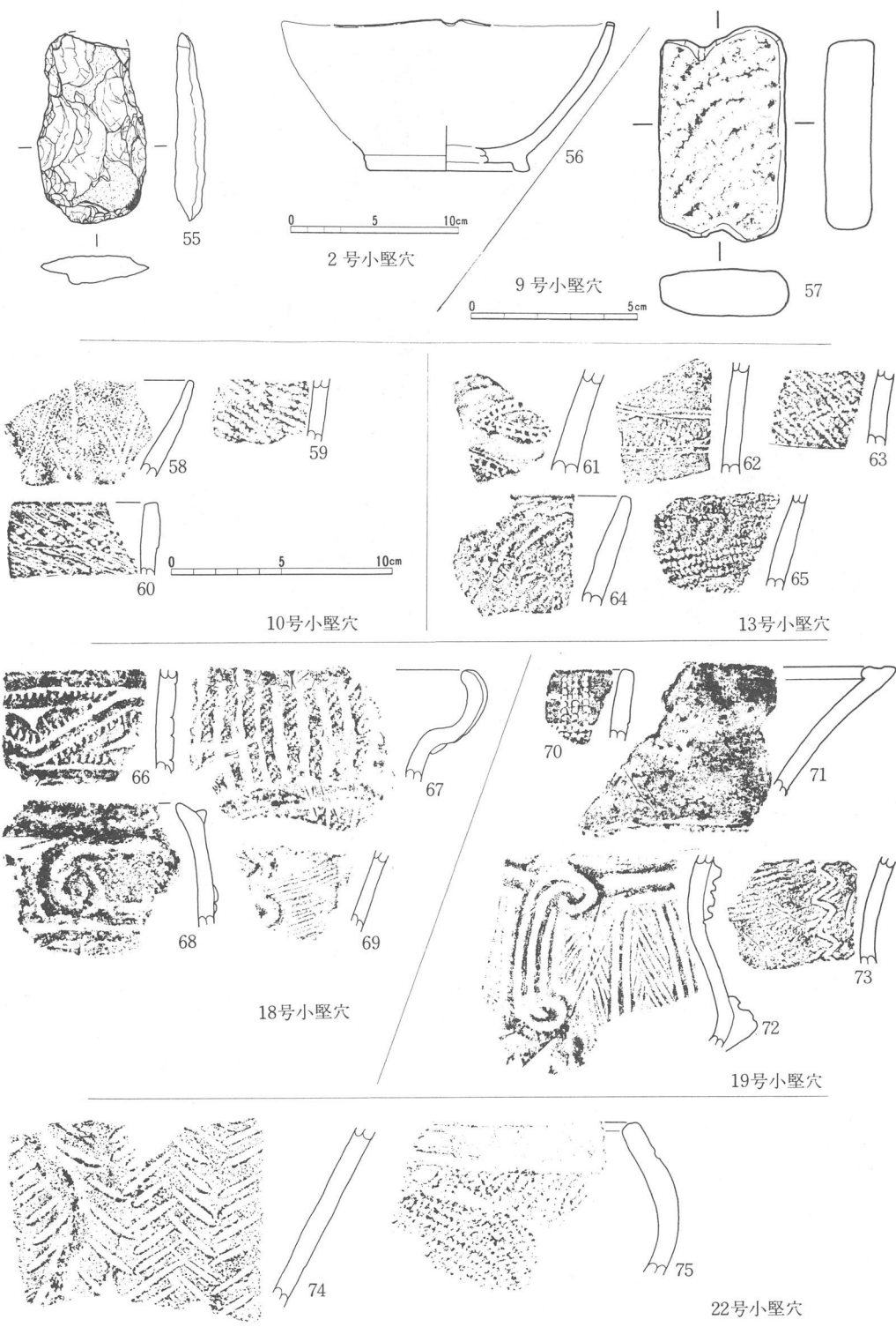
第20 図 千鹿頭社遺跡5区縄文時代等小堅穴出土遺物 (56... S = 1/4, 57... S = 1/2, 他は S = 1/3)
