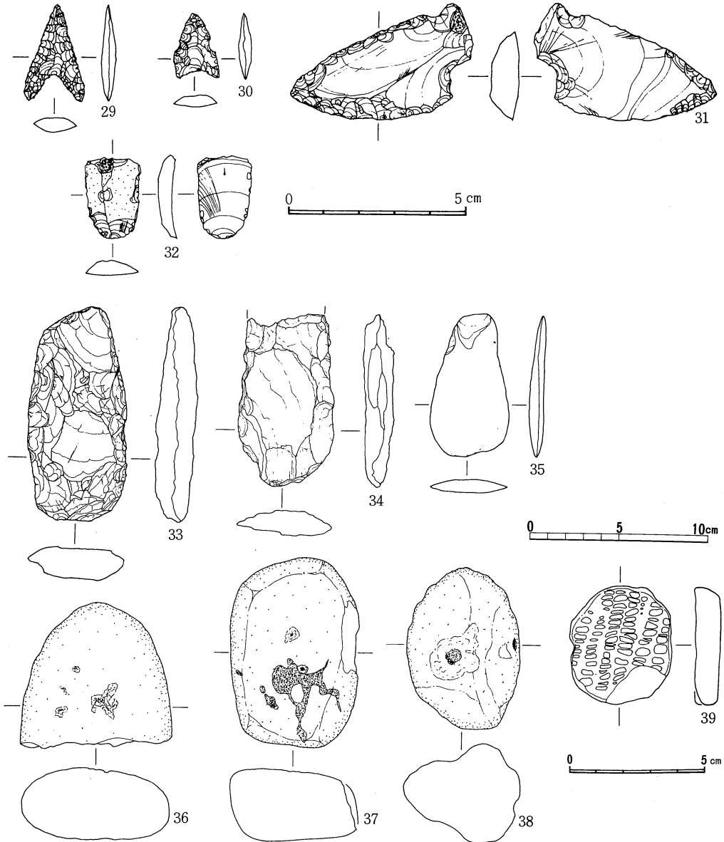
第13図 千鹿頭社遺跡52号住居跡出土遺物1 (29～32・S=2/3、33～38・S=1/3、39・S=1/2)
