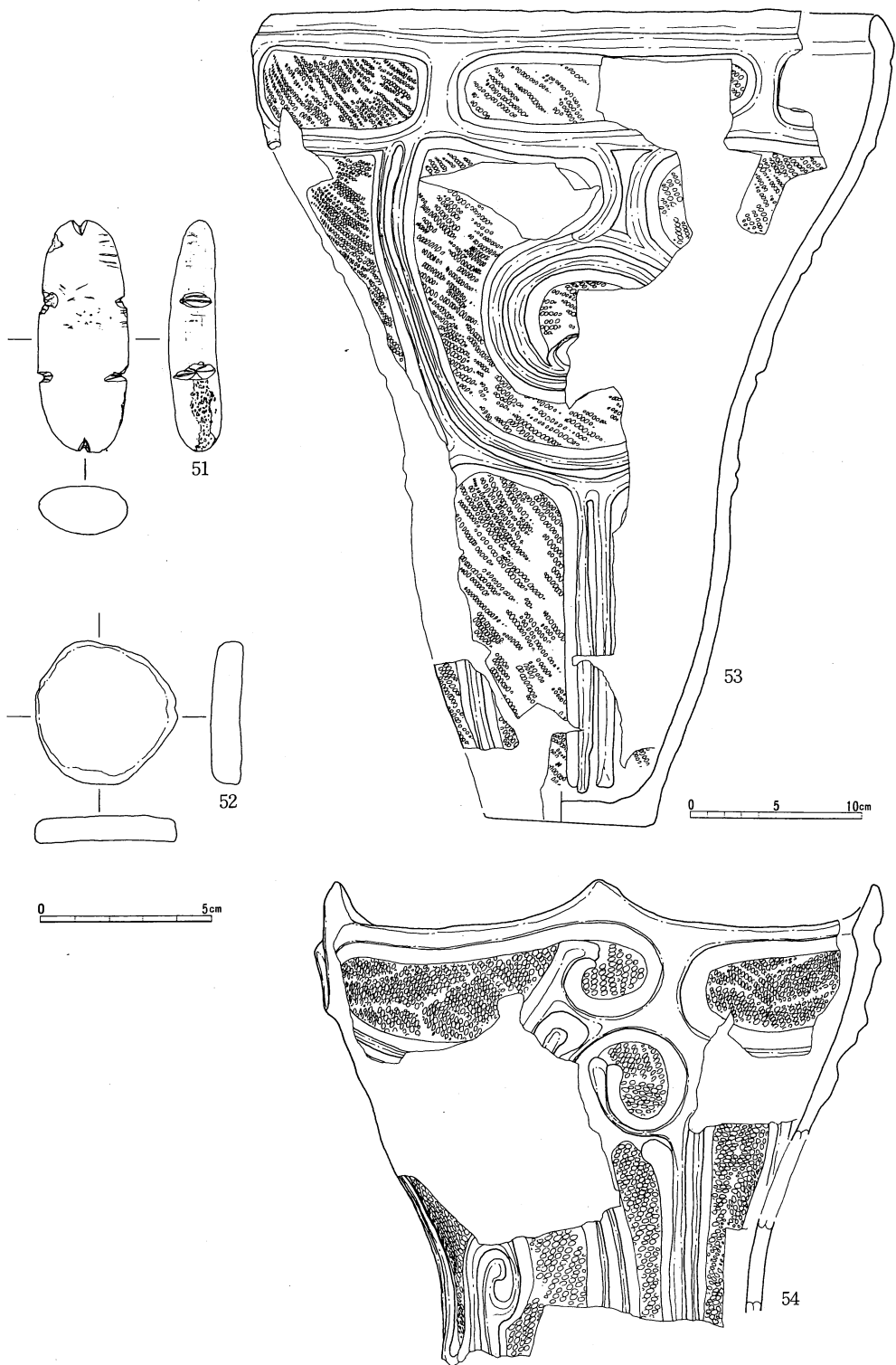
第17图 千鹿頭社5区54号住居跡出土遺物 (51・52… S=1/2、53・54… S=1/4)
