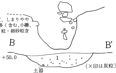
第18図 千鹿頭社遺跡5区縄文時代等小堅穴平面図・セクション図1 (S=1/40)
