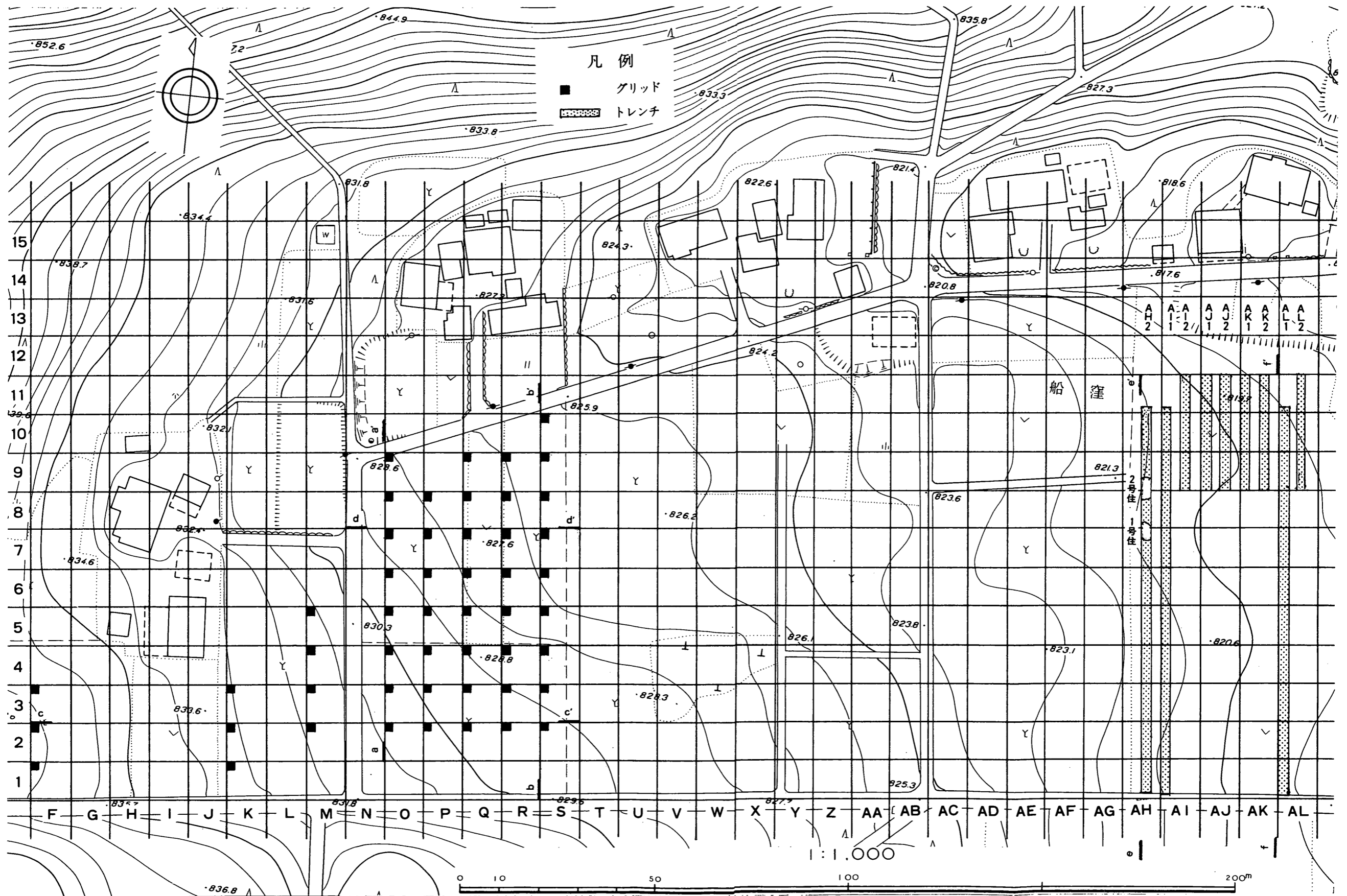
第7図 調査範囲設定及び平面実測図
