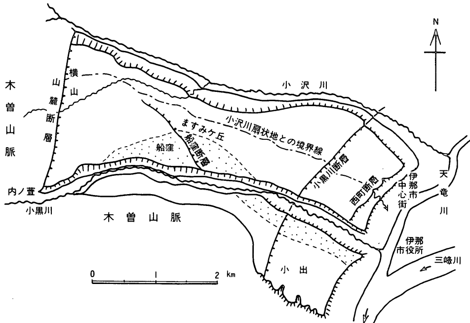
第2図 小黒川扇状地の全体図と船窪の位置
