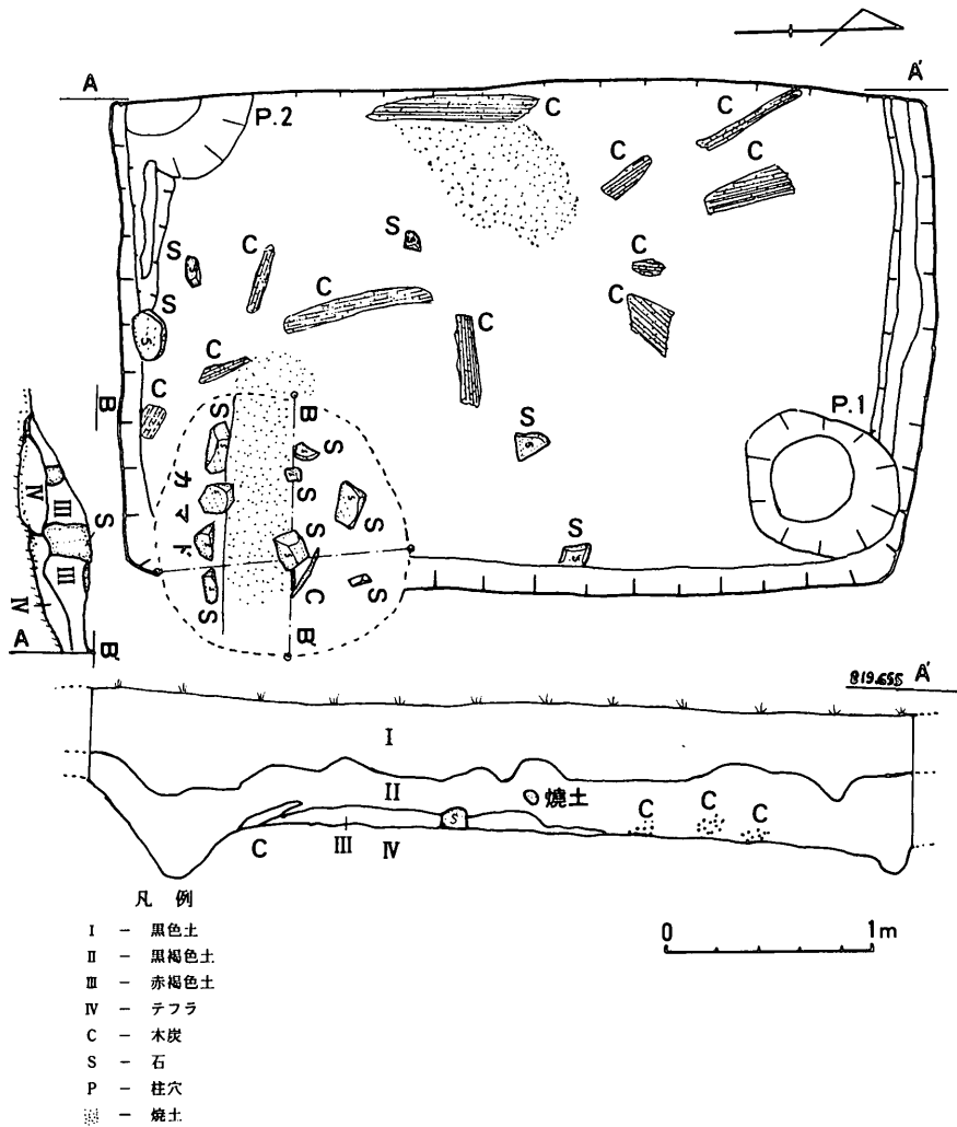
第10図 第1号住居址実測図
