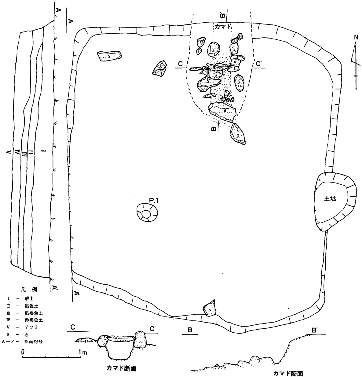
第12図 第2号住居址実測図
