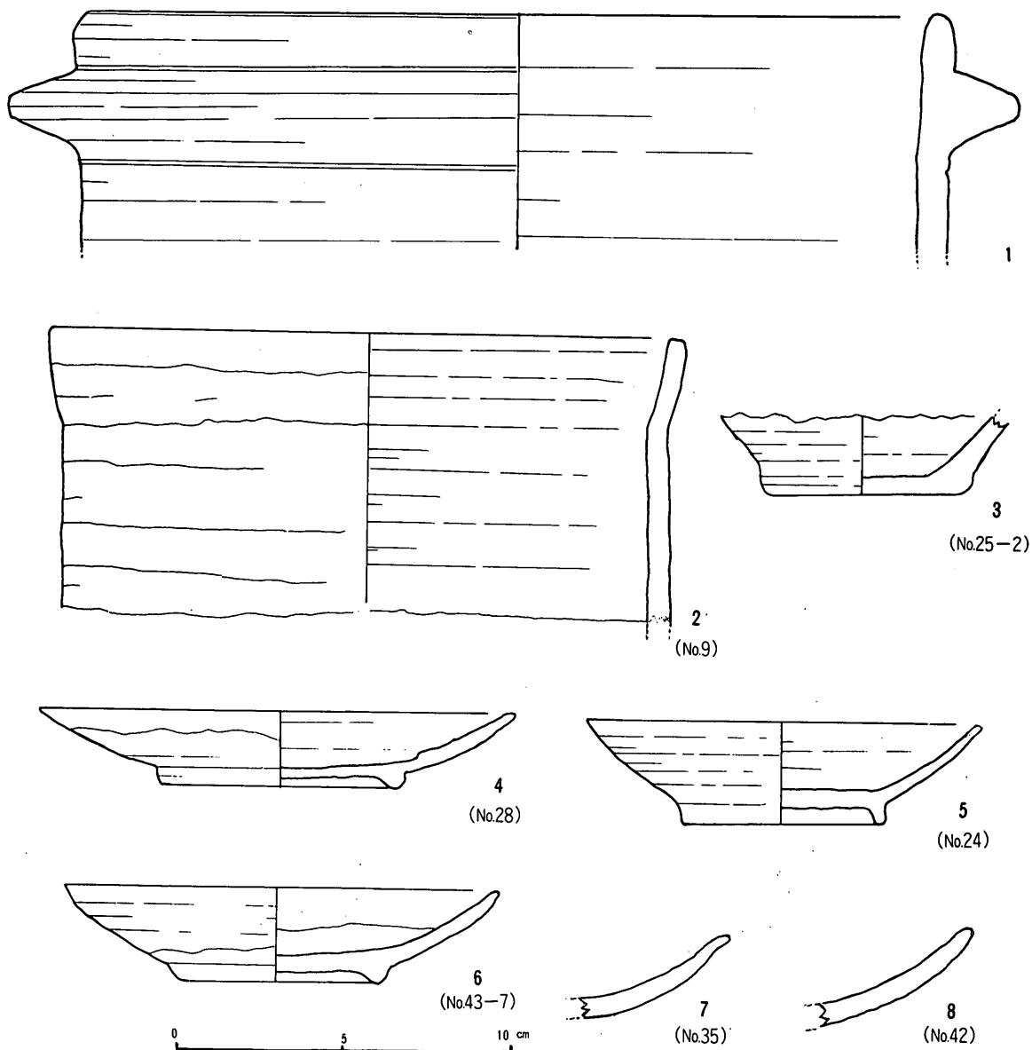
第13図 第2号住居址出土遺物実測図(1:2)
