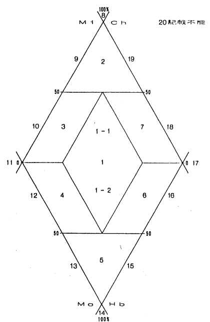
第57図 菱形ダイアグラム位置分類図
