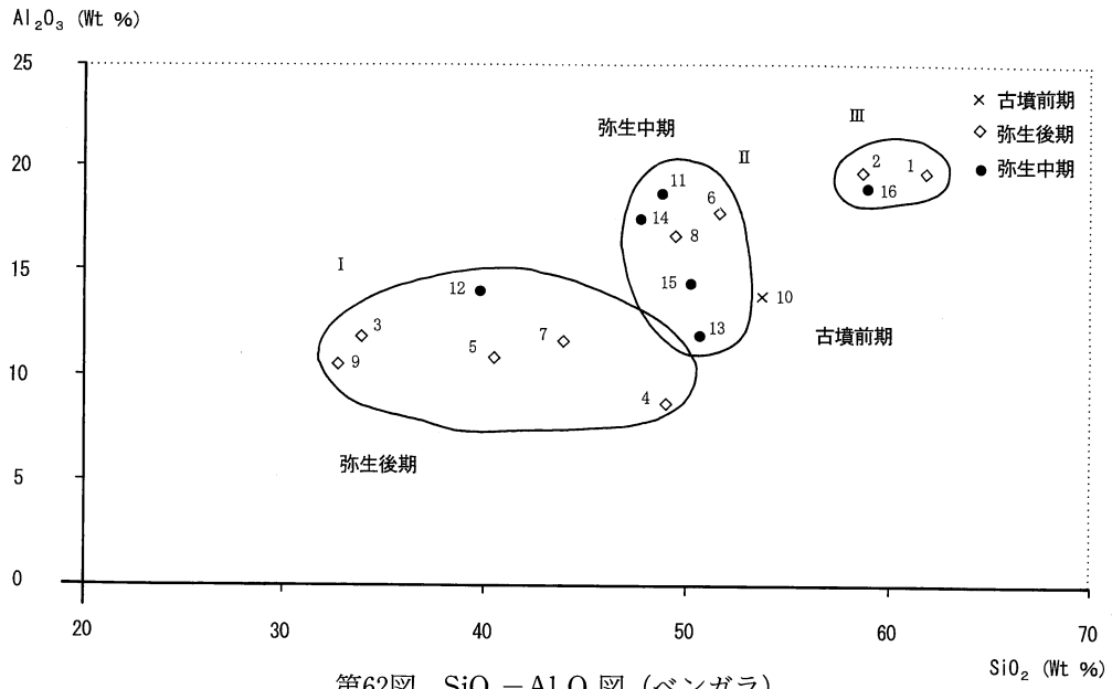
第62図 SiO_2 - Al_2O_3 図 (ベンガラ)
