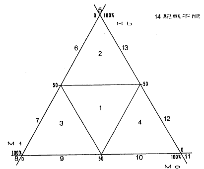
第56図 三角ダイアグラム位置分類図
