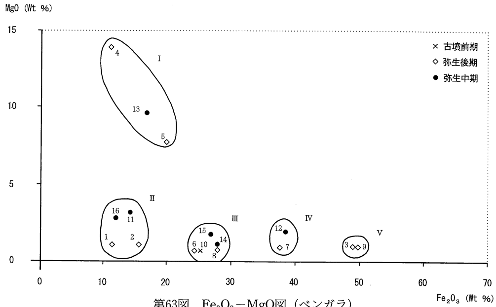
第63図 Fe_2O_3 - MgO 図 (ベンガラ)
