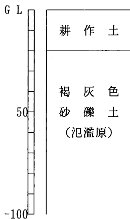
調査地標準土層柱状図
