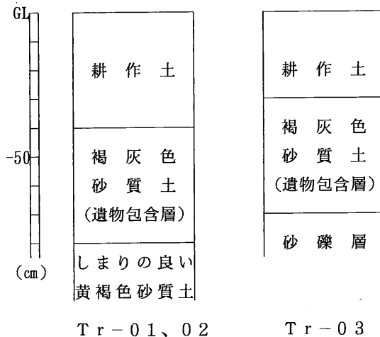
調査地標準土層柱状図
