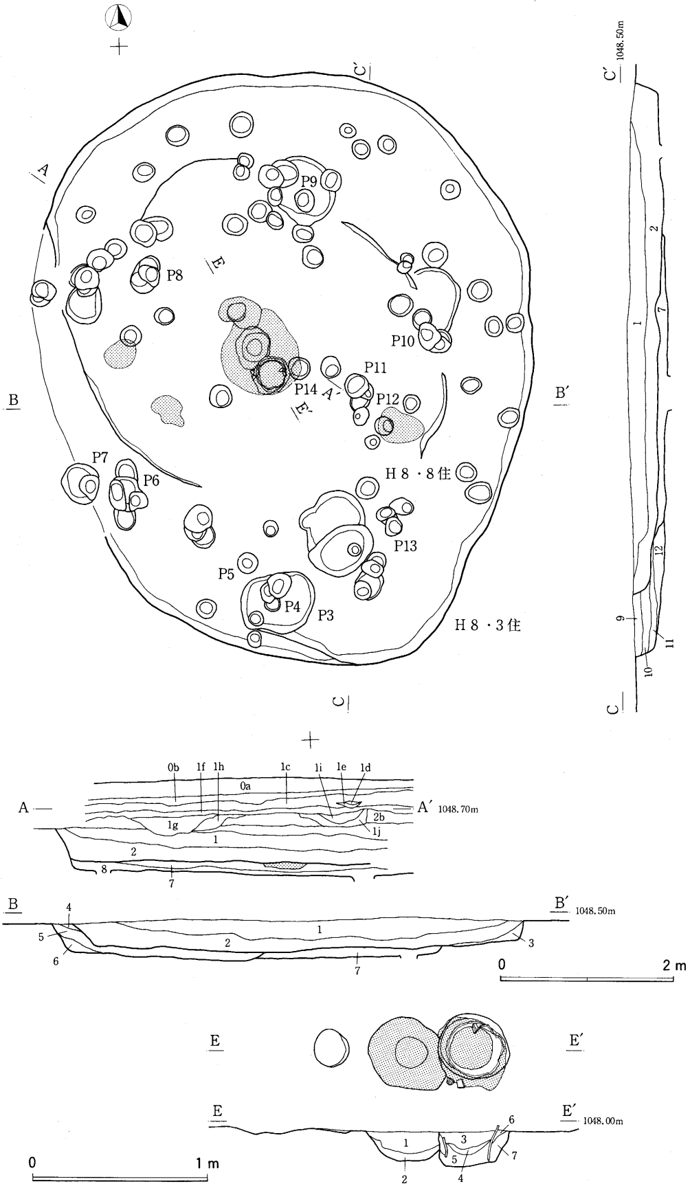
第8図 H 8 · 3号、8号住居址 (S = 1/60) と炉址 (S = 1/30)
