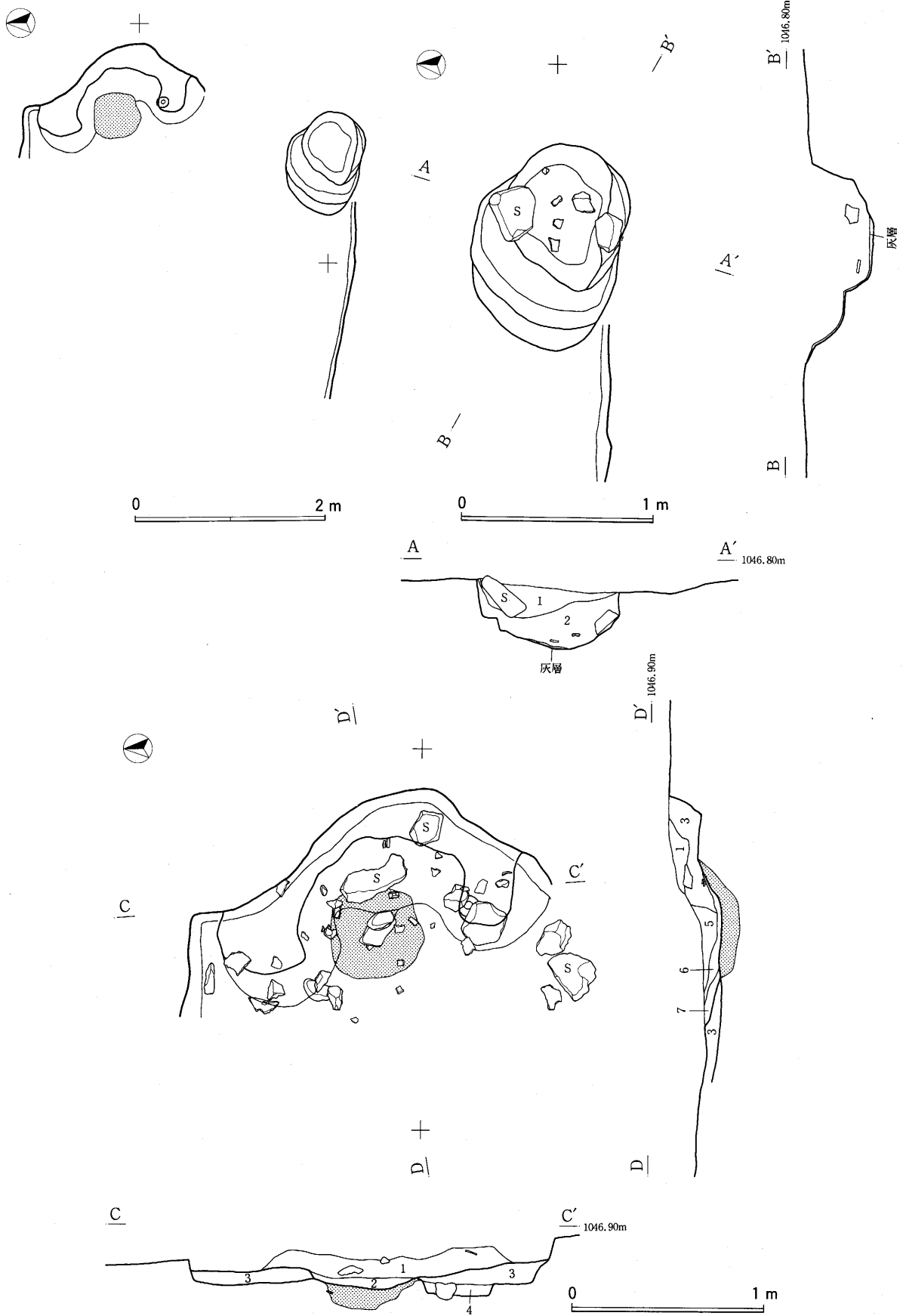
第10図 H8・6号住居址 (S = 1/60) 土壇・カマド (S = 1/30)
