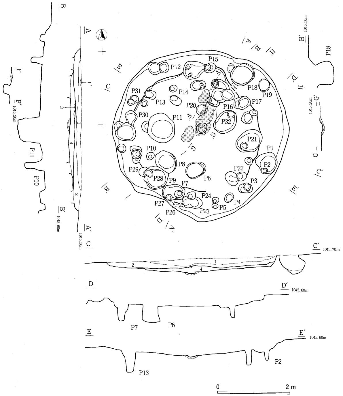
第6图 H8·1号住居址 (S = 1/60)
