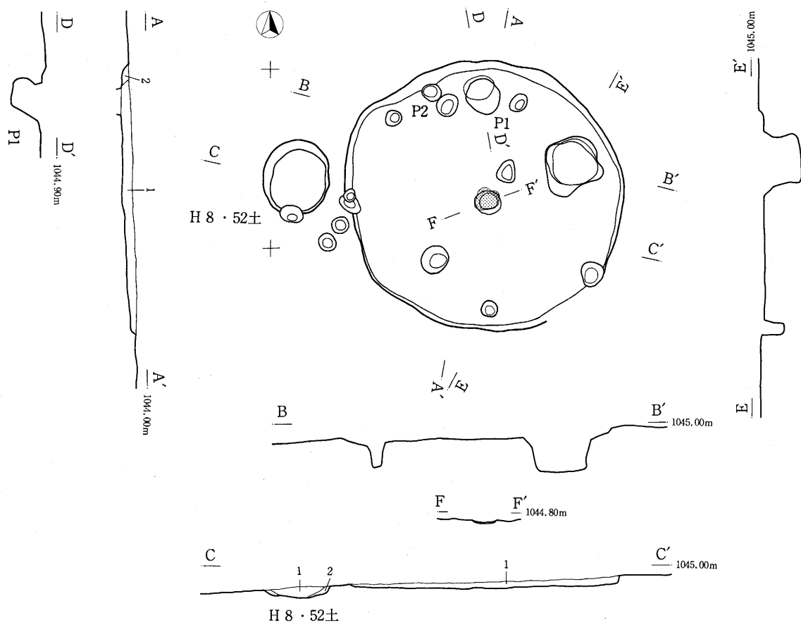
第7图 H 8 · 2号住居址、第52号土坑 (S = 1/60)
