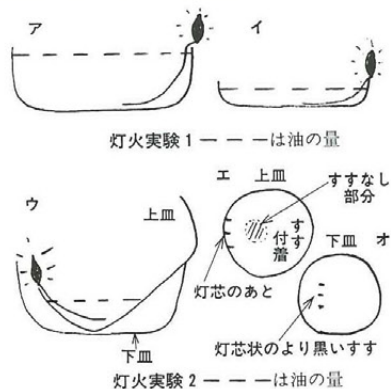
油皿を二枚使って灯をともした実験（鳥羽英継による） 一枚を傾けて使うことで少ない油でも火をつけることができた。 高価な油を使うための工夫としての可能性も考えられる。
