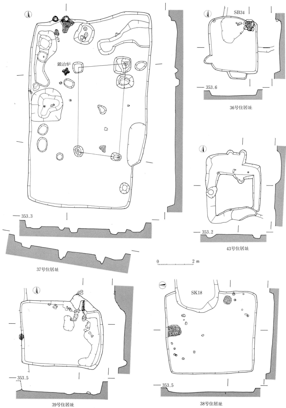
64图 F区住居址实测图 (36号·37号·38号·39号·43号)
