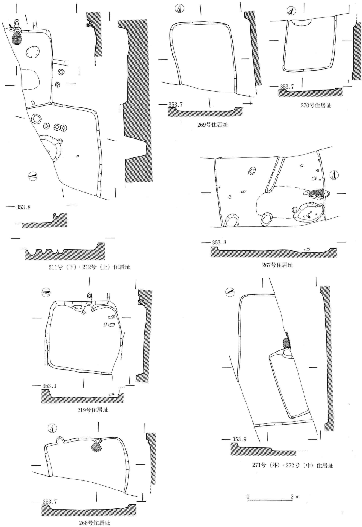
98图 I区住居址实测图(211号·212号·219号·267号·268号·269号·270号·271号·272号)
