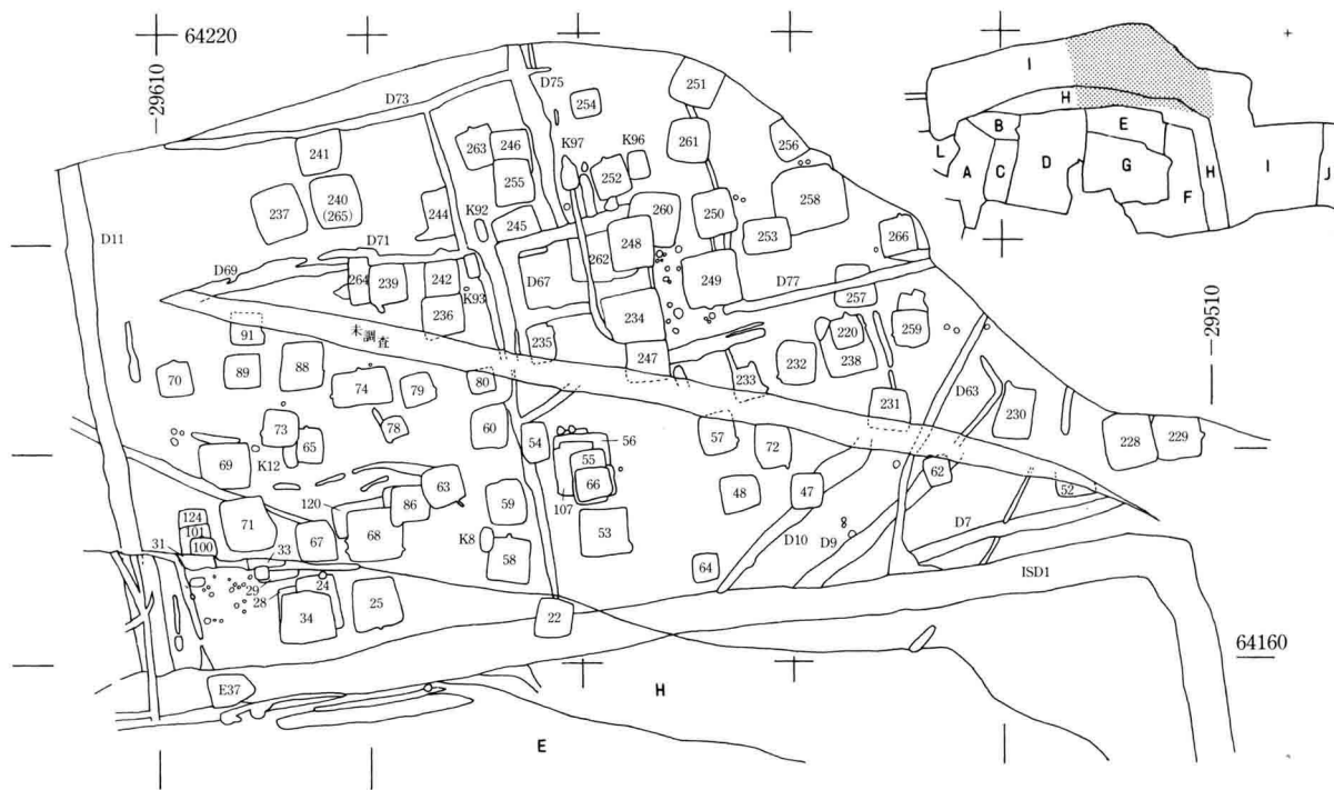
99図 第IV群I区(中)・E・H区遺構分布図(1:800)
