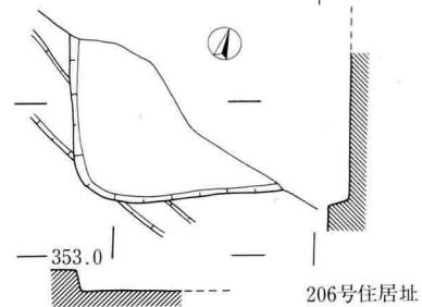
96图 I区住居址实测图(193号·194号·195号·199号·200号·204号·206号)
