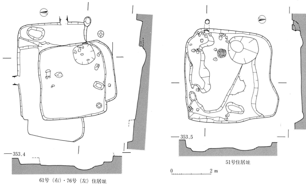
83図 I区住居址実測図(51号・61号・76号)
