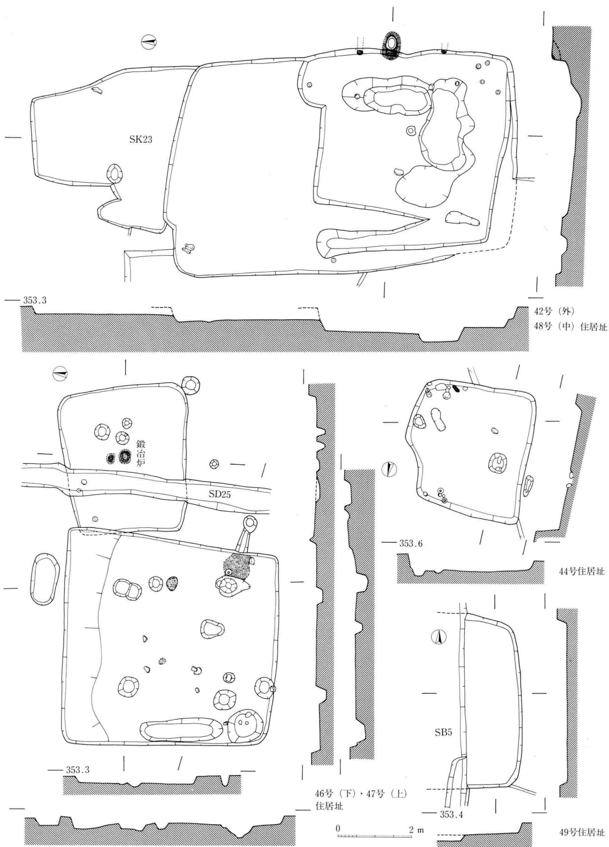
65图 F区住居址实测图 (42号·44号·46号·47号·48号·49号)
