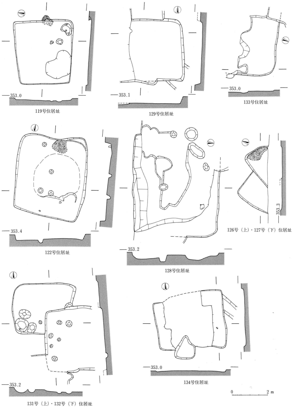
92图 I区住居址实测图(119号·122号·126号·127号·128号·129号·131号·132号·133号·134号)
