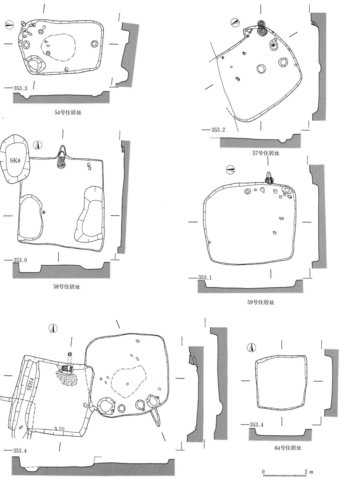
102图 I区住居址实测图 (54号·57号·58号·59号·63号·64号·86号)
