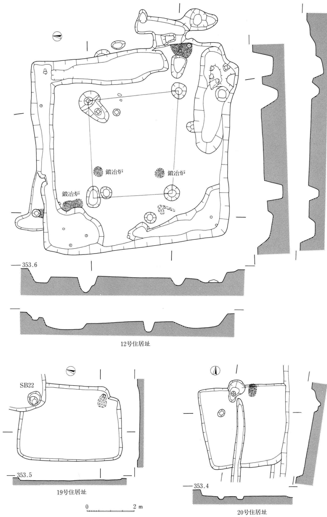
71图 G区住居址实测图 (12号·19号·20号)
