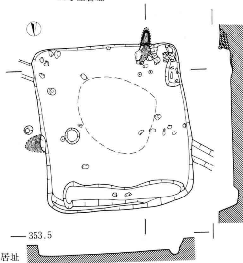
76图 H区住居址实测图 (26号·27号·30号·35号·36号·38号·39号)
