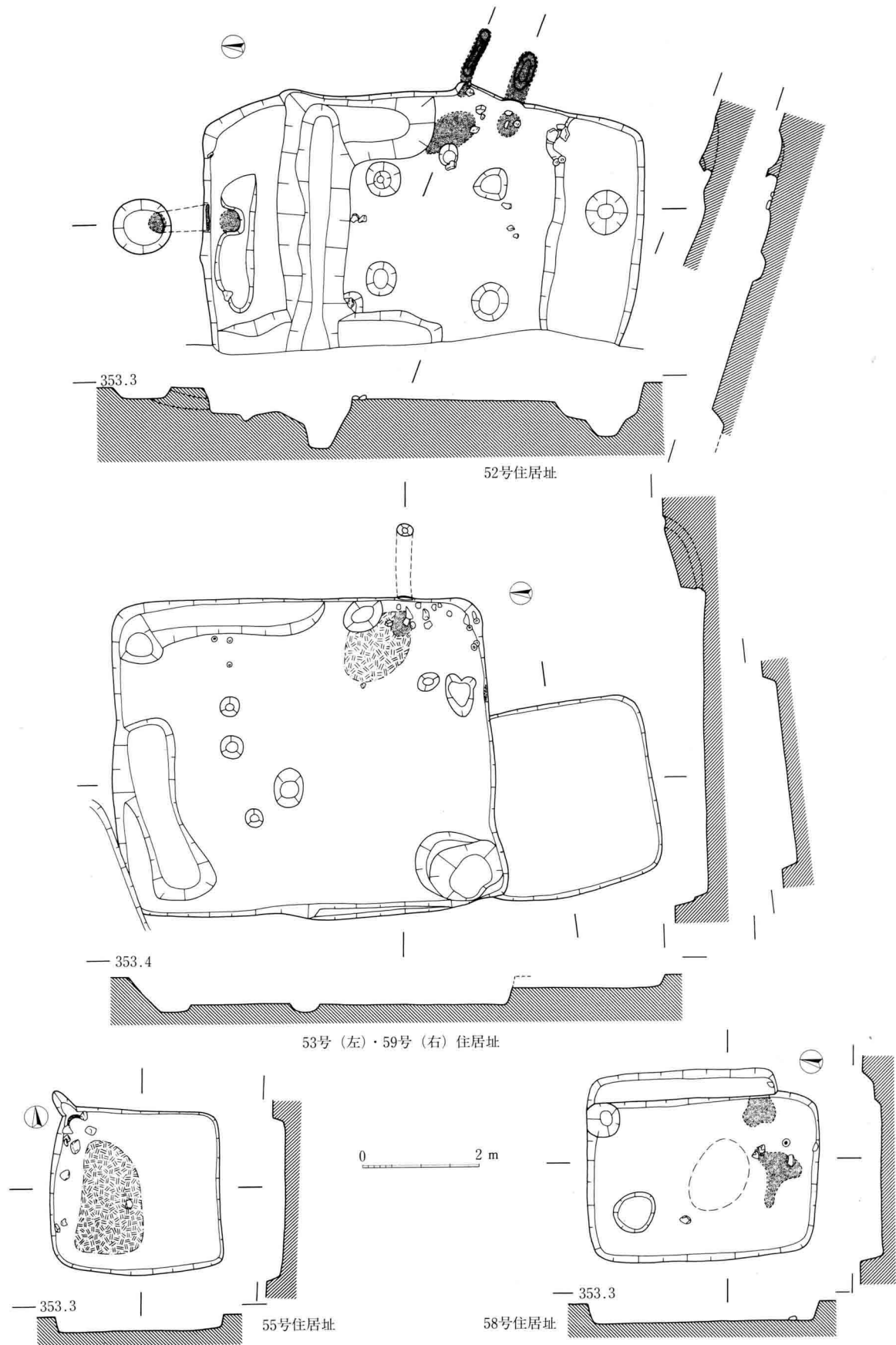
79图 H区住居址实测图 (52号·53号·55号·58号·59号)
