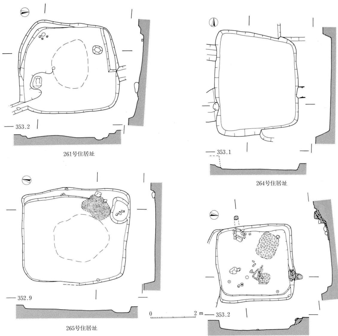
111图 I区住居址实测图 (261号·264号·265号·266号)
