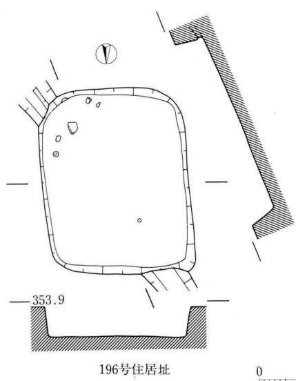
95图 I区住居址实测图(190号·191号·192号·196号·197号·198号)
