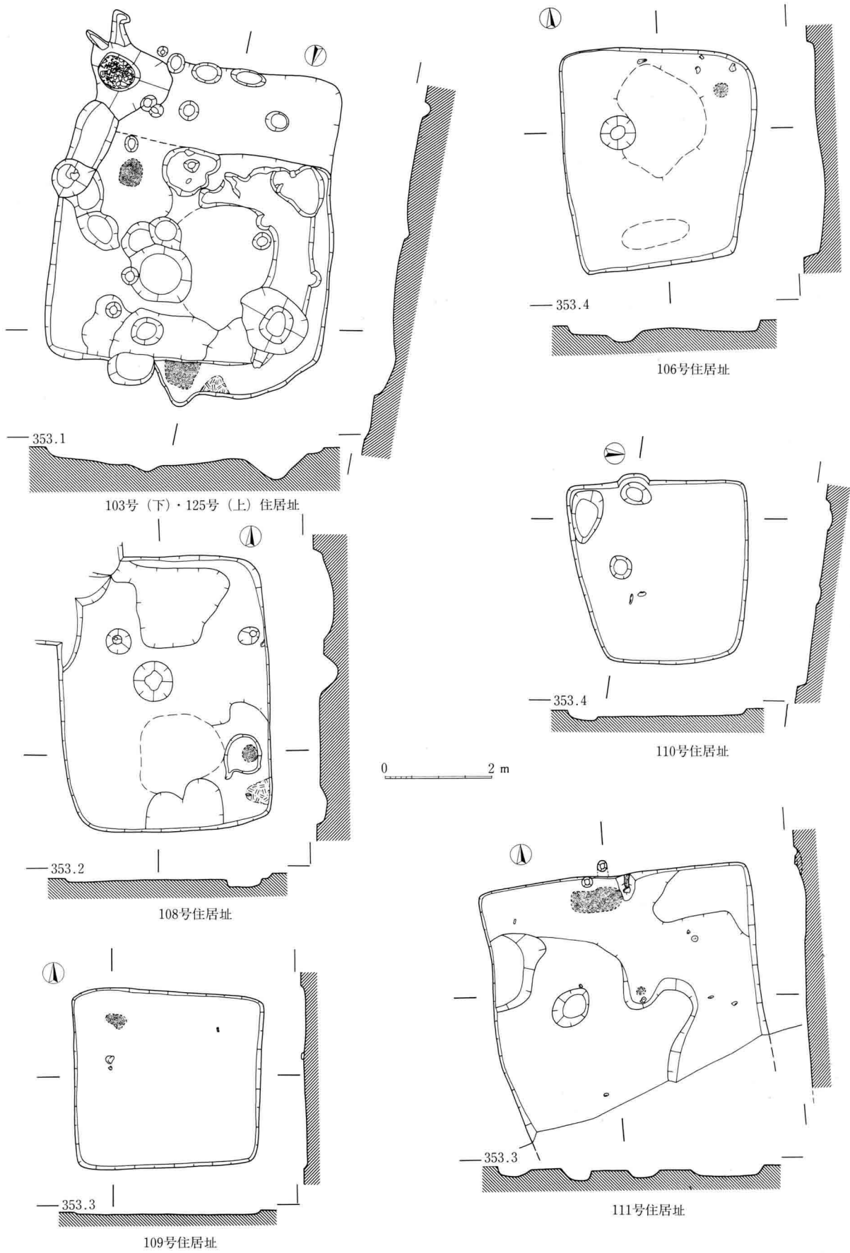
90图 I区住居址实测图(103号·106号·108号·109号·110号·111号·125号)
