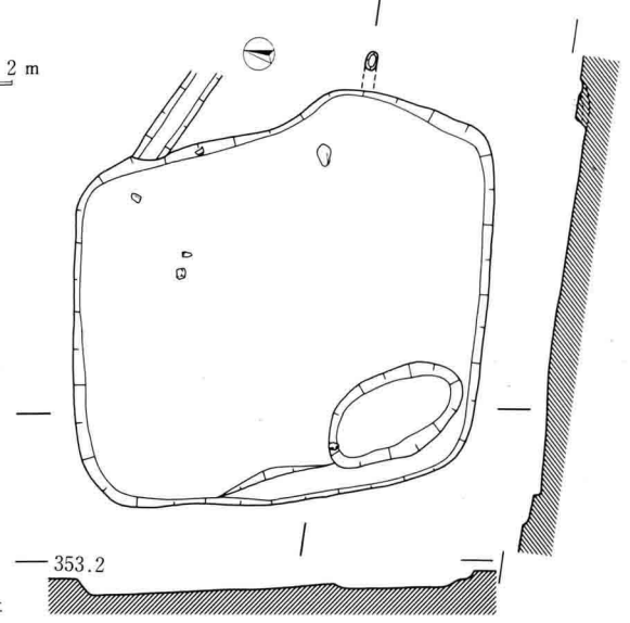
103图 I区住居址实测图(60号·67号·68号·69号·70号·71号)
