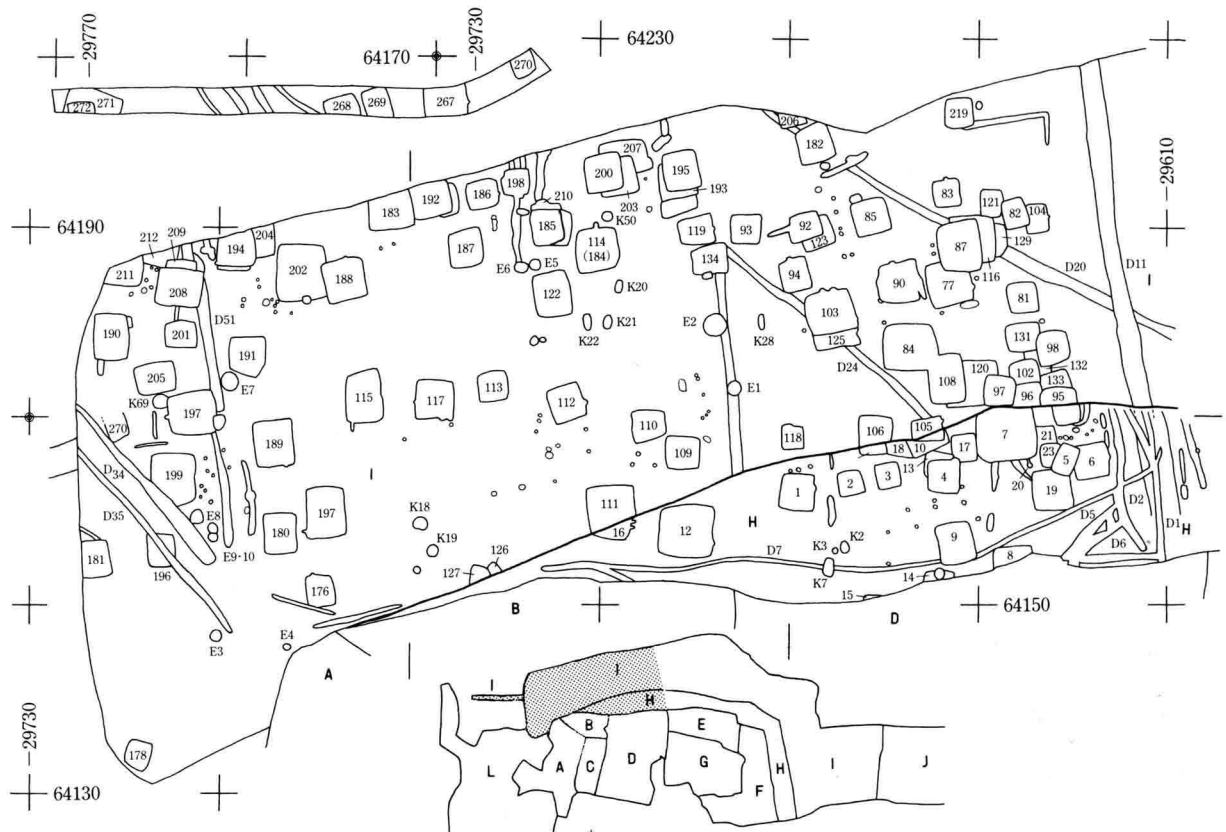
84図 第三群I区、H区西遺構分布図(1:800)
