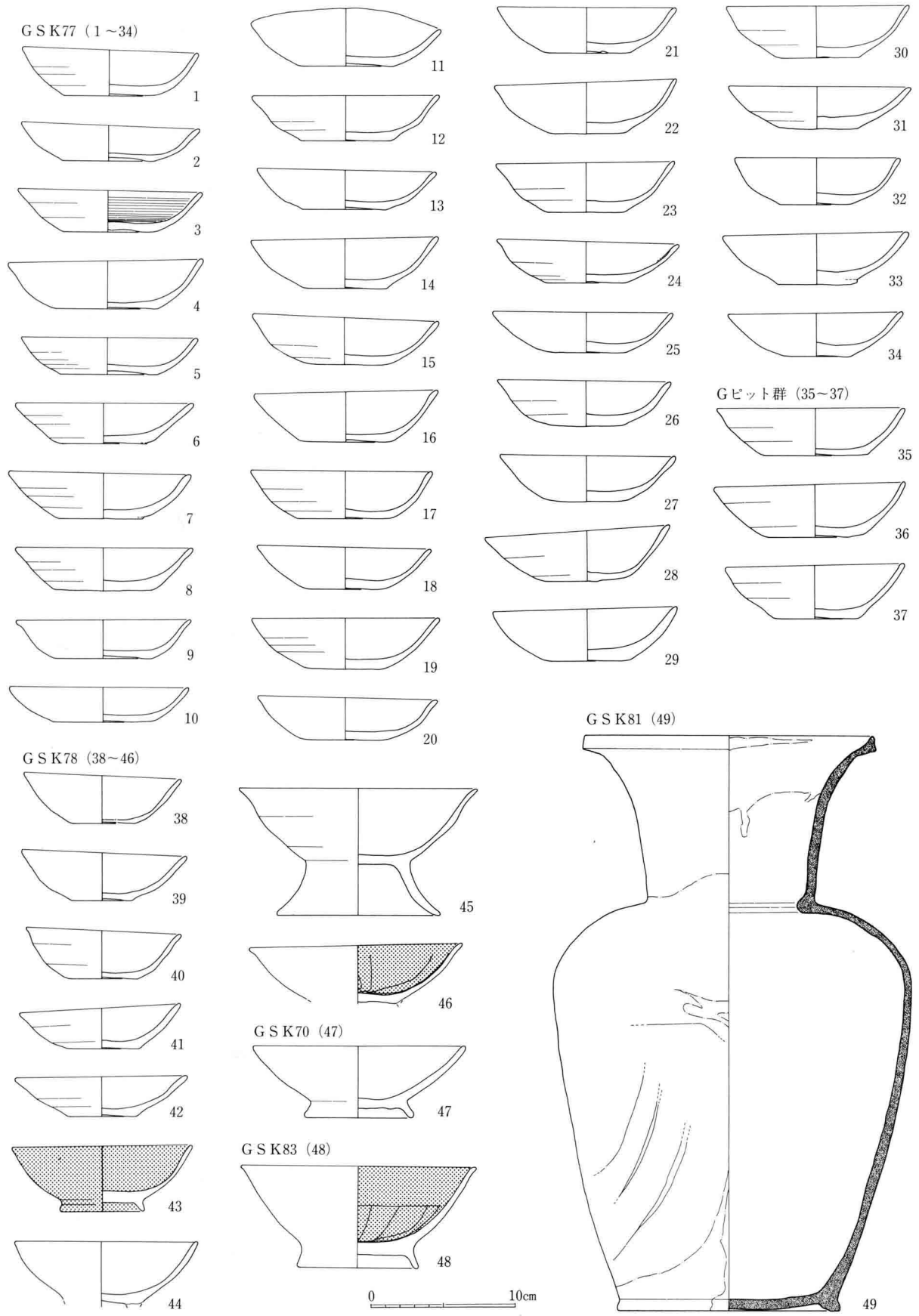
249図 GSK70・77・78・81・83, Gピット群出土土器実測図(1:4)
