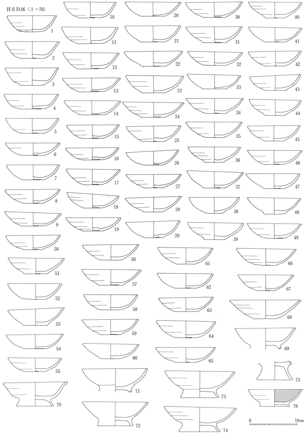
256图 HSD36出土土器实测图(1:4)
