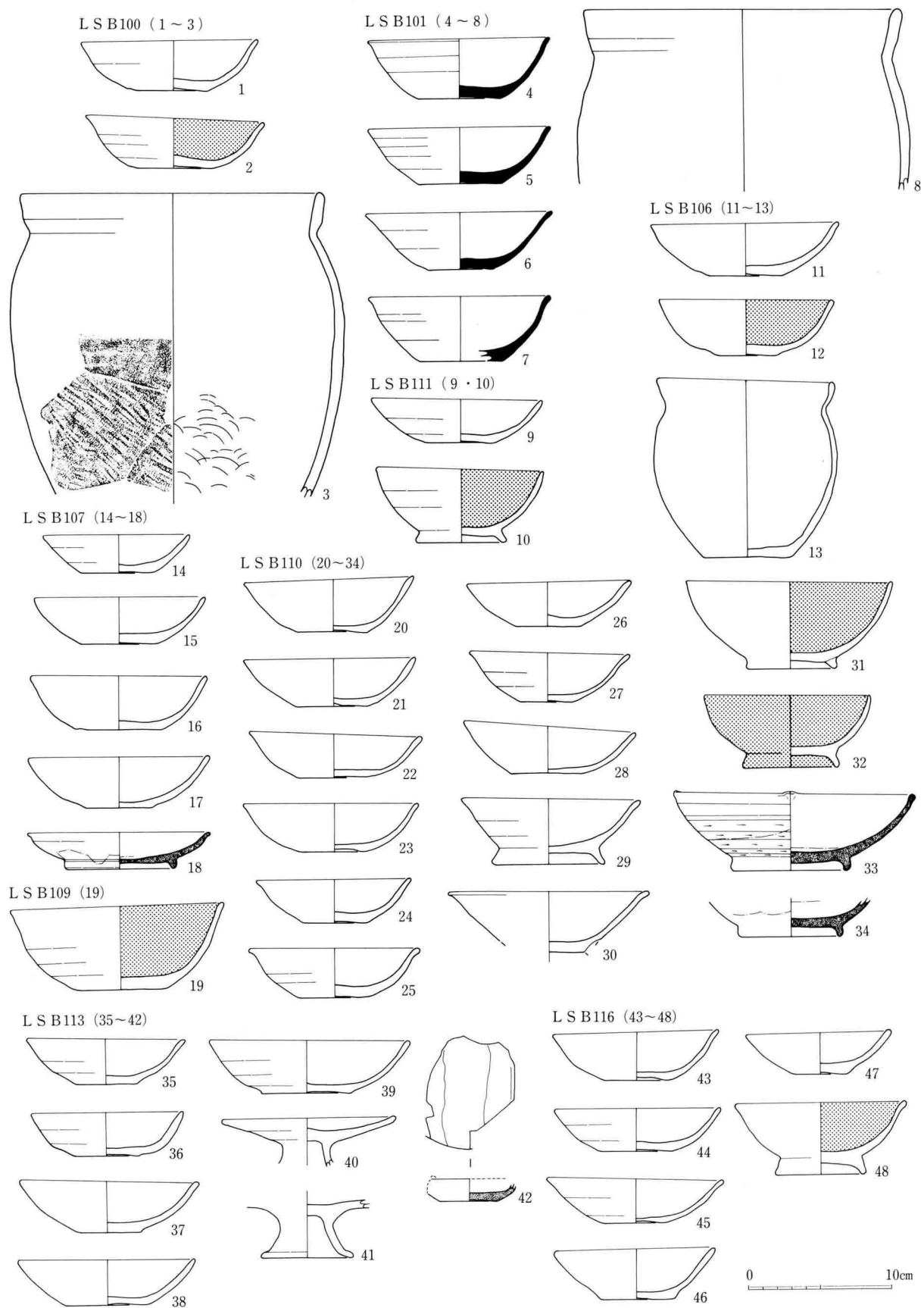
223図 L S B 100・101・106・107・109~111・113・116出土土器実測図(1:4)
