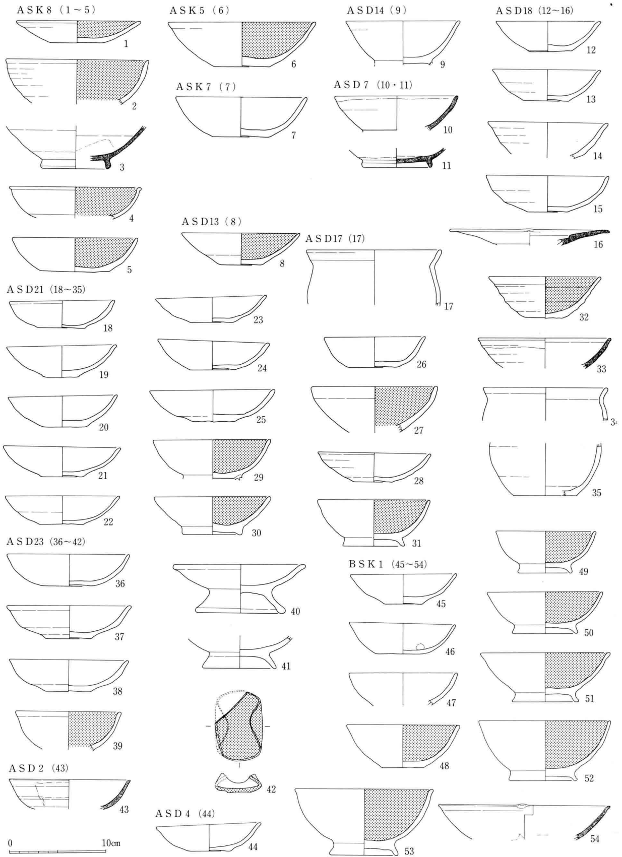
232图 ASK 5·7·8, ASD 2·4·7·13·14·17·18·21·23, BSK 1出土土器实测图(1:4)
