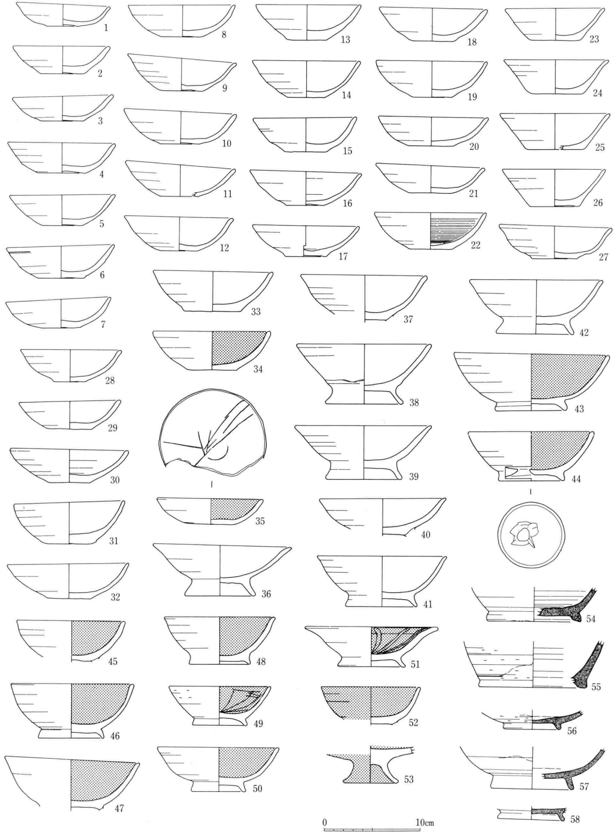
241图 ESD 1 出土土器实测图 (1:4)
