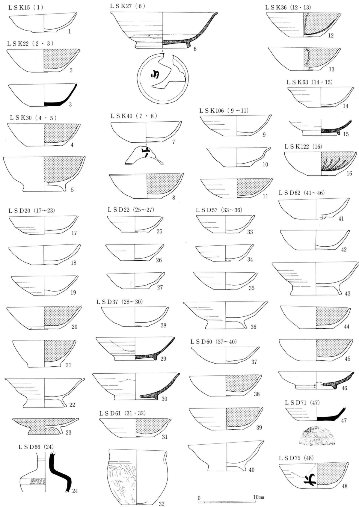
264图 LSK15·22·27·30·36·40·63·106·122, LSD20·22·37·57·60~62·66·71·75出土土器实测图(1:4)
