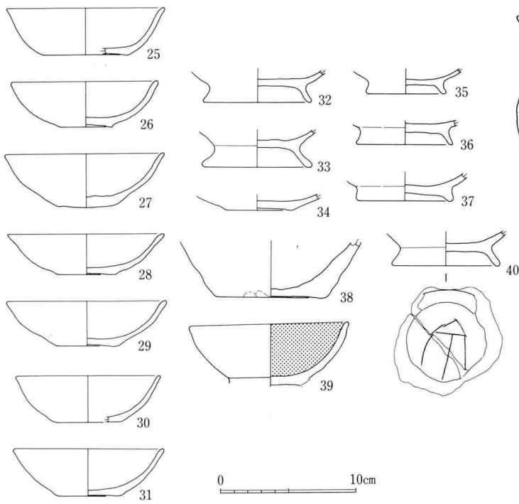
233图 BSK 4 · 11, CSK 2 · 8, CSD 6 · 12出土土器实测图 (1 : 4)
