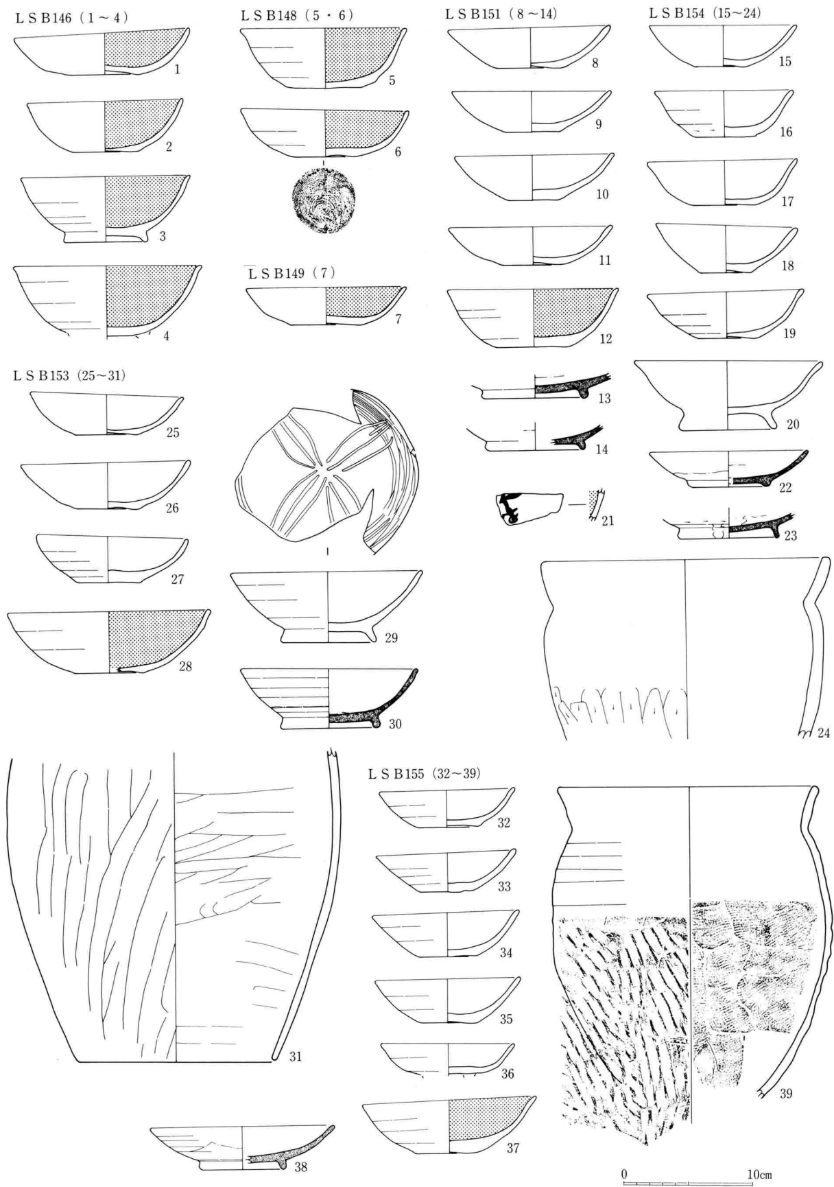
227图 LSB146·148·149·151·153~155出土土器实测图(1:4)
