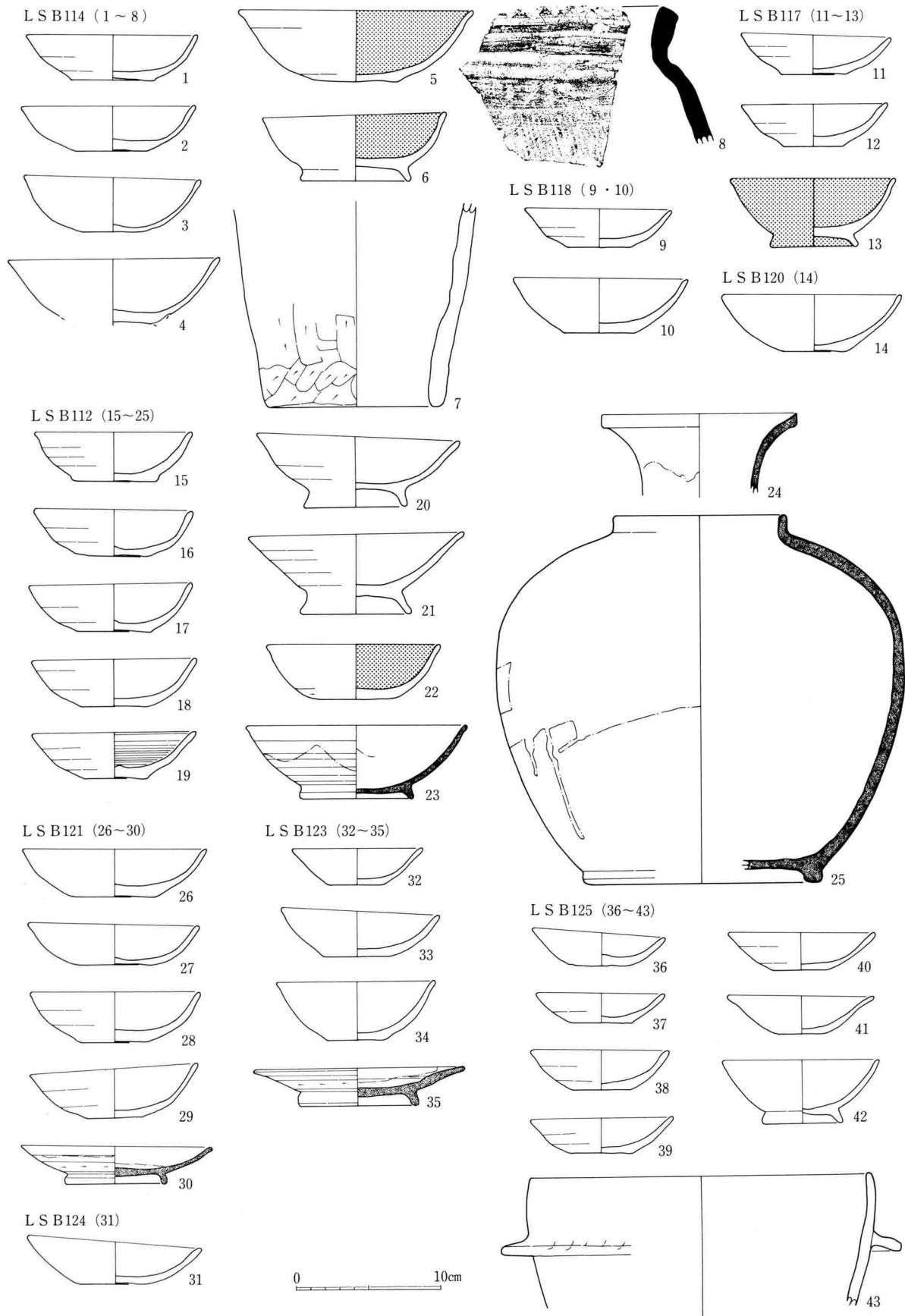
224図 LS B112・114・117・118・120・121・123~125出土土器実測図(1:4)
