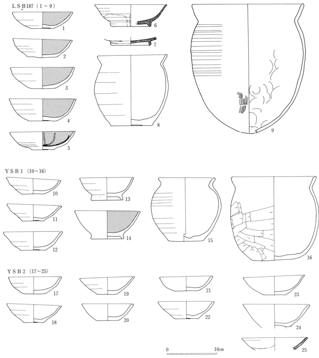
231图 LSB187, YSB 1・2 出土土器实测图 (1:4)
