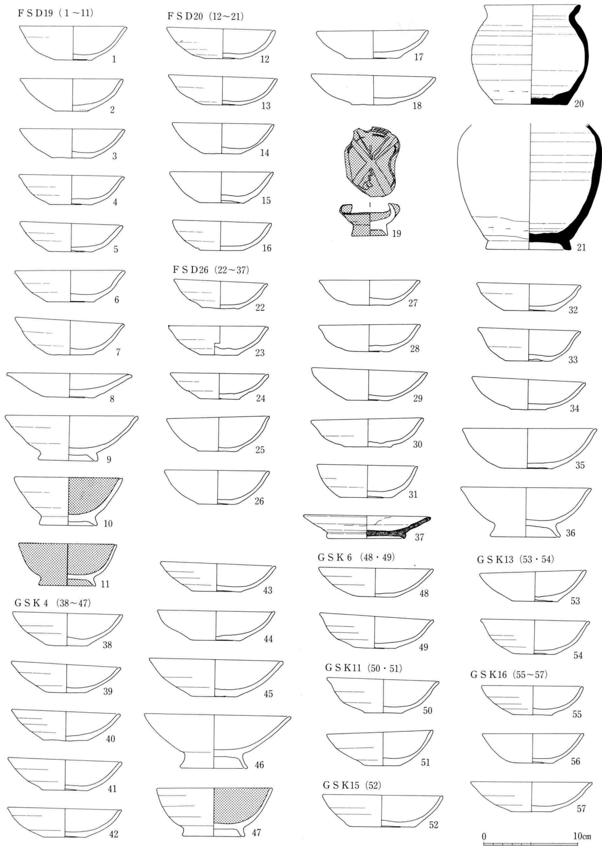
245图 FSD19·20·26, GSK4·6·11·13·15·16出土土器实测图(1:4)
