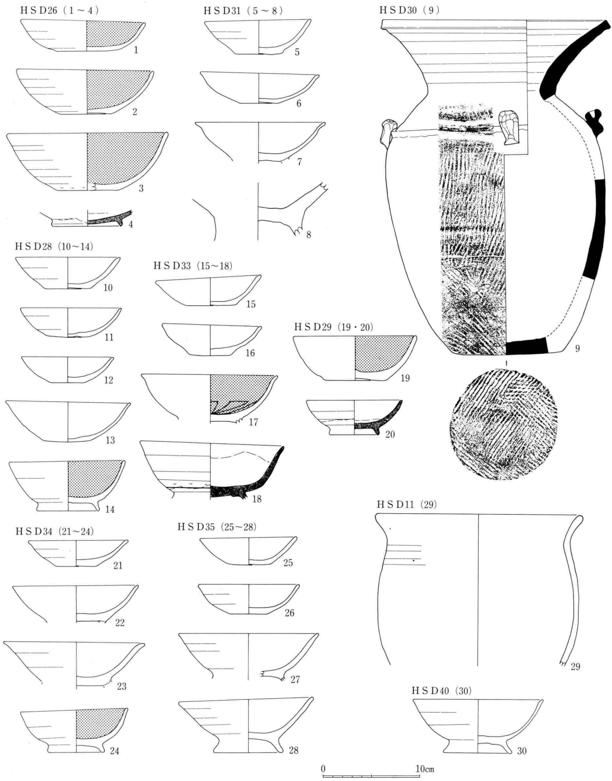
257图 HSD11·26·28~31·33~35·40出土土器实测图(1:4)
