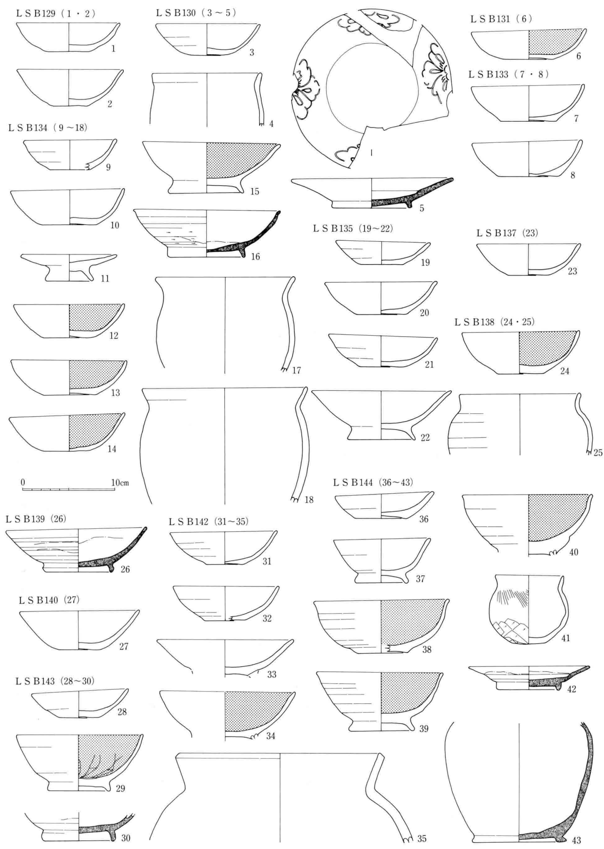
226図 LS B129~131 · 133~135 · 137~140 · 142~144出土土器実測図 (1 : 4)
