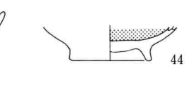
218图 LSB44·47·49·52~55·57出土土器实测图(1:4)
