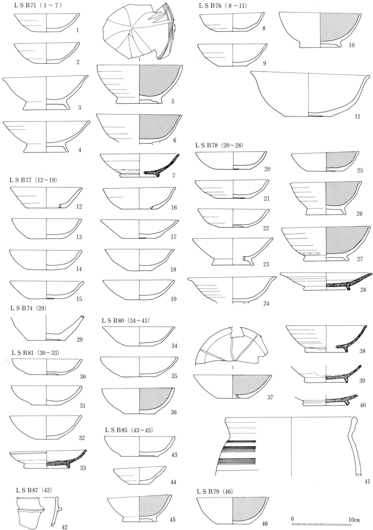
220图 LSB71・74・76~81・85・87出土土器实测图(1:4)
