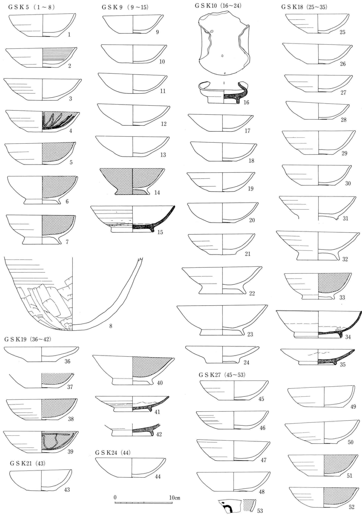
246图 GSK 5 · 9 · 10 · 18 · 19 · 21 · 24 · 27出土土器实测图 (1 : 4)
