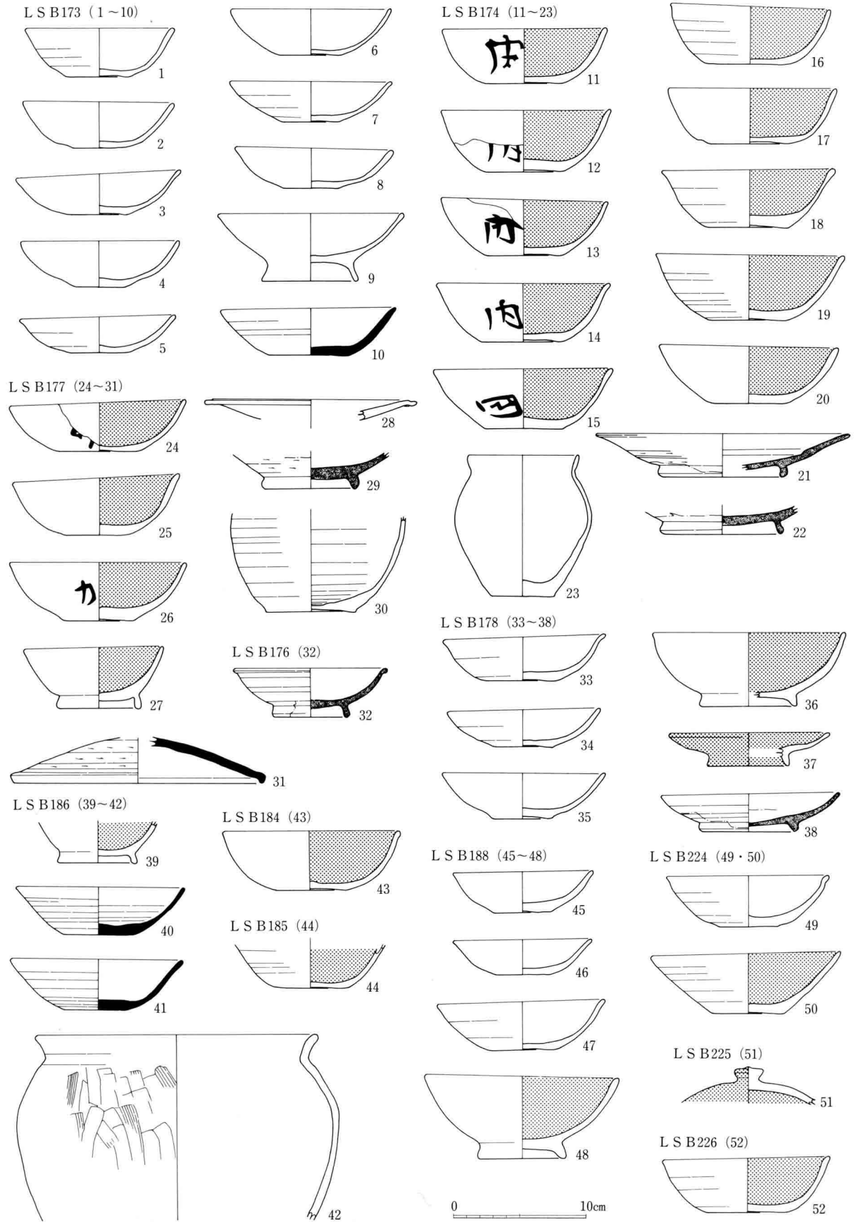
230図 LS B173・174・176~178・184~186・188・224~226出土土器実測図(1:4)
