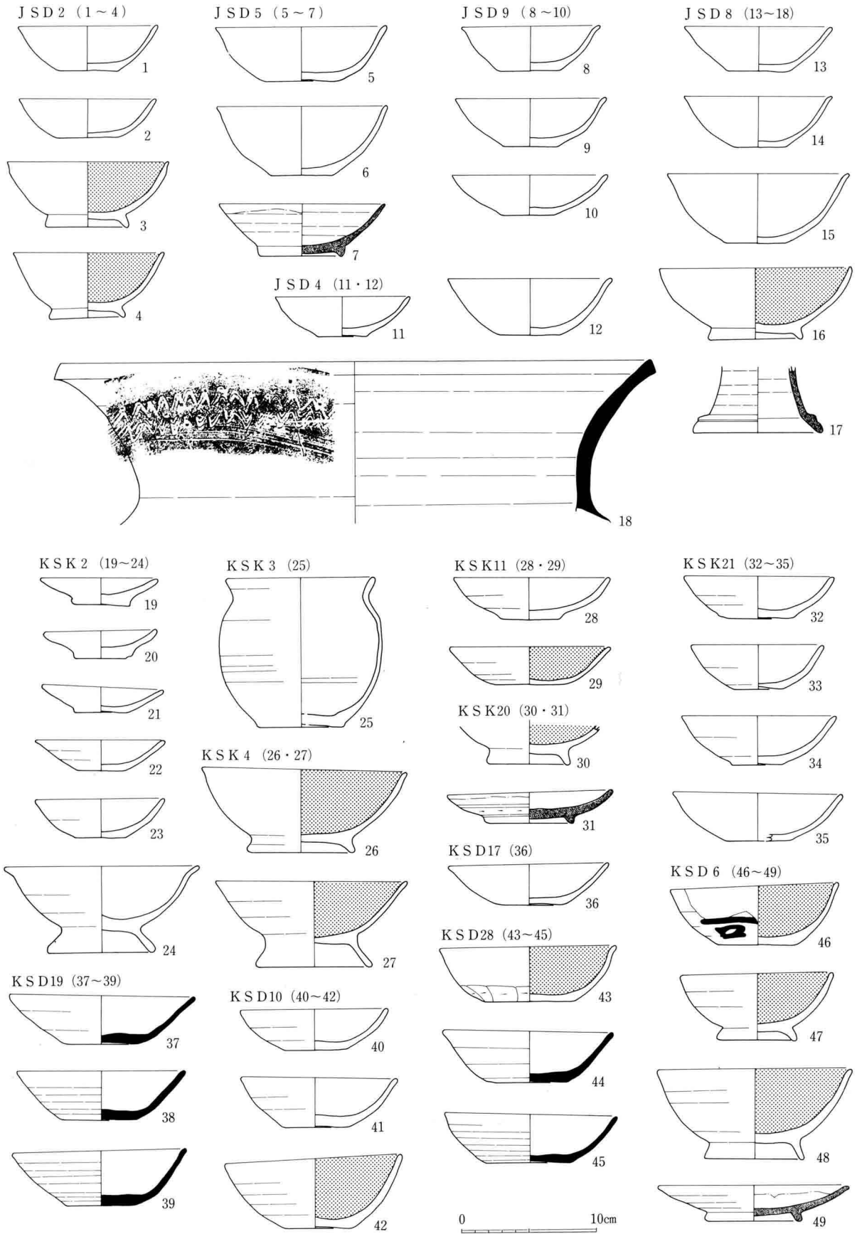
263図 JSD 2・4・5・8・9, KSK 2~4・11・20・21, KSD 6・10・17・19・28出土土器実測図(1:4)
