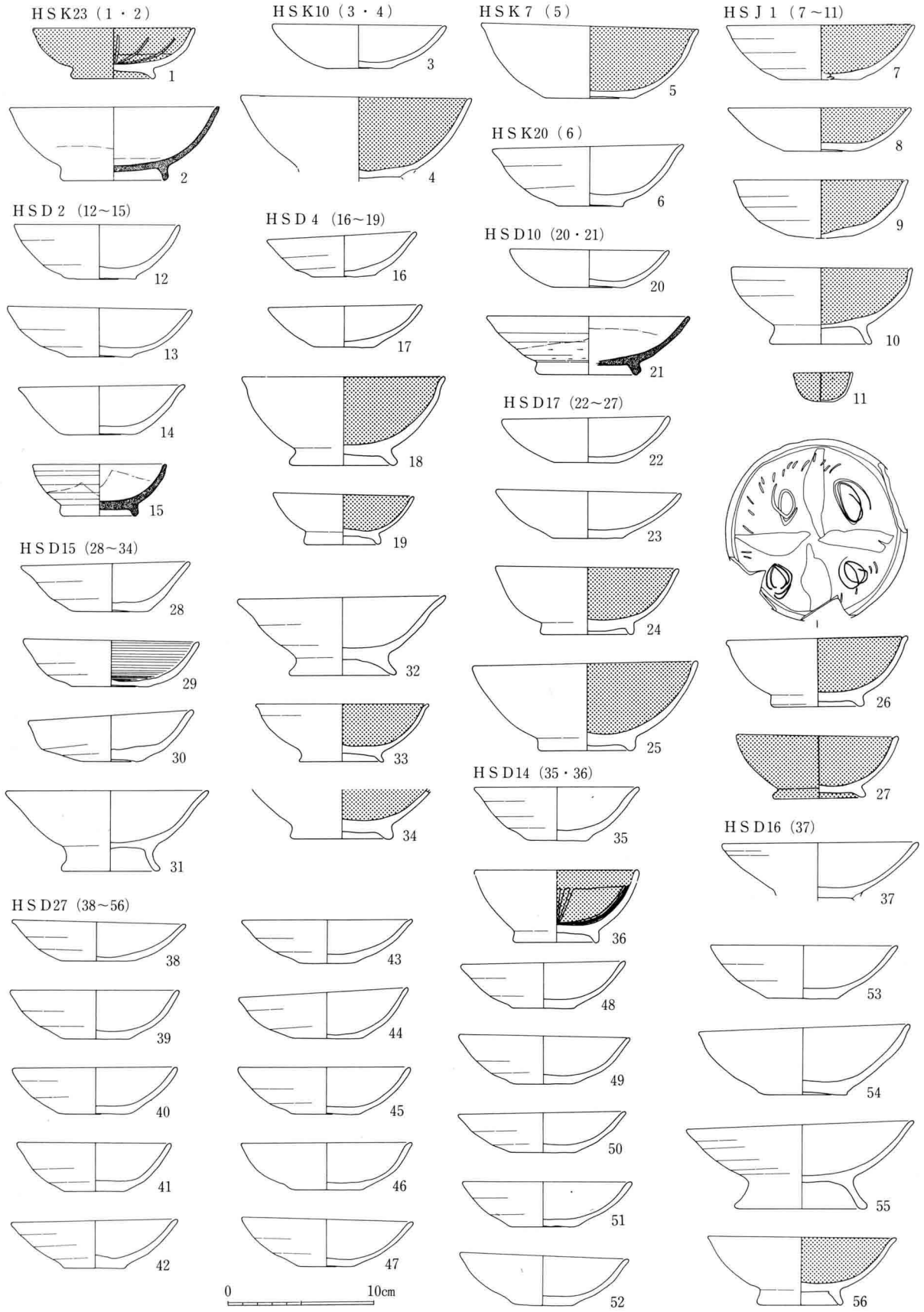
255图 HSK7·10·20·23, HSJ1, HSD2·4·10·14~17·27出土土器实测图(1:4)
