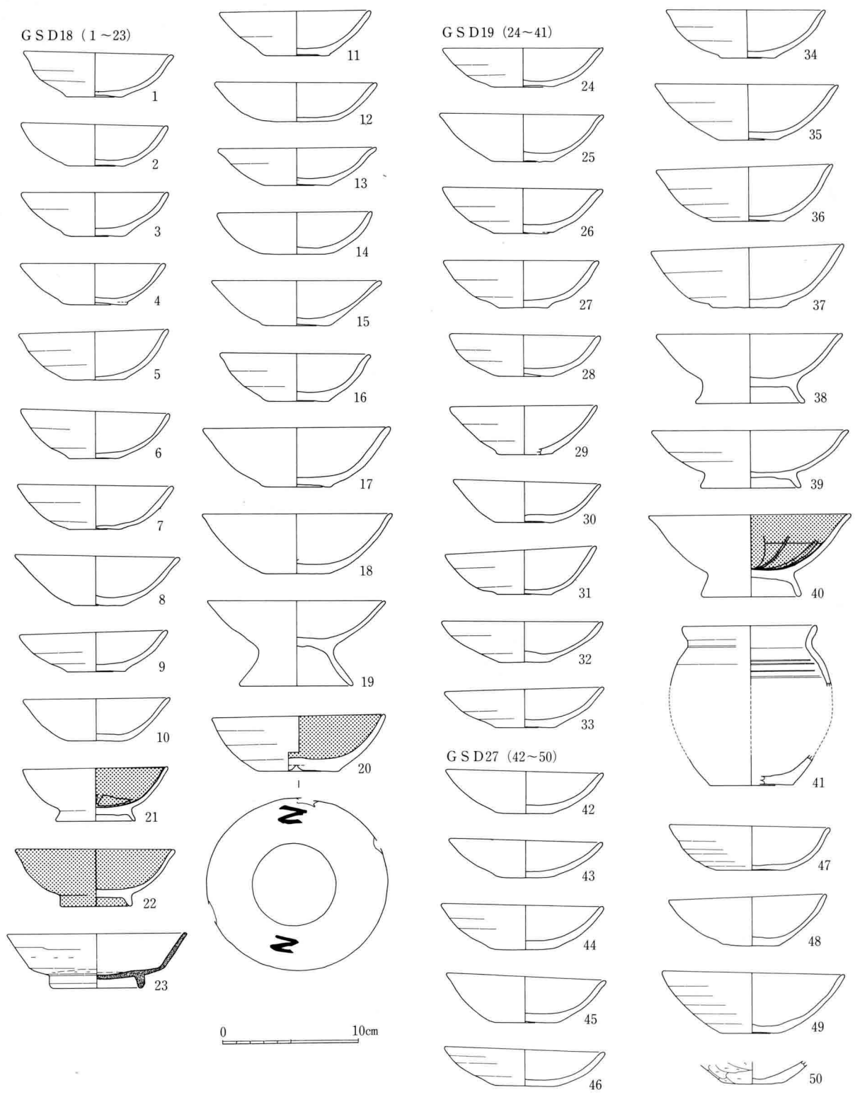
254图 GSD18·19·27出土土器实测图(1:4)
