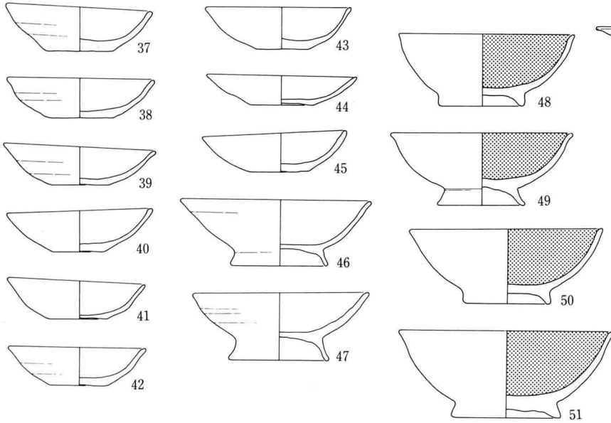
243图 FSD 4·5·23·31·32出土土器実測図(1:4)
