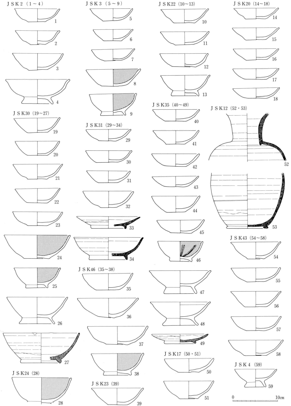
261図 J S K 2 ~ 4 · 12 · 17 · 20 · 22~24 · 30 · 31 · 35 · 43 · 46出土土器実測図 (1 : 4)
