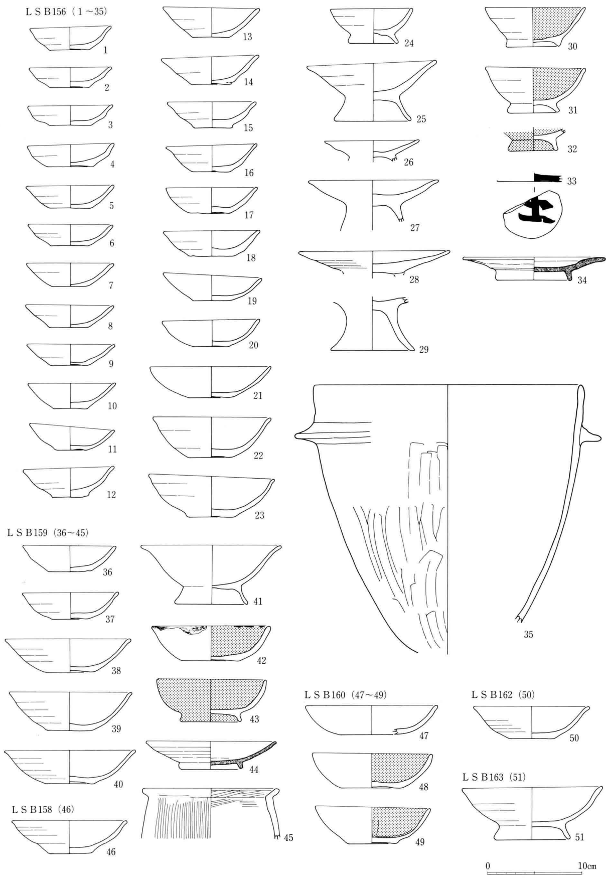
228图 L S B 156 · 158~160 · 162 · 163出土土器实测图 (1 : 4)
