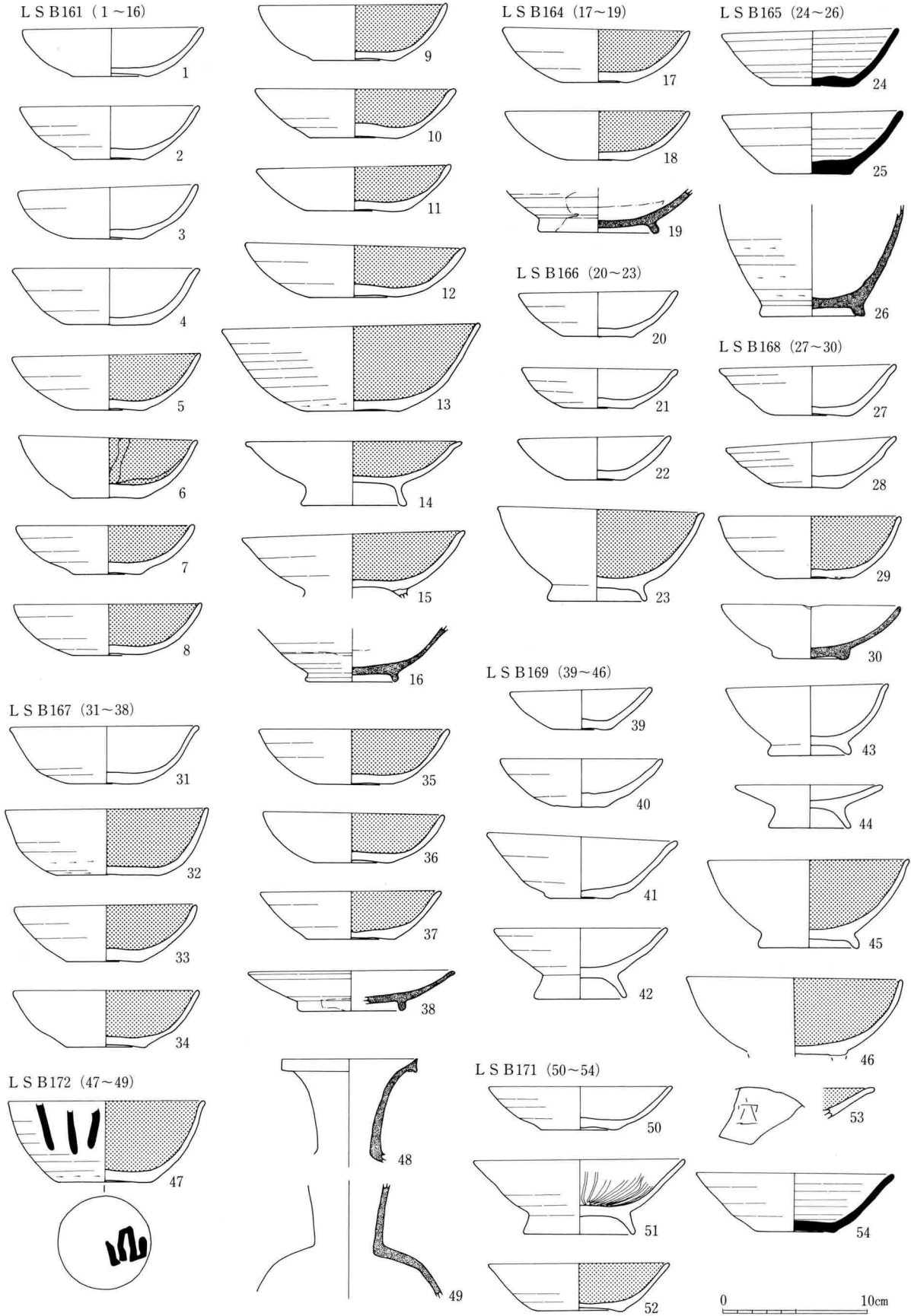
229图 LS B161・164~169・171・172出土土器实测图(1:4)
