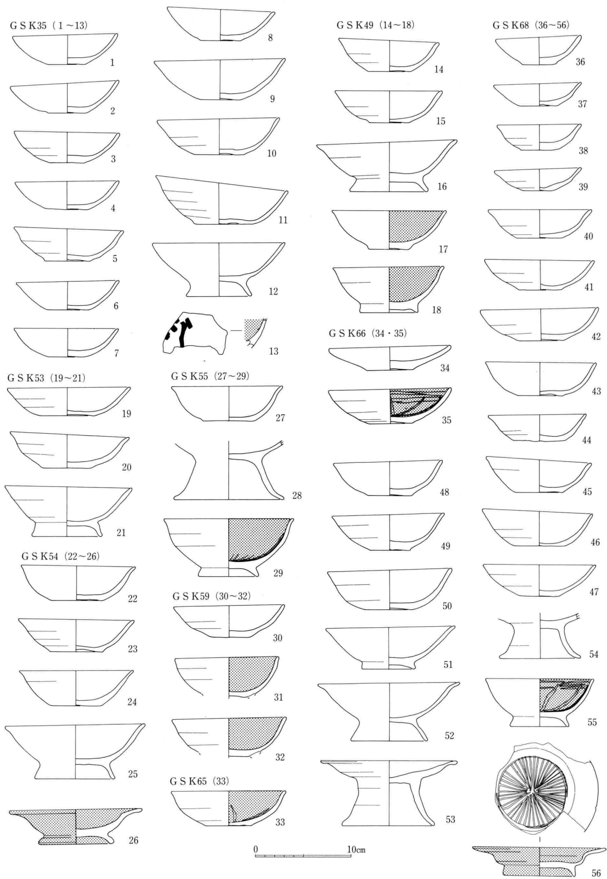
248图 GSK35·49·53~55·59·65·66·68出土土器实测图(1:4)
