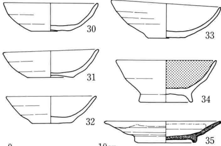
204図 K S B22・25・30~33・35出土土器実測図(1:4)
