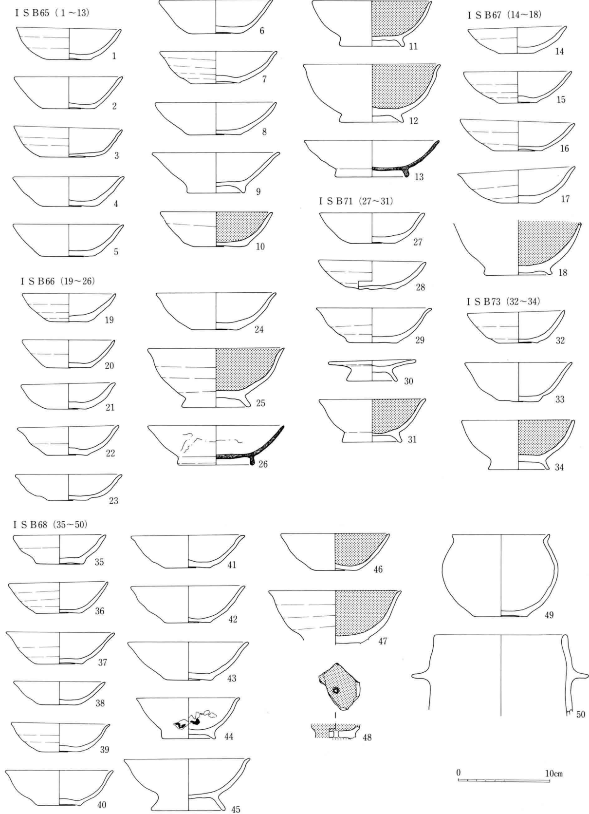
163图 I S B65~68·71·73出土土器实测图(1:4)
