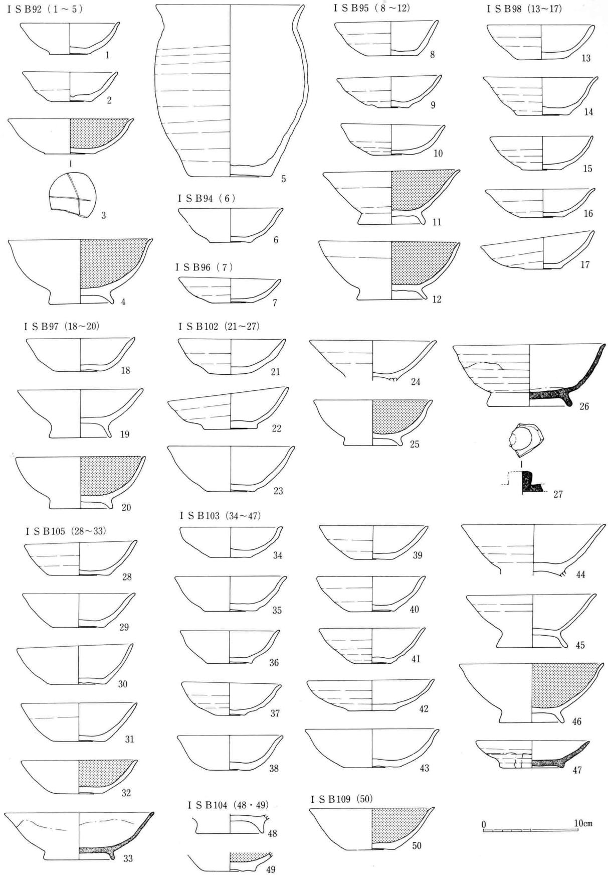
150图 I S B92·94~98·102~105·109出土土器实测图(1:4)
