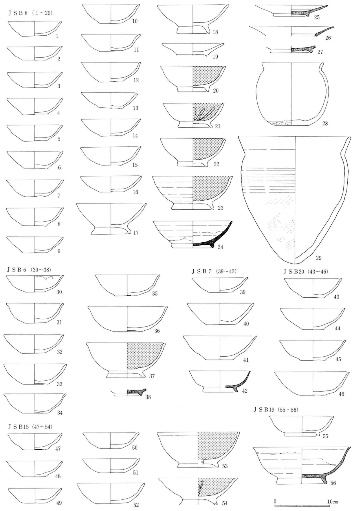
188图 J S B 6 ~ 8 · 15 · 19 · 20出土土器实测图 (1 : 4)
