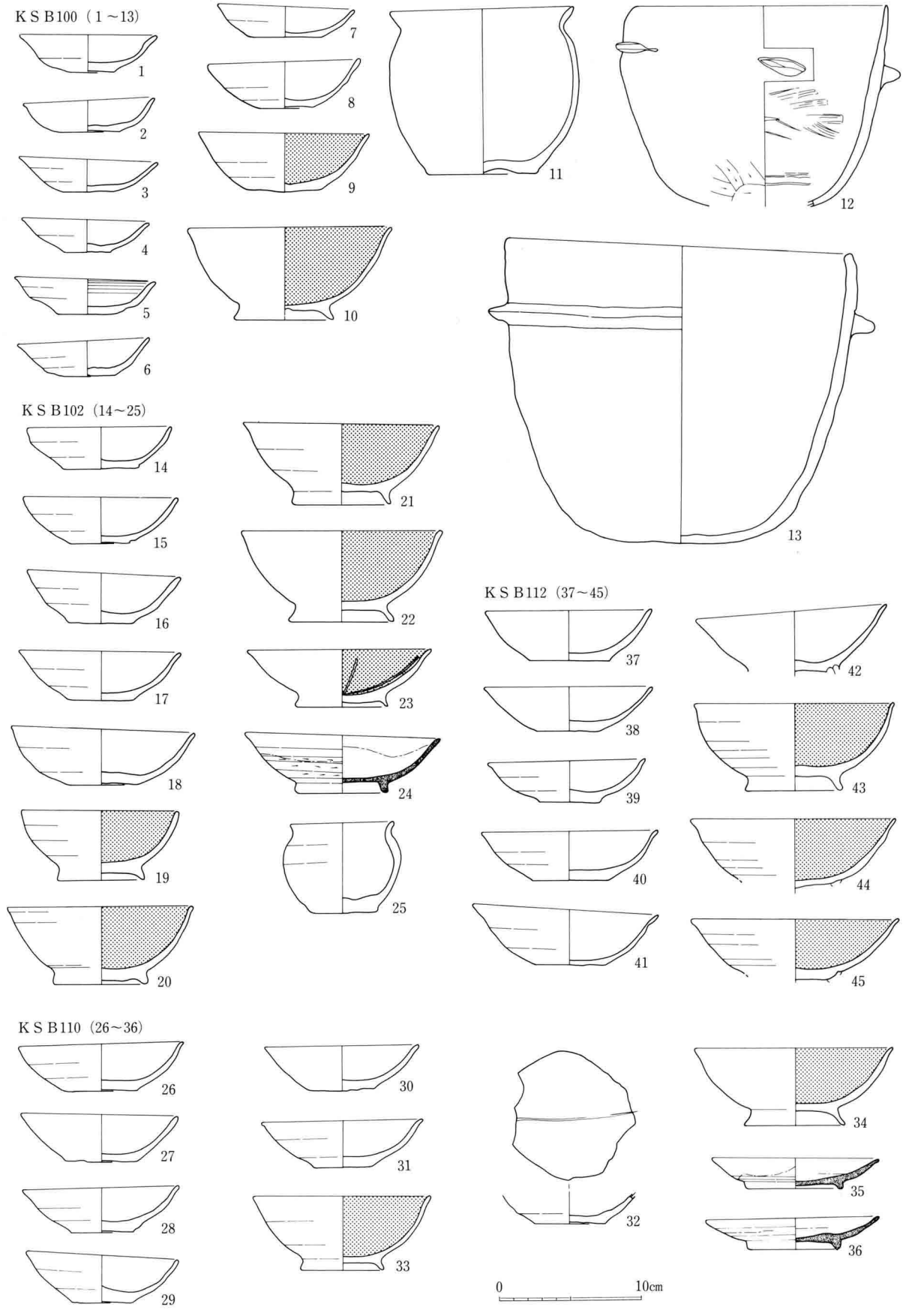
212图 KSB100·102·110·112出土土器实测图(1:4)
