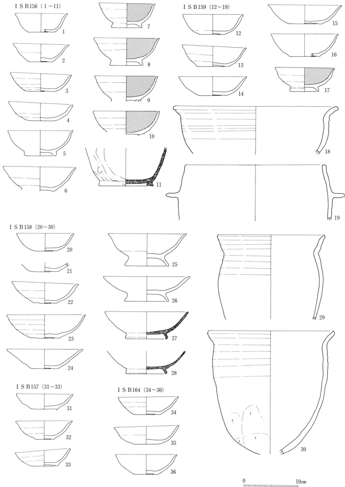
180图 I S B156~159・164出土土器实测图(1:4)
