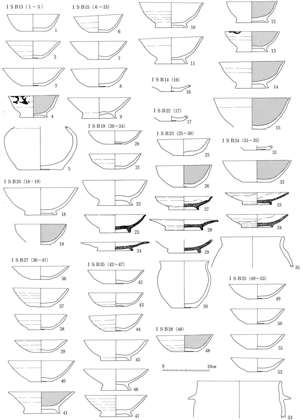
174图 I S B 13~15 · 19 · 20 · 22~25 · 27 · 28 · 35出土土器実测图 (1 : 4)
