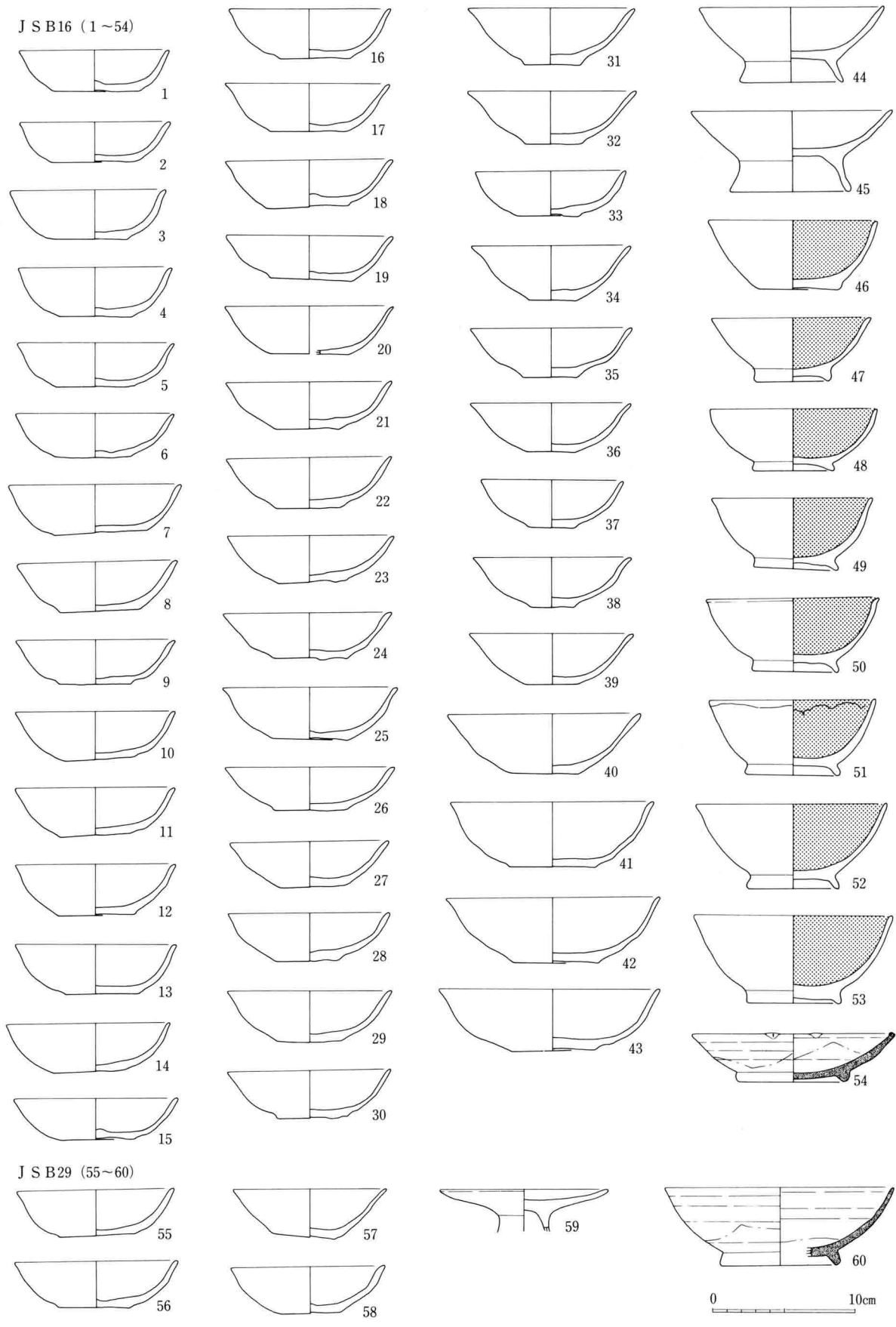
189图 J S B16·29出土土器实测图(1:4)
