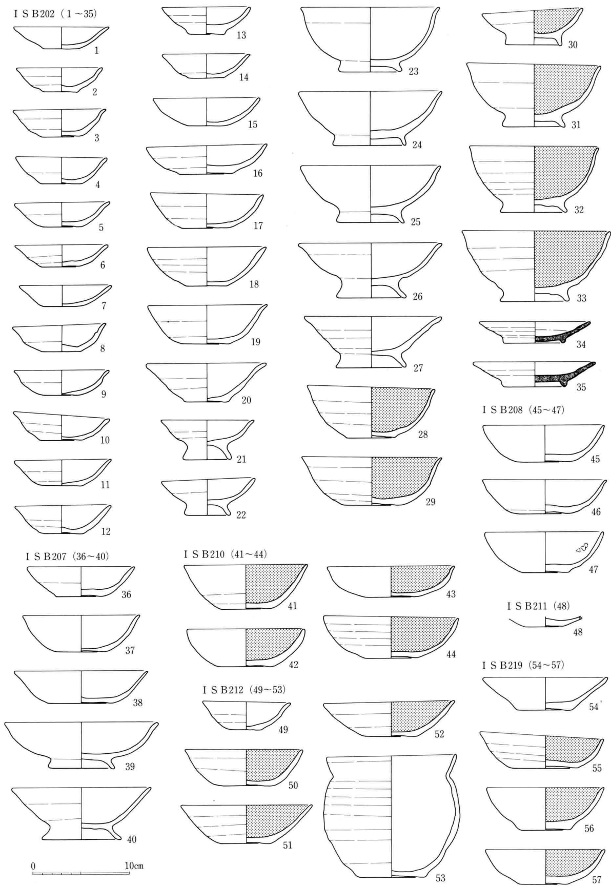
157图 I S B 202 · 207 · 208 · 210~212 · 219出土土器实测图 (1 : 4)
