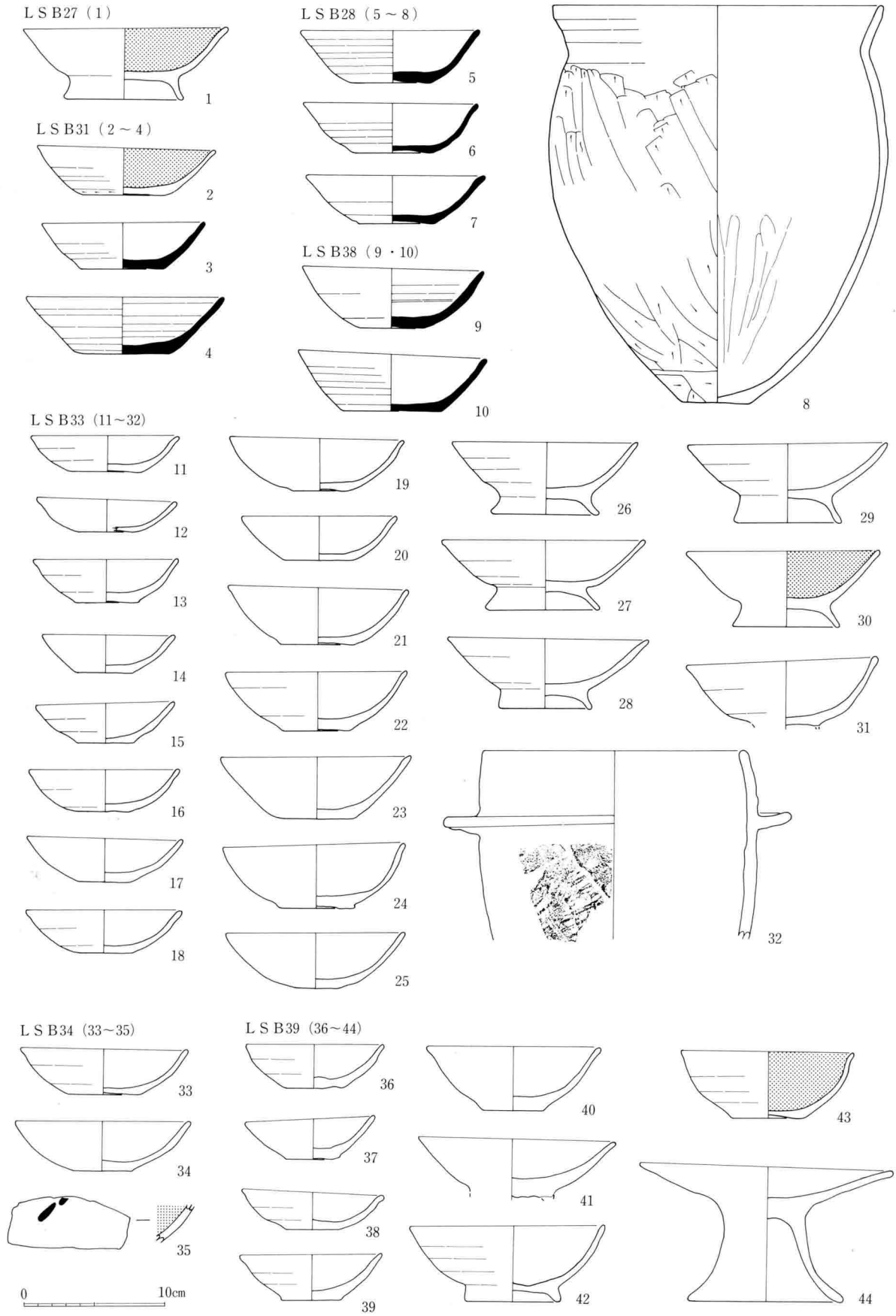
216图 LS B27·28·31·33·34·38·39出土土器实测图(1:4)
