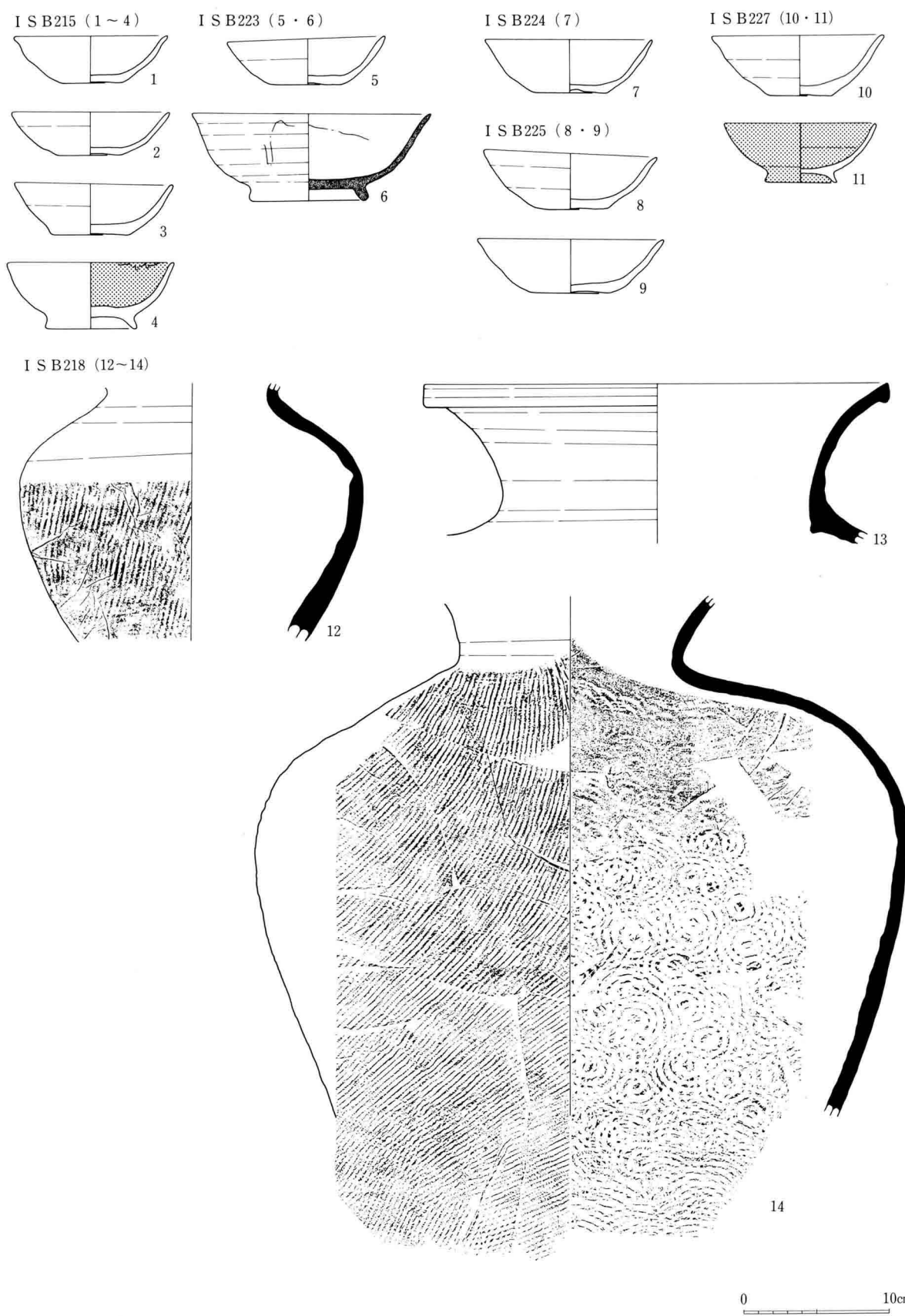
185图 I S B 215 · 218 · 223~225 · 227出土土器实测图 (1 : 4)
