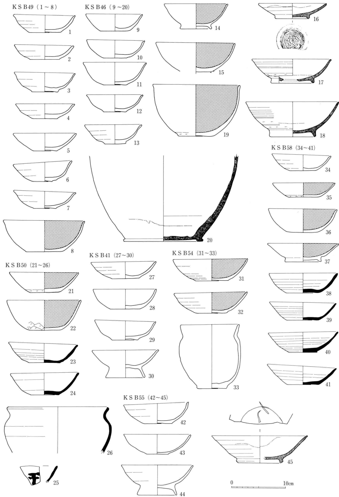
206图 KS B41·46·49·50·54·55·58出土土器实测图(1:4)
