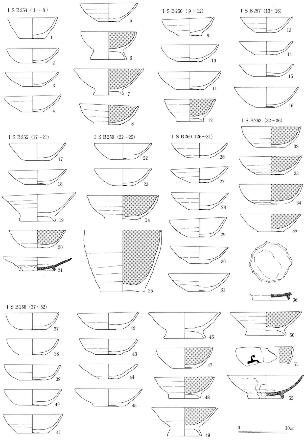
170図 I S B 254~260・263出土土器実測図 (1 : 4)
