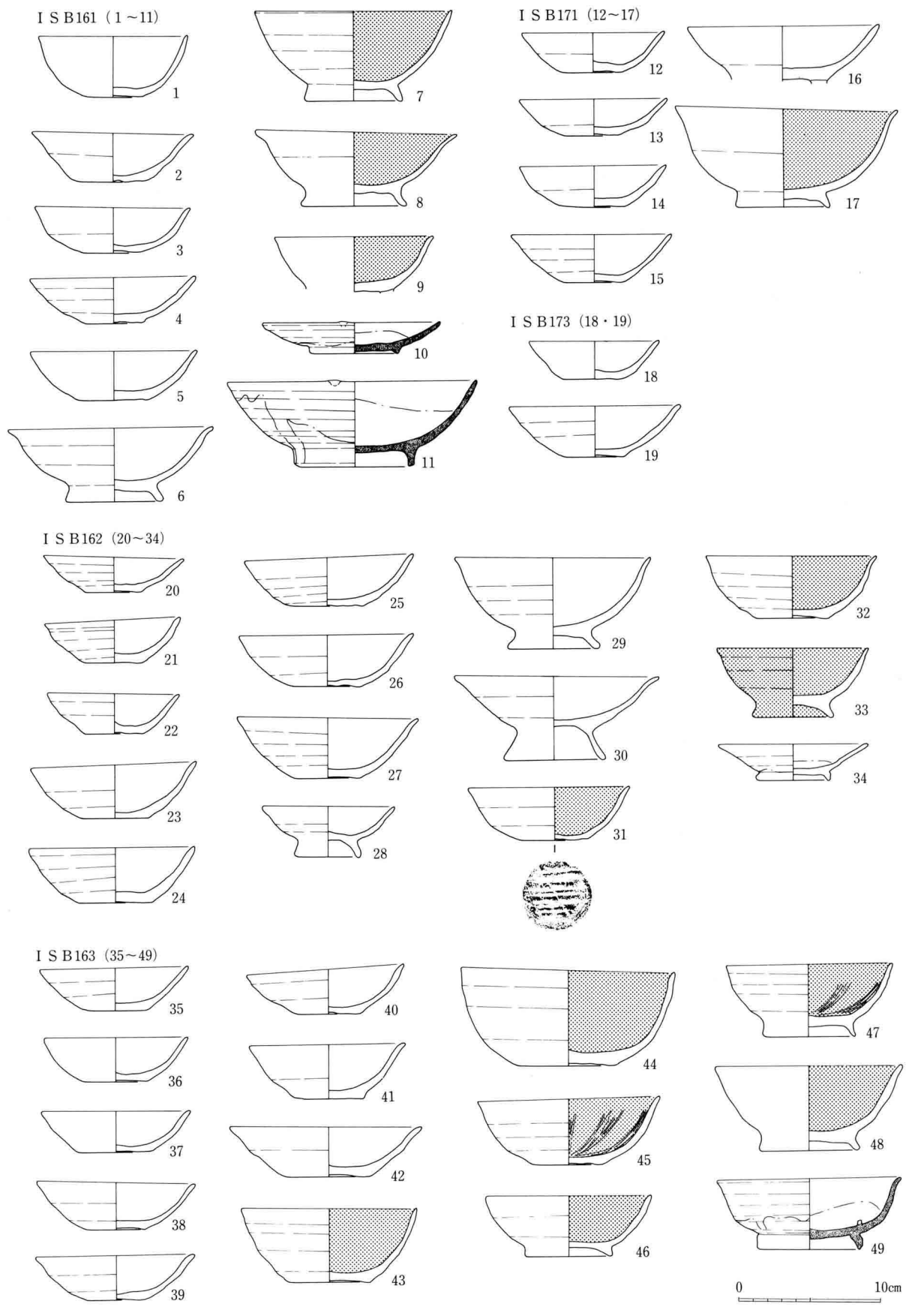
181图 I S B161~163·171·173出土土器实测图(1:4)
