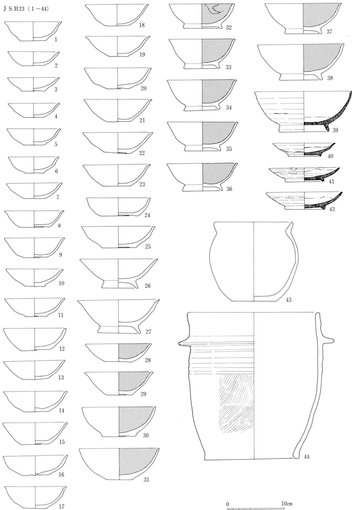
192図 J S B23出土土器実測図 (1 : 4)
