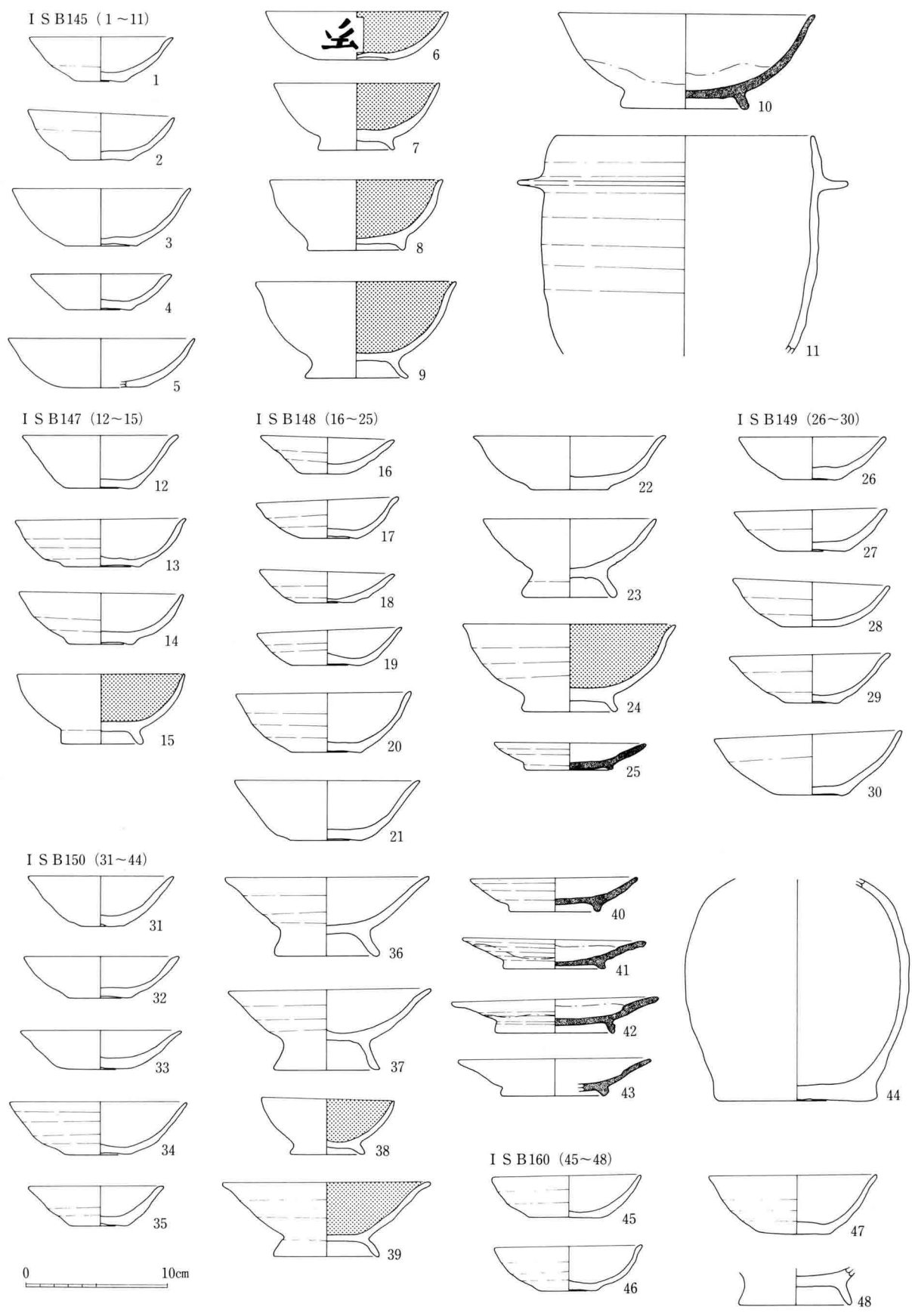
178图 I S B 145 · 147~150 · 160出土土器实测图 (1 : 4)
