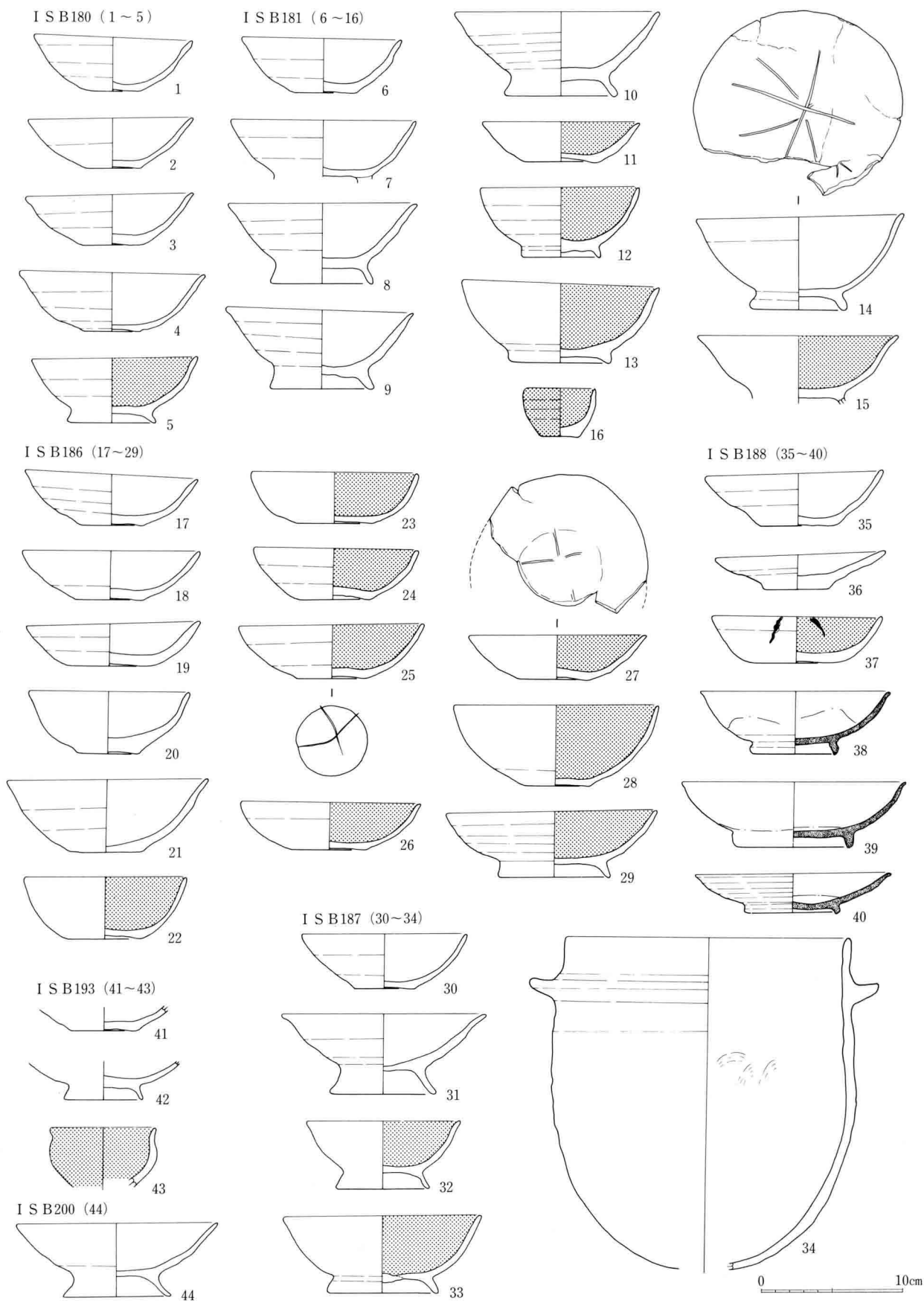
154图 I S B 180 · 181 · 186~188 · 193 · 200出土土器实测图 (1 : 4)
