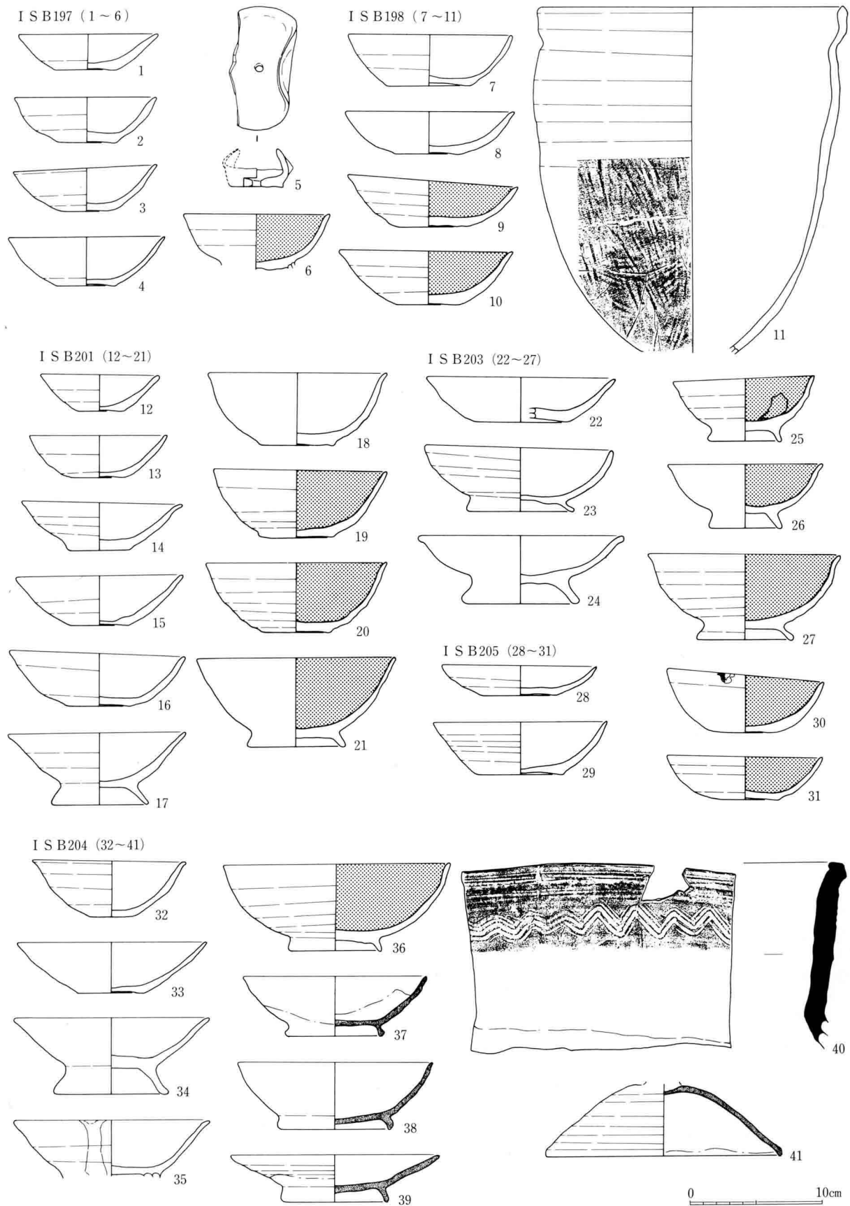
156图 I S B 197 · 198 · 201 · 203 ~ 205出土土器实测图 (1 : 4)
