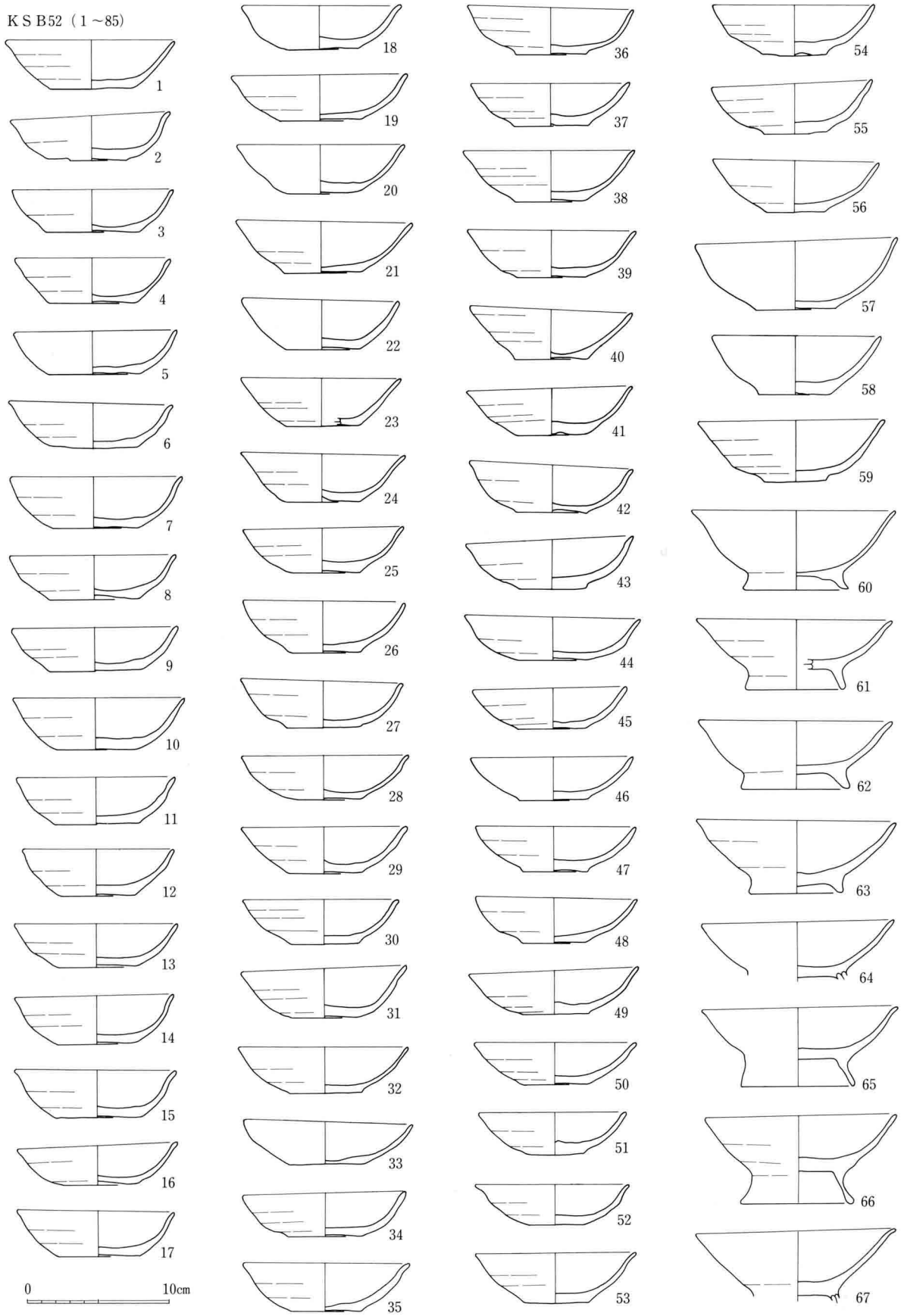
207图 KS B52出土土器实测图 (1 : 4)
