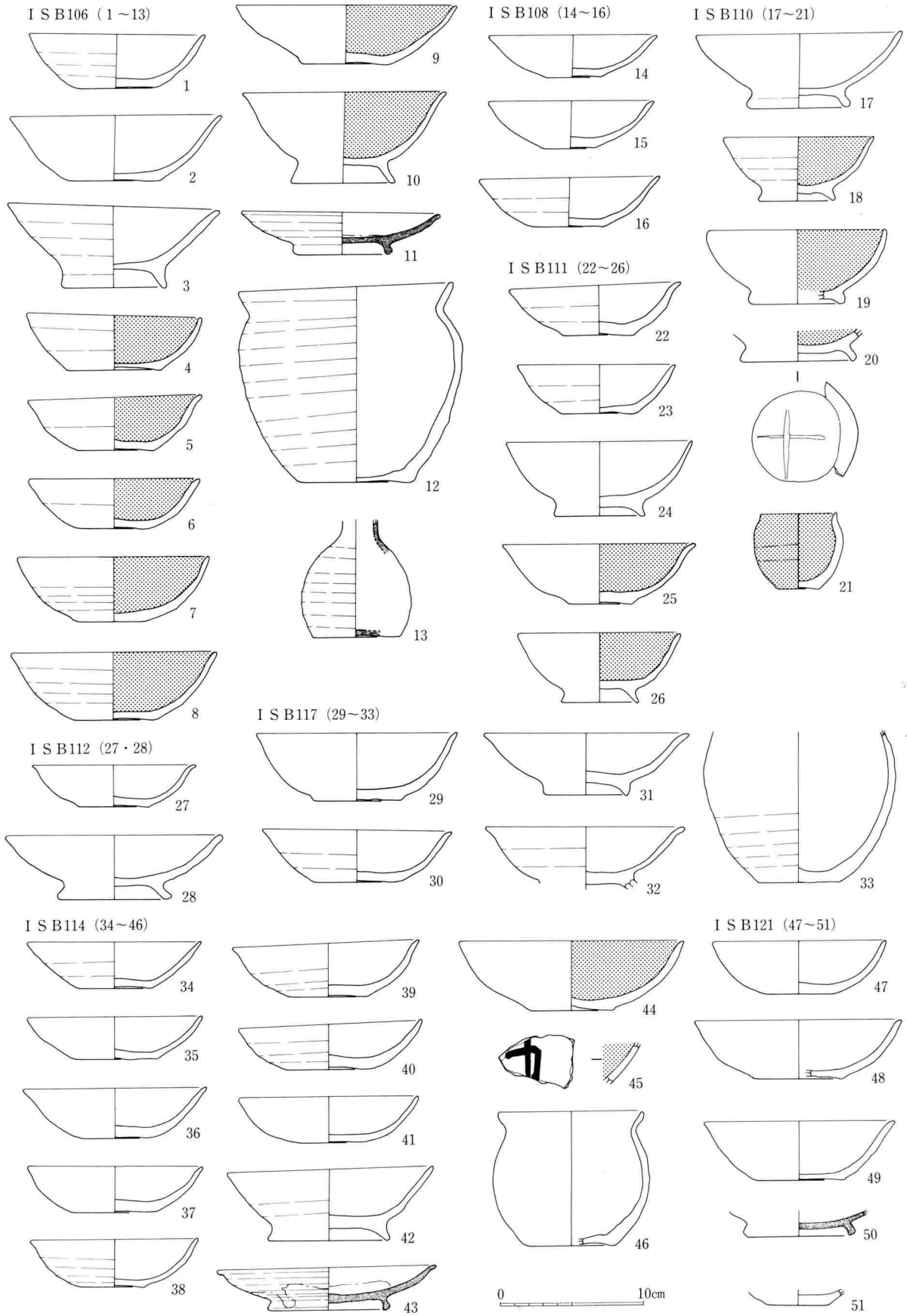
151图 I S B 106 · 108 · 110~112 · 114 · 117 · 121出土土器实测图 (1 : 4)
