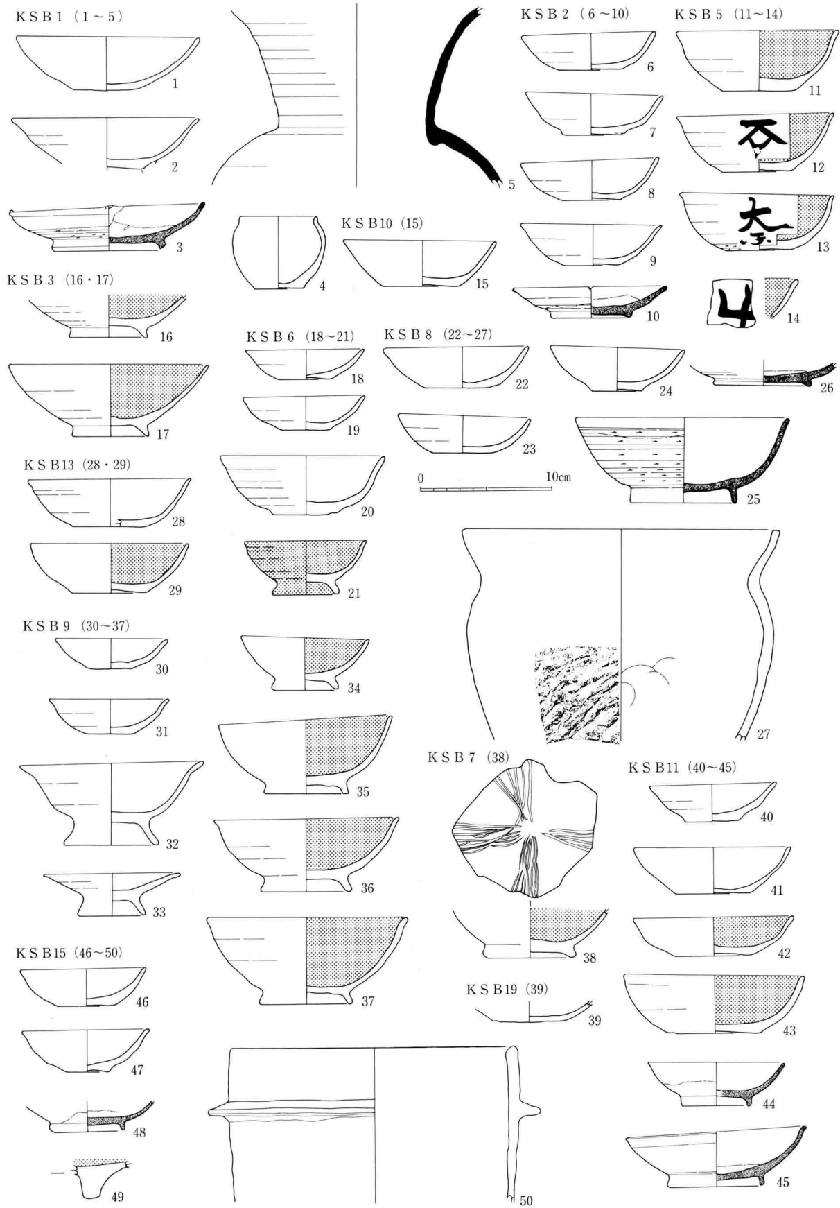
201図 KSB 1~3・5~11・13・15・19出土土器実測図(1:4)
