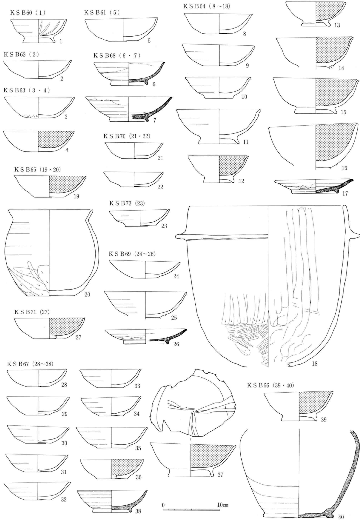
209図 K S B60~71・73出土土器実測図 (1 : 4)
