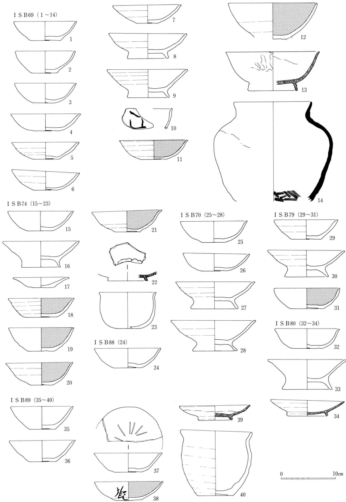
164图 I S B69 · 70 · 74 · 79 · 80 · 88 · 89出土土器实测图 (1 : 4)
