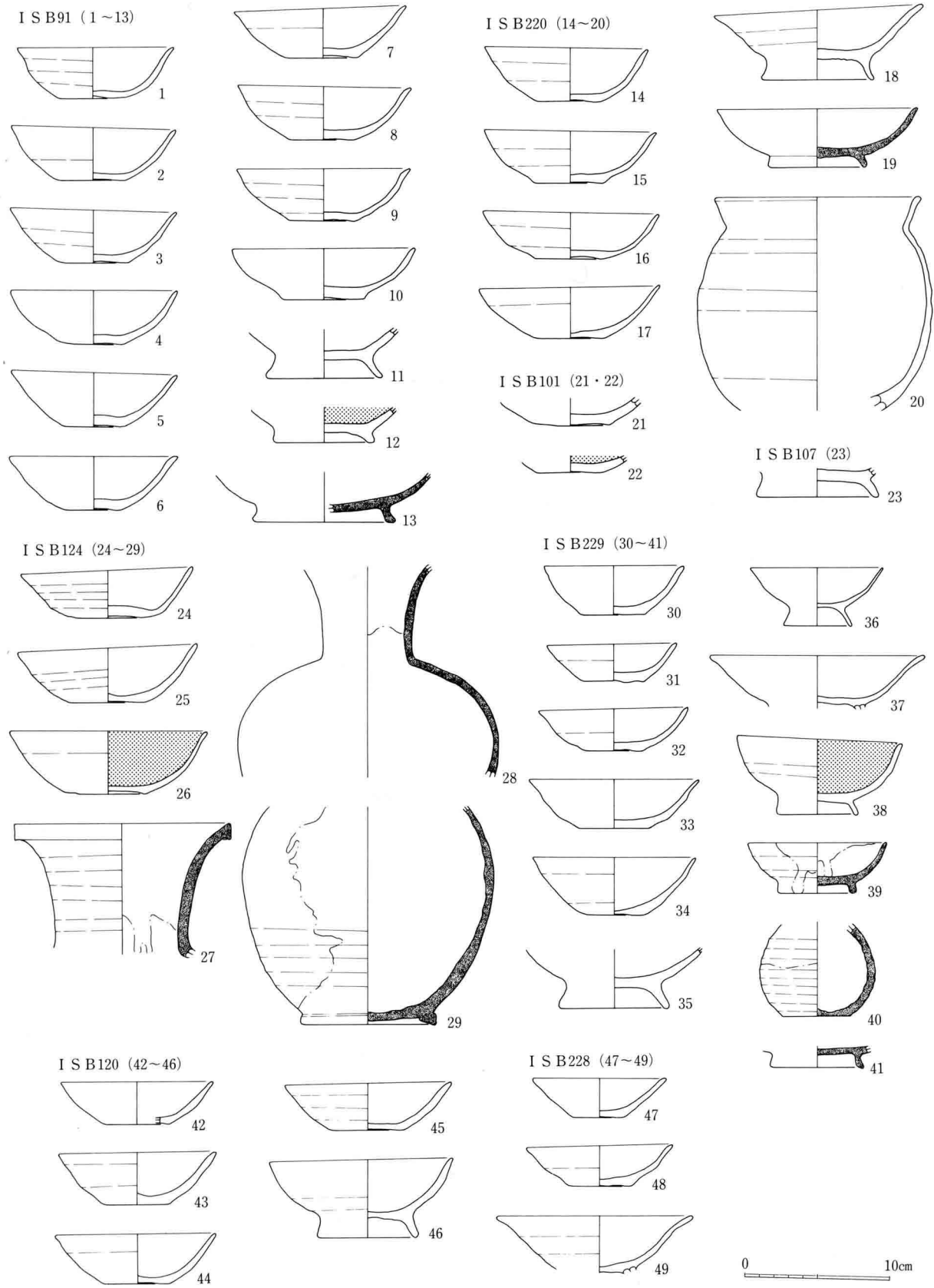
166图 I S B91 · 101 · 107 · 120 · 124 · 220 · 228 · 229出土土器实测图 (1 : 4)
