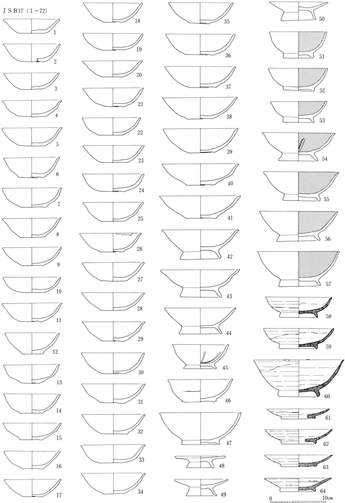
190图 J S B17出土土器实测图 (1 : 4)
