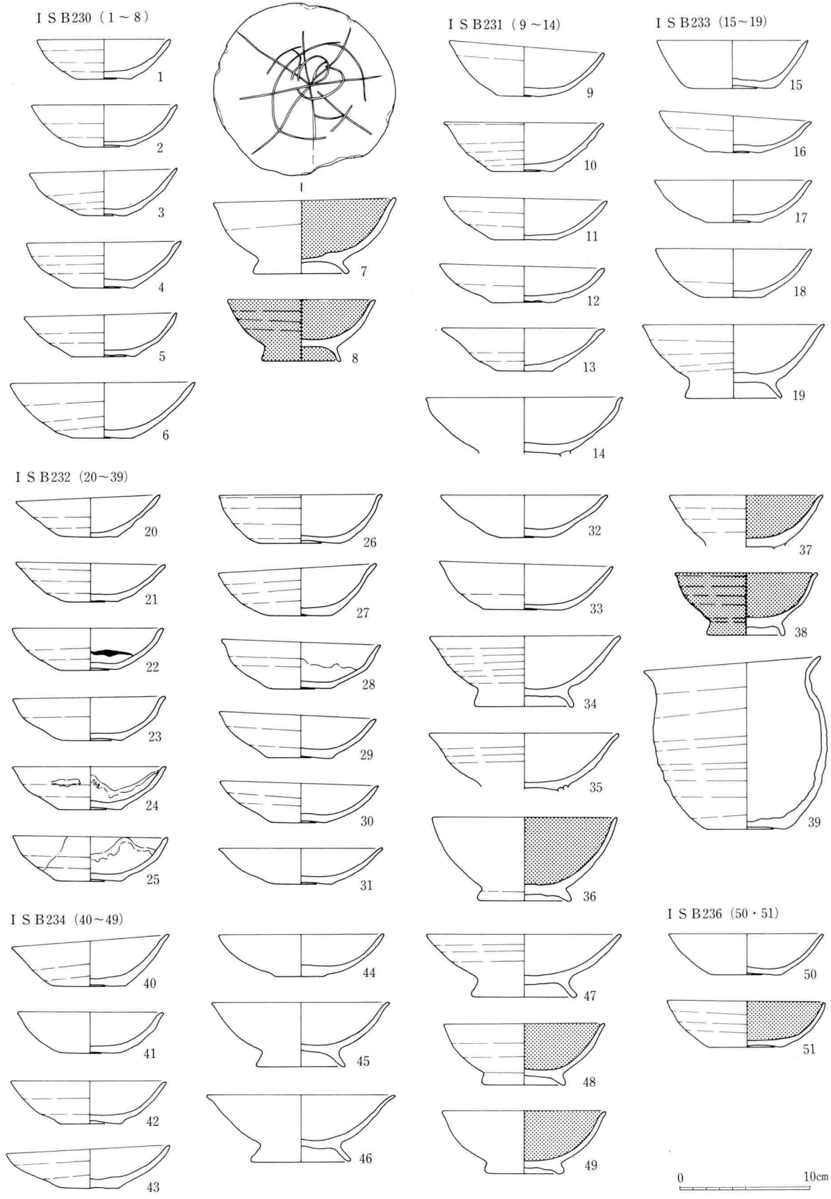
167图 I S B 230~234·236出土土器实测图(1:4)
