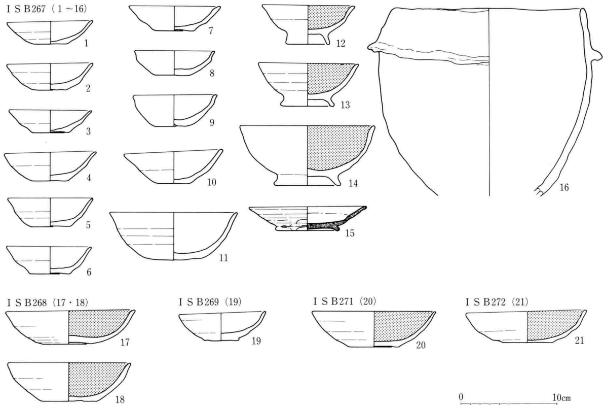
158図 I S B 267~269・271・272出土土器実測図(1:4)
