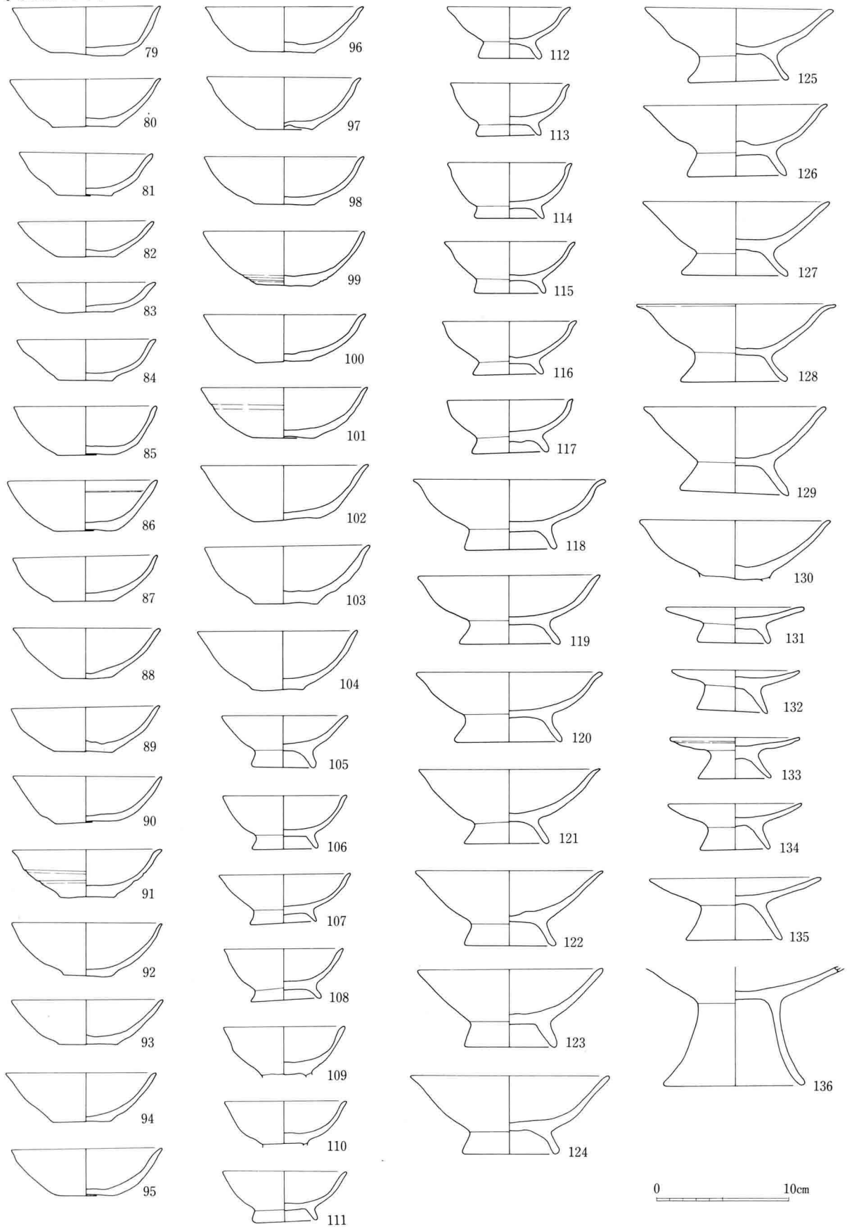
196図 J S B26出土土器実測図 (1 : 4)
