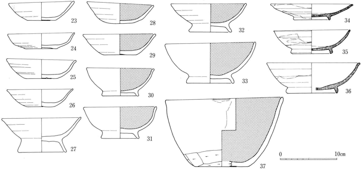
214図 LSB9~16出土土器実測図(1:4)
