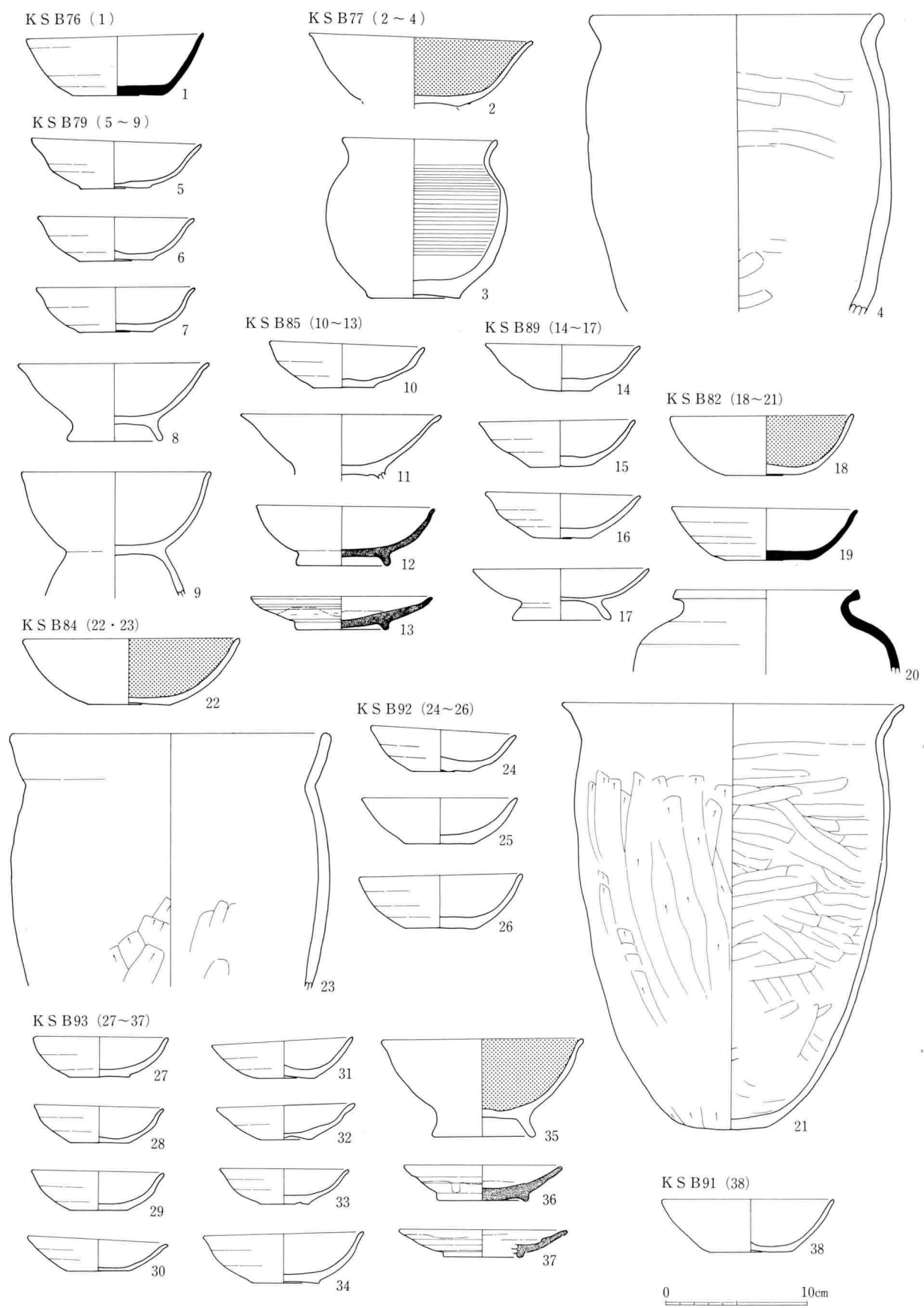
210图 K S B 76 · 77 · 79 · 82 · 84 · 85 · 89 · 91~93出土土器实测图 (1 : 4)
