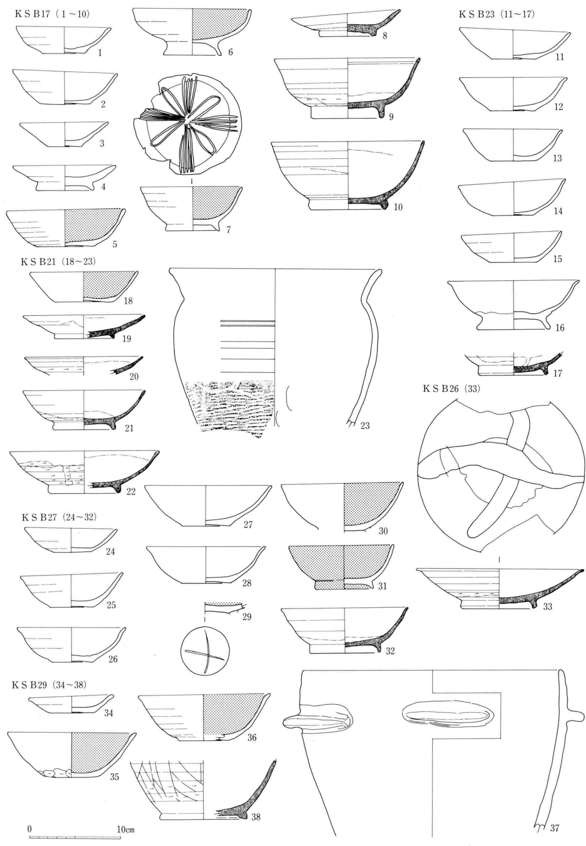
203図 KSB17・21・23・26・27・29出土土器実測図(1:4)
