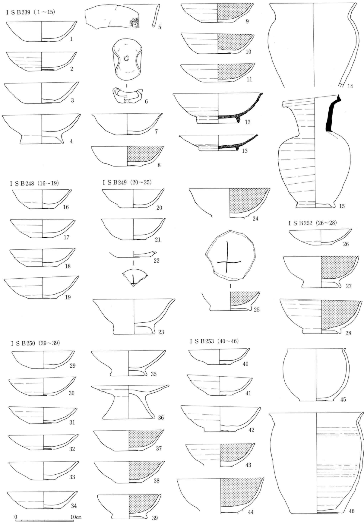
169图 I S B239 · 248~250 · 252 · 253出土土器实测图 (1 : 4)
