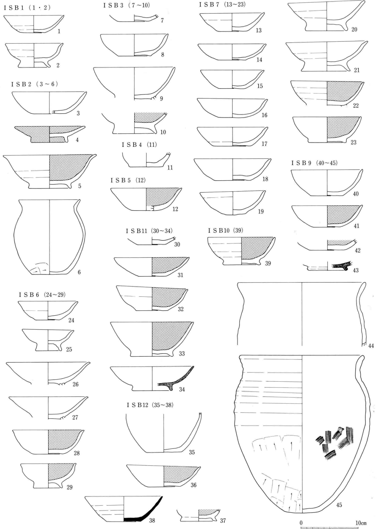
173图 ISB 1~7·9~12出土土器实测图(1:4)
