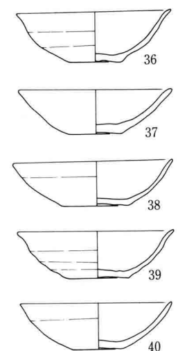
182图 I S B166 · 168~170 · 172出土土器实测图 (1 : 4)
