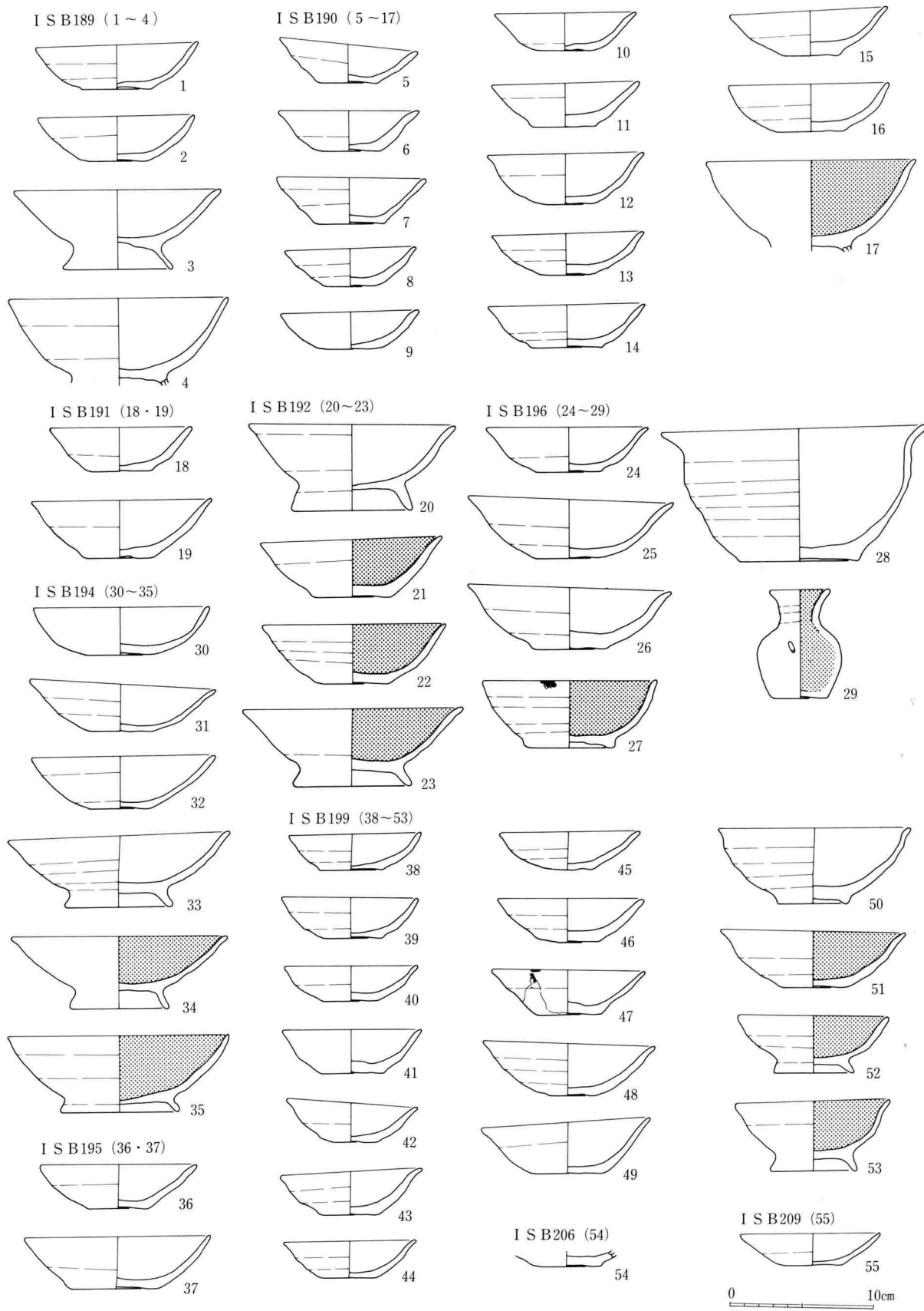
155図 IS B189~192・194~196・199・206・209出土土器実測図(1:4)
