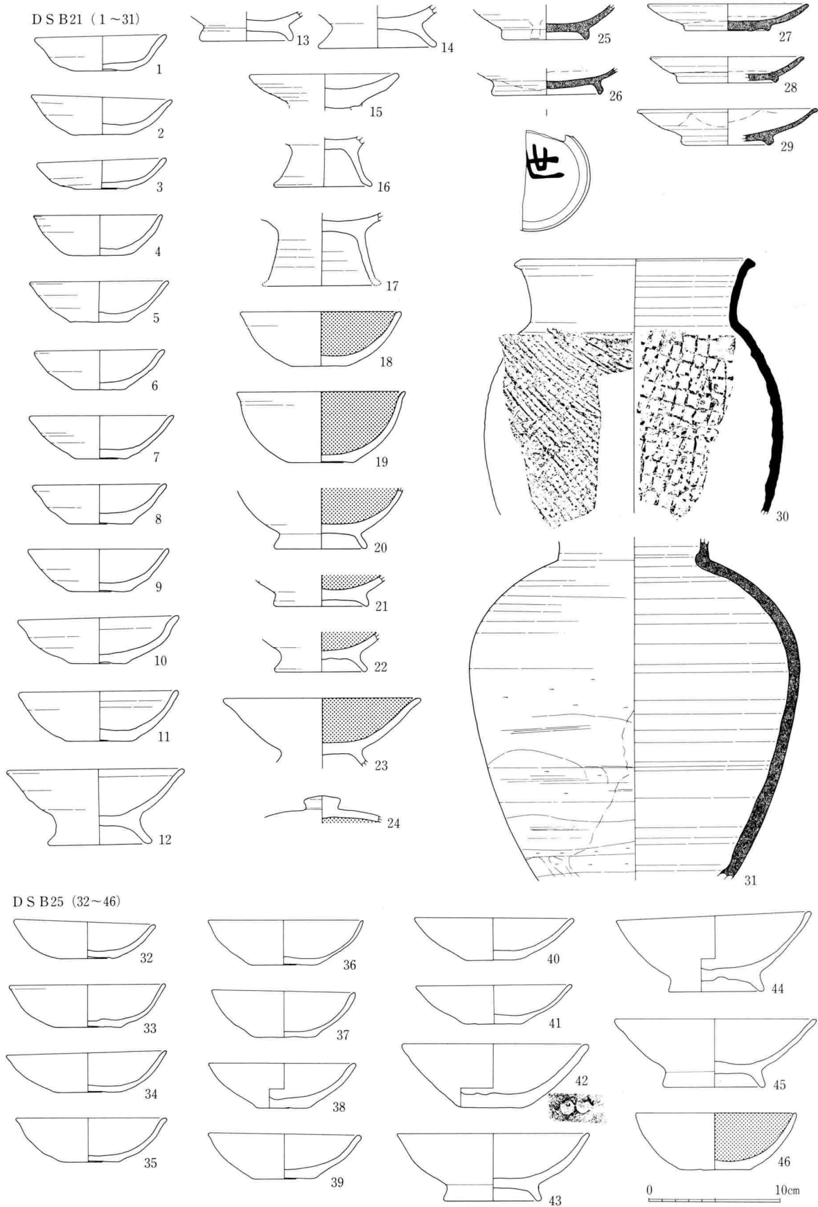
44图 DS B21·25出土土器实测图(1:4)
