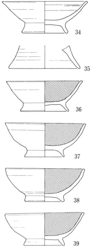
6 图 AS B15 · 16 · 23出土土器实测图 (1 : 4)
