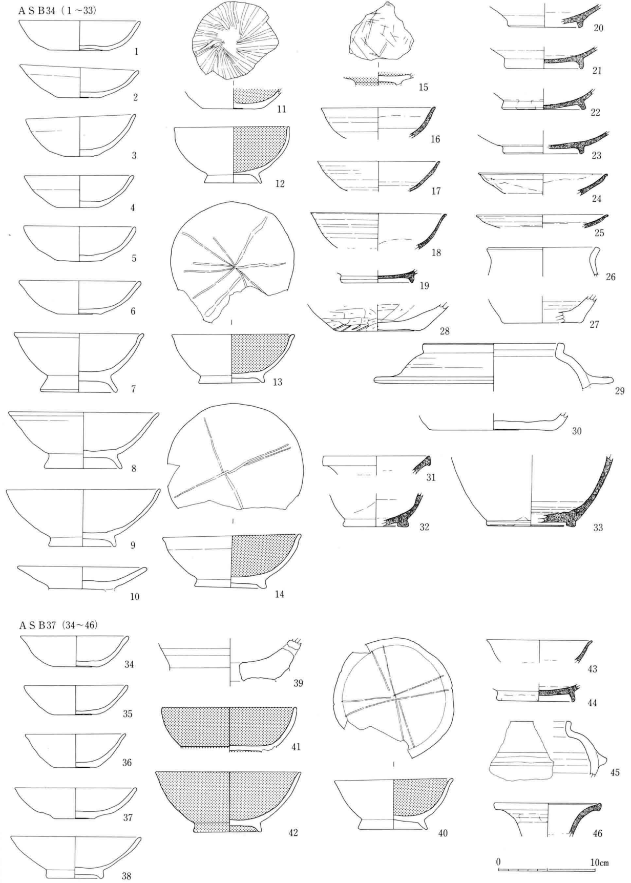
11图 ASB34·37出土土器实测图(1:4)
