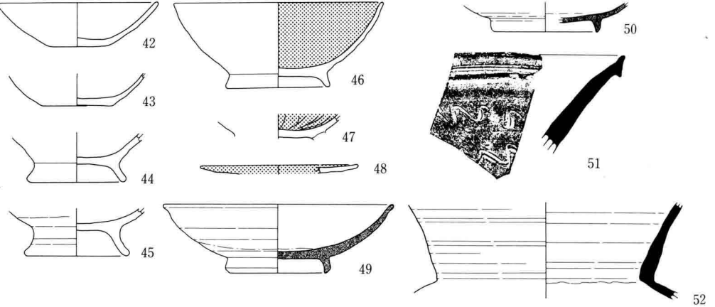
32图 C S B16·26·30出土土器实测图(1:4)
