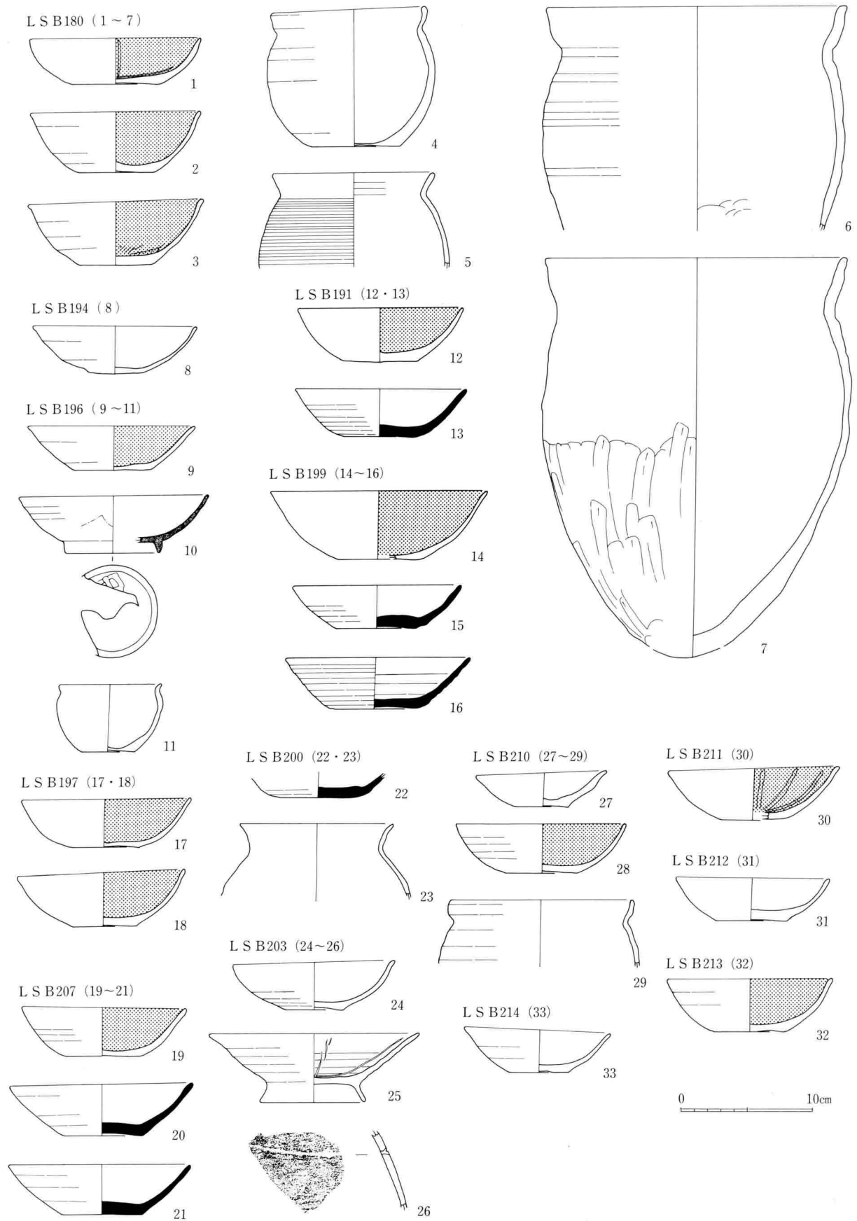
66图 L S B180·191·194·196·197·199·200·203·207·210~214出土土器实测图(1:4)
