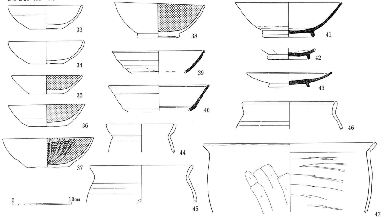
33图 C S B17·28出土土器实测图 (1:4)
