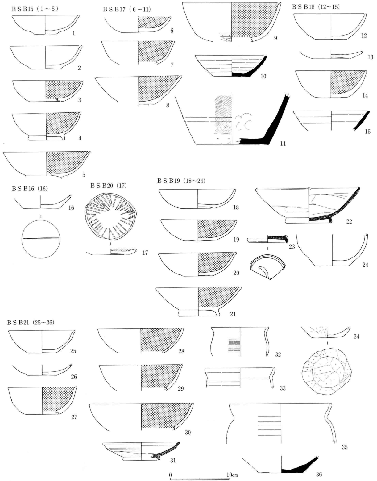
25図 BSB15~21出土土器実測図(1:4)
