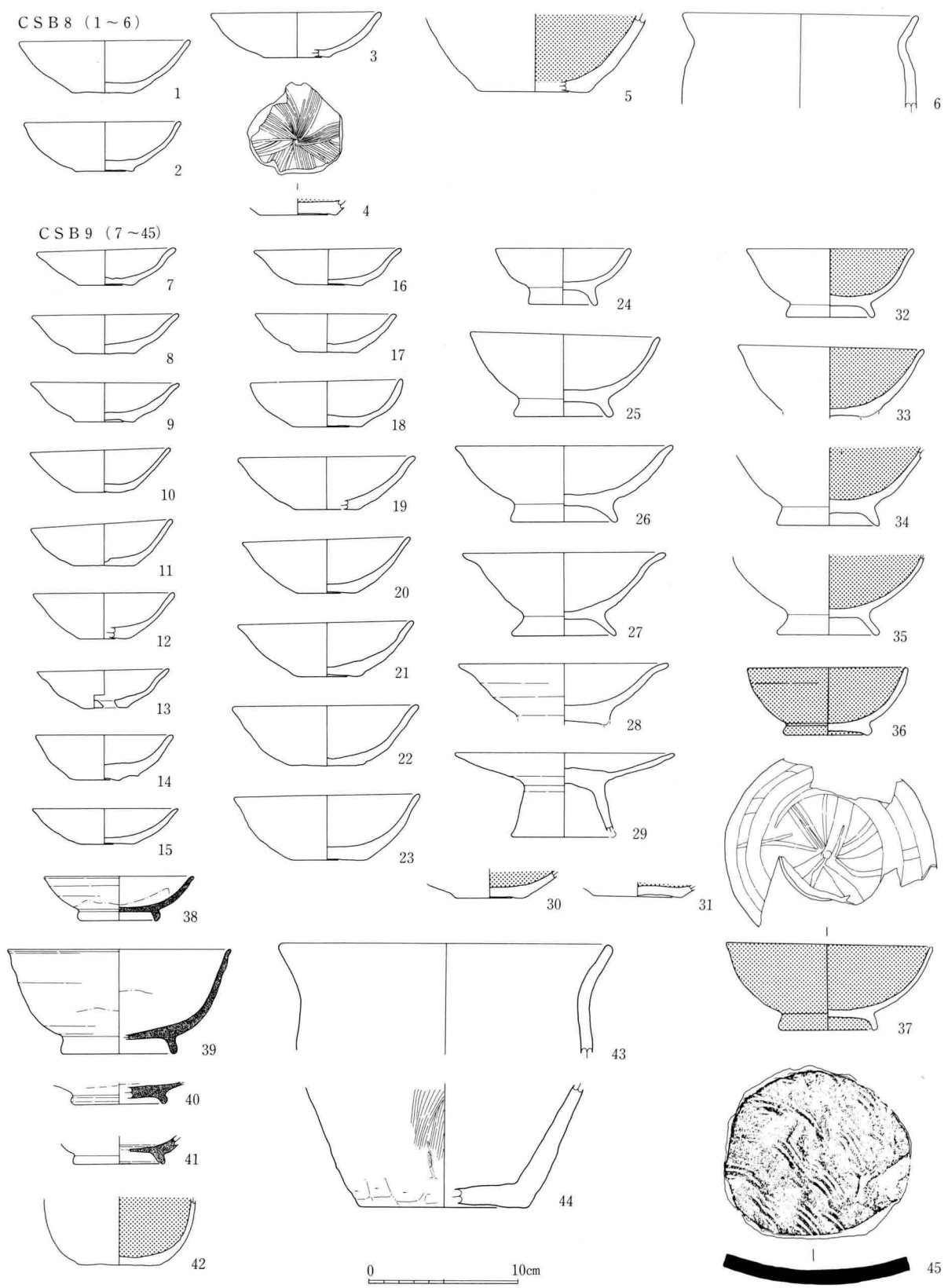
28图 CSB 8・9 出土土器实测图 (1:4)
