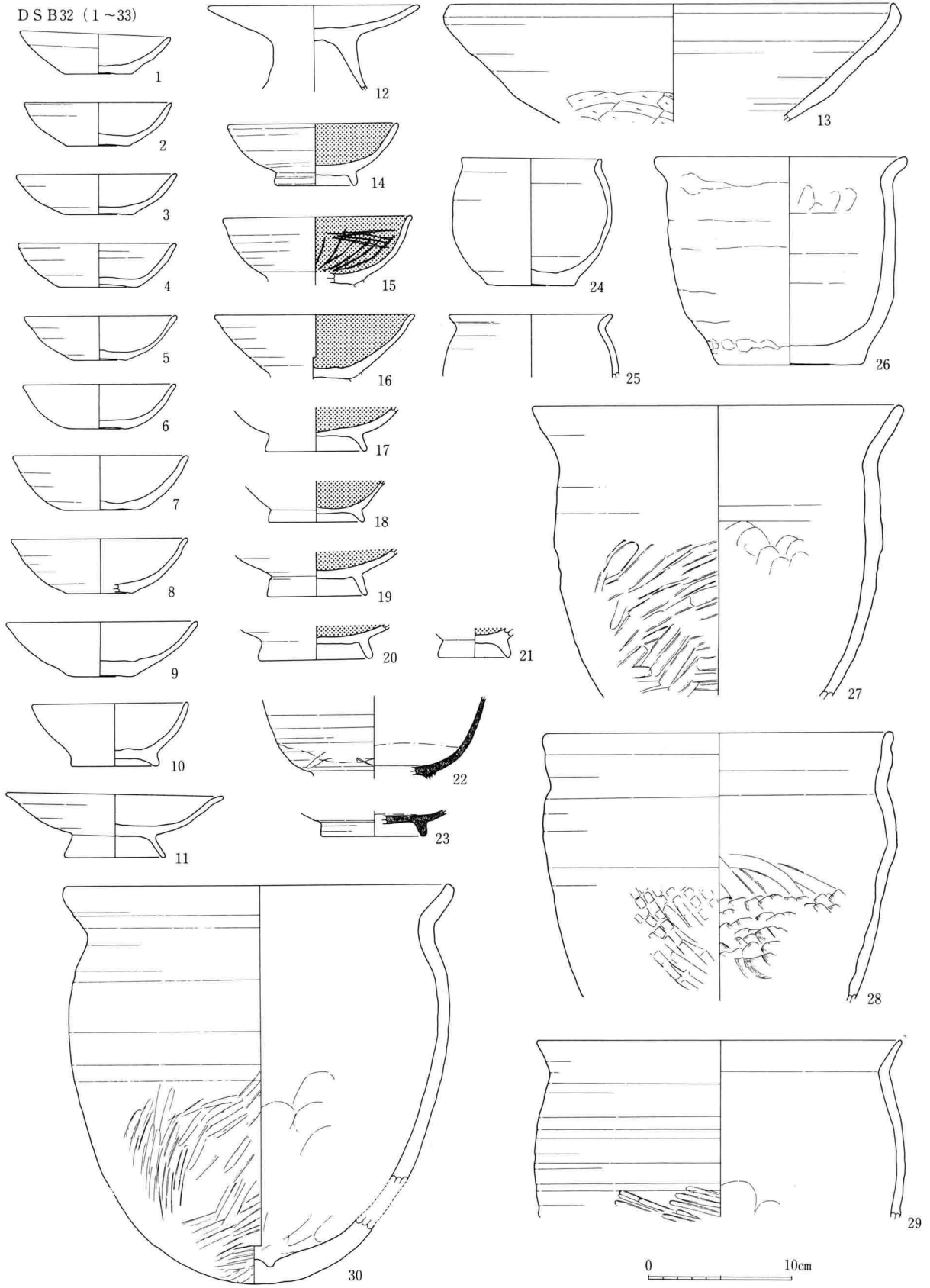
48图 DSB32出土土器实测图(1:4)
