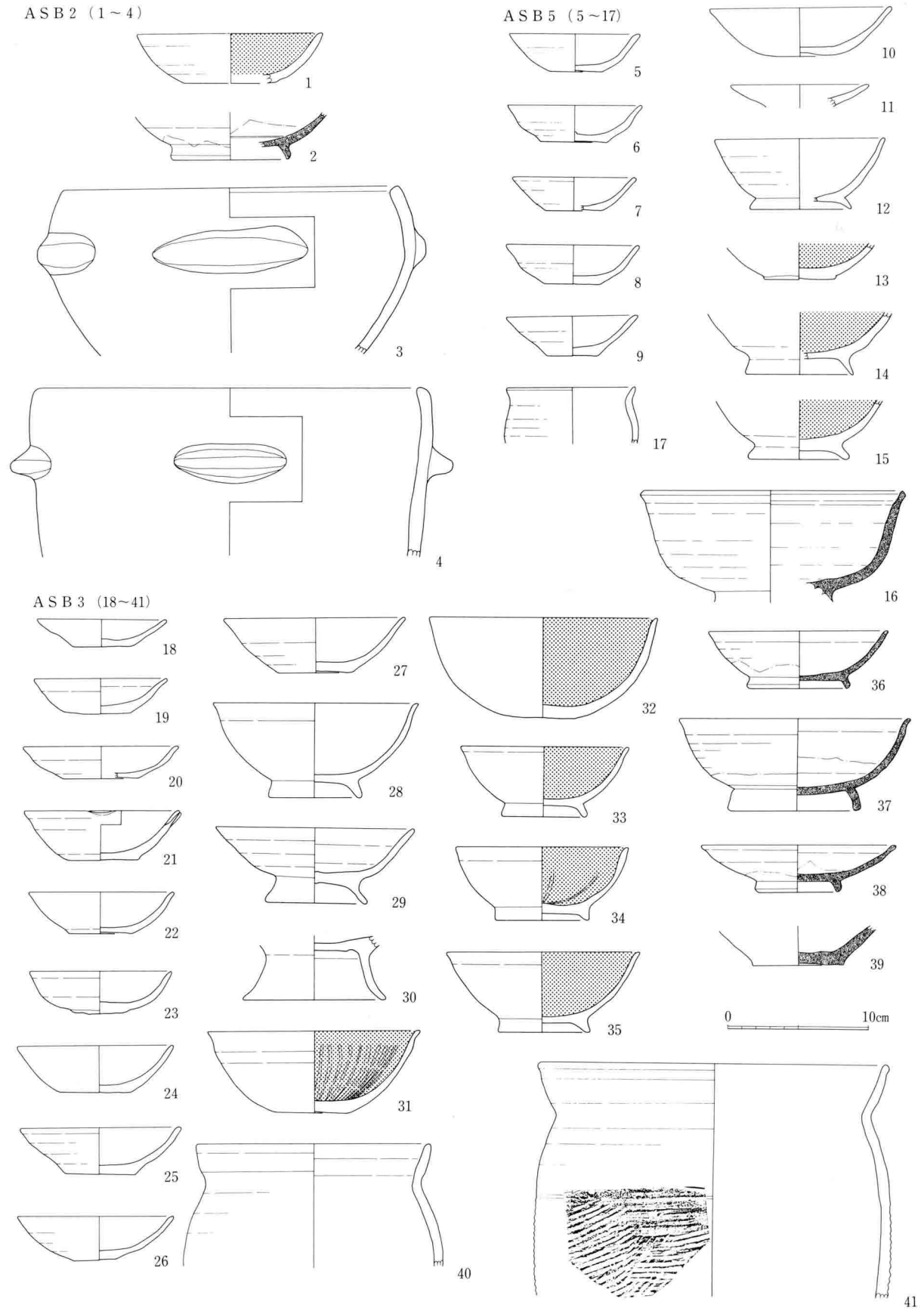
2图 ASB 2·3·5 出土土器实测图 (1:4)
