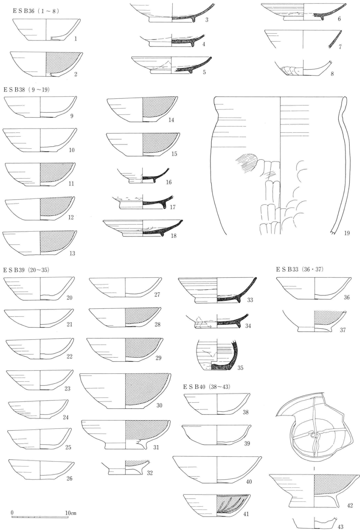
76图 ESB33·36·38~40出土土器实测图(1:4)
