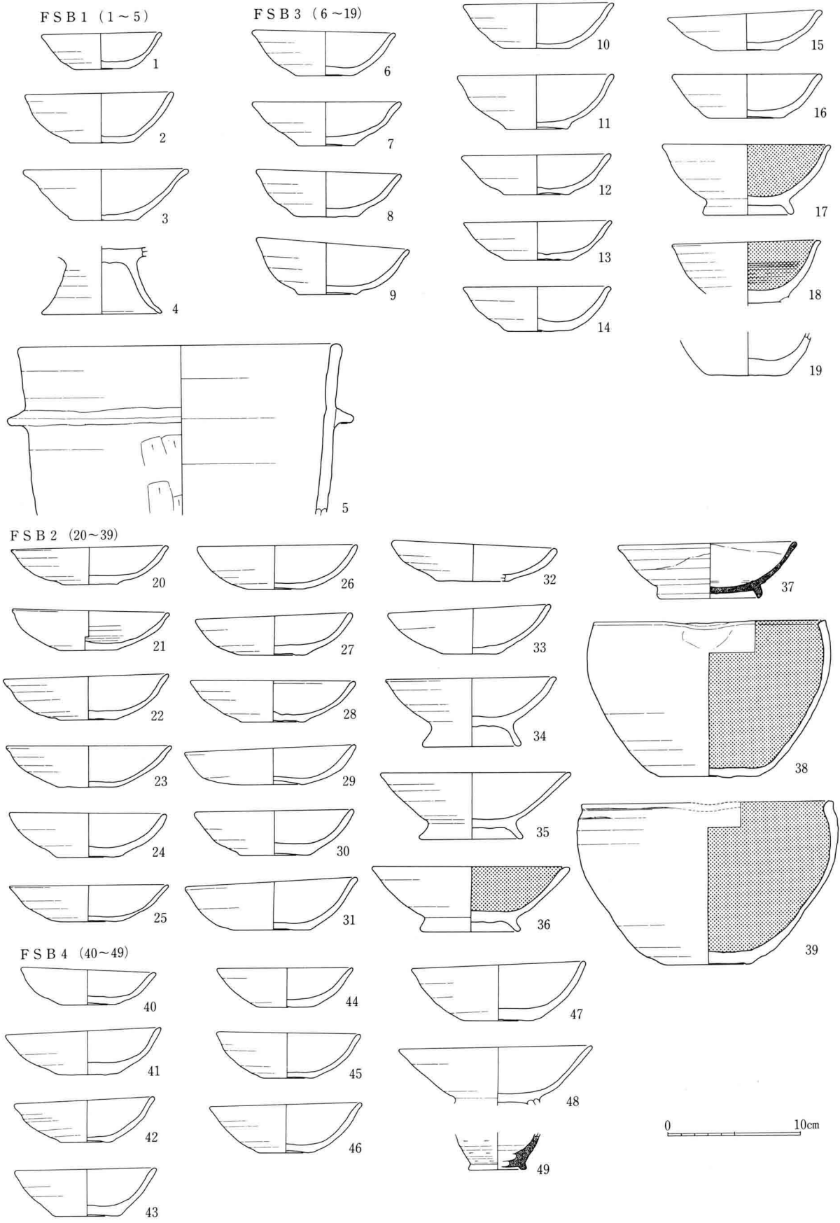
77图 FSB 1~4 出土土器实测图 (1:4)
