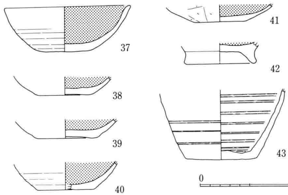
16图 A S B50 · 52 · 56 · 58出土土器实测图 (1 : 4)
