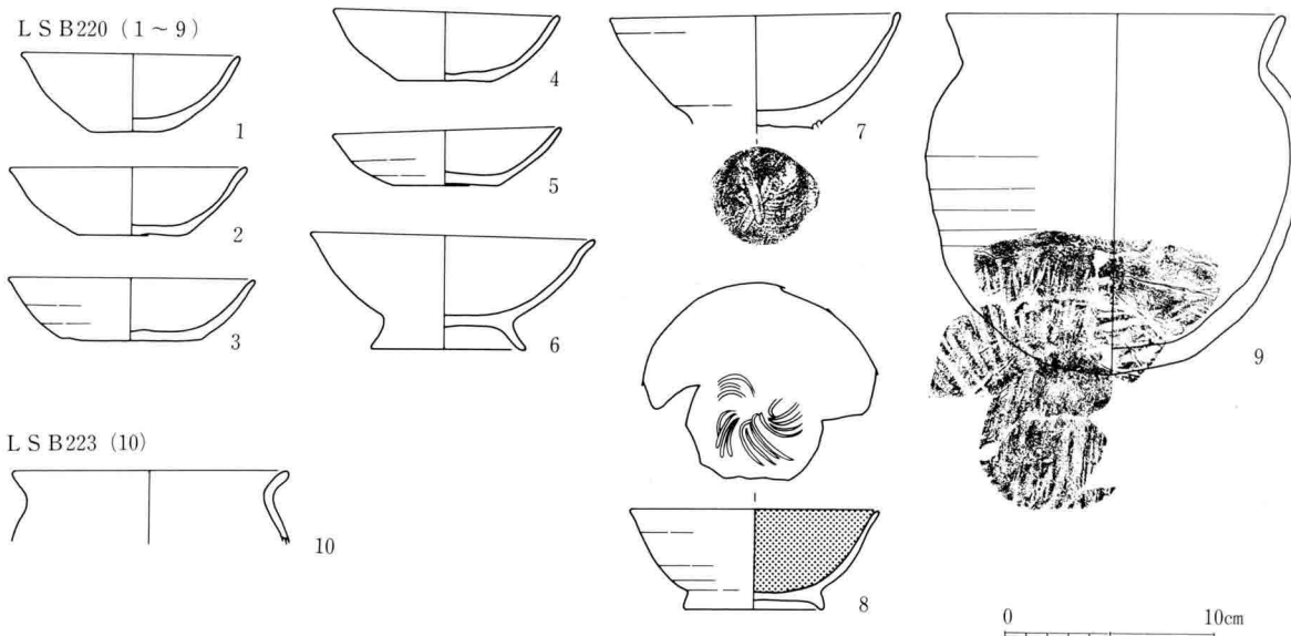
68図 L S B 220・223出土土器実測図(1:4)
