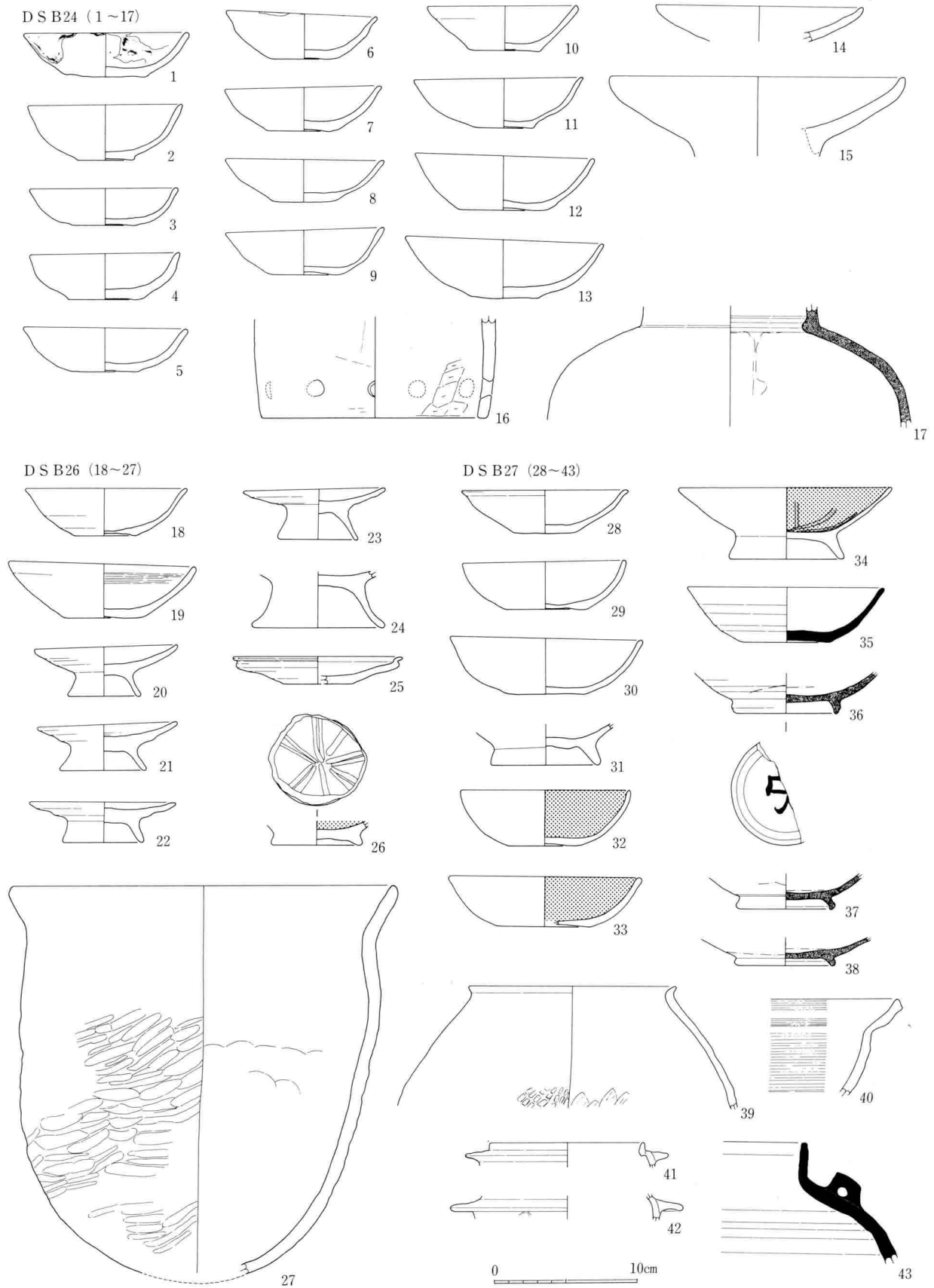
46图 DS B24・26・27出土土器実測図(1:4)
