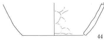
26图 CSB 1~3·5 出土土器实测图 (1:4)
