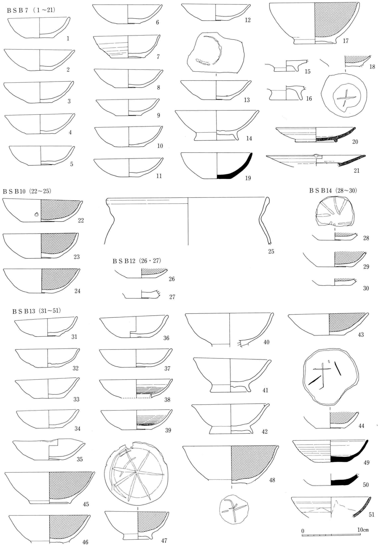
24图 BSB 7・10・12~14出土土器实测图(1:4)
