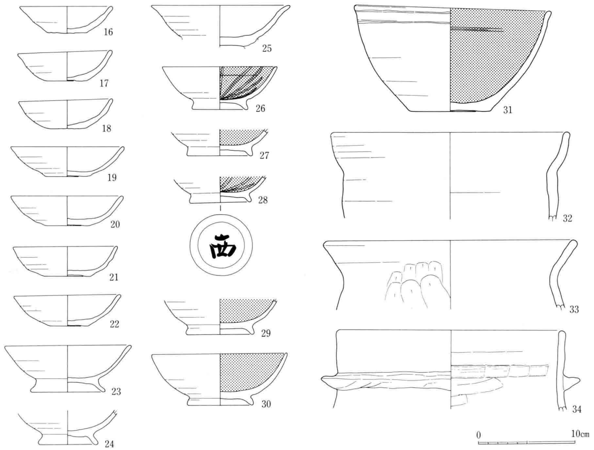
43図 DSB17・19出土土器実測図(1:4)
