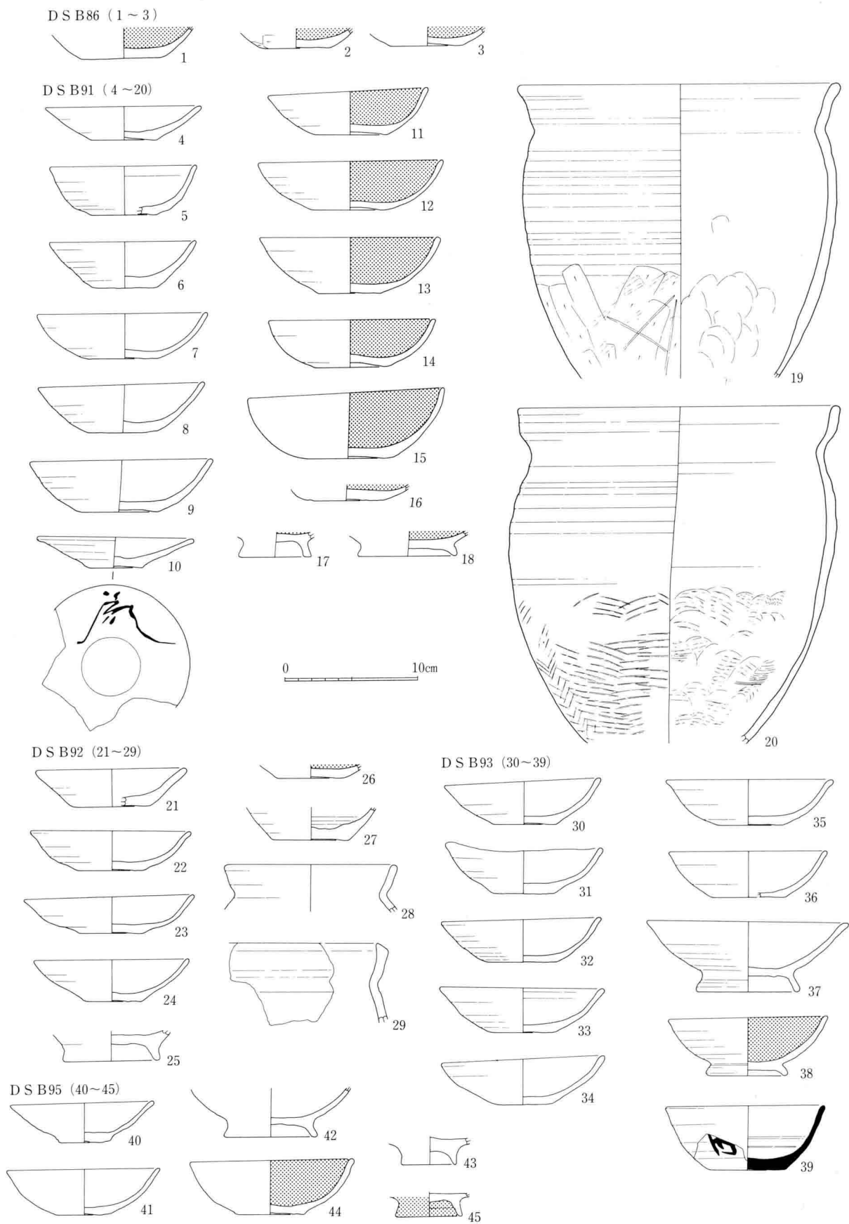
58图 DS B86・91~93・95出土土器実测图(1:4)
