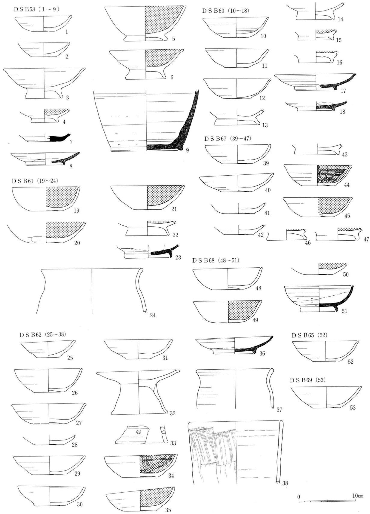
53图 DS B58 · 60~62 · 65 · 67~69出土土器实测图 (1 : 4)
