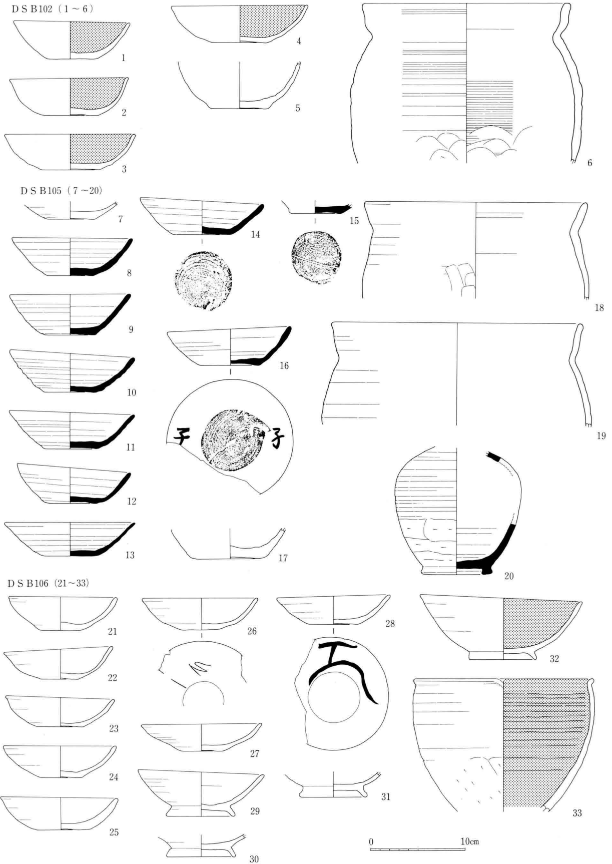
61図 D S B102・105・106出土土器実測図（1：4）
