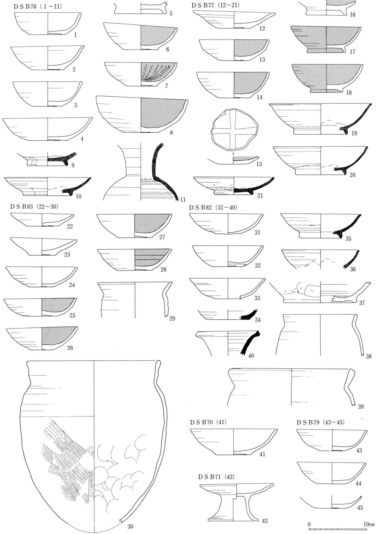
56图 DSB70·71·76·77·79·82·83出土土器实测图(1:4)
