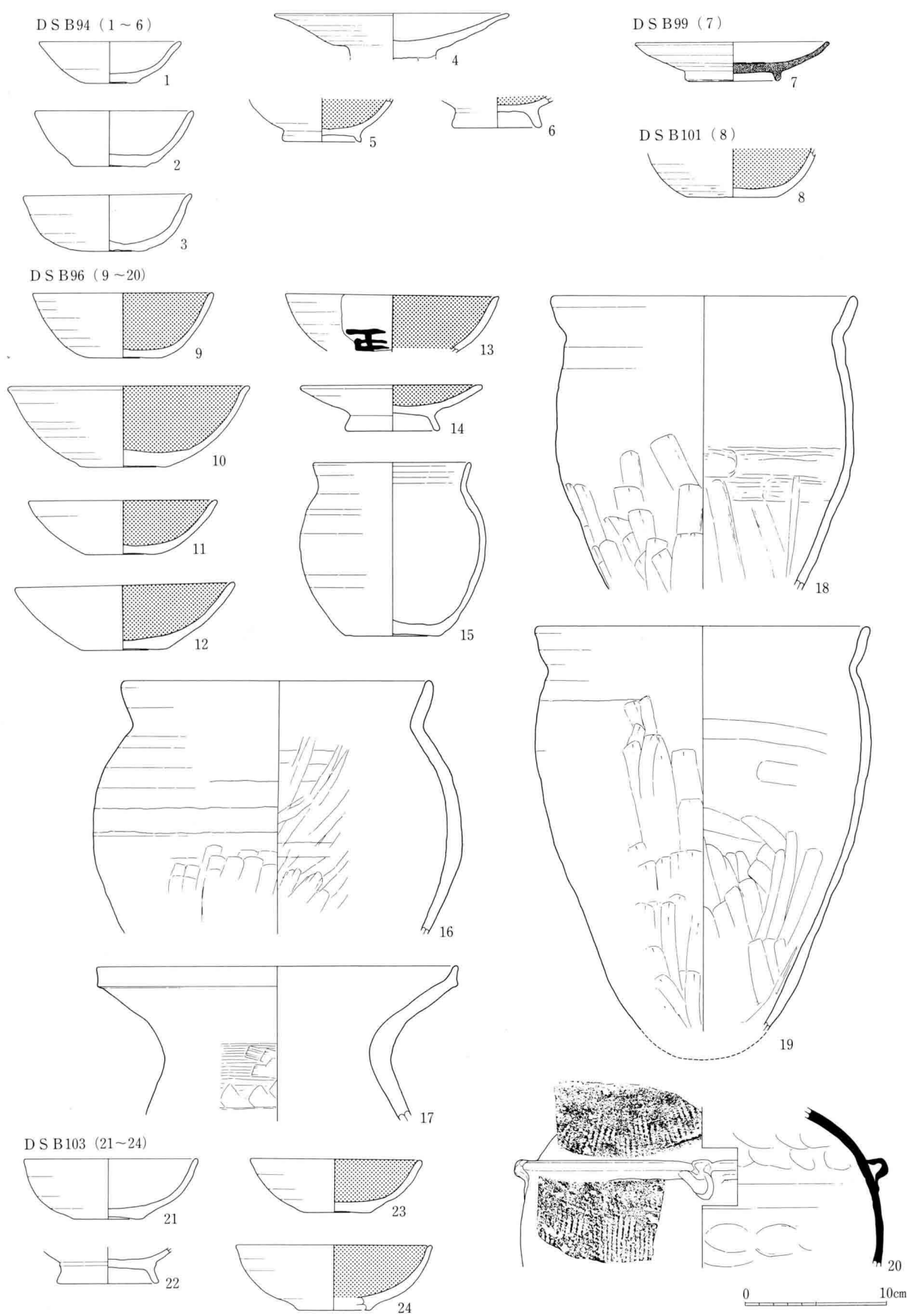
59图 DSB94·96·99·101·103出土土器实测图(1:4)
