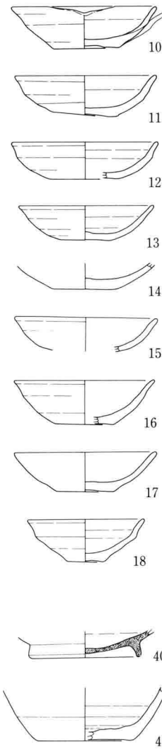
6 图 AS B15 · 16 · 23出土土器实测图 (1 : 4)
