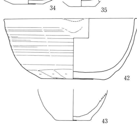
40图 DSB 6・8・9出土土器实测图(1:4)
