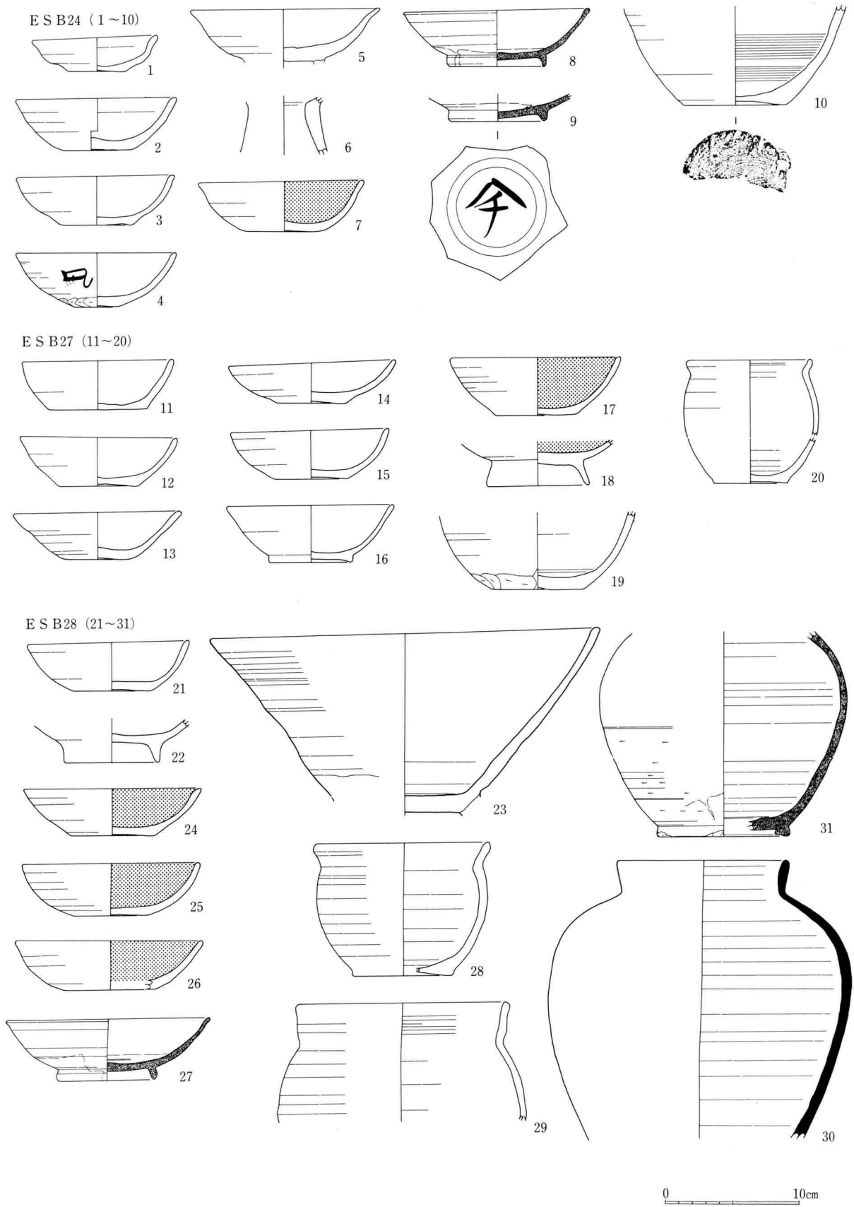
75図 ESB24・27・28出土土器実測図(1:4)
