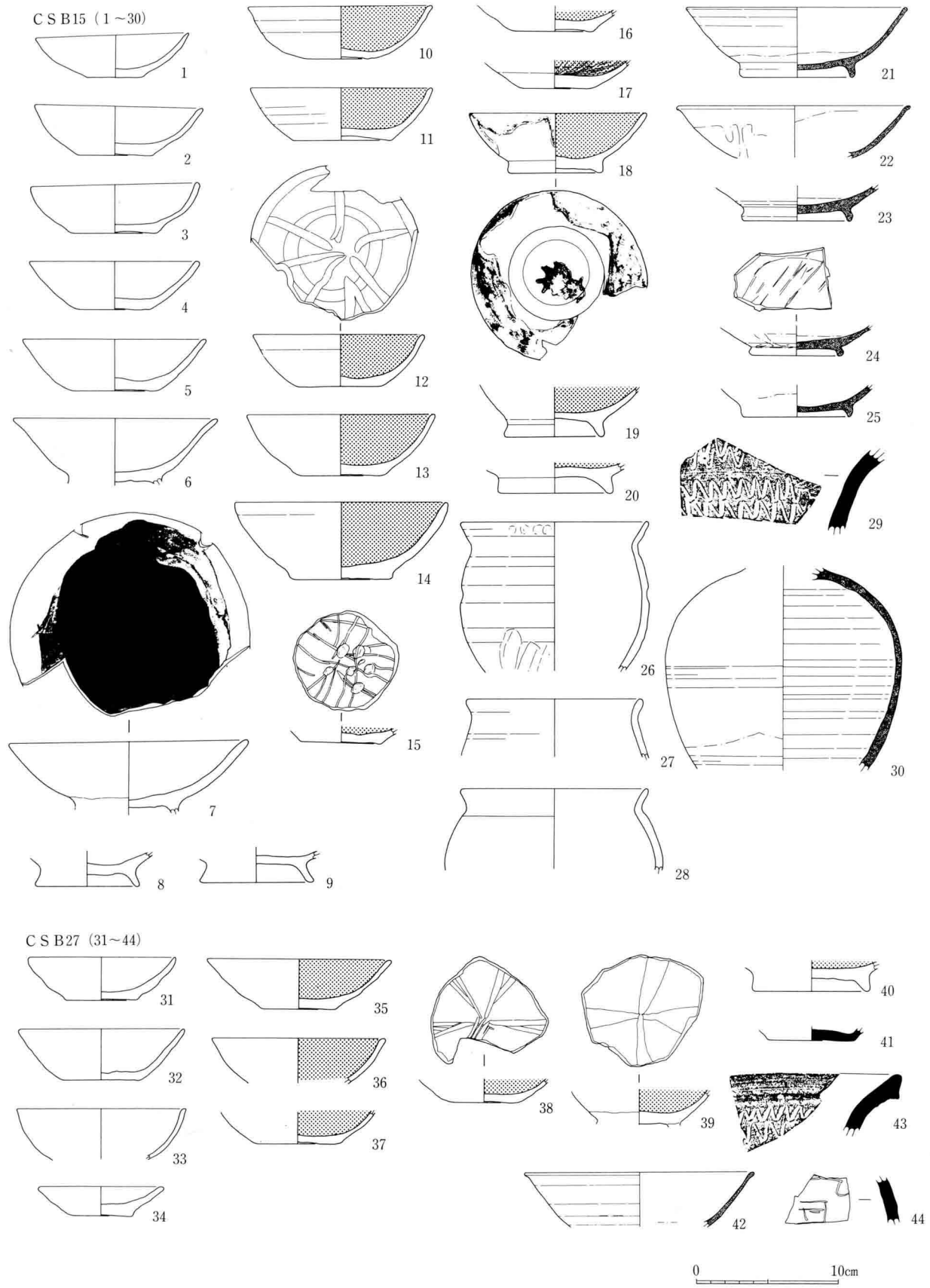
31图 CS B15·27出土土器实测图(1:4)
