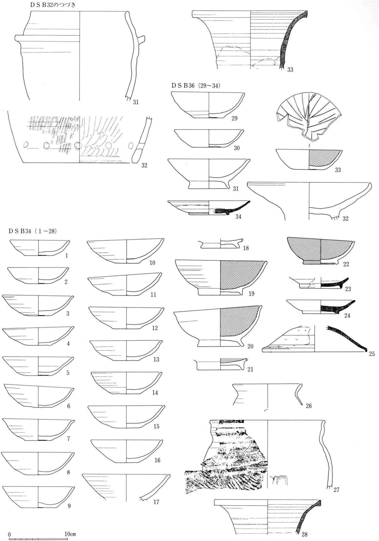
49図 DSB32・34・36出土土器実測図(1:4)
