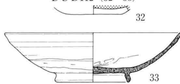
62图 DSB107·108·110·112·113出土土器实测图(1:4)
