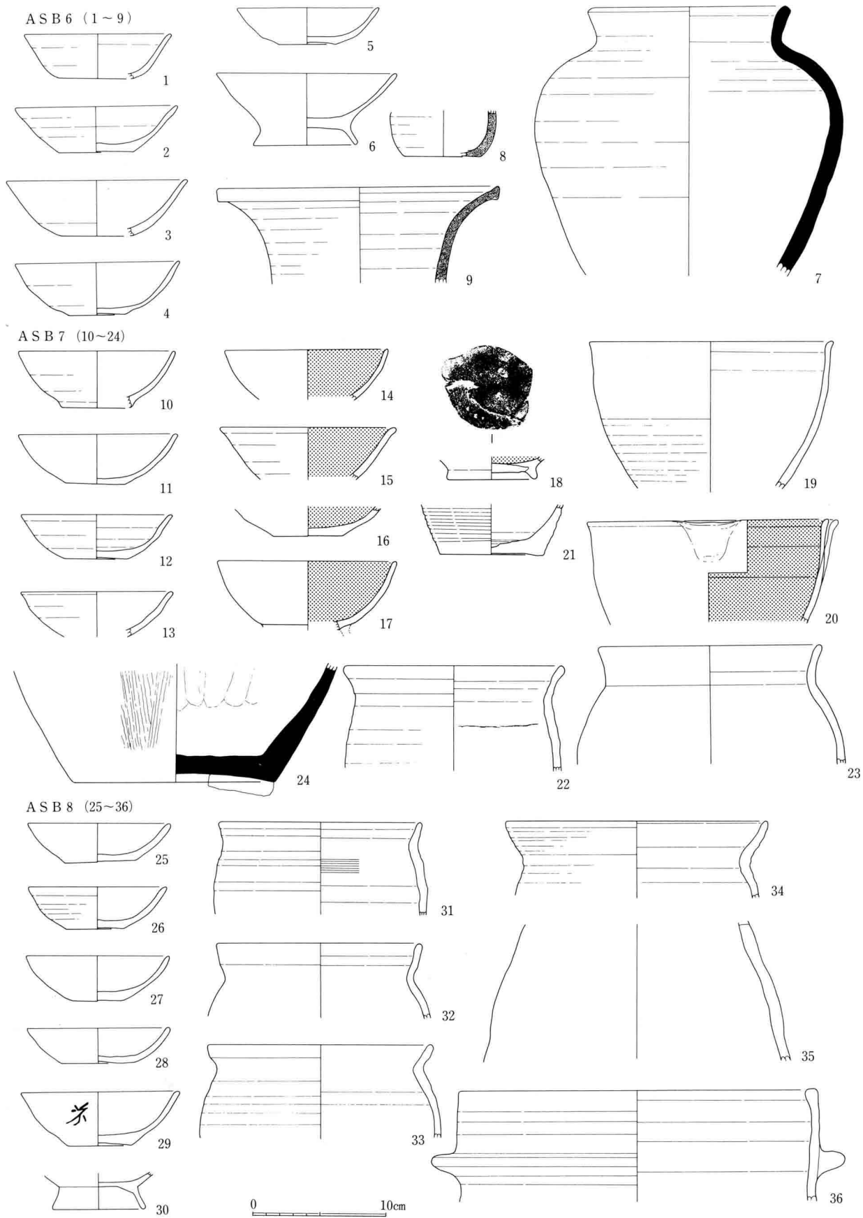
3 図 ASB 6 ~ 8 出土土器実測図 (1 : 4)
