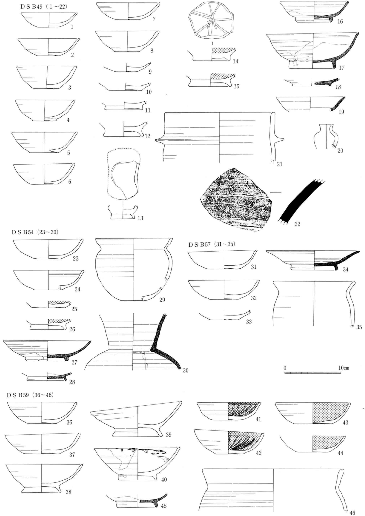
52图 DSB49·54·57·59出土土器实测图(1:4)
