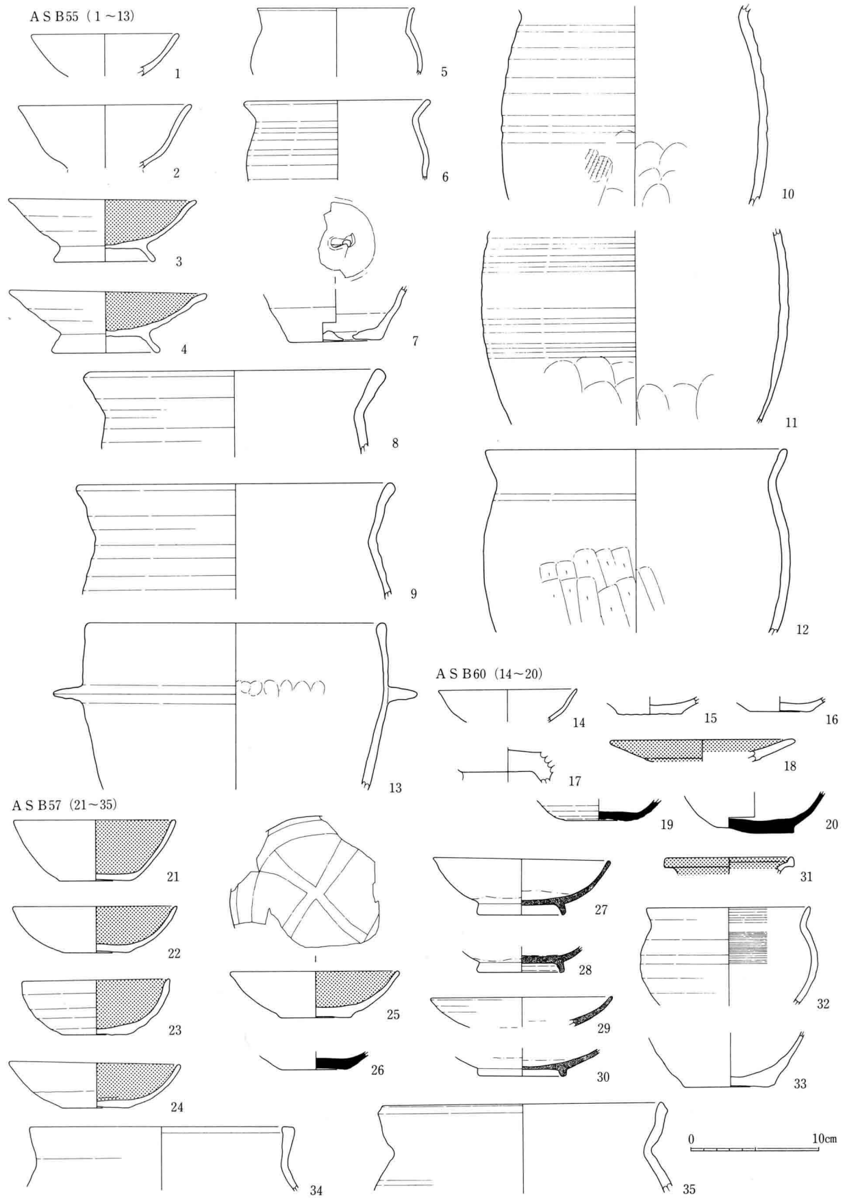
17图 ASB55·57·60出土土器实测图(1:4)
