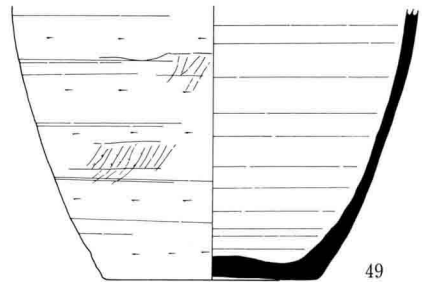
70图 ESB 1~3·6·7 出土土器实测图 (1:4)
