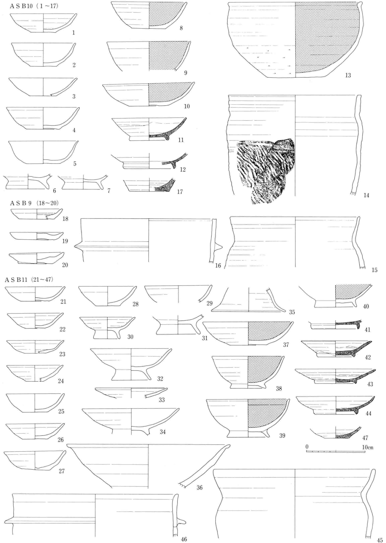
4 図 ASB9~11出土土器実測図(1:4)
