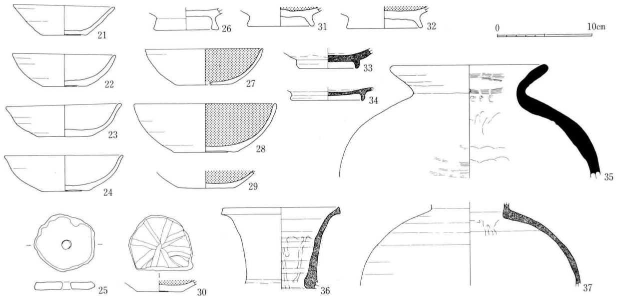
55图 DSB64·74出土土器实测图(1:4)
