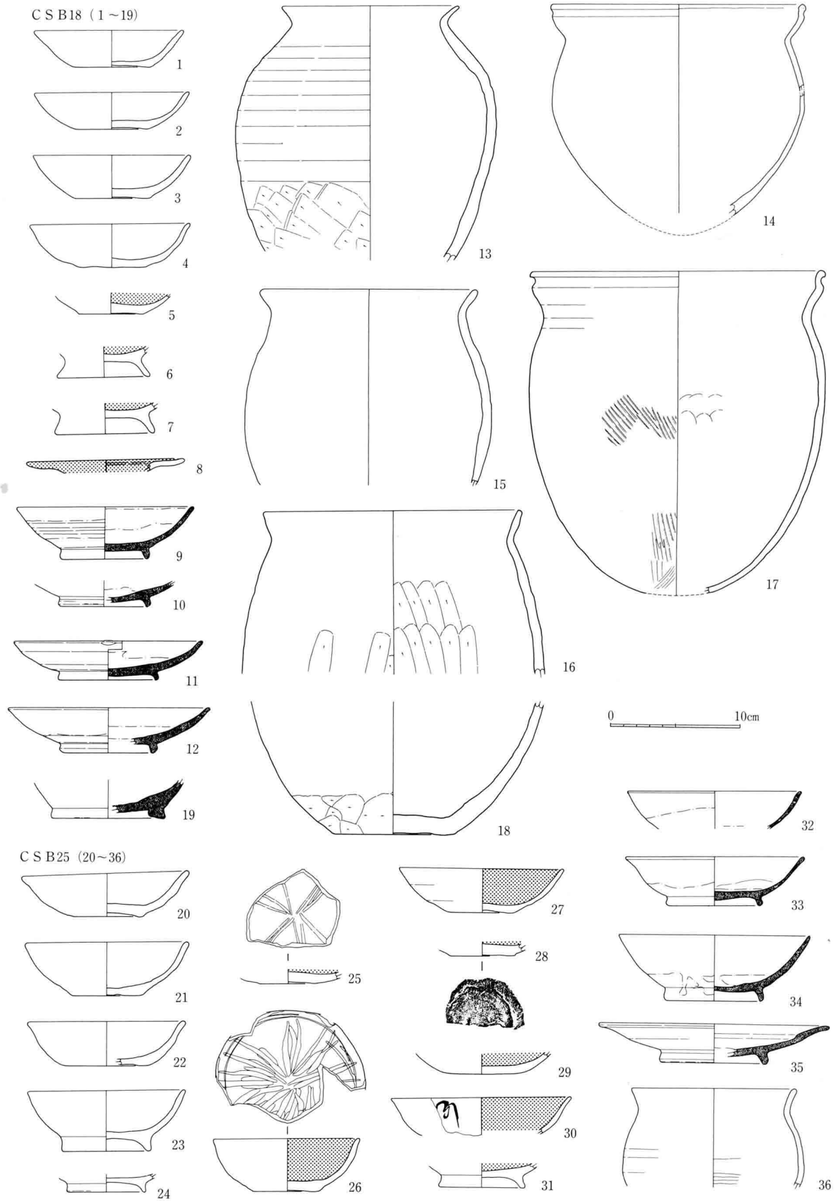
34图 CSB18·25出土土器实测图(1:4)
