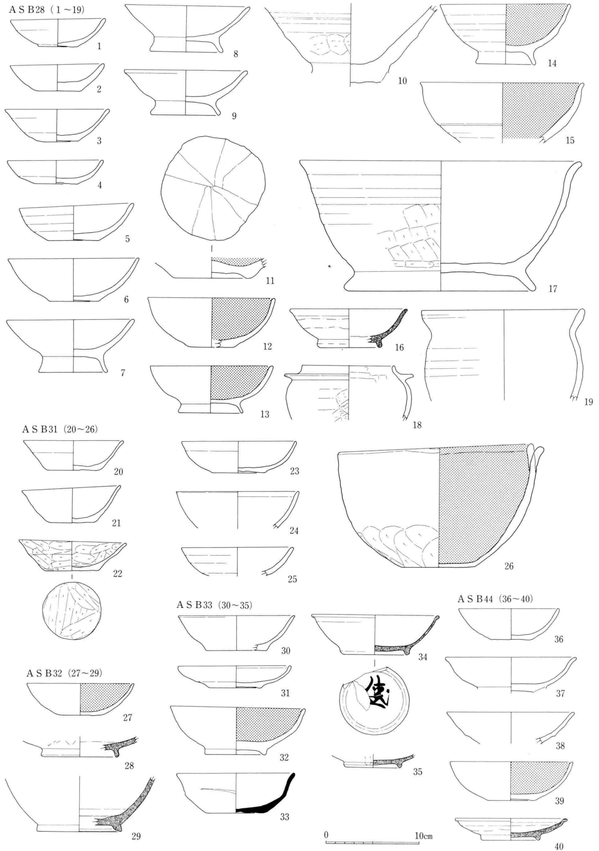
10图 ASB28・31~33・44出土土器实测图(1:4)
