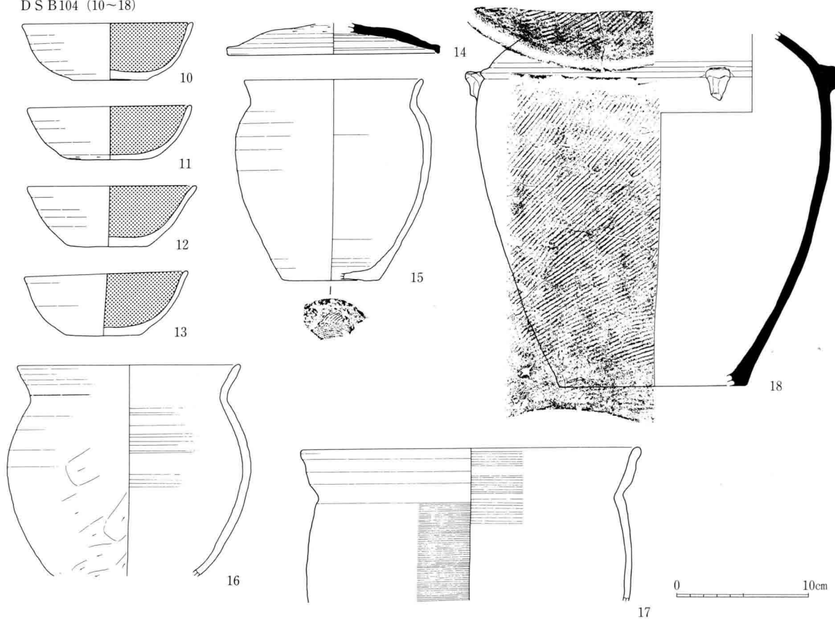
60図 DSB100・104出土土器実測図(1:4)
