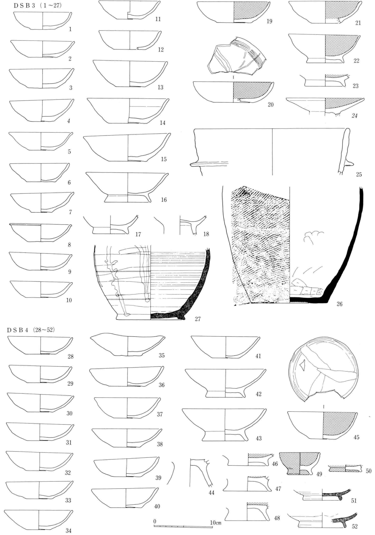
38图 DSB 3 · 4 出土土器实测图 (1 : 4)
