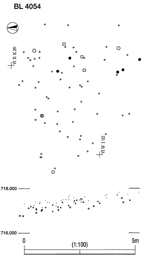
第4地点 BL4053・4054・4055・4056 遺物分布図 (貫ノ木遺跡)
