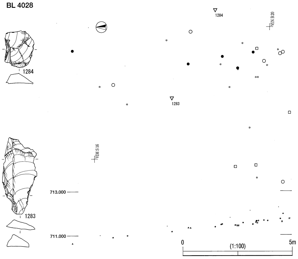
第4地点 BL4026・4027・4028 遺物分布図 (貫ノ木遺跡)
