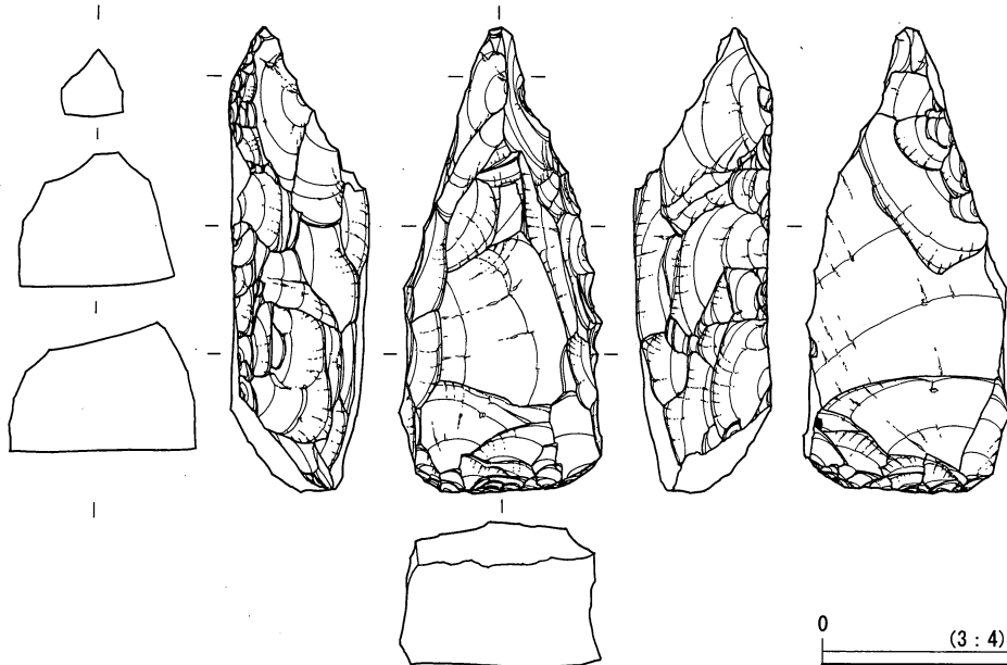
石器実測図 17 (槍先形尖頭器 6・角錐状石器) (西岡 A 遺跡)
