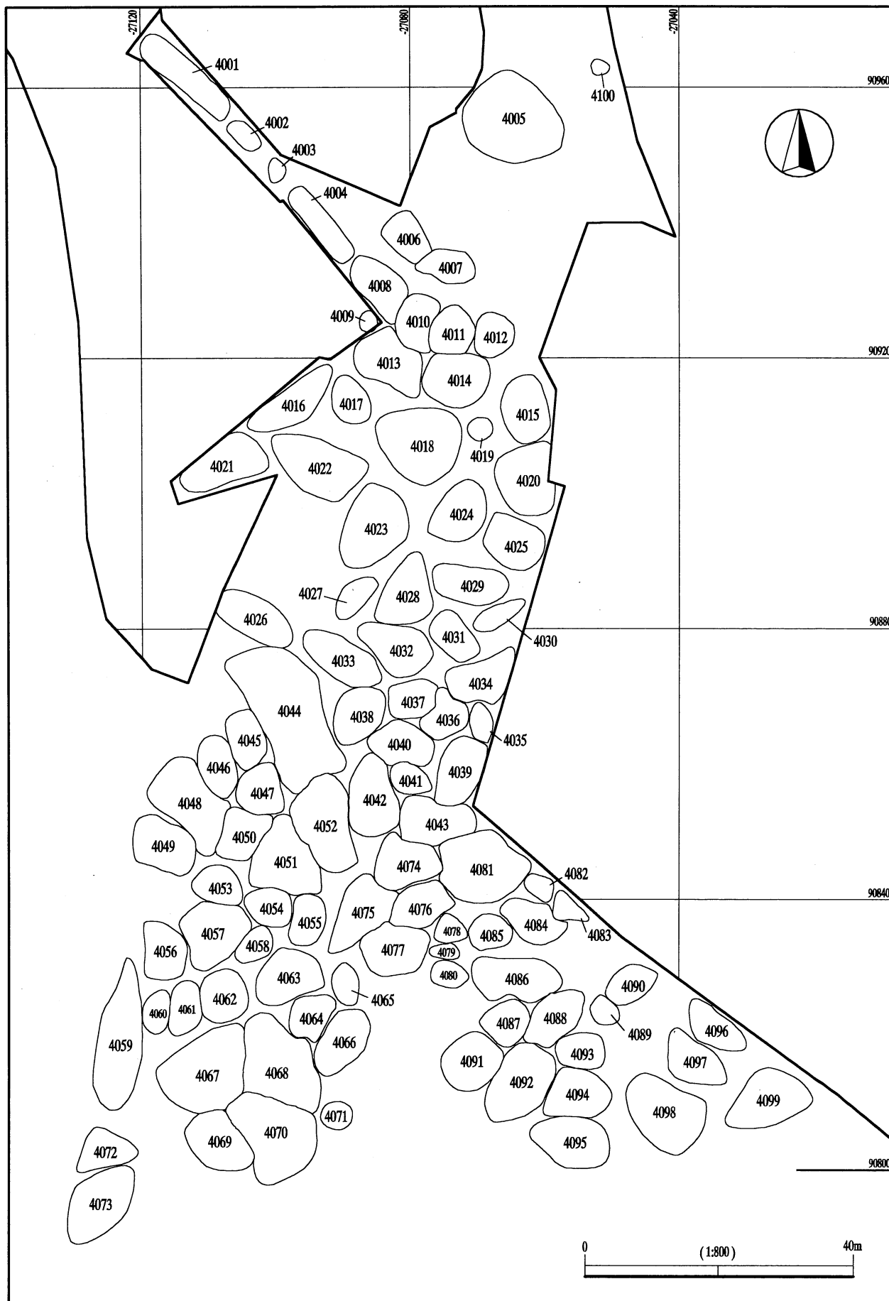
第4地点 ブロック配置図 (貫ノ木遺跡)
