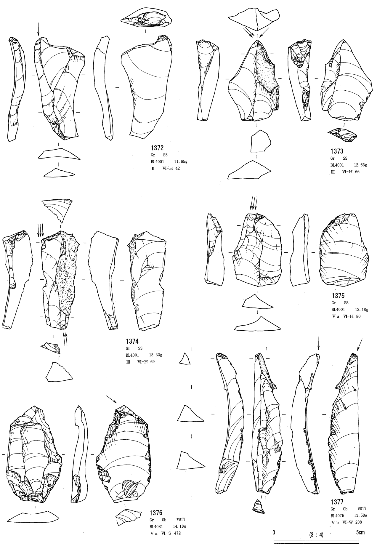
第4地点 石器実測図 29 (彫器 1) (貫ノ木遺跡)
