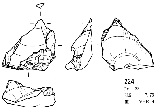
石器実測図 38 (挟入削器 3・揉錐器) (西岡 A 遺跡)
