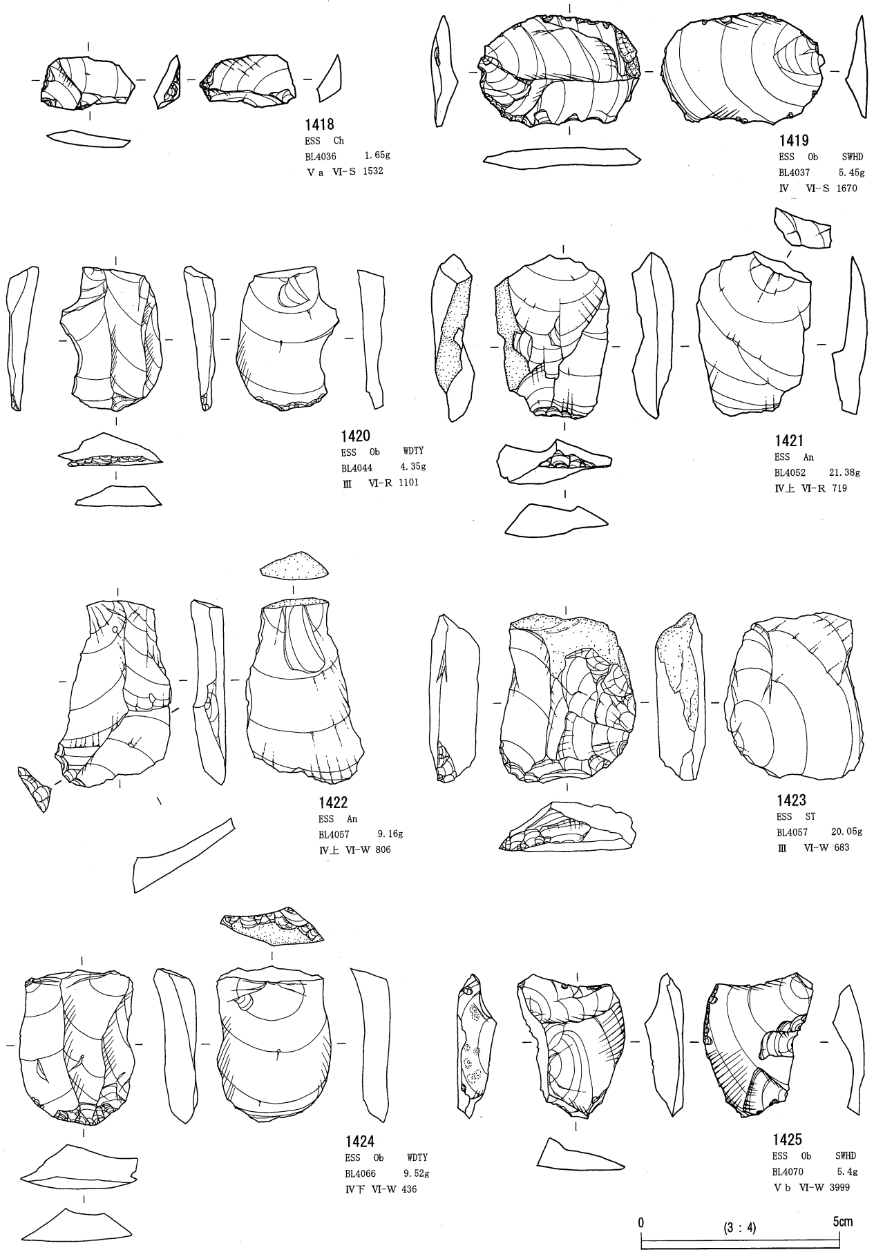
第4地点 石器実測図 39 (搔器状石器 2) (貫ノ木遺跡)
