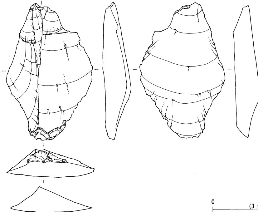
第2地点 石器実測図45 (搔器8) (貫ノ木遺跡)
