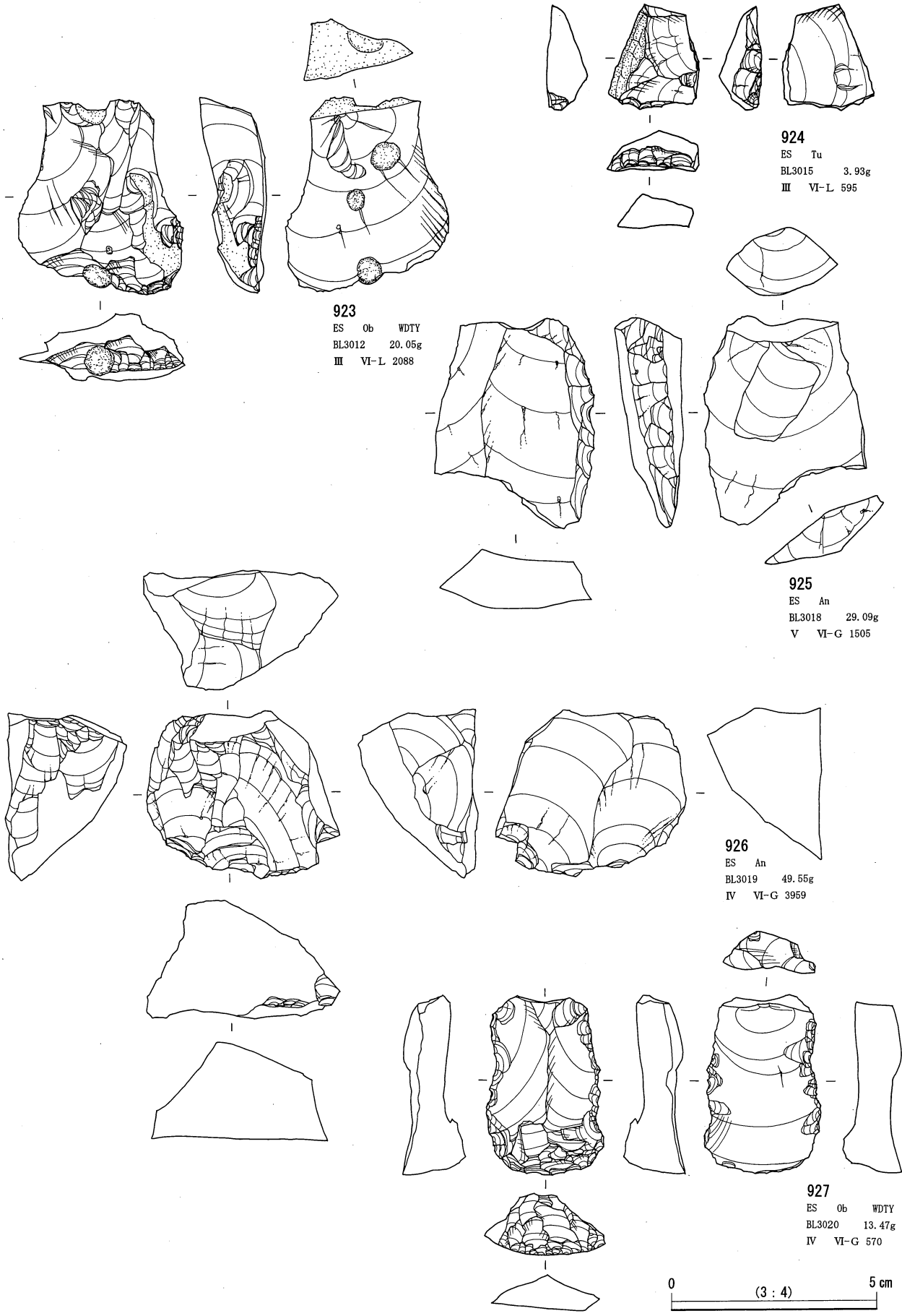
第3地点 石器実測図 34 (搔器 1) (貫ノ木遺跡)
