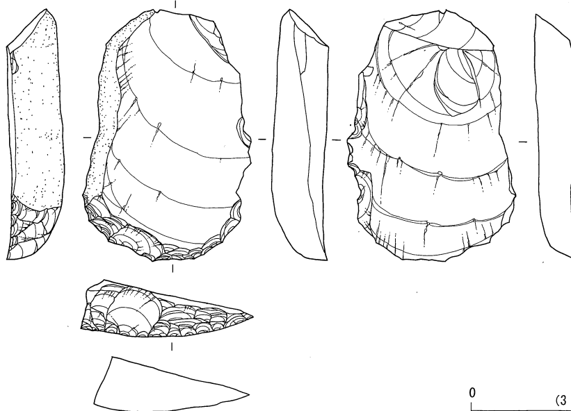
第1地点 石器実測図 21 (搔器 6) (貫ノ木遺跡)
