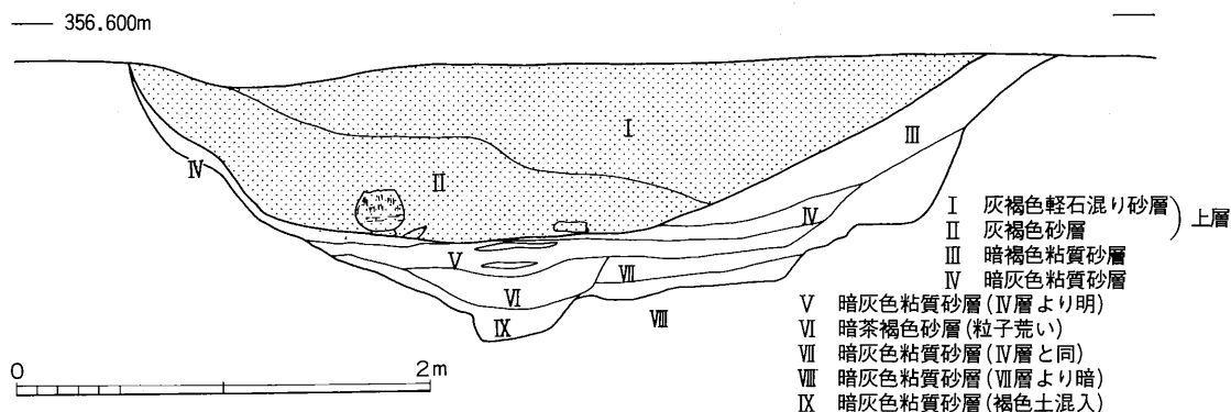
第20図 1号溝址断面図
