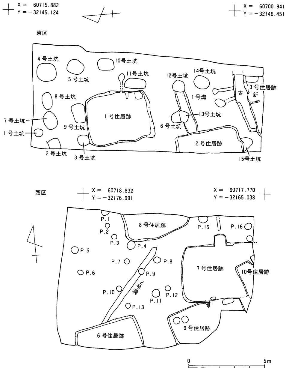
第7図 城ノ内遺跡全体図 (1 : 150)
