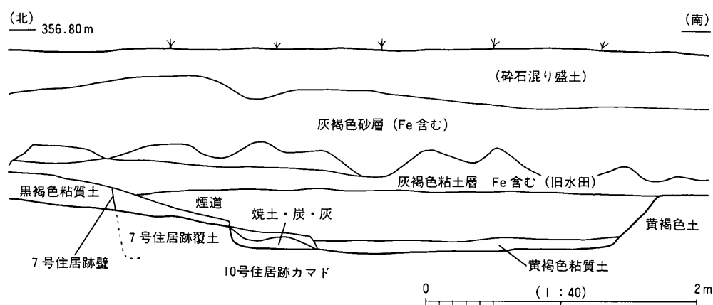
第8図 城ノ内遺跡基本層序
