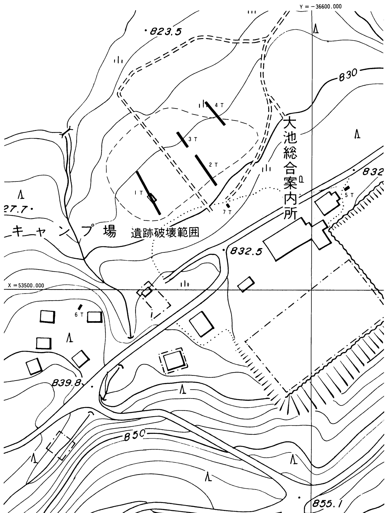
第25図 大池南遺跡調査区配置図 (1:1,000)
