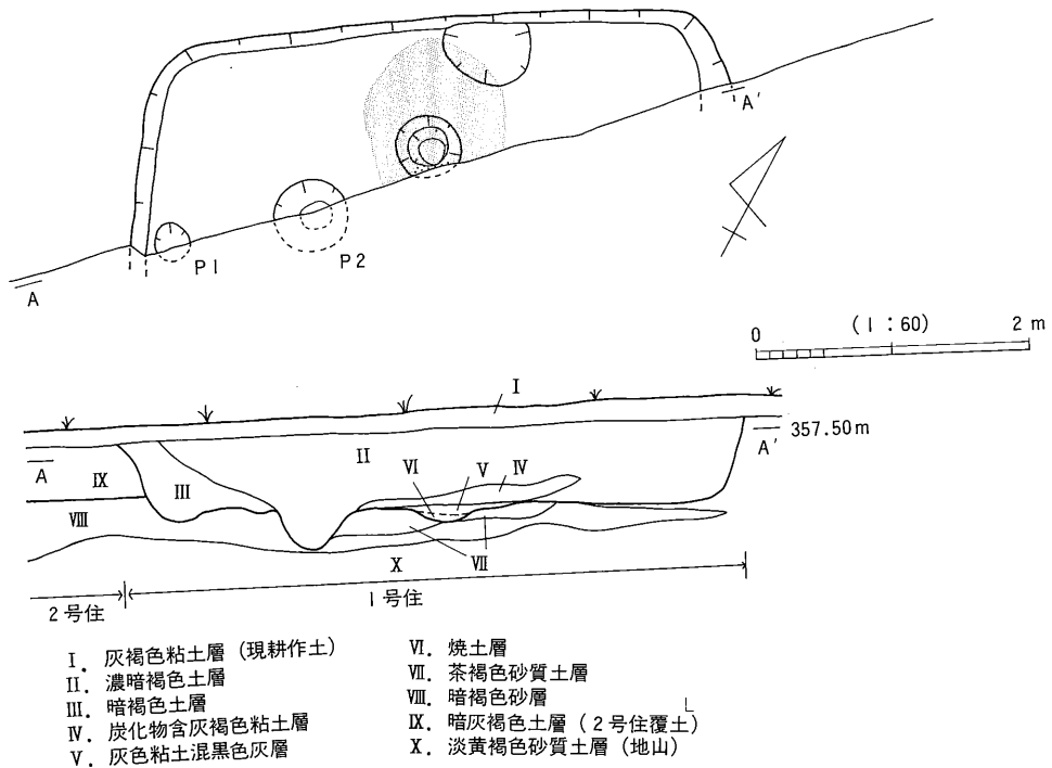
第72図 郷津遺跡1号住居址
