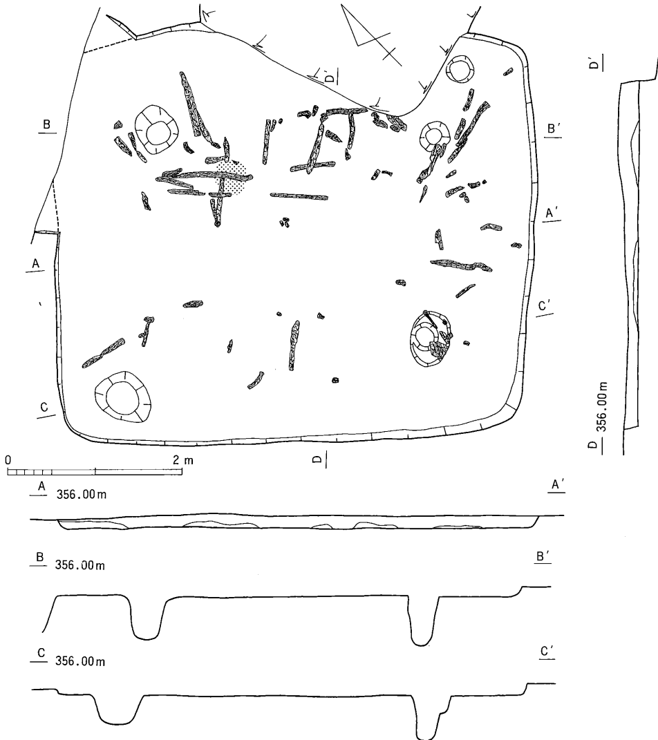
第63図 2号住居址
