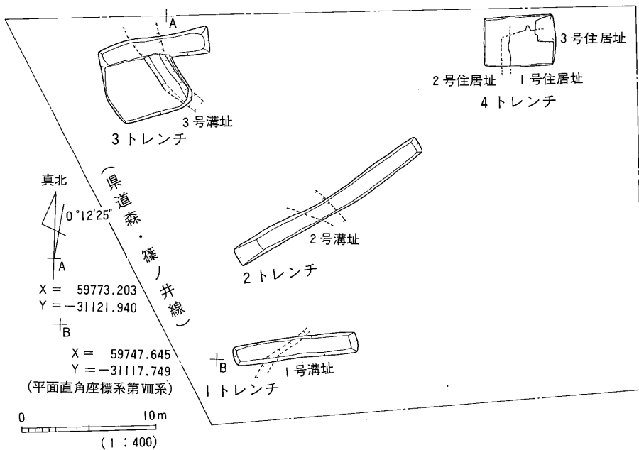
第76図 調査全体図
