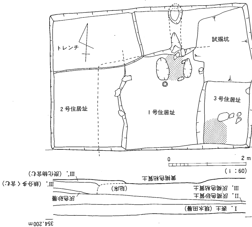
第77図 1号住居址
