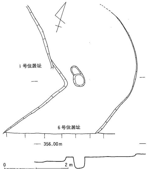
第59図 6号住居址
