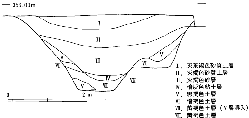
第67図 5号溝址断面図
