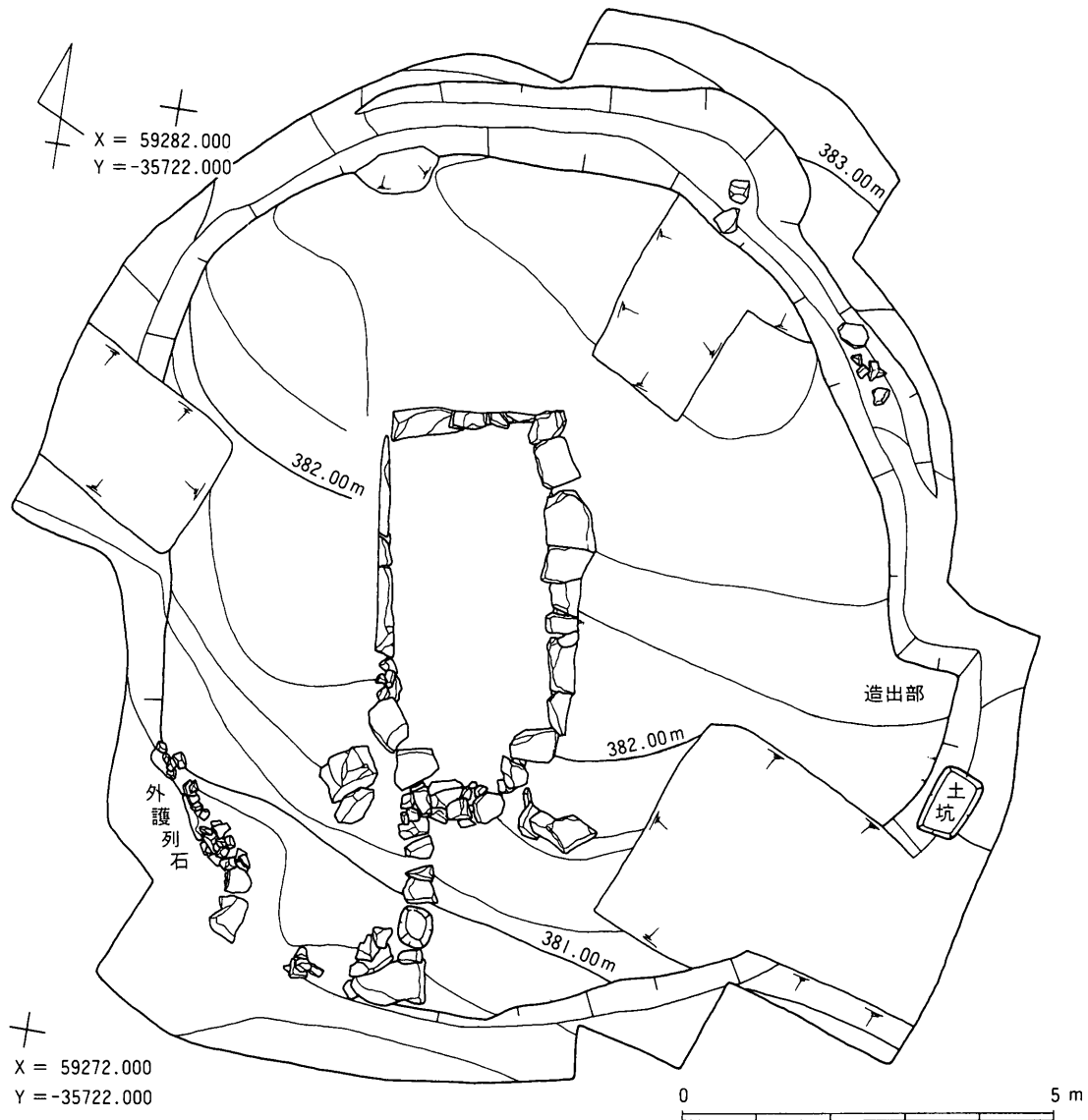
第19図 一本松古墳遺構全体図
