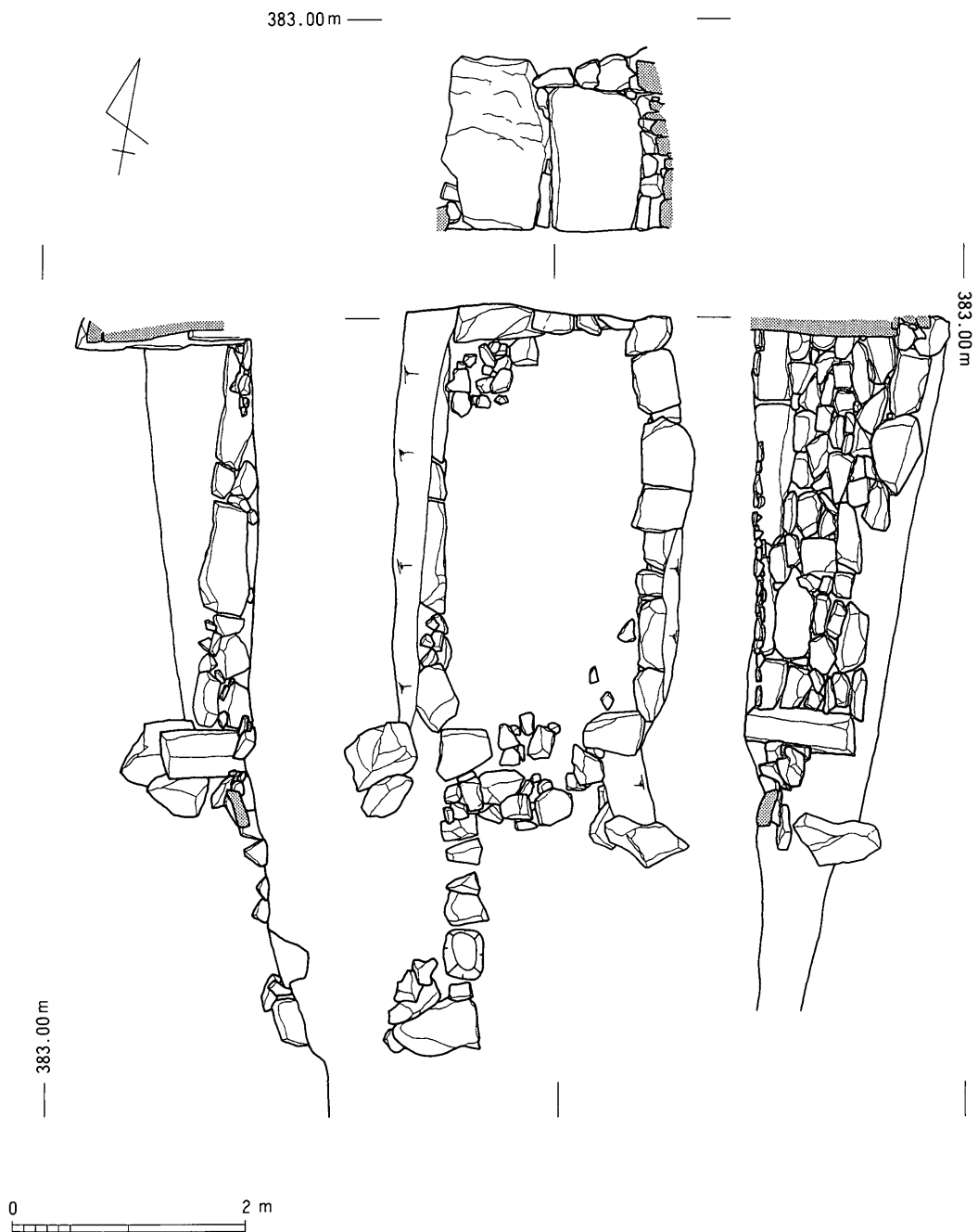
第20図 一本松古墳石室展開図
