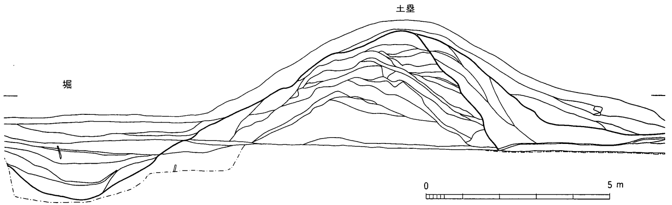
第17図 松田館跡土塁断面図
