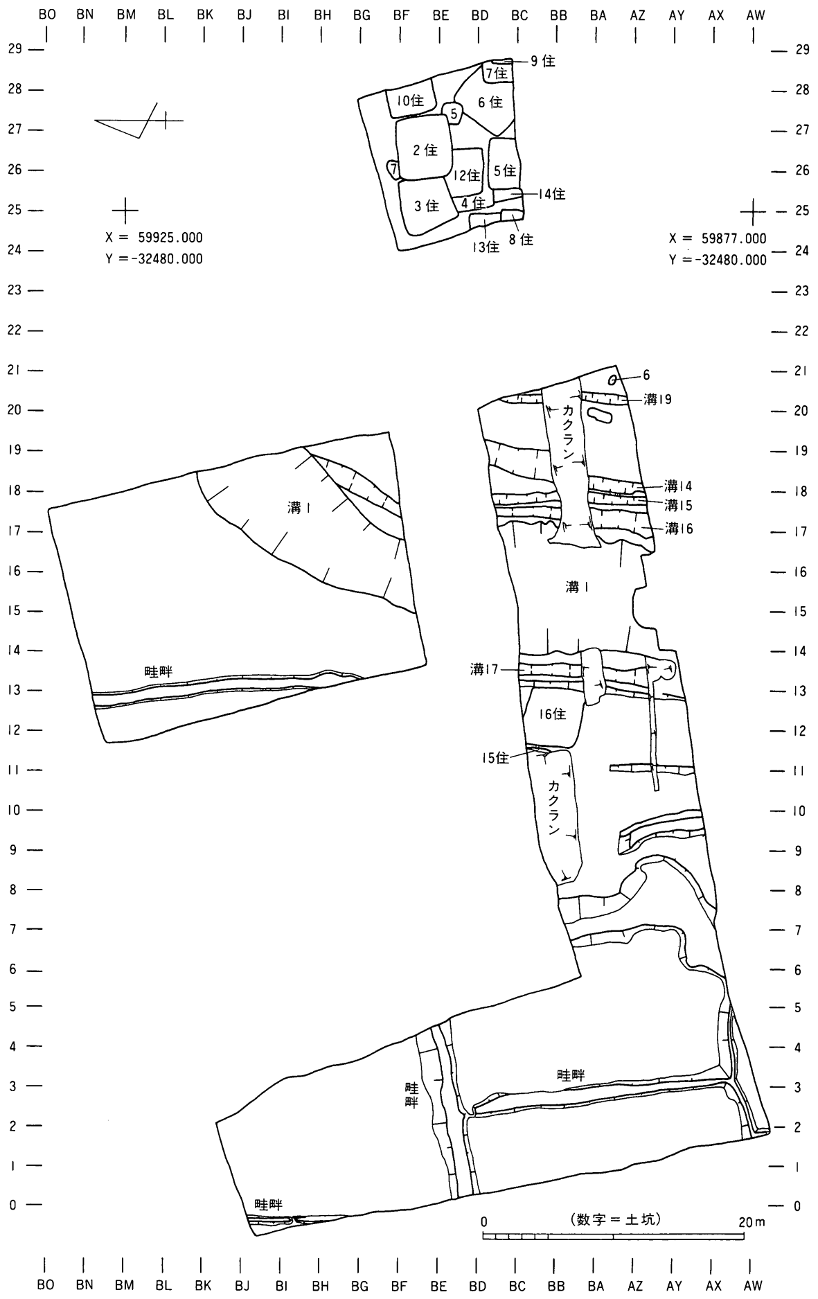
第11図 大塚遺跡遺構全体図
