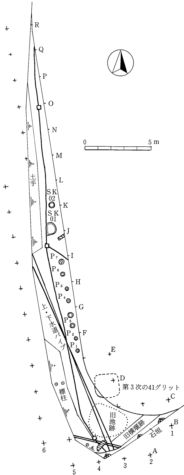
第5図 遺構全体図 (地下障害物を含む)
