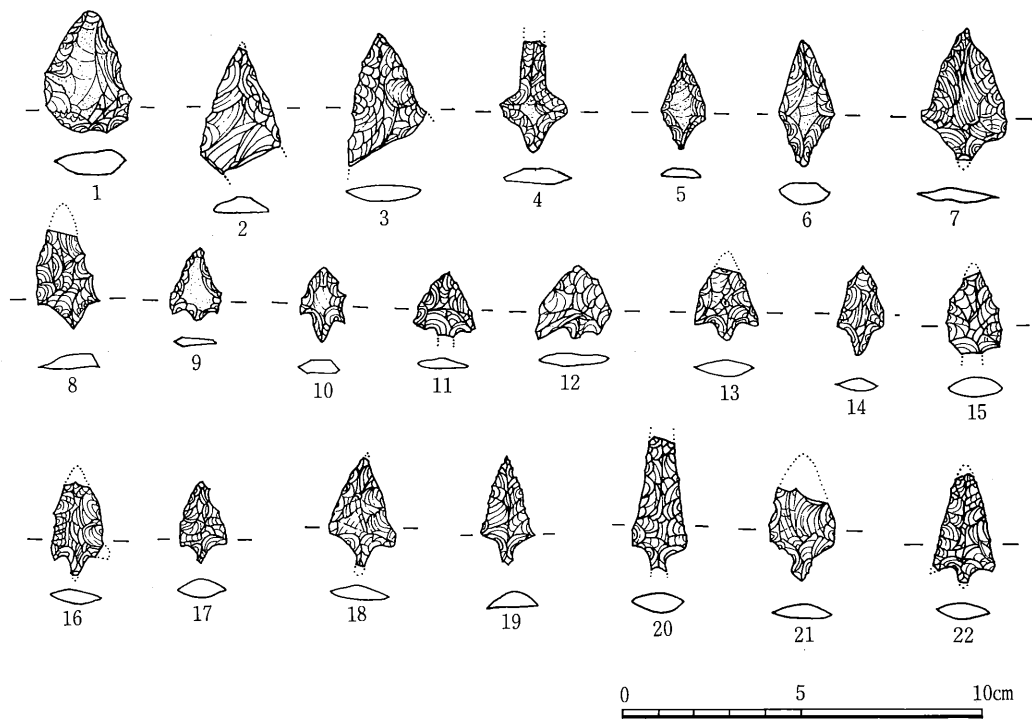
第11图 石器实测图
