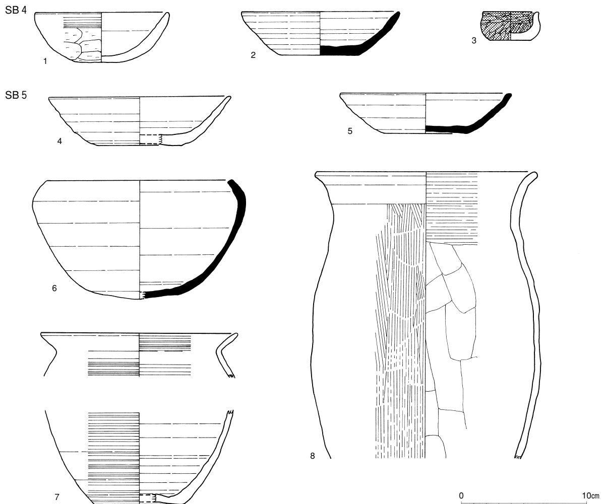
第23図 SB 4・SB 5 出土遺物実測図
