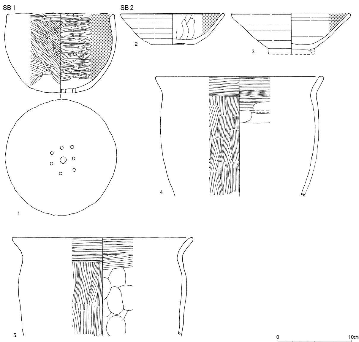
第40図 SB1・SB2 出土遺物実測図
