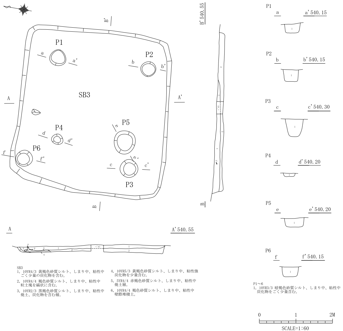
第33図 SB 3 実測図
