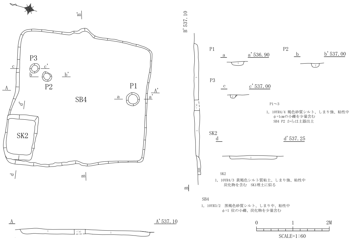
第17図 SB4 実測図
