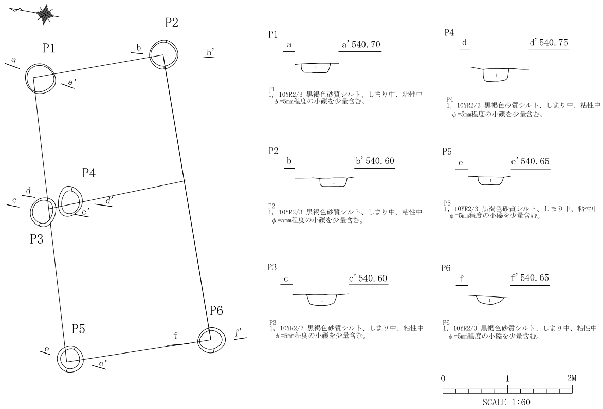
第39図 ST 4 実測図
