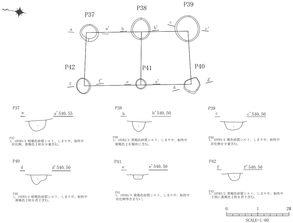
第38図 ST 3 実測図
