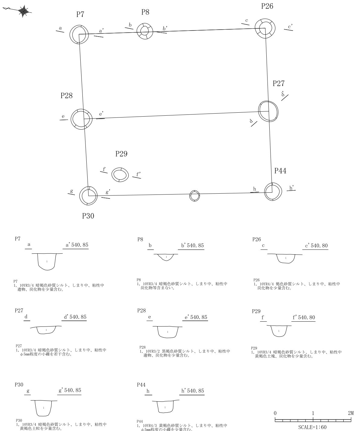
第37図 ST2 実測図
