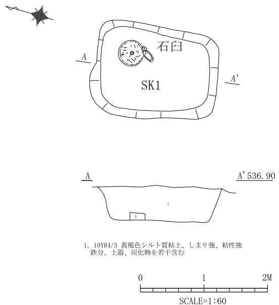
第21図 SK 1 実測図
