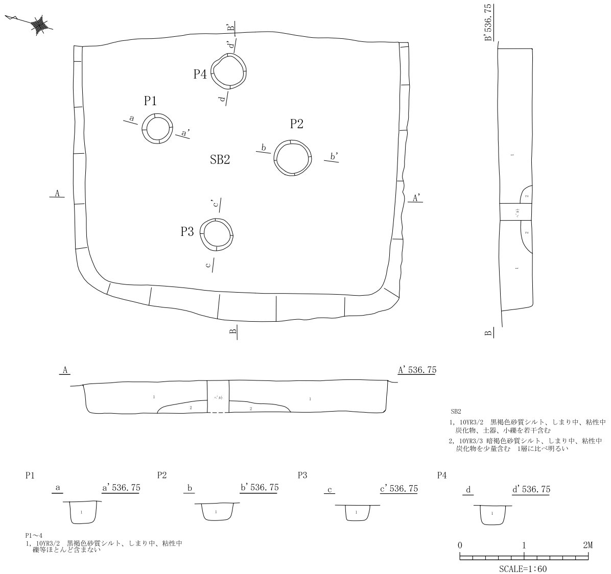
第15図 SB 2 実測図
