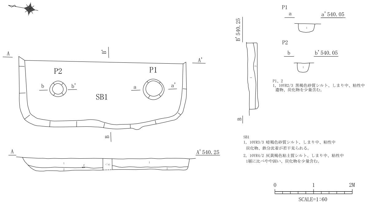
第31図 SB1 実測図
