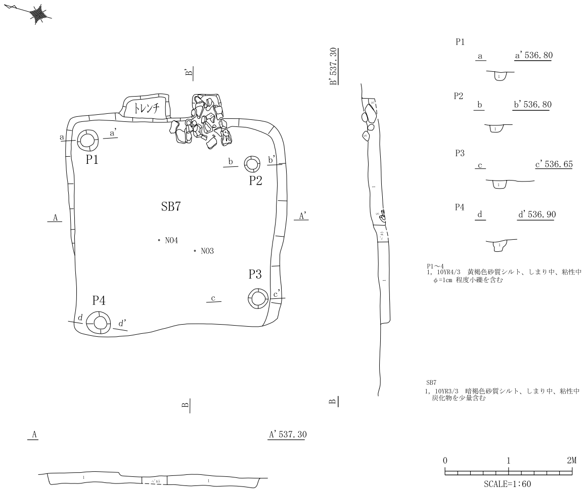
第19図 SB 7 実測図
