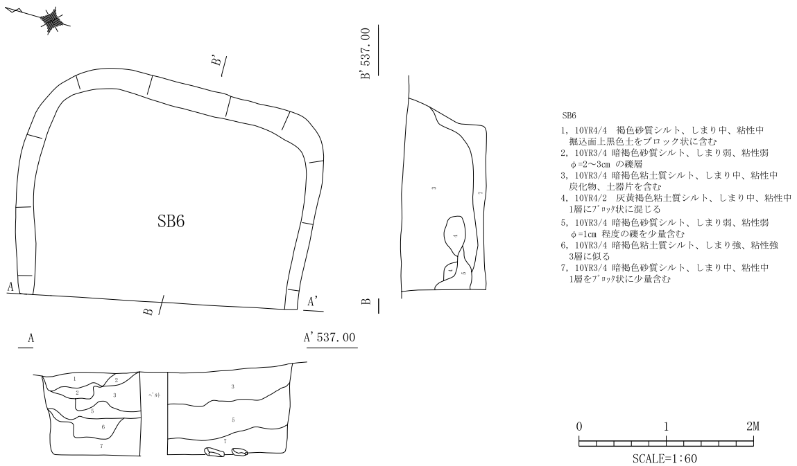
第20図 SB 6 実測図
