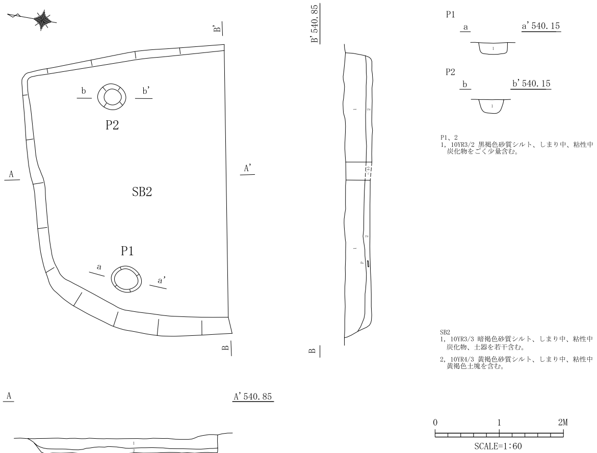
第32図 SB 2 実測図
