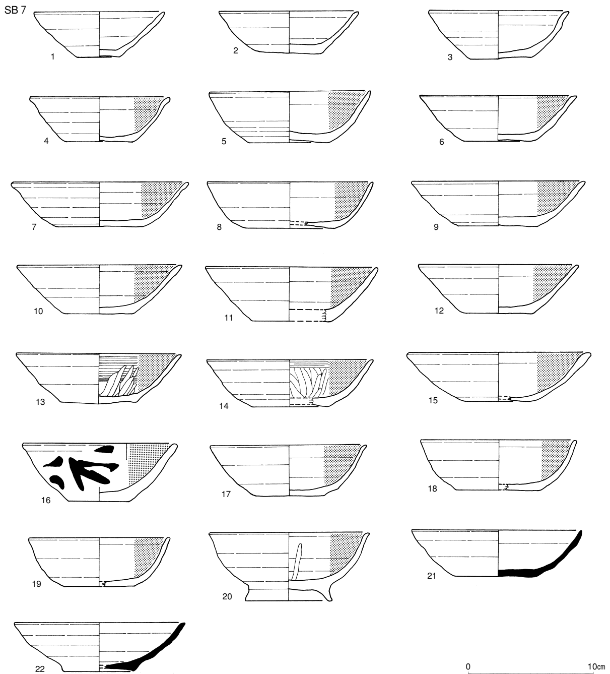
第24図 SB7 出土遺物実測図
