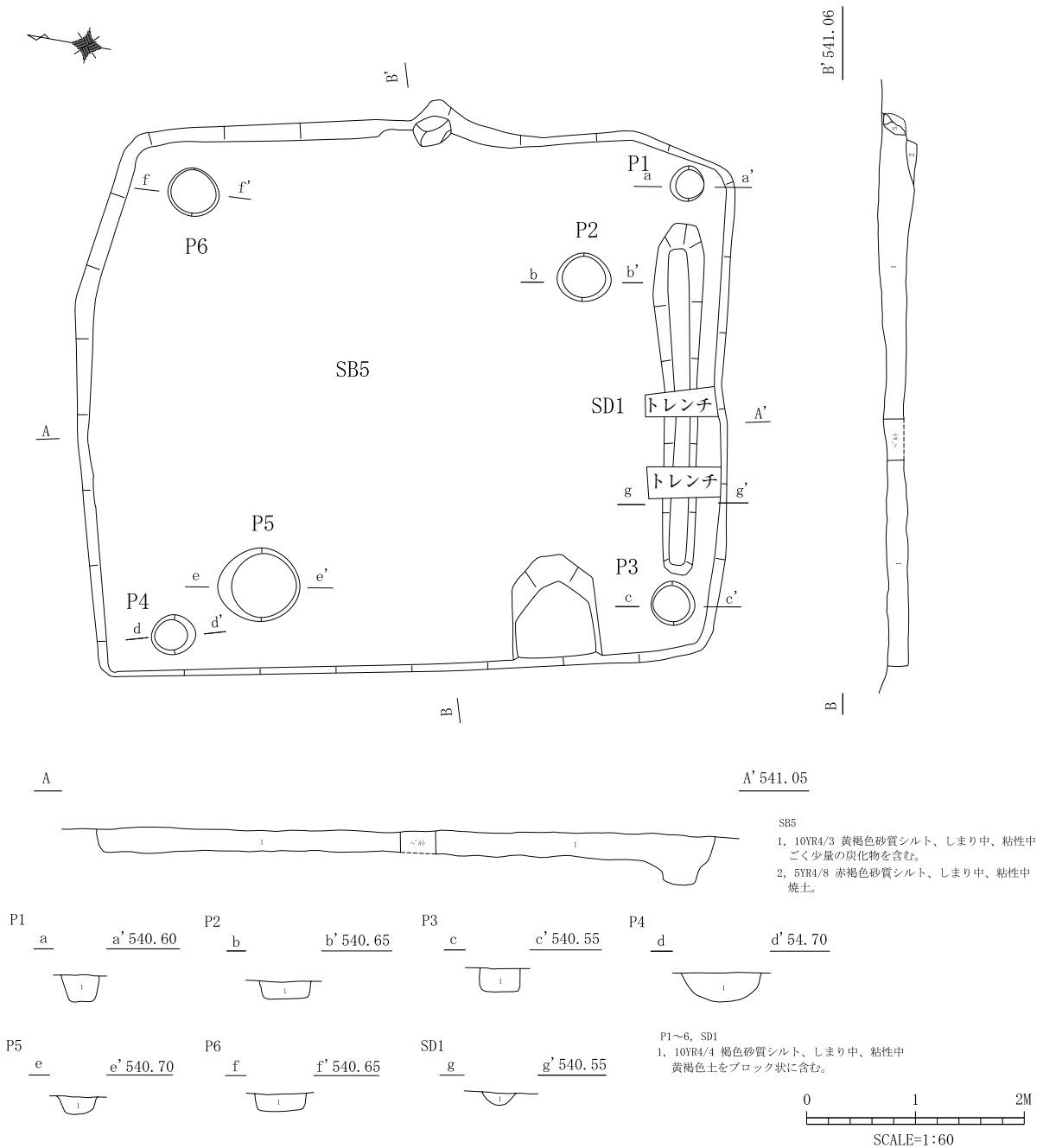
第35図 SB5 実測図
