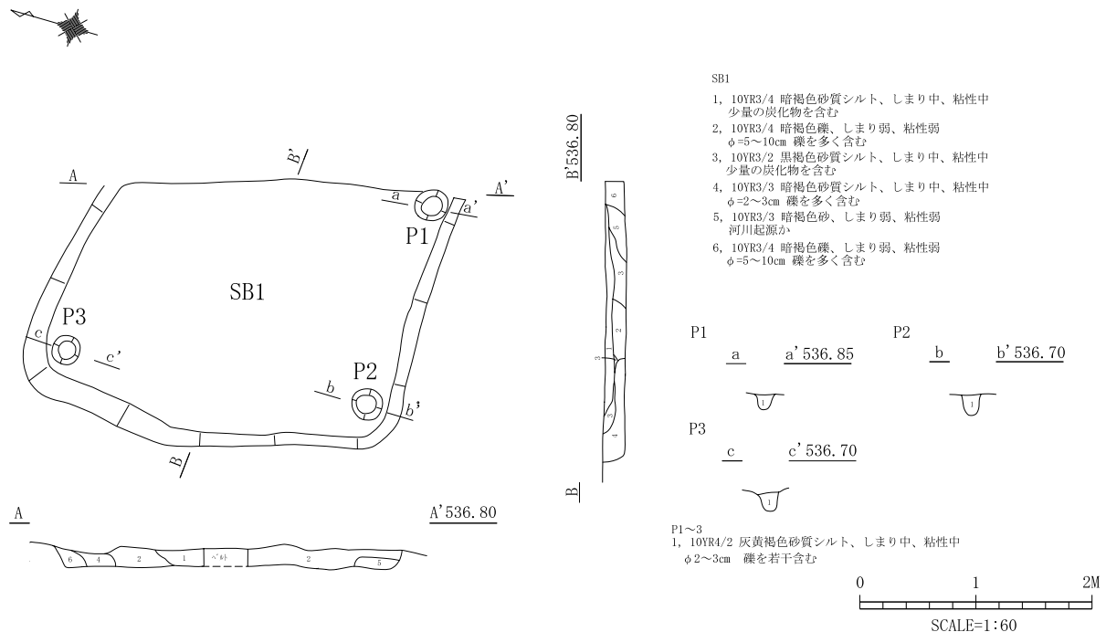
第14図 SB1 実測図
