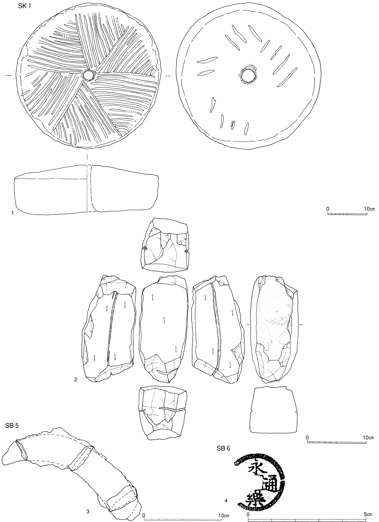
第27図 石製品・金属製品実測図
