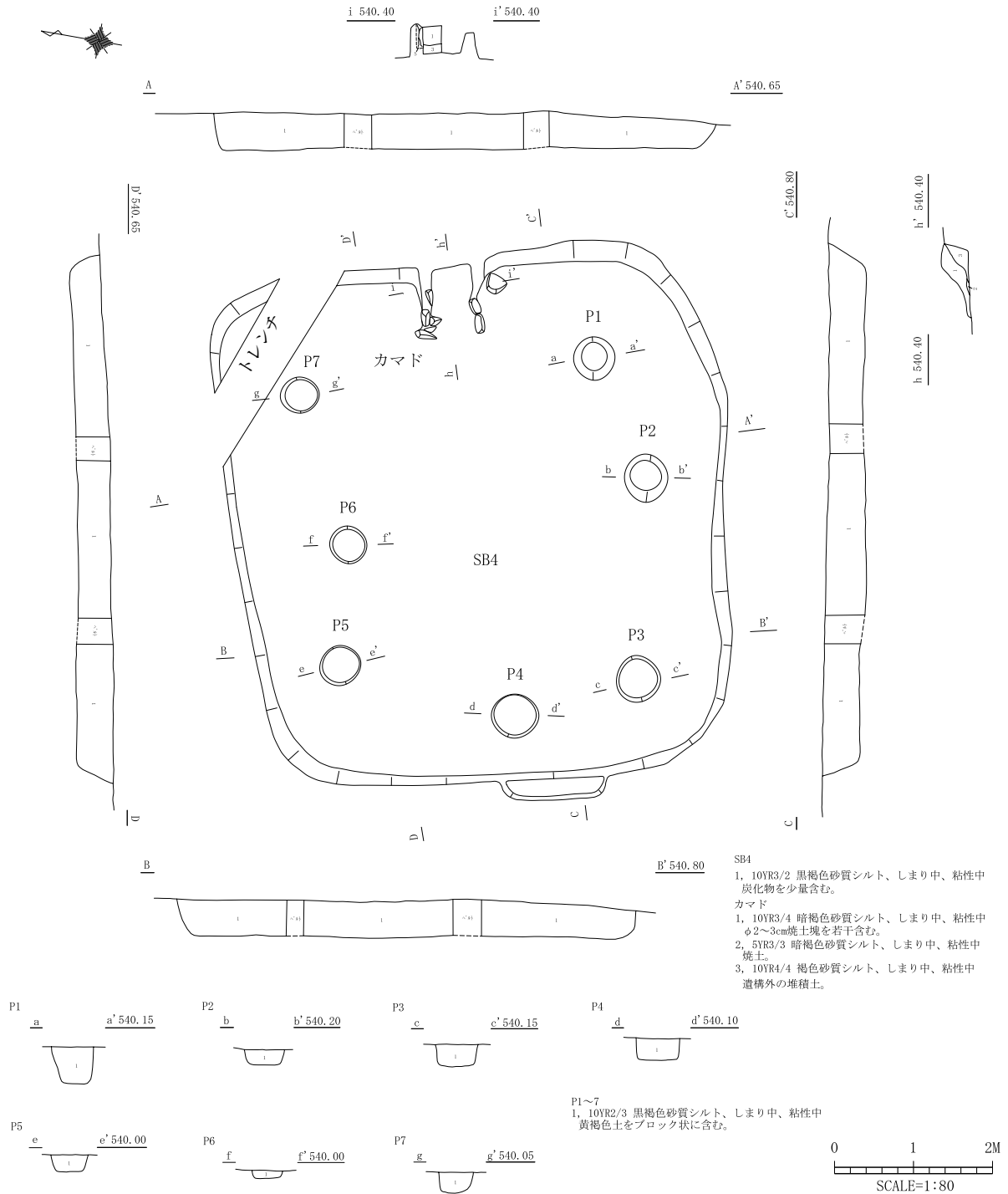
第34図 SB4 実測図
