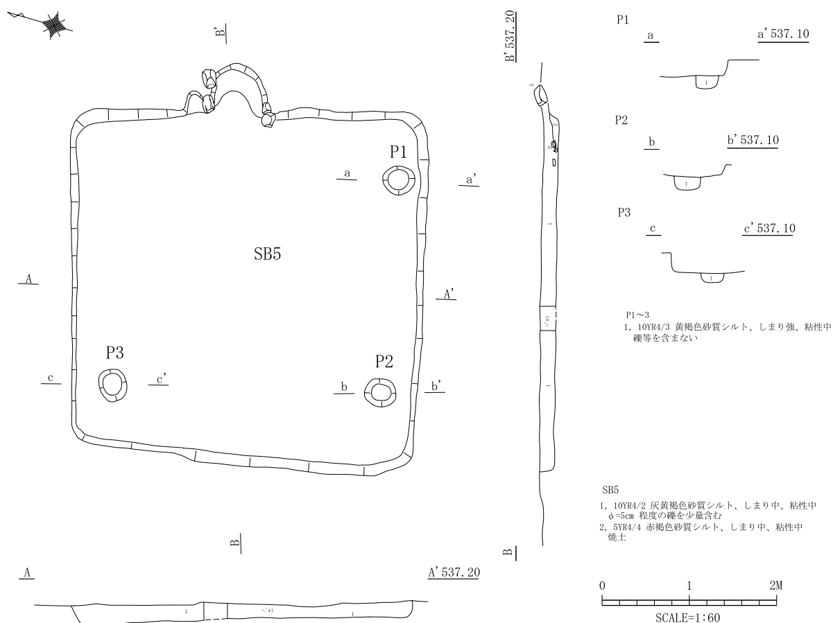
第18図 SB5 実測図
