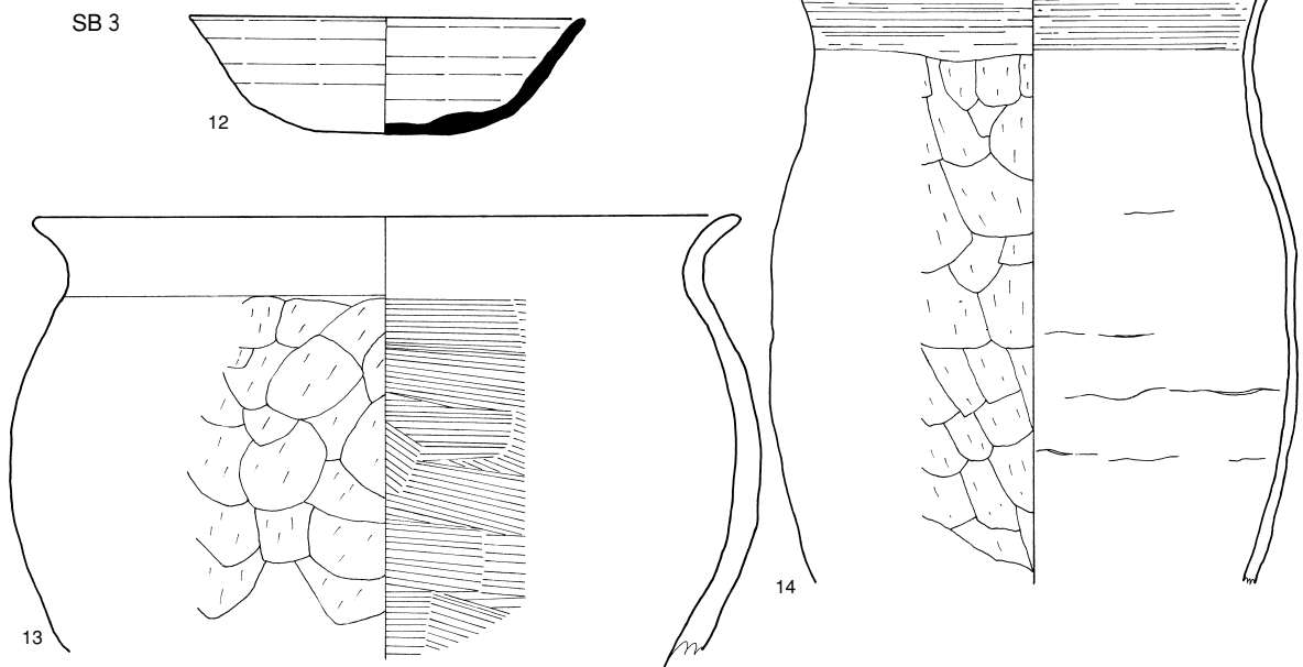
第22図 SB 2・SB 3 出土遺物実測図
