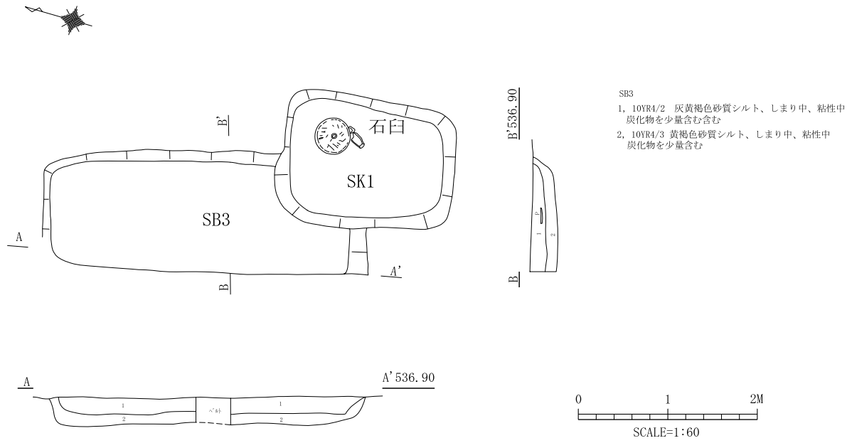
第16図 SB3 実測図
