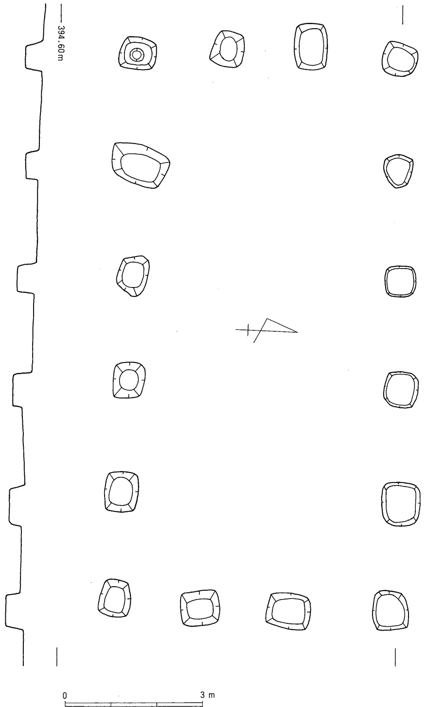
第25図 3号掘立柱建物跡
