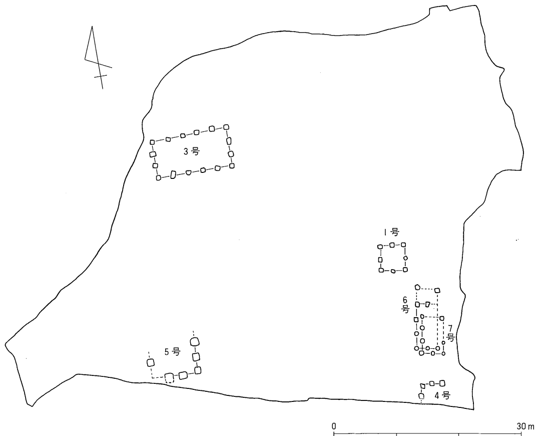
第32図 掘立柱建物跡配置図
