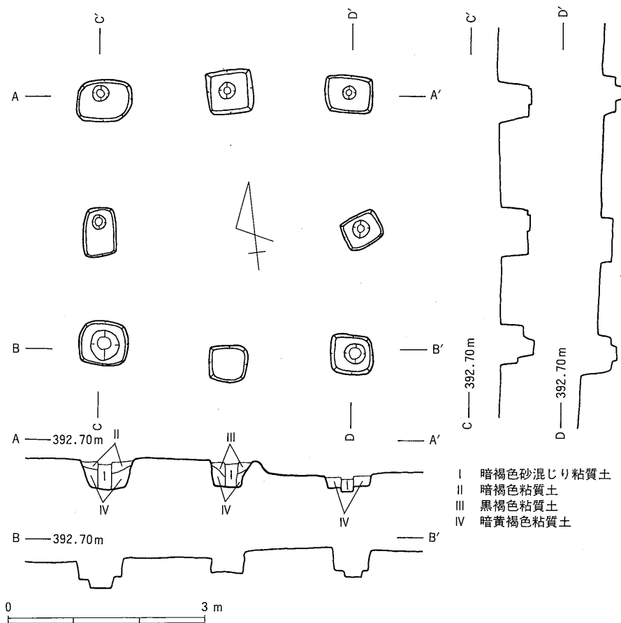
第24図 1号掘立柱建物跡
