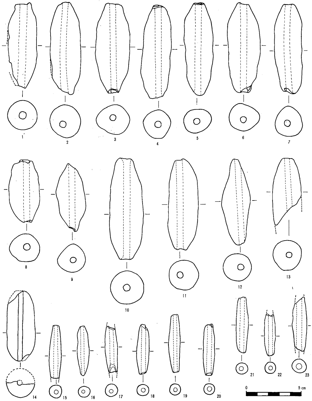
図290 十二ノ后遺跡出土土錘(その1)実測図
