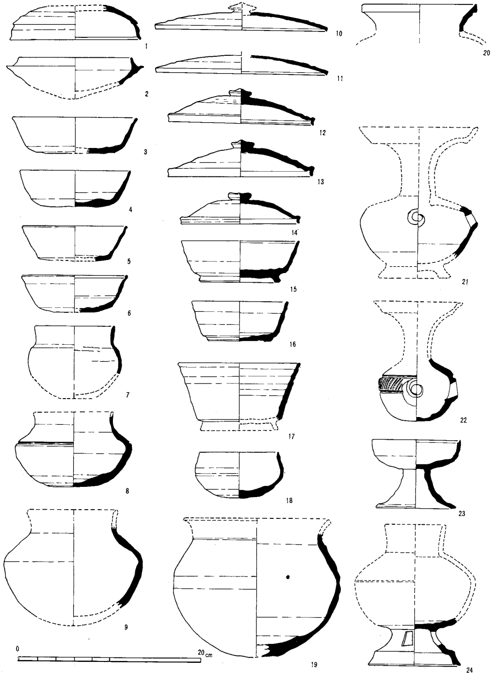
図207 十二ノ后遺跡3号フンド出土土器実測図
