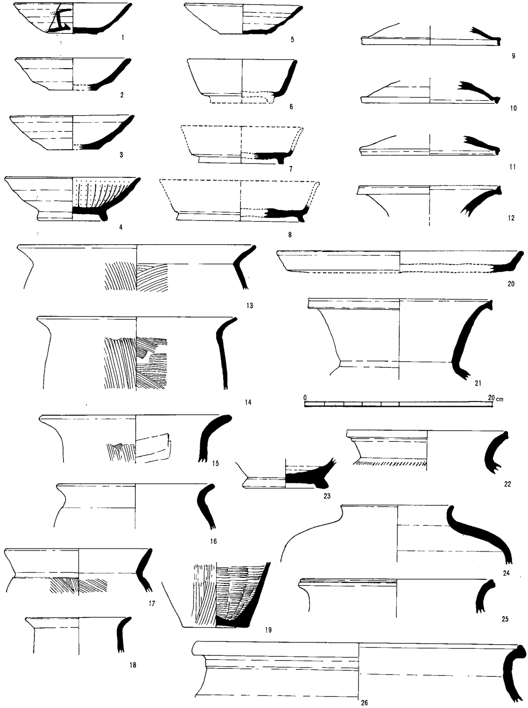
图194 十二ノ后遺跡2号住居址出土土器実測図
