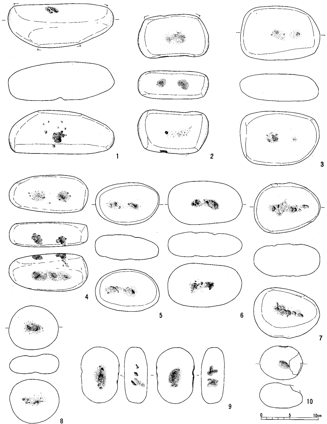
図276 十二ノ后遺跡出土凹石(その2)実測図
