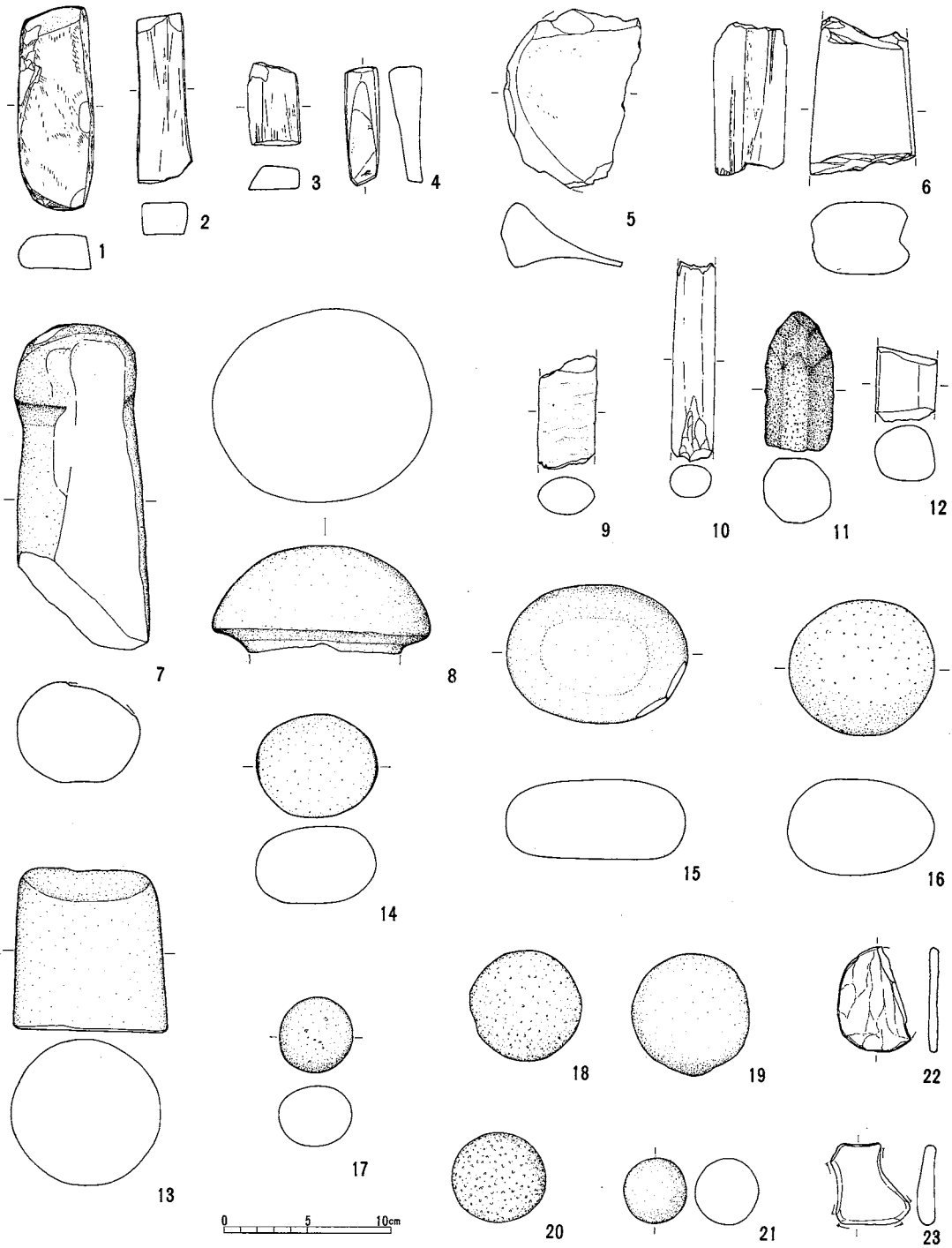
图273 十二ノ后遺跡出土磨石実測図
