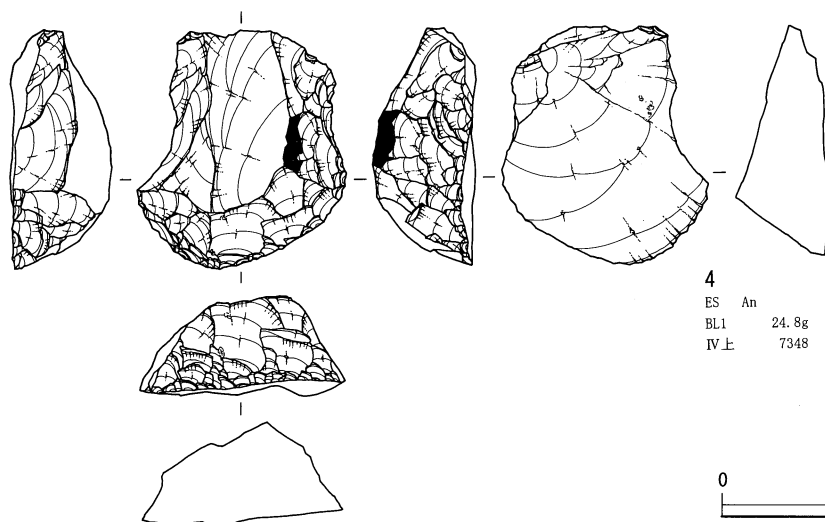
日向林III石器文化 石器実測図 1
