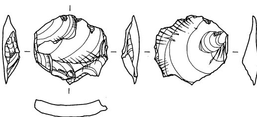
日向林 I 石器文化 石器実測図66 (貝殻状刃器14)
