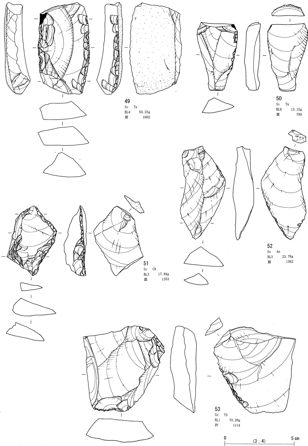
大平I 石器文化 石器実測図9
