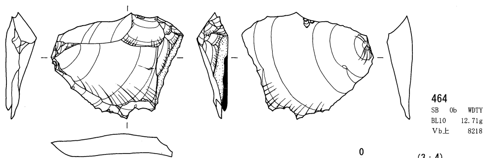
日向林 I 石器文化 石器実測図71 (貝殻状刃器19)
