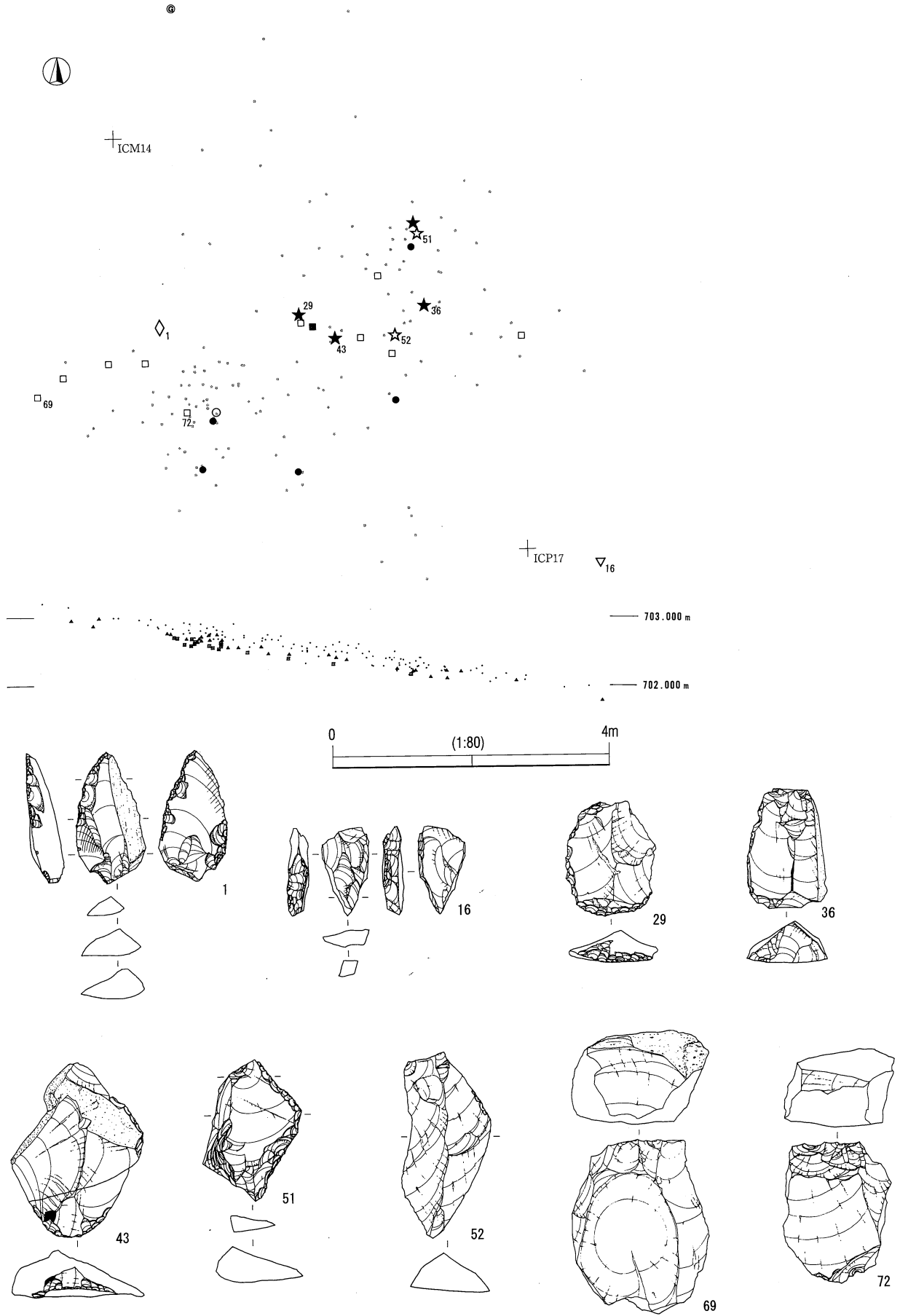
大平 I 石器文化 BL3遺物分布図
