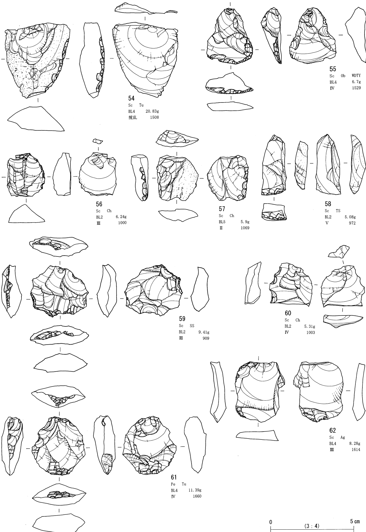
大平 I 石器文化 石器実測図10
