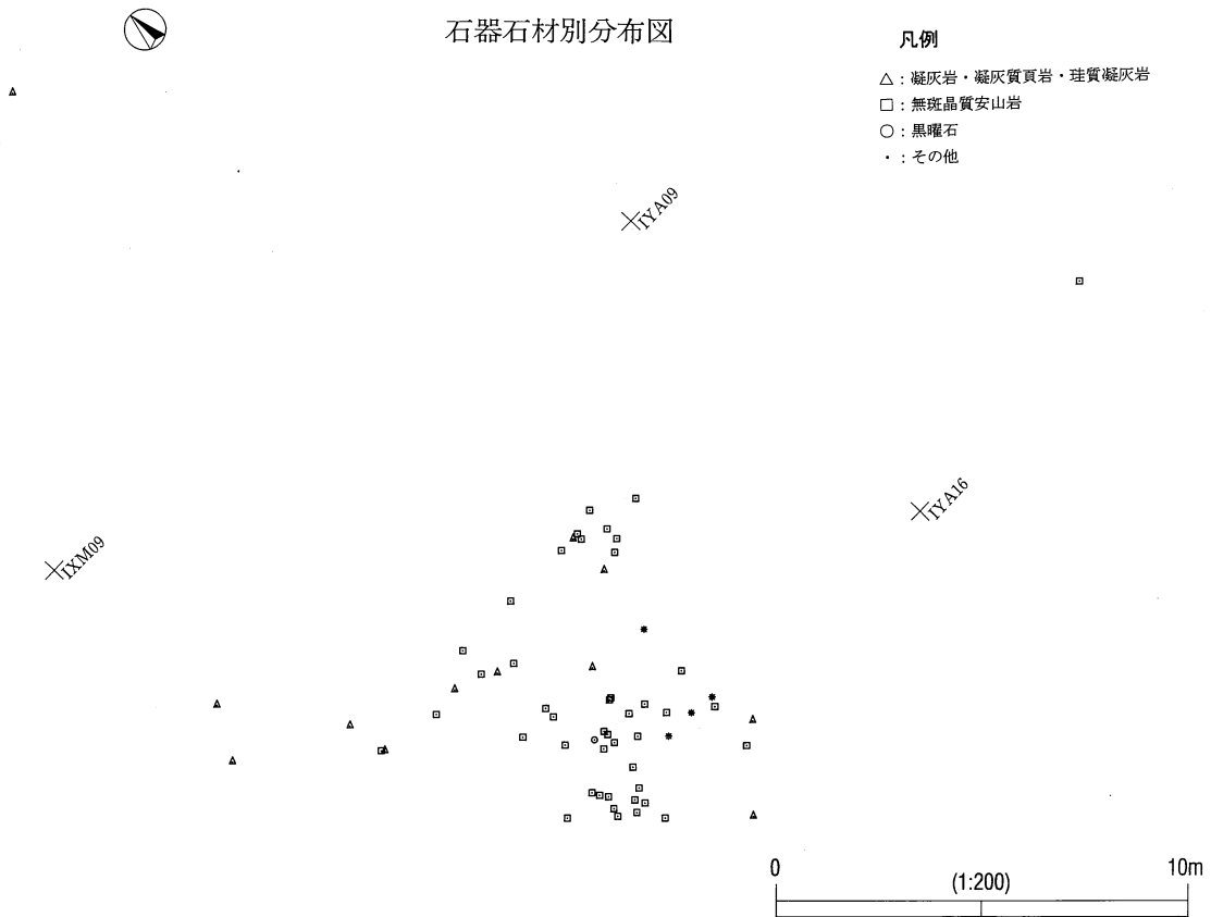
日向林III石器文化 全体図
