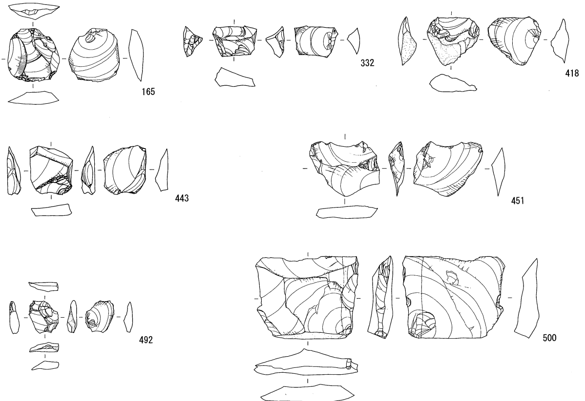
日向林I石器文化 ブロック外遺物分布図
