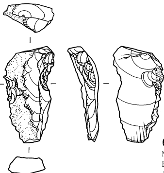
日向林 I 石器文化 石器実測図90 (削器 6・挟入削器 1)
