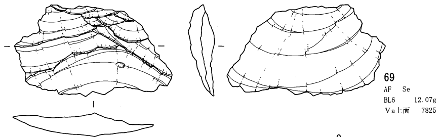
日向林 I 石器文化 石器実測図24 (斧形石器刃部破片 2・斧形石器製作剥片 1)
