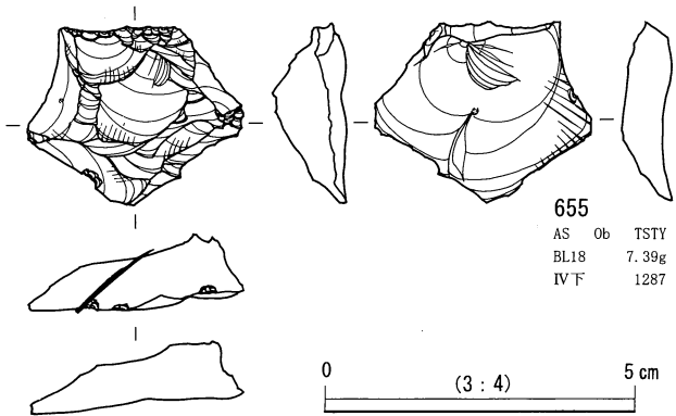
日向林 I 石器文化 石器実測図97 (厚刃搔器 1)
