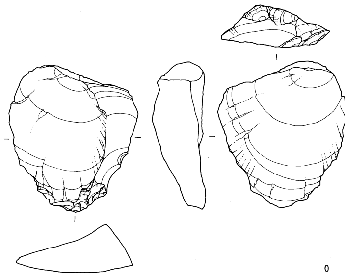
七ツ栗 I 石器文化 石器実測図 4
