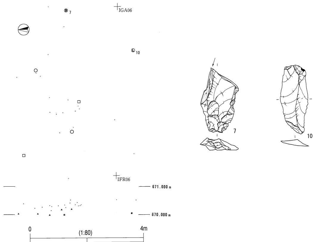
日向林IV石器文化 BL3・BL4遺物分布図 (上:BL3・下:BL4)
