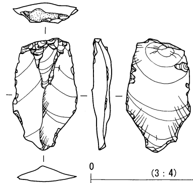
日向林I石器文化 石器実測図104 (微細剝離のある剥片2)
