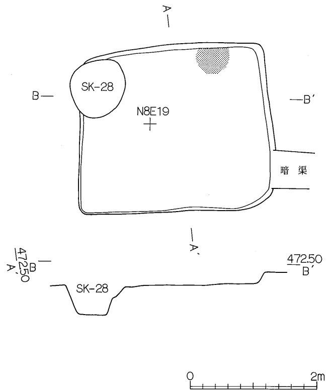
第9图 第4号住居址实测图
