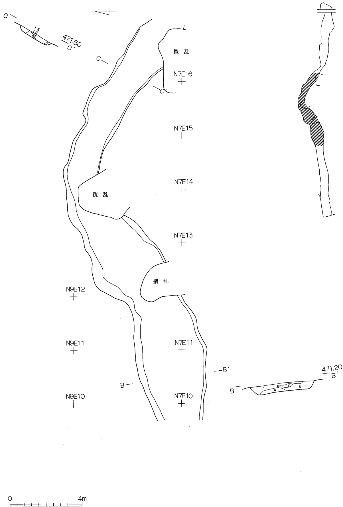
第60图 第1号沟址实测图(2)
