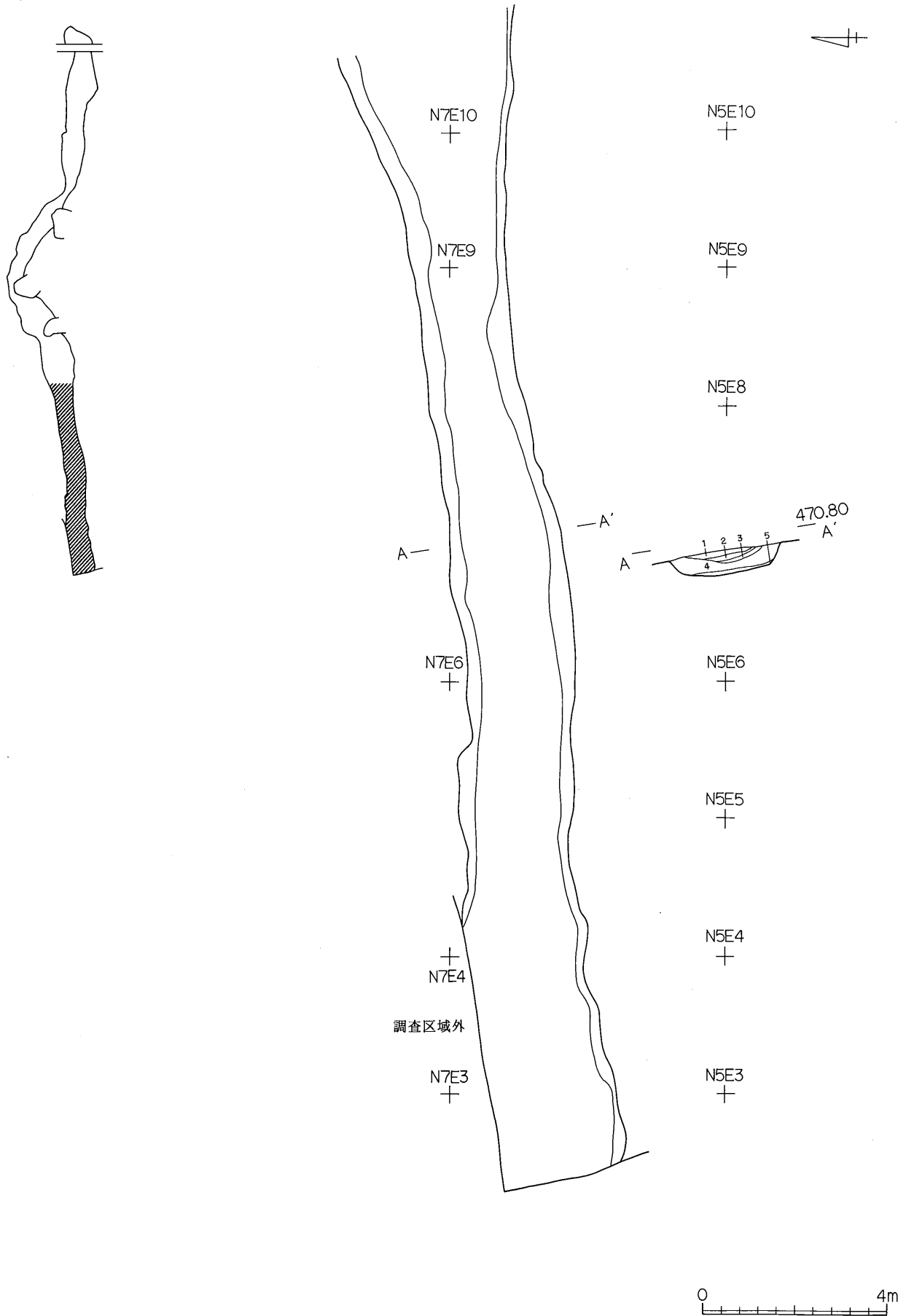
第61図 第1号溝址実測図(3)
