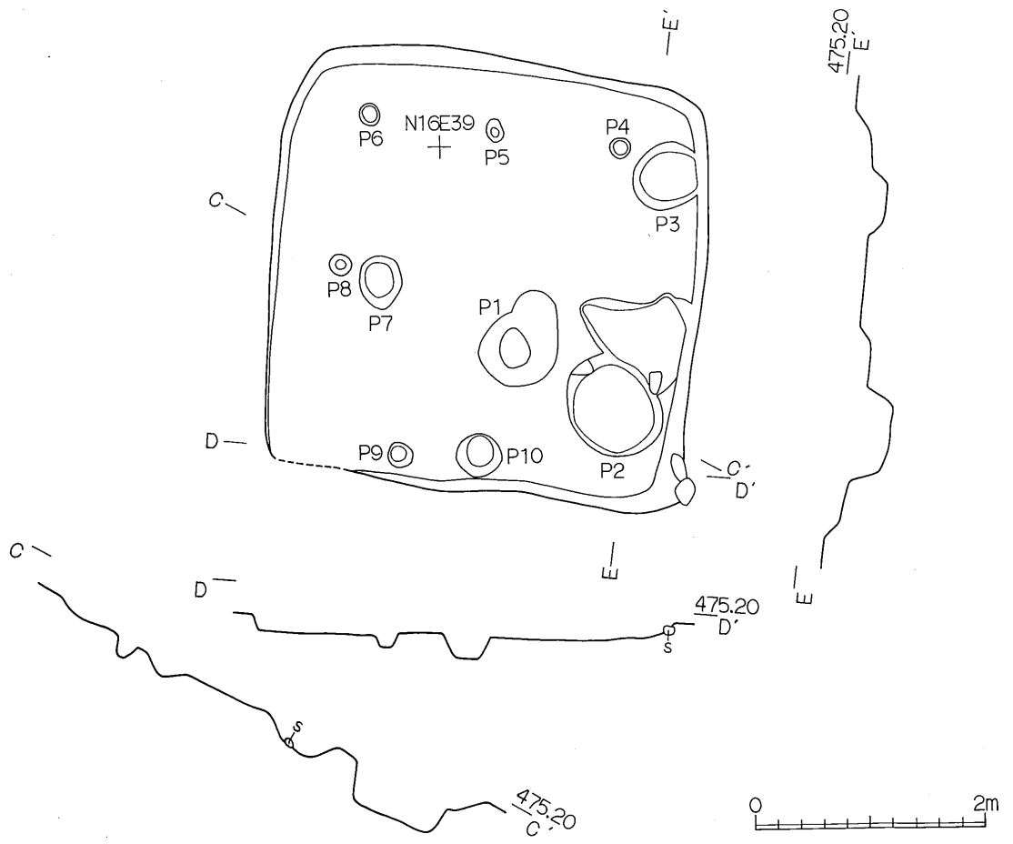
第21图 第13号住居址掘り方实测图
