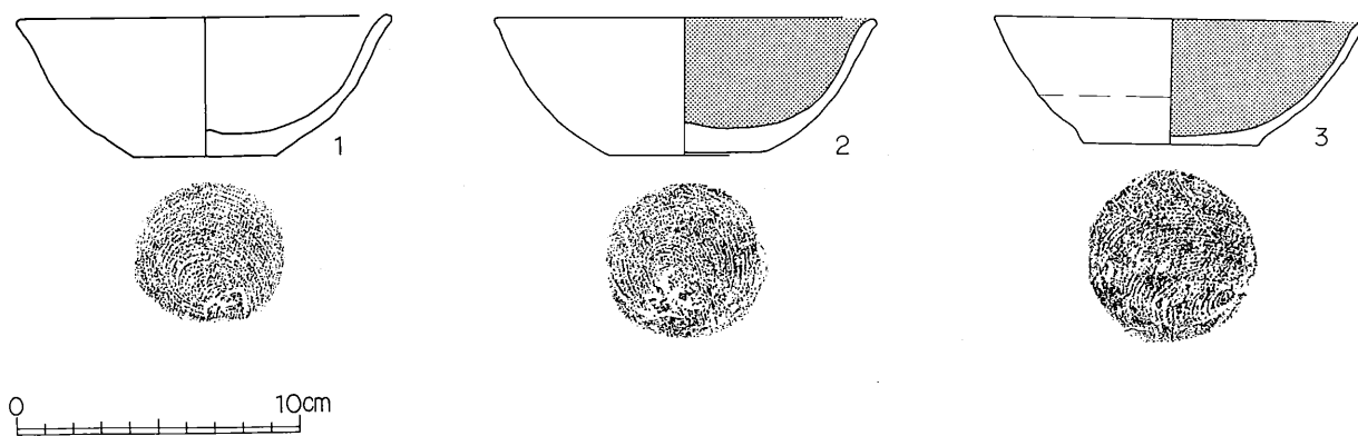
第92图 第22号住居址出土遺物实测图(1)
