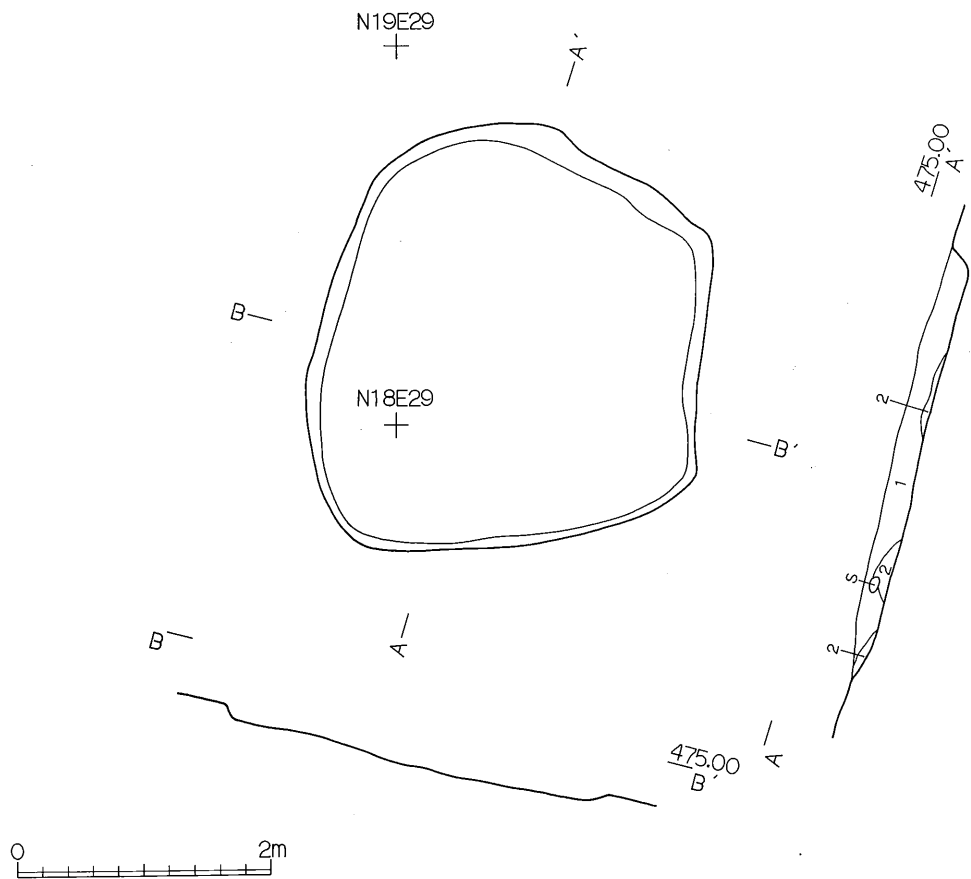
第26图 第17号住居址实测图
