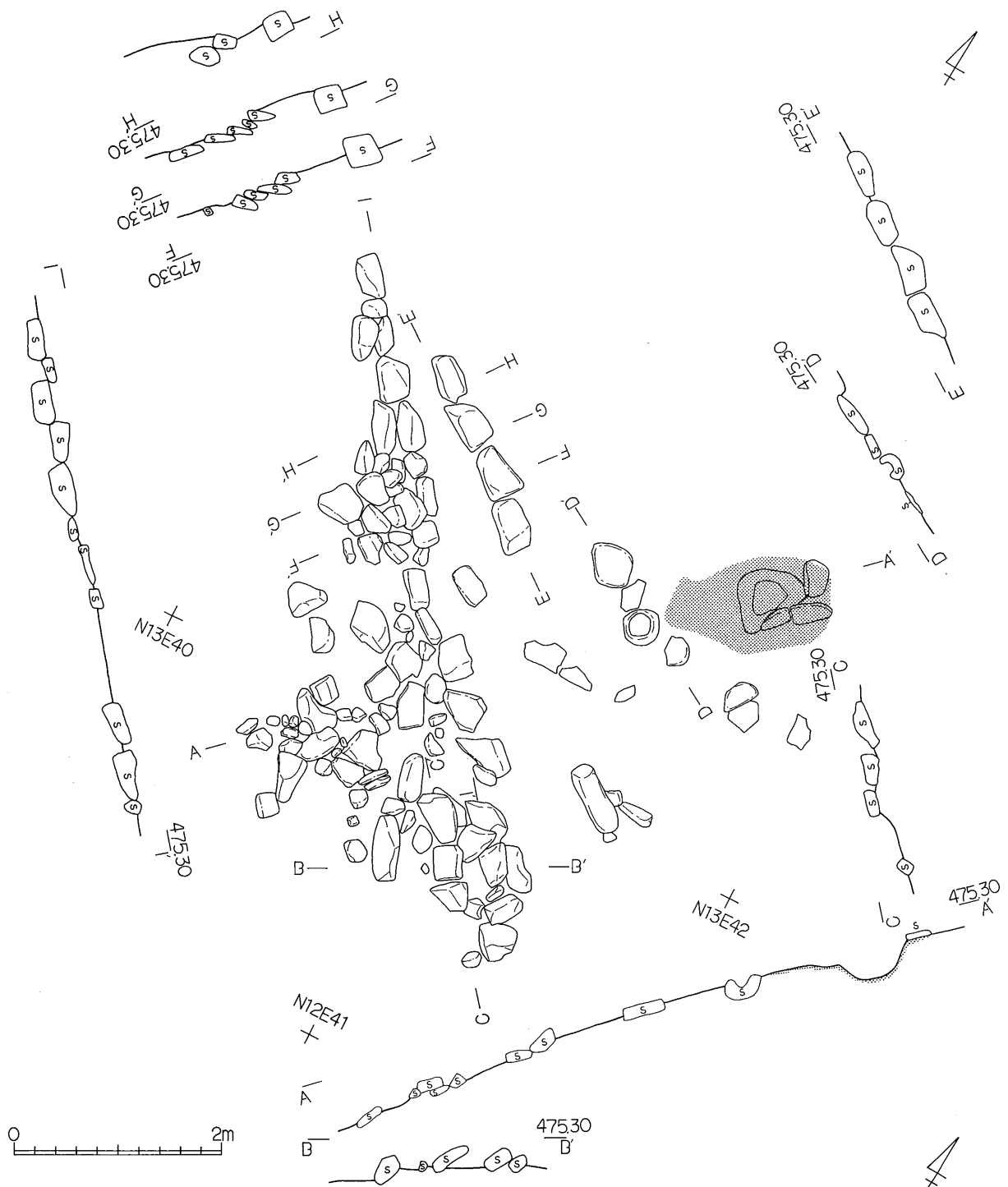
第34图 第24号住居址实测图
