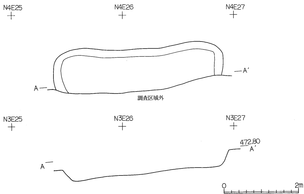
第6图 第2号住居址实测图
