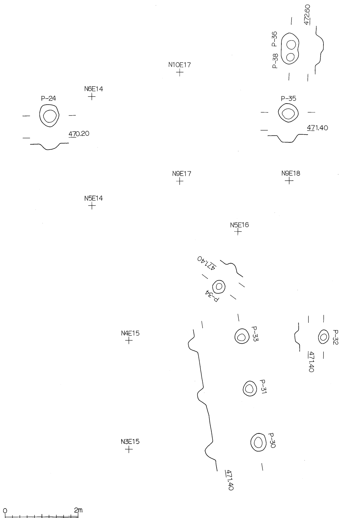
第64図 ピット実測図(3)
