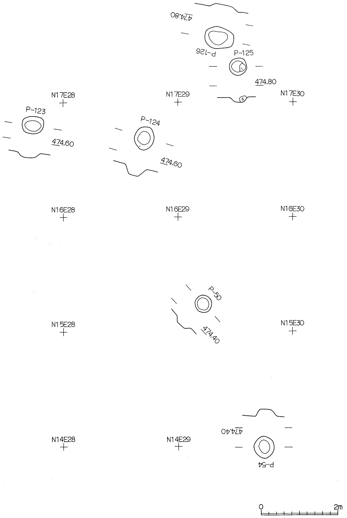
第67図 ピット実測図(6)
