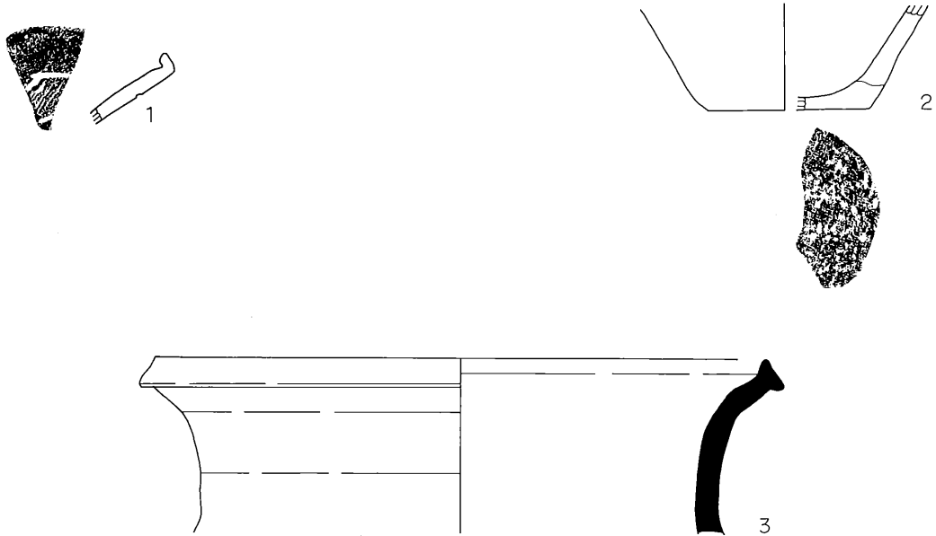
第97图 第3号土壤出土遺物実測図
