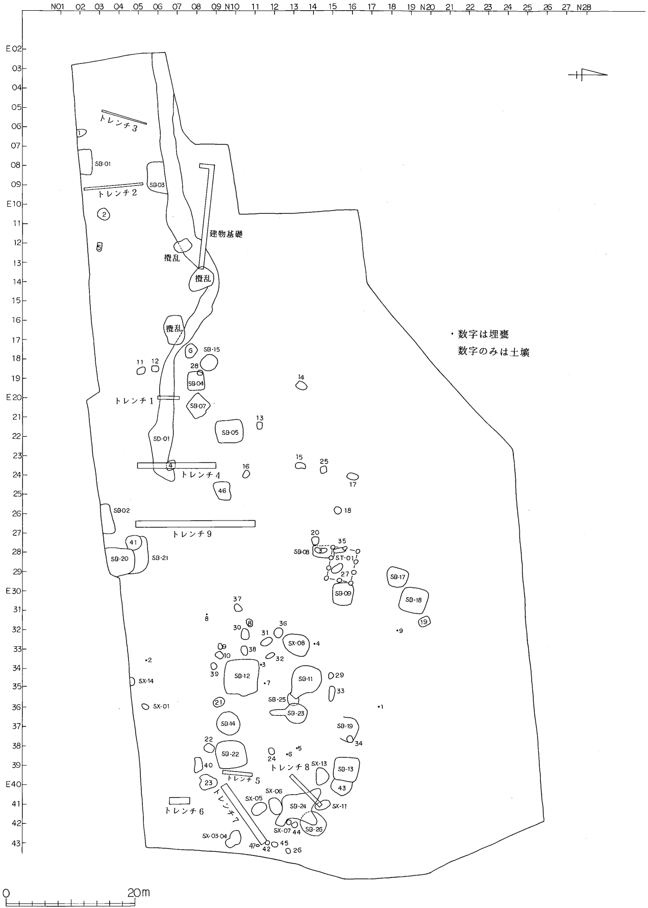
第4図 遺構配置図
