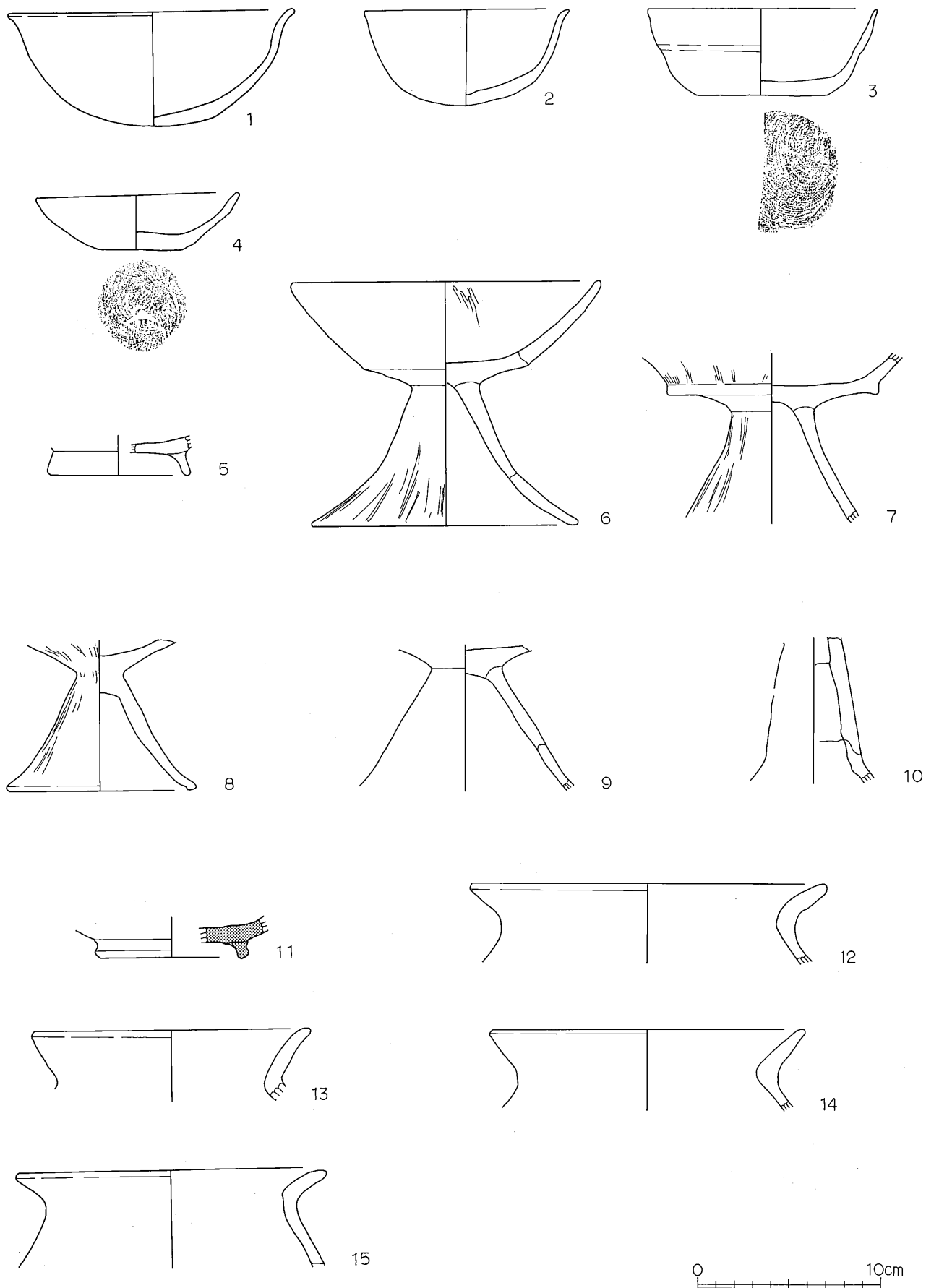
第 139图 第 1 号沟址出土遗物实测图(1)
