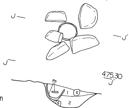
第35图 第24号住居炉址实测图
