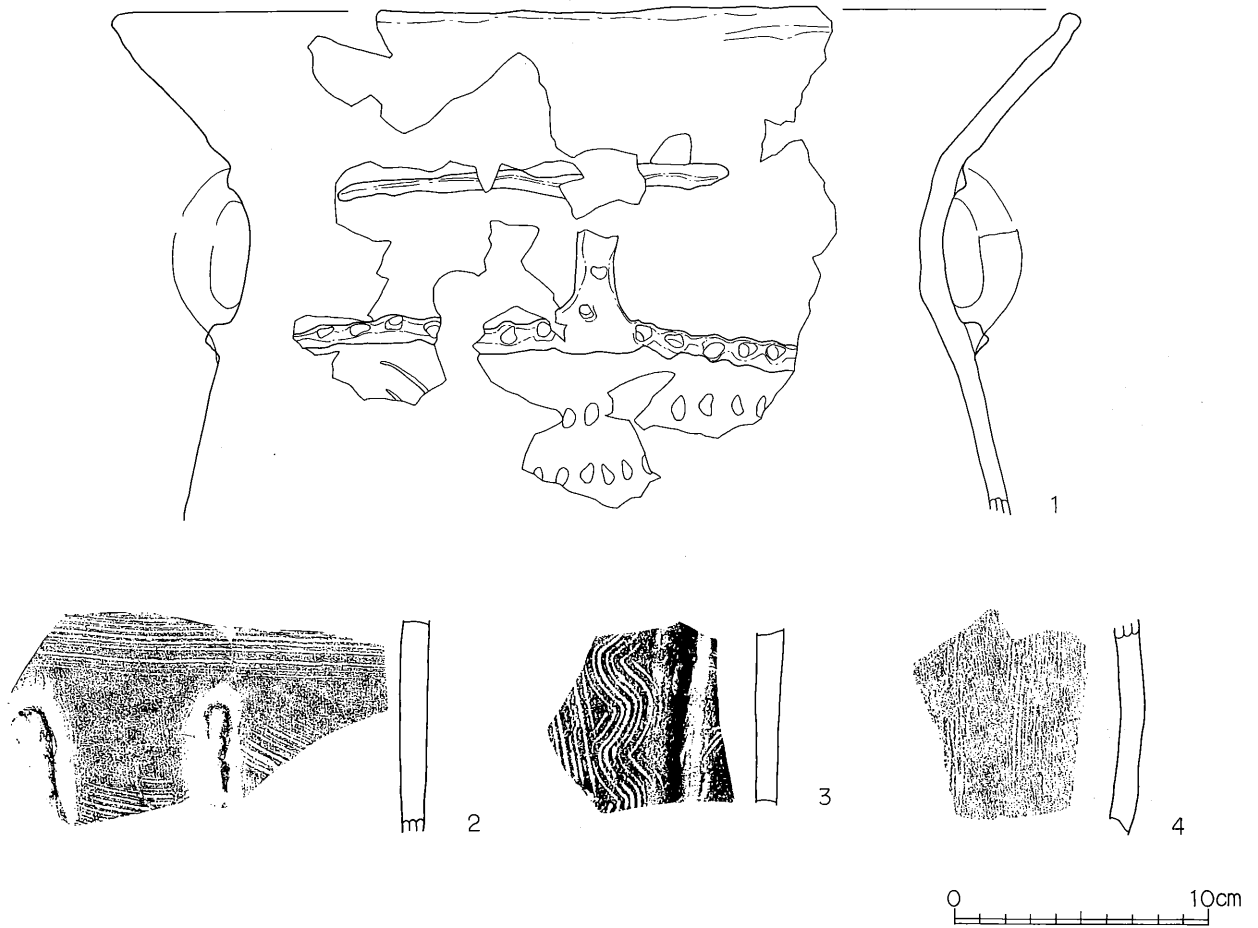
第 137图 第 11 号集石出土遺物実測図(1)
