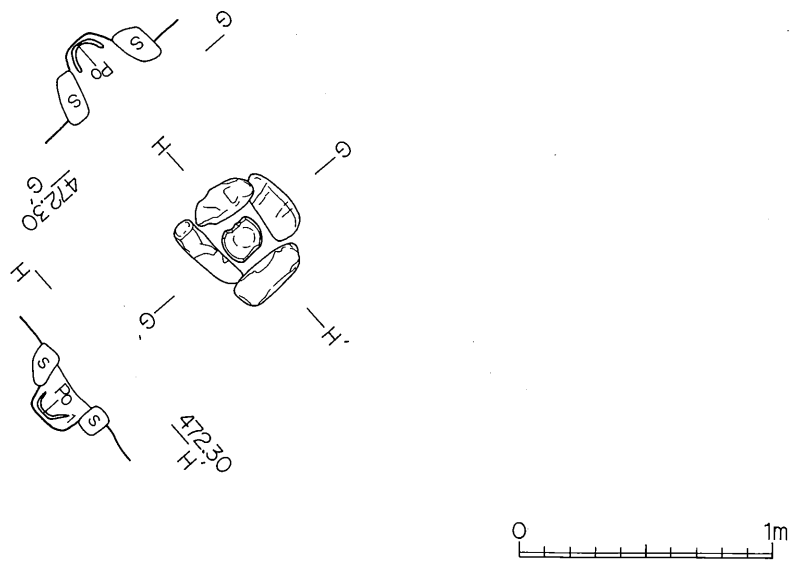
第25图 第15号住居炉址实测图
