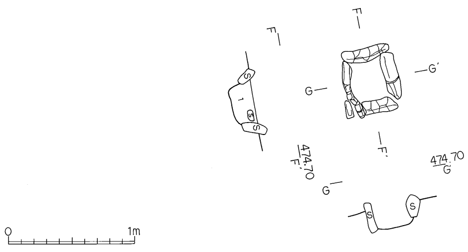
第33图 第23号住居址实测图
