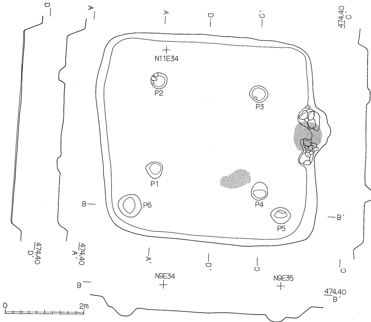
第18图 第12号住居址实测图
