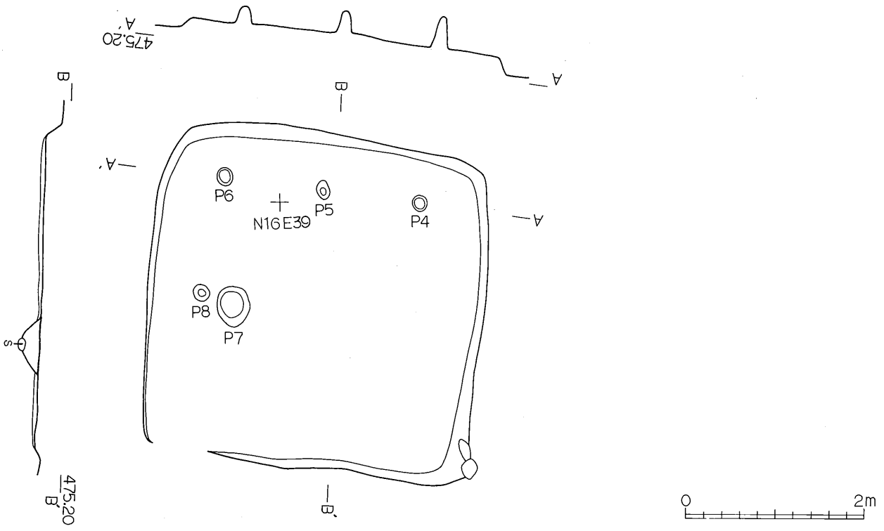
第20图 第13号住居址实测图
