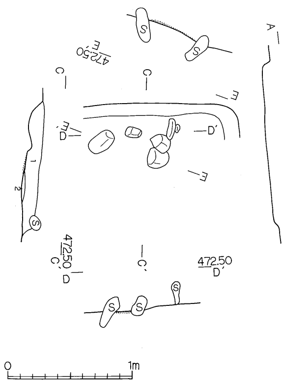
第8图 第4号住居址实测图
