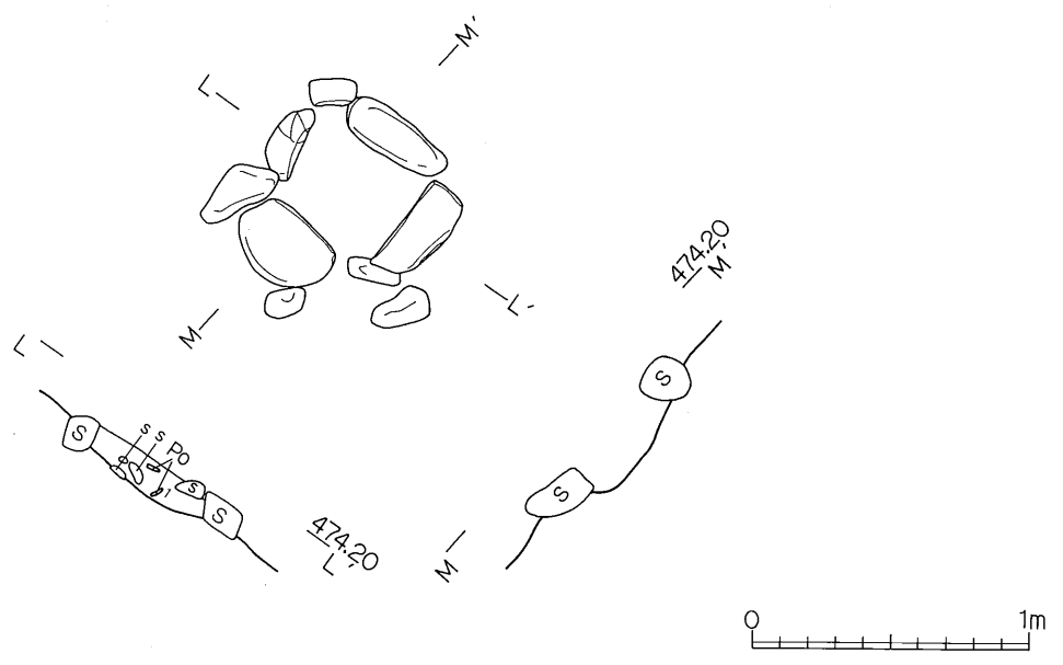
第17図 第11号住居炉址実測図
