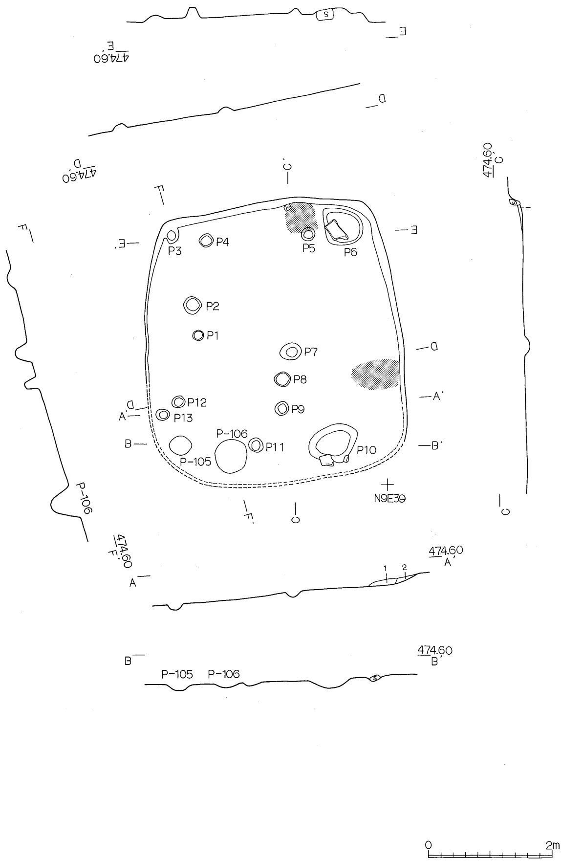
第31图 第22号住居址实测图
