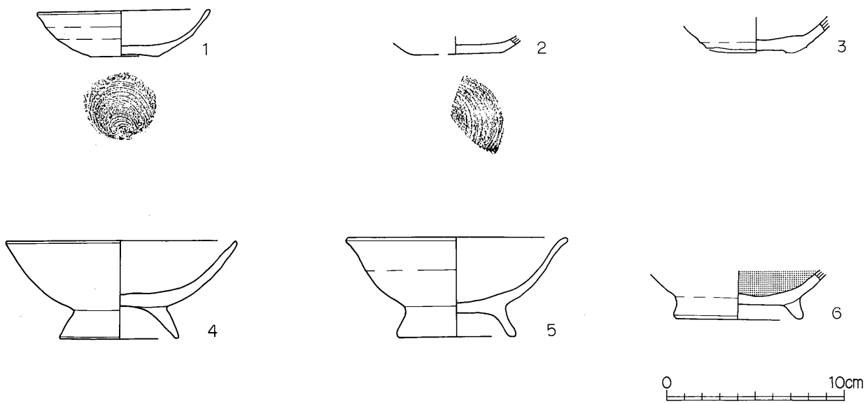
第76图 第3号住居址出土遗物实测图(1)
