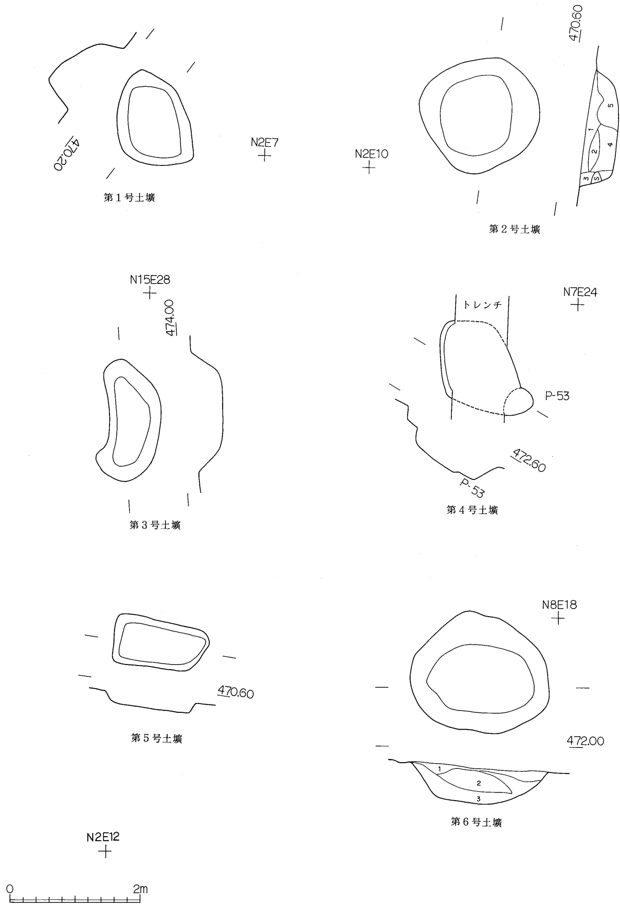
第40図 土壤実測図(1)
