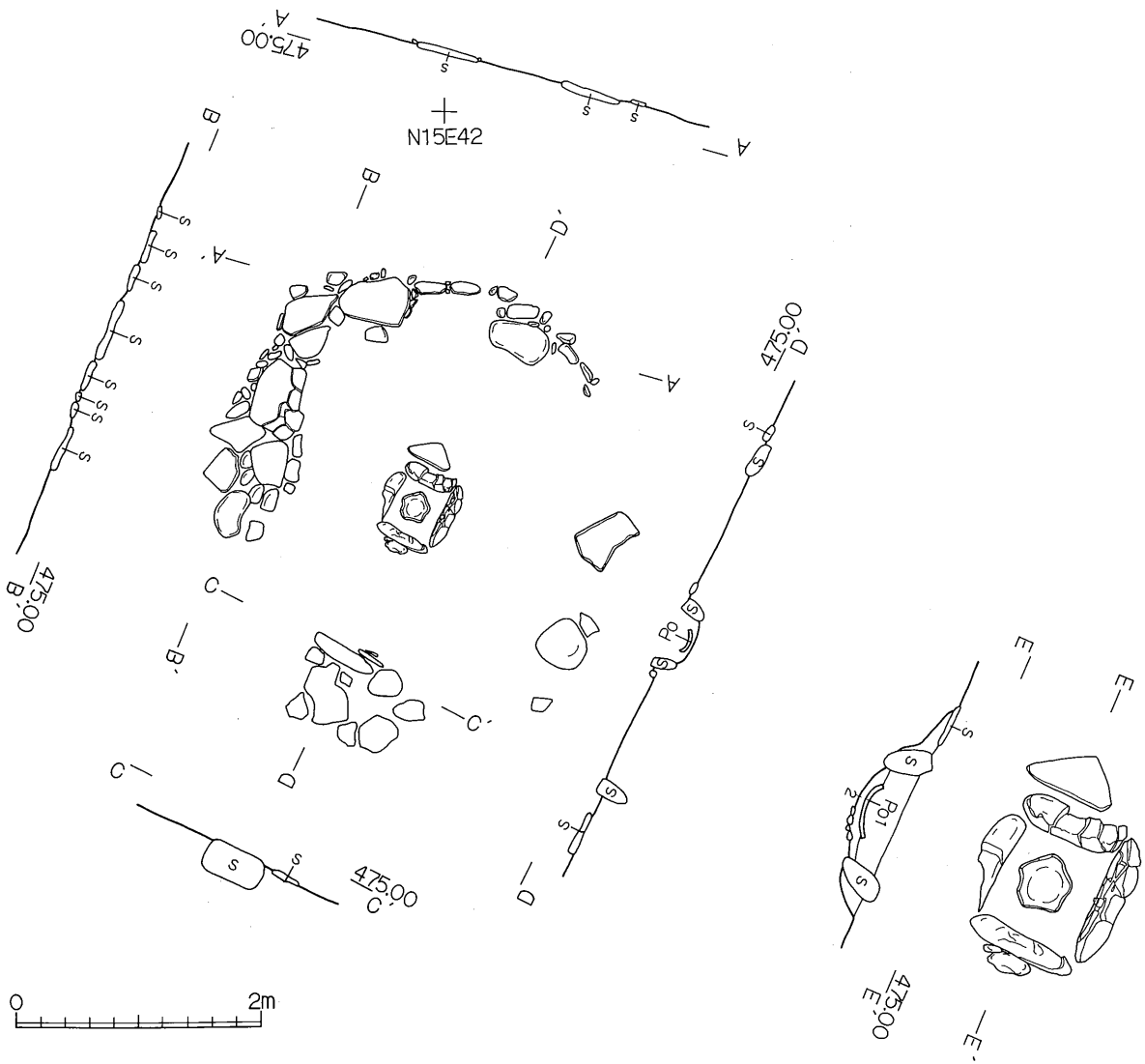
第37图 第26号住居址实测图
