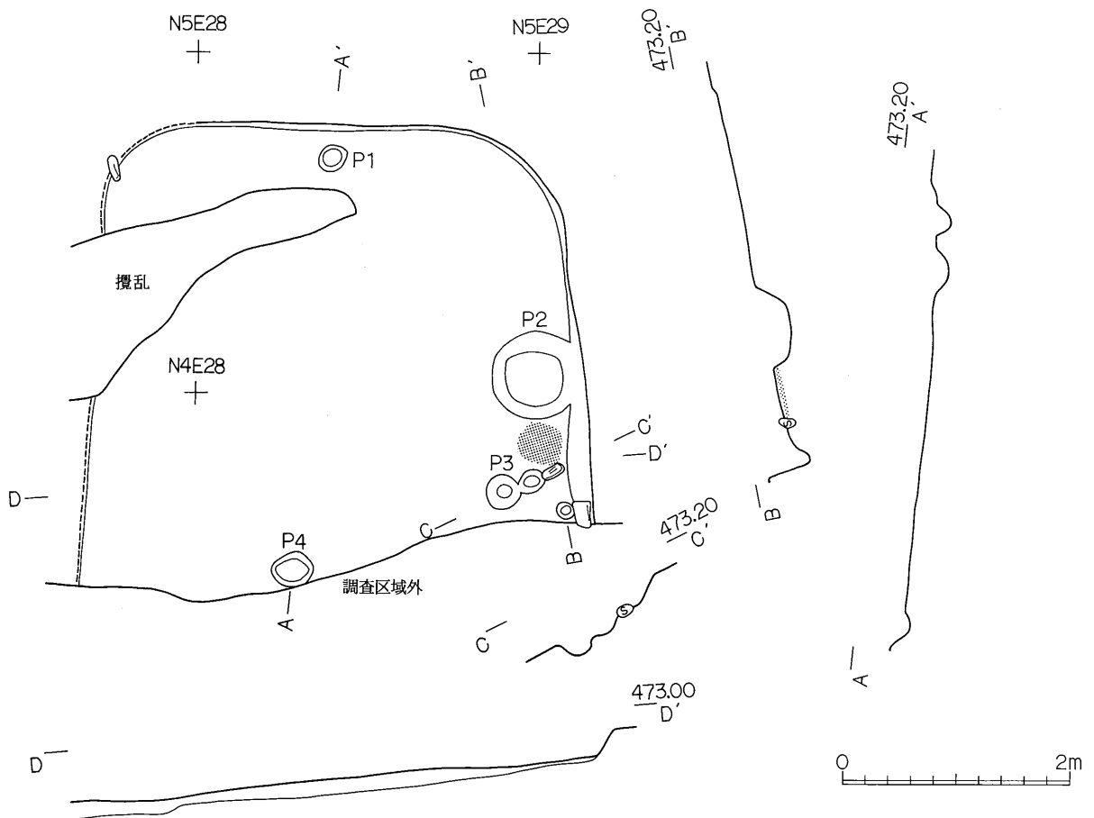
第29图 第20号住居址实测图
