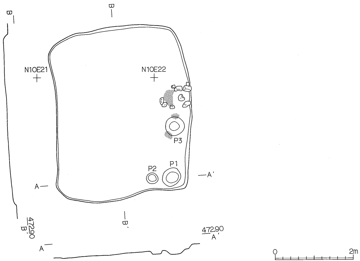
第10图 第5号住居址实测图
