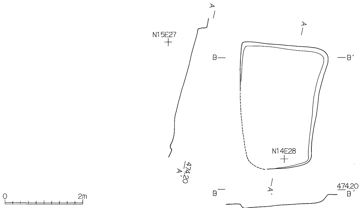
第13图 第8号住居址实测图
