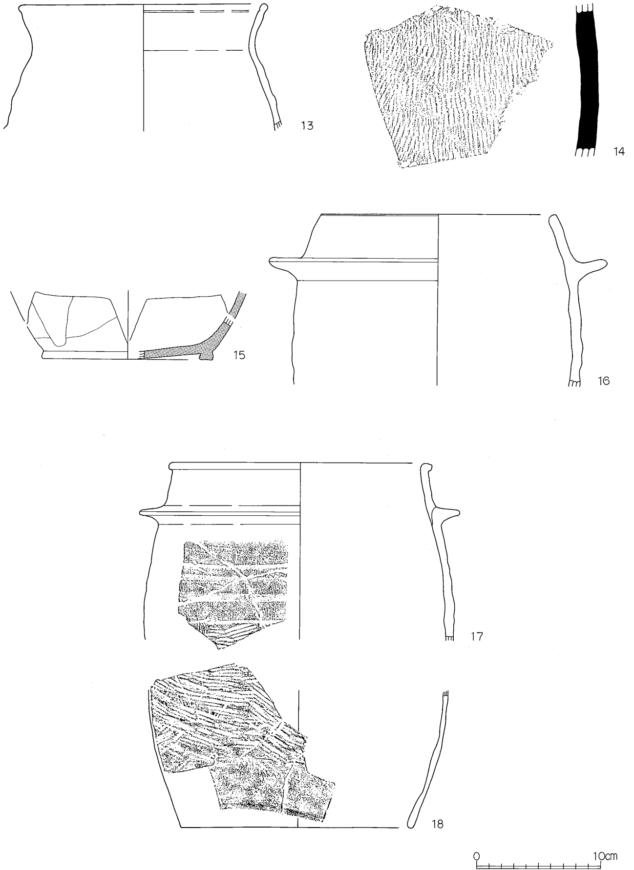
第90图 第20号住居址出土遺物実測図(2)
