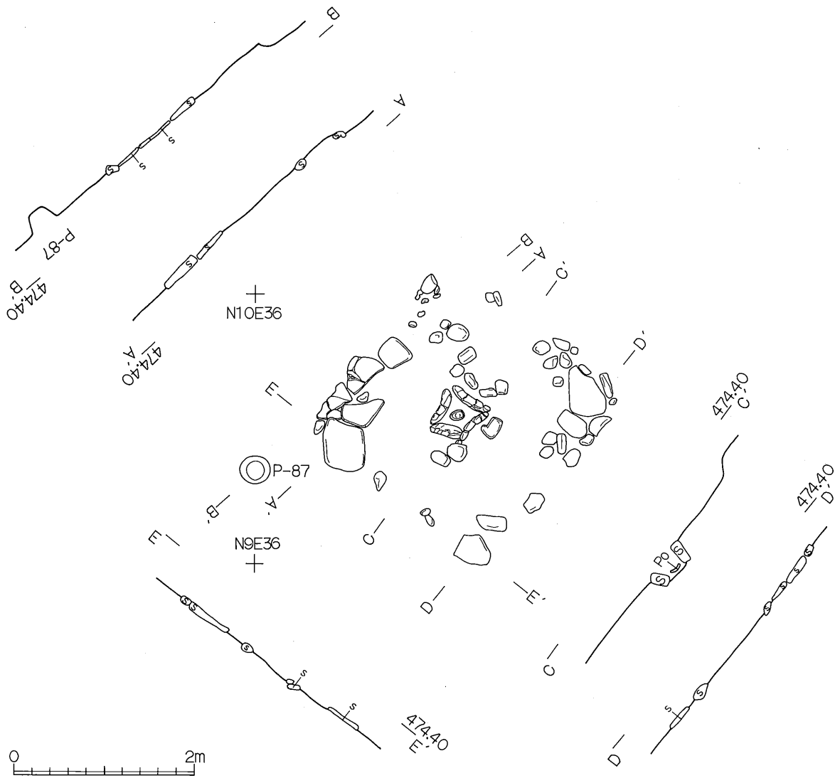
第22图 第14号住居址实测图
