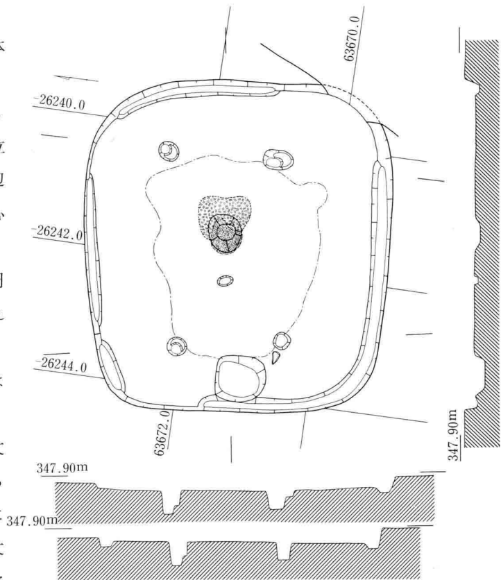
第117図 SA 142 (1 : 80)
