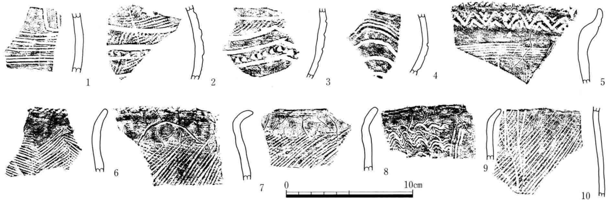
第76図 SA123遺物実測図
