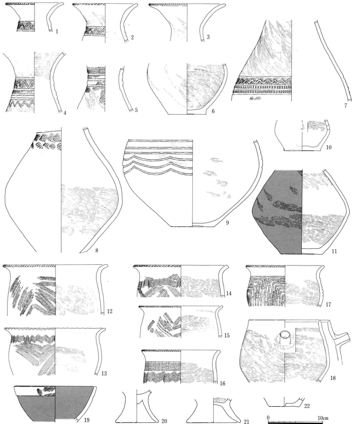
第106図 SA137遺物実測図(1)
