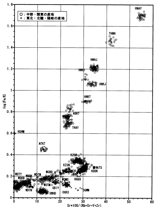
第101図 旧検出器による東日本・隠岐の産地原石判別図
