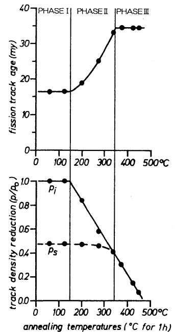
第107図 プラトー法
