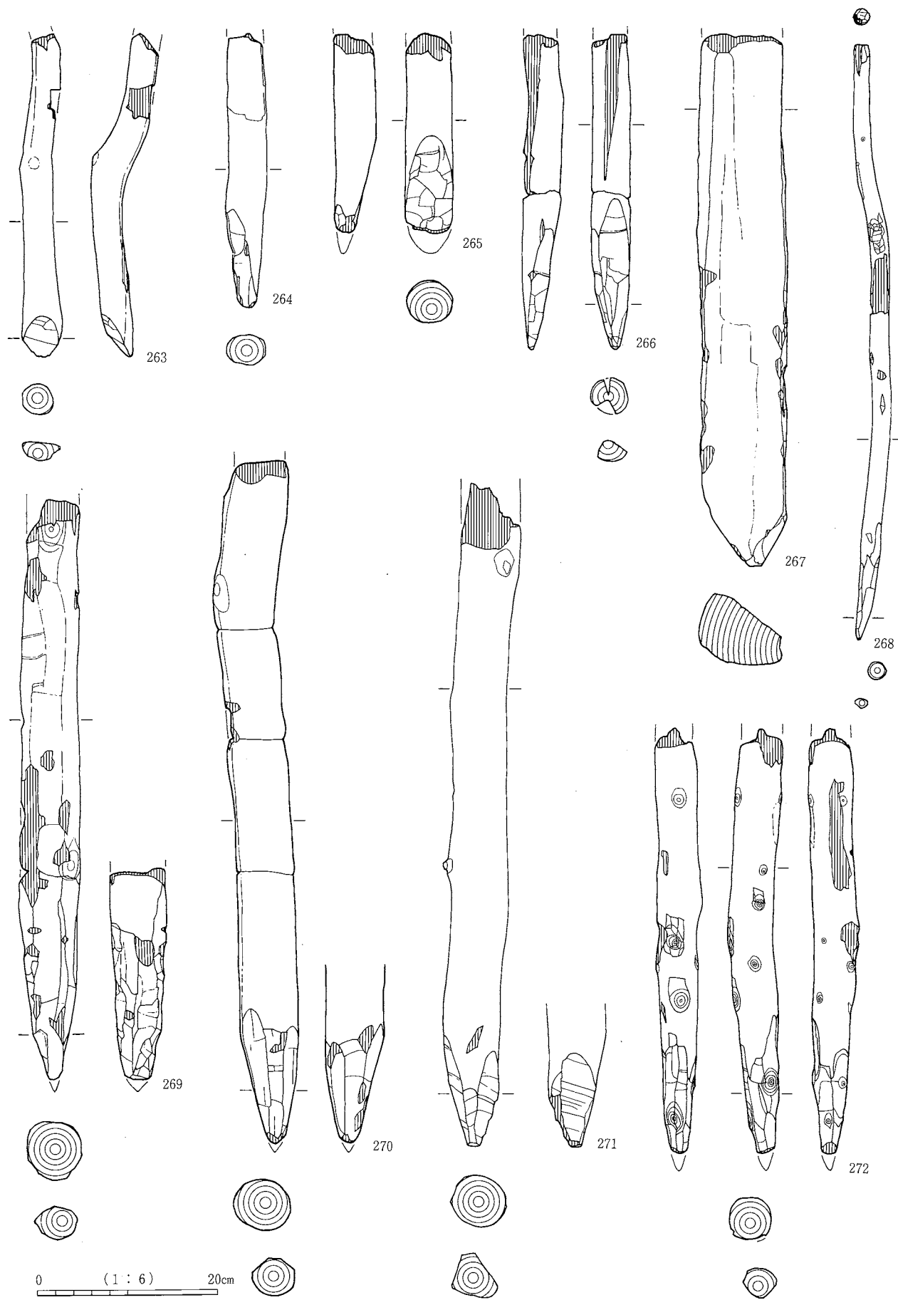
土木1 杭(1)
