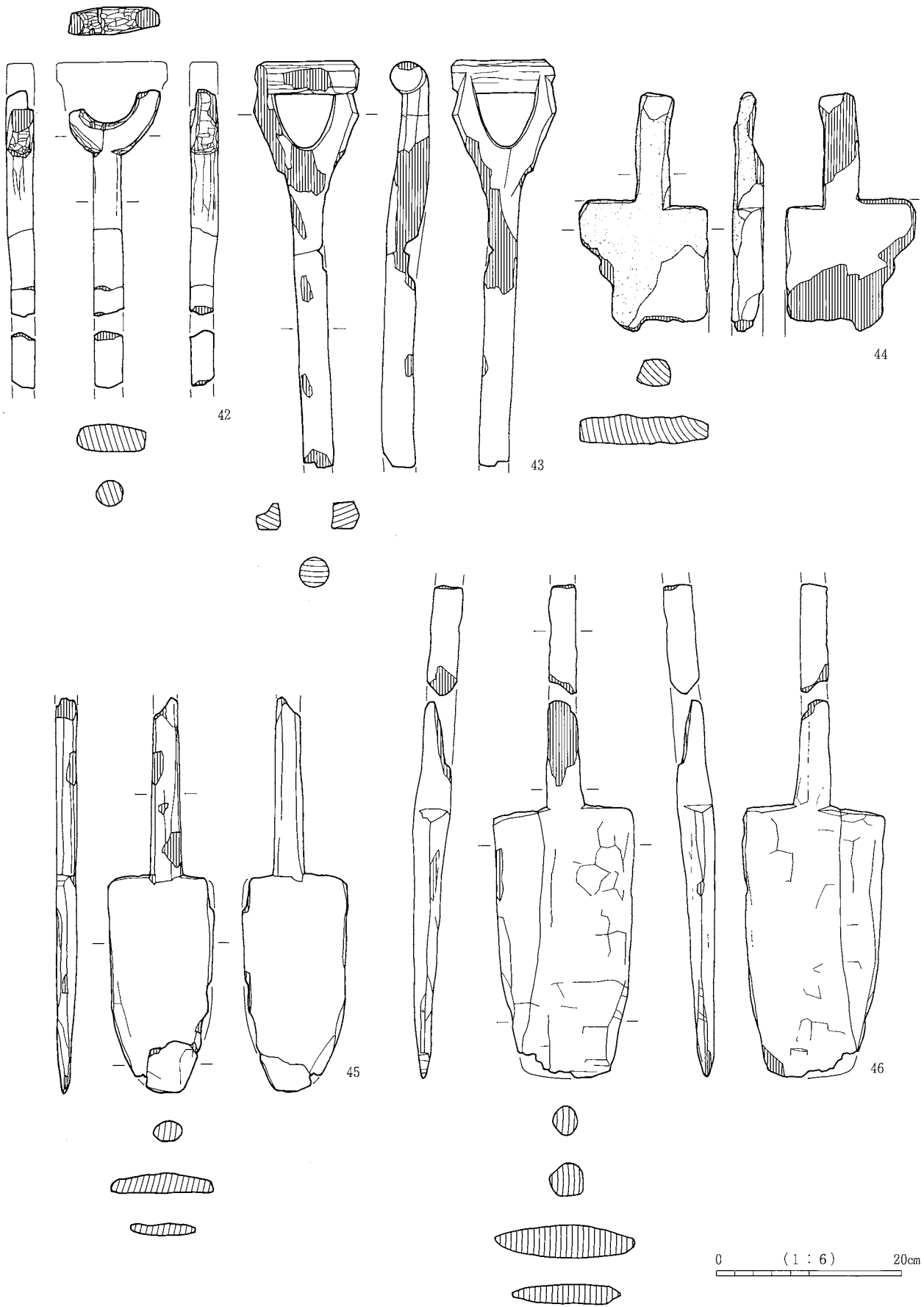
農具8 一木鋤
