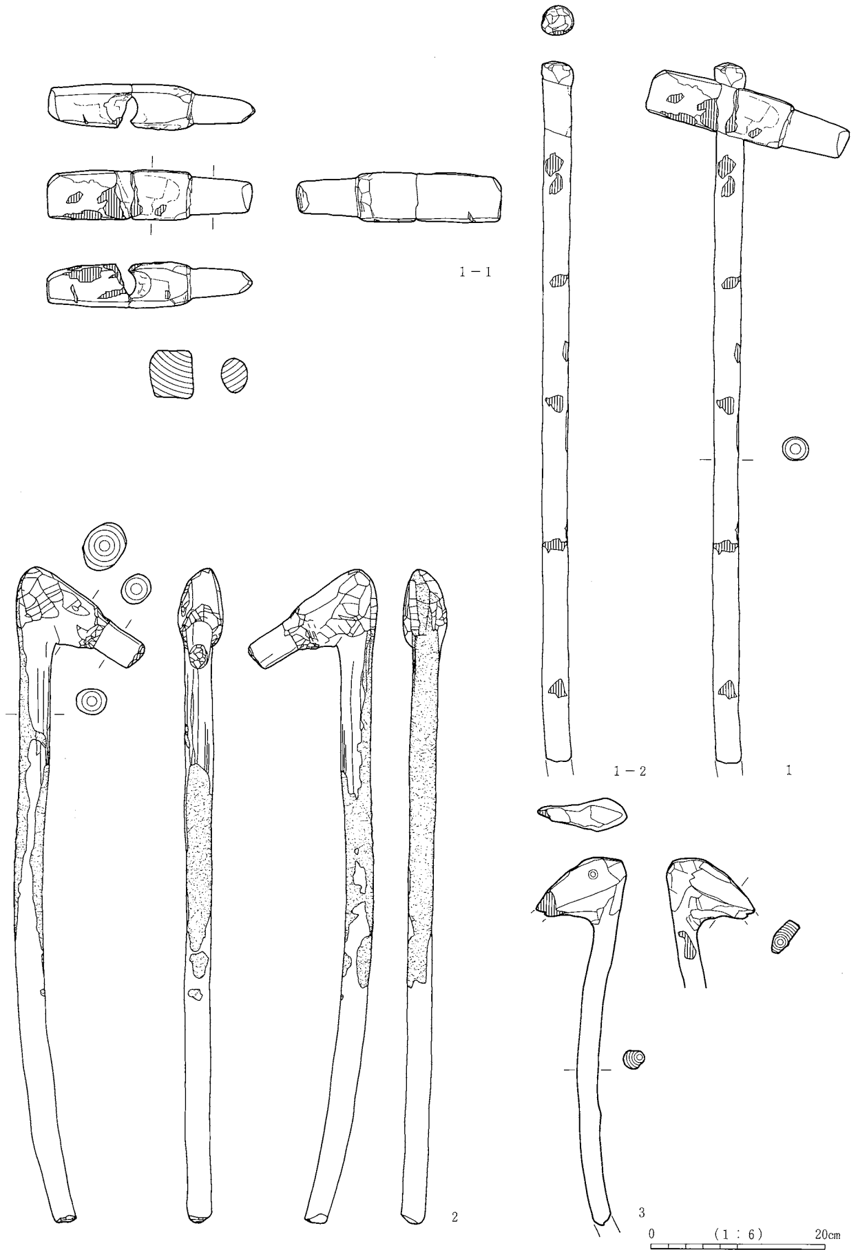
工具1 斧柄(1)
