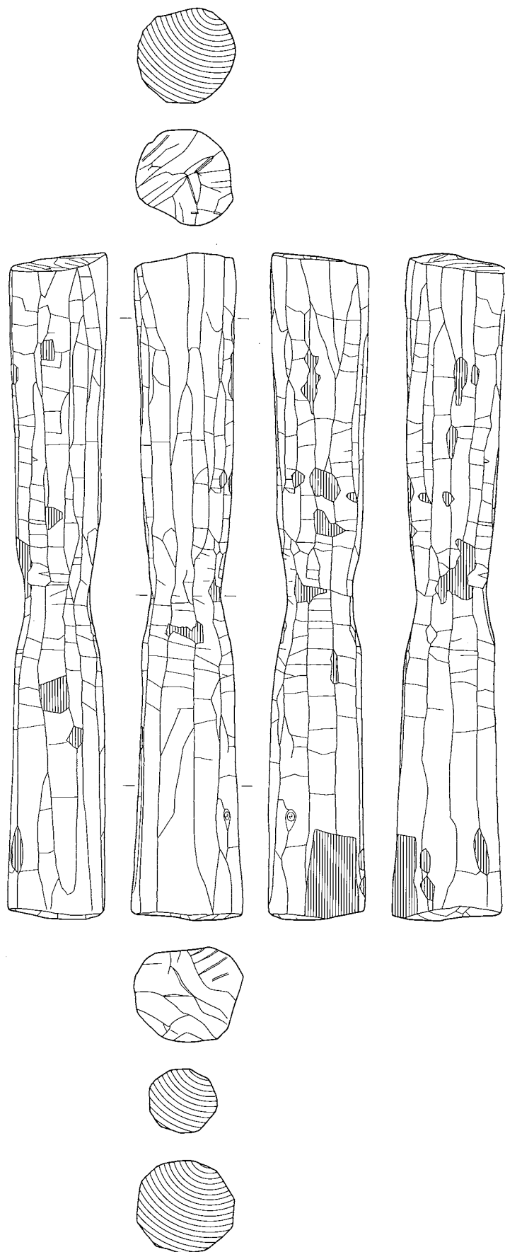
農具12 豎杵(3)
