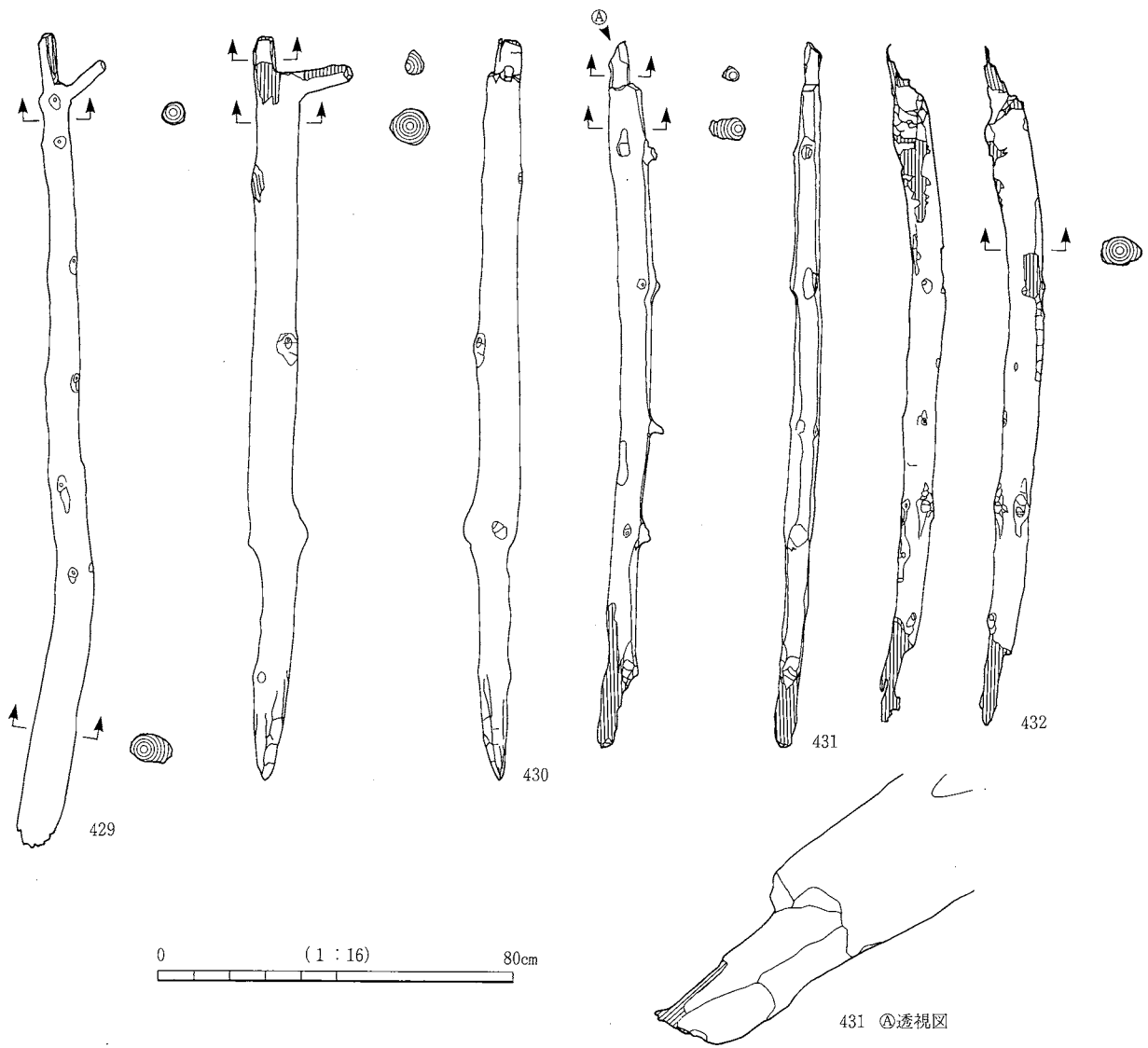
小屋組の形成材 (推定)
