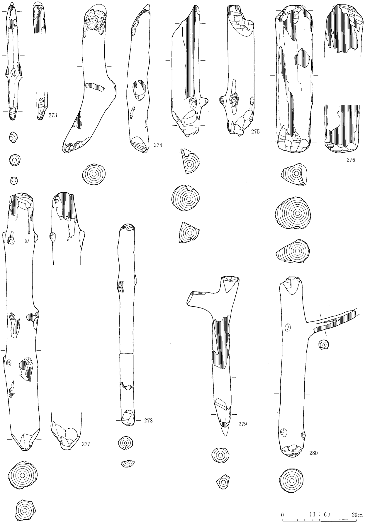
土木2 杭(2)
