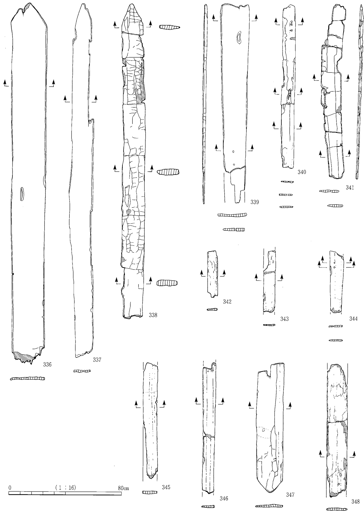
壁板
