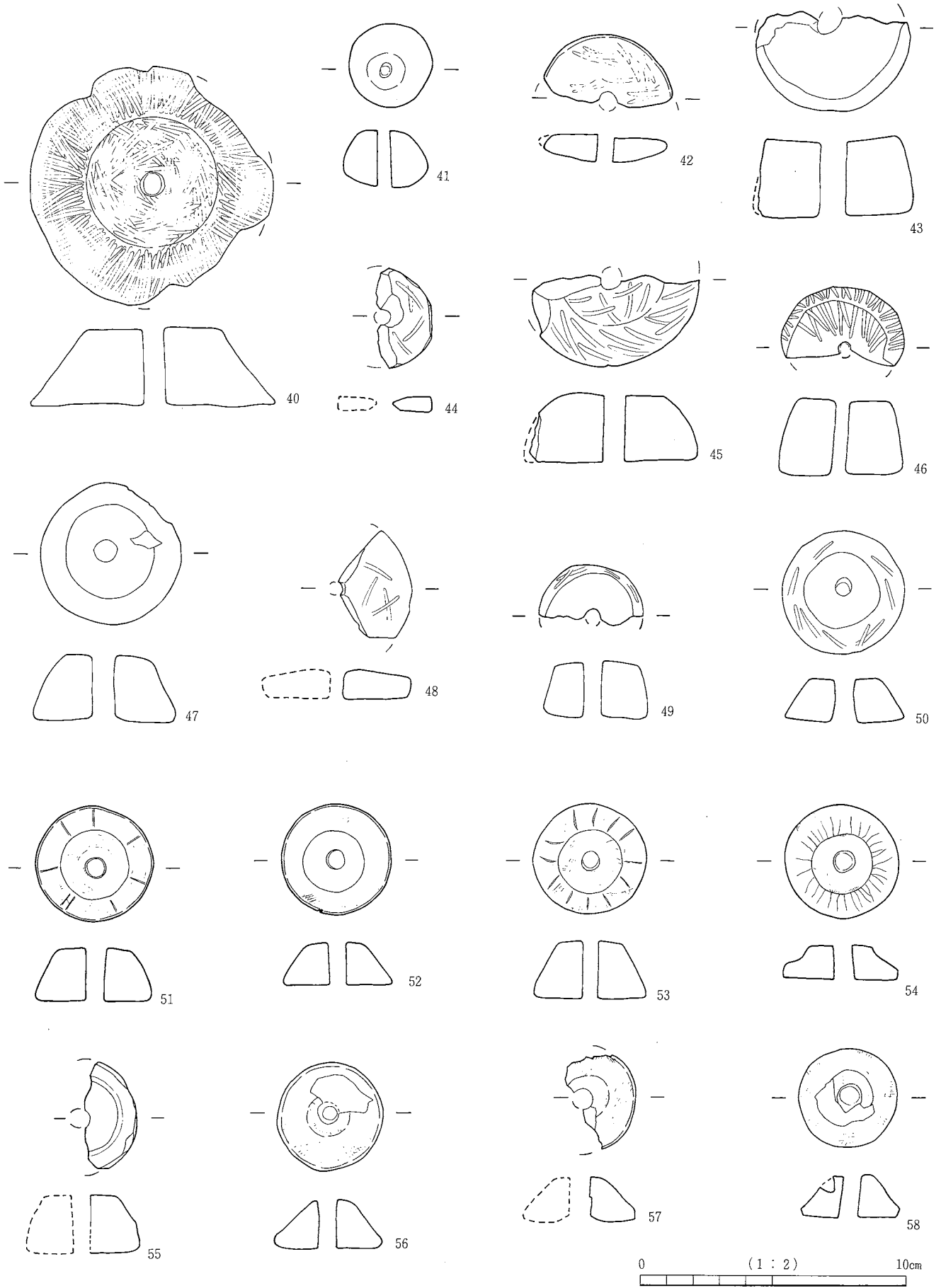
土製紡錘車 (40~50)
