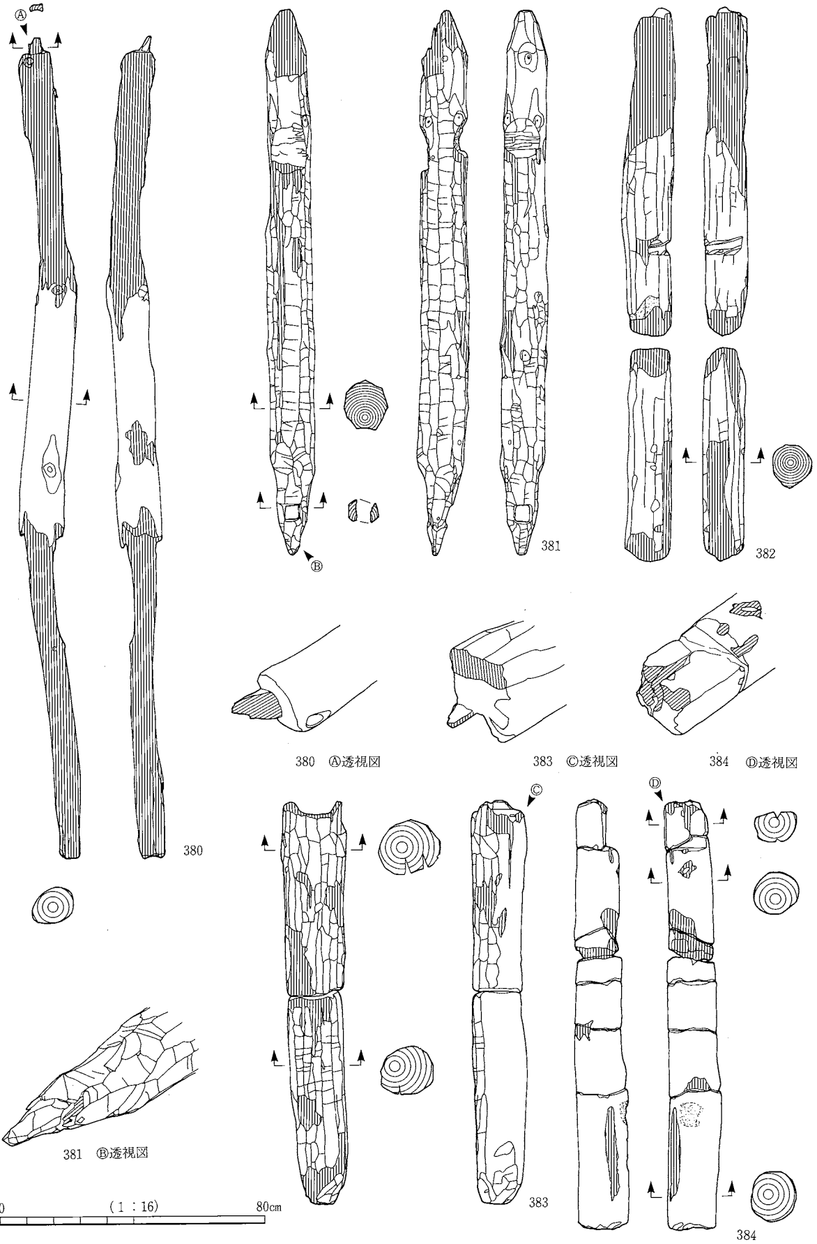
柱2 柄付(2)
