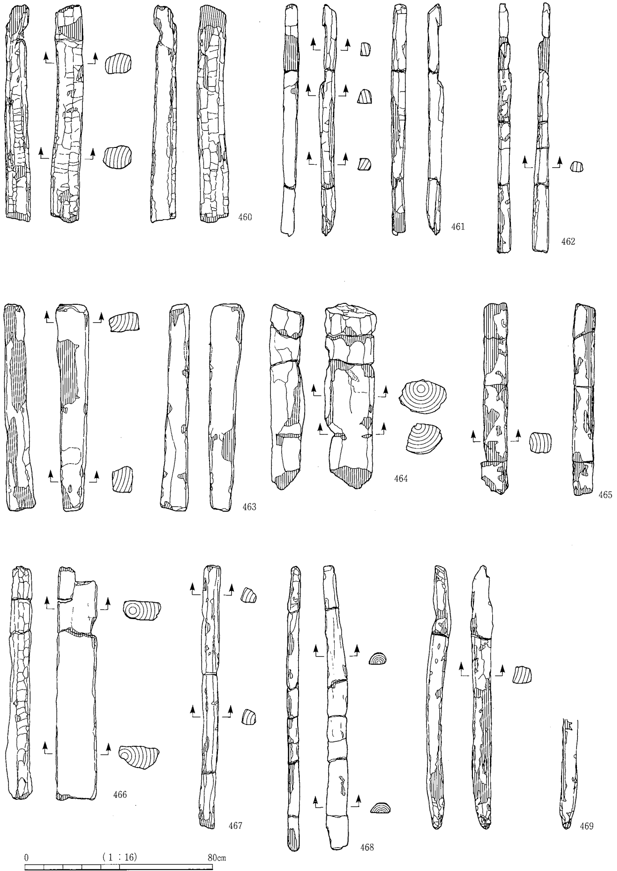
用途不明材 3
