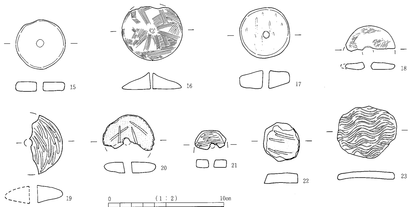
紡錘車
