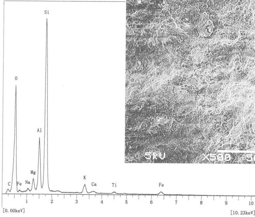
D. 基部原材面のEDX分析チャート
