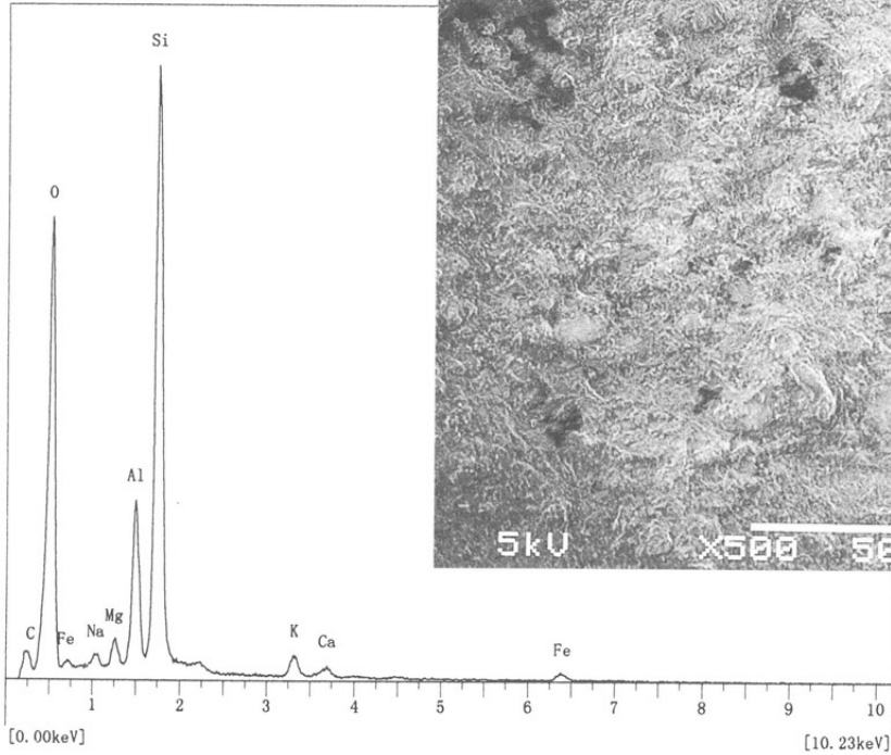
E. 摩耗・光沢部のEDX分析チャート
