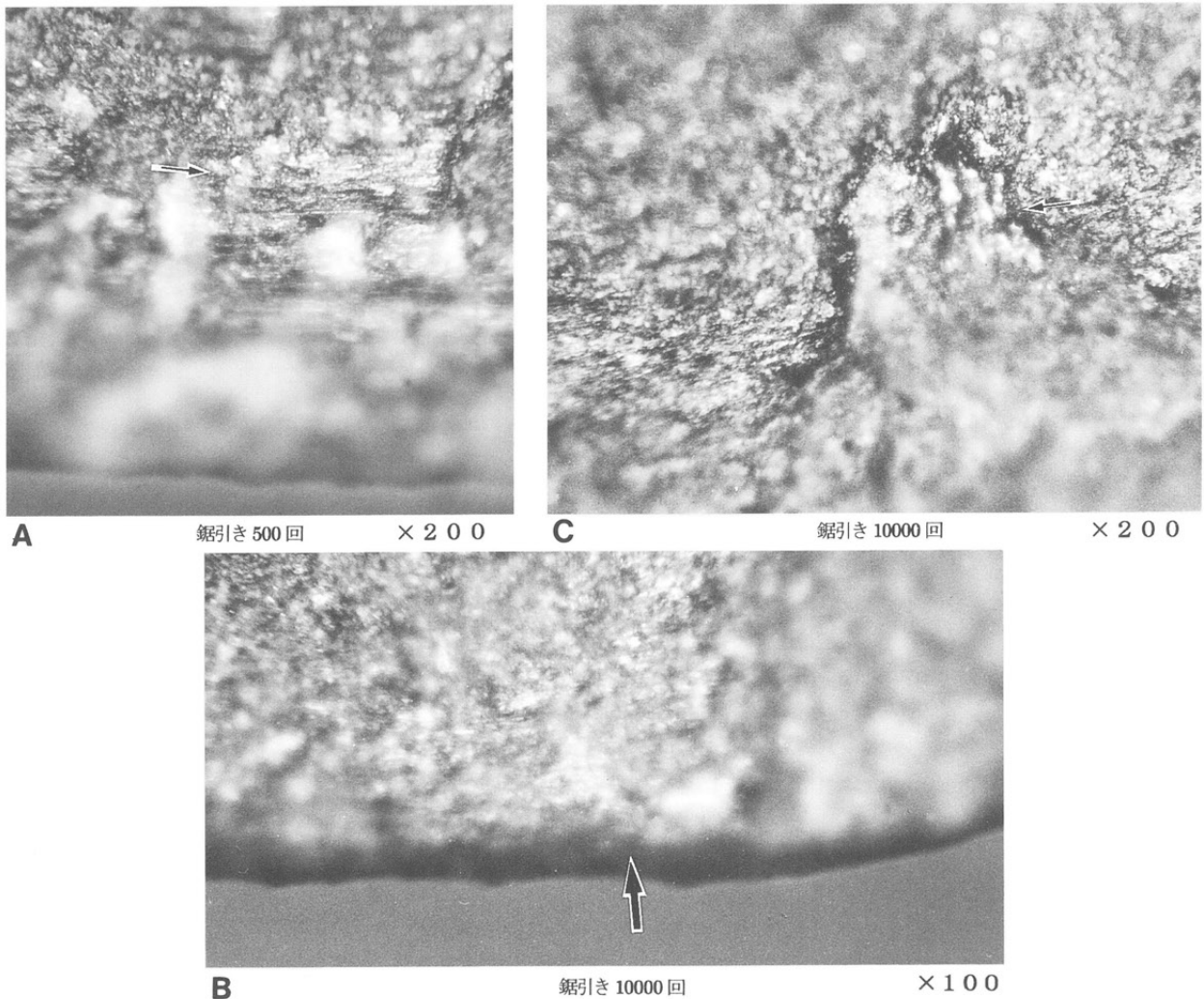
第315図 稲藁の鋸引き
