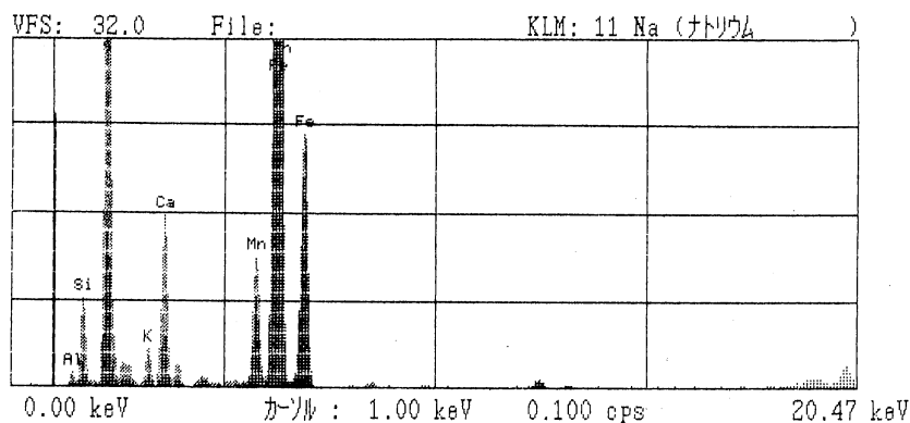
第329図 「鉄」類似資料の成分分析値
