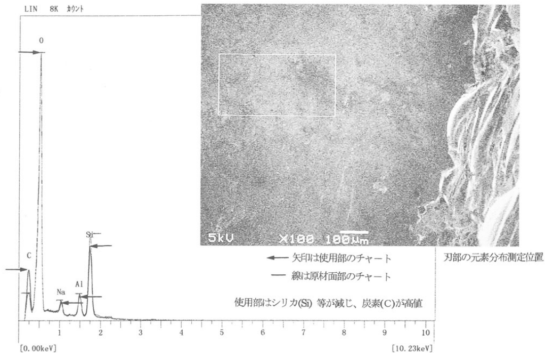
A. EDX分析値の比較チャート図
