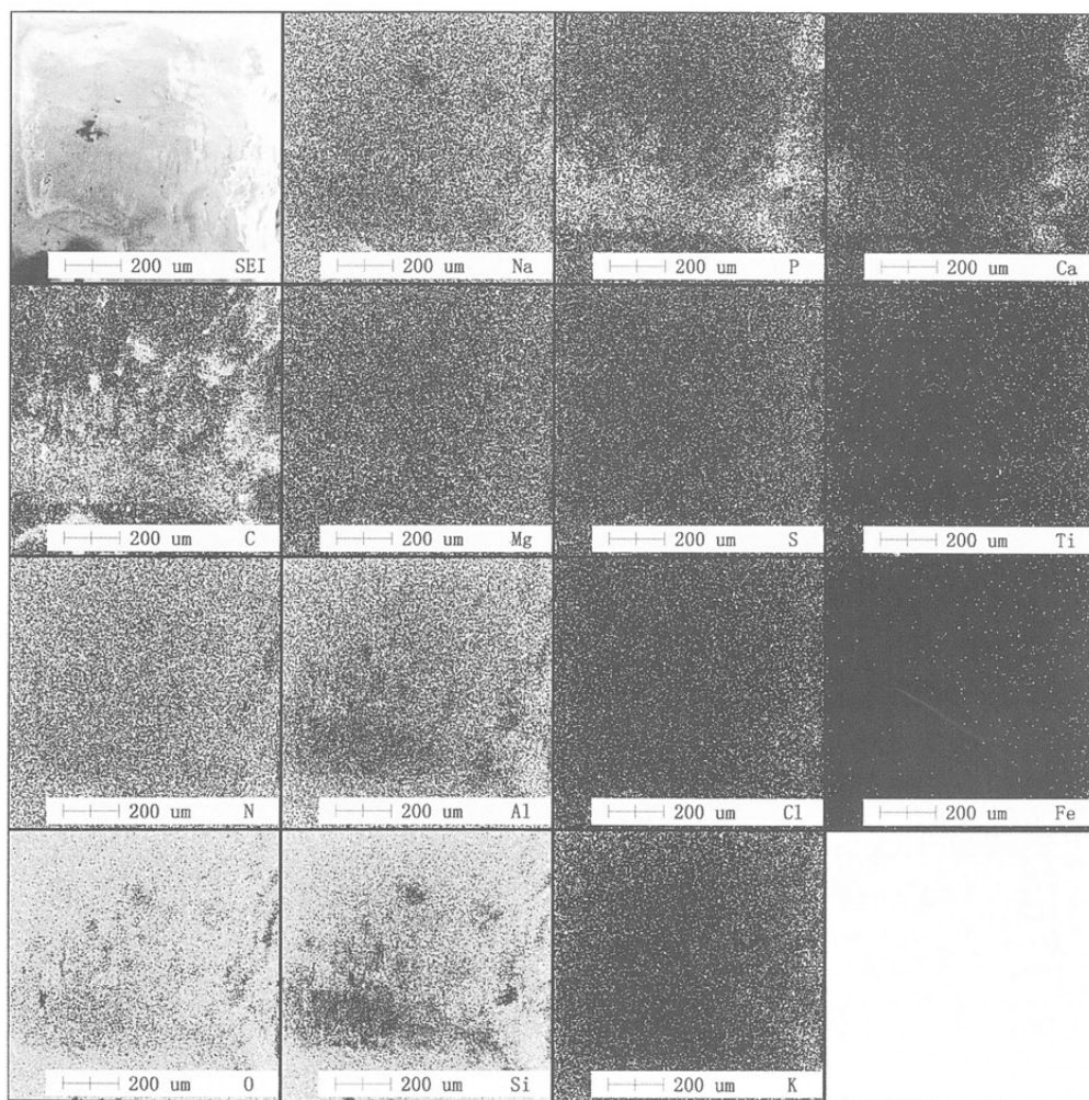
刃部の主要元素分布 (14 元素)
