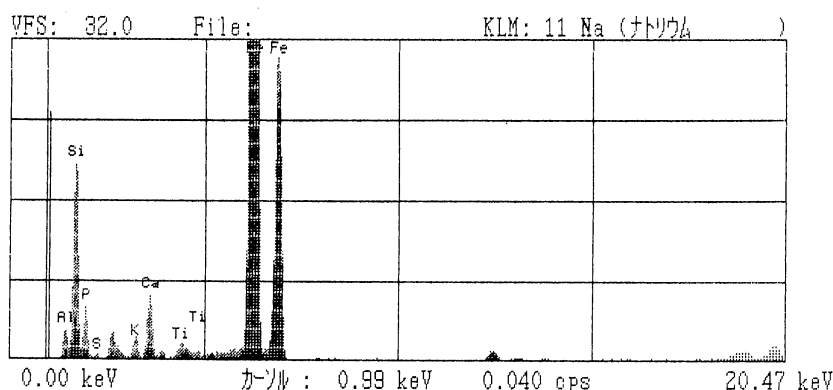
第328図 「鉄」資料の成分分析値
