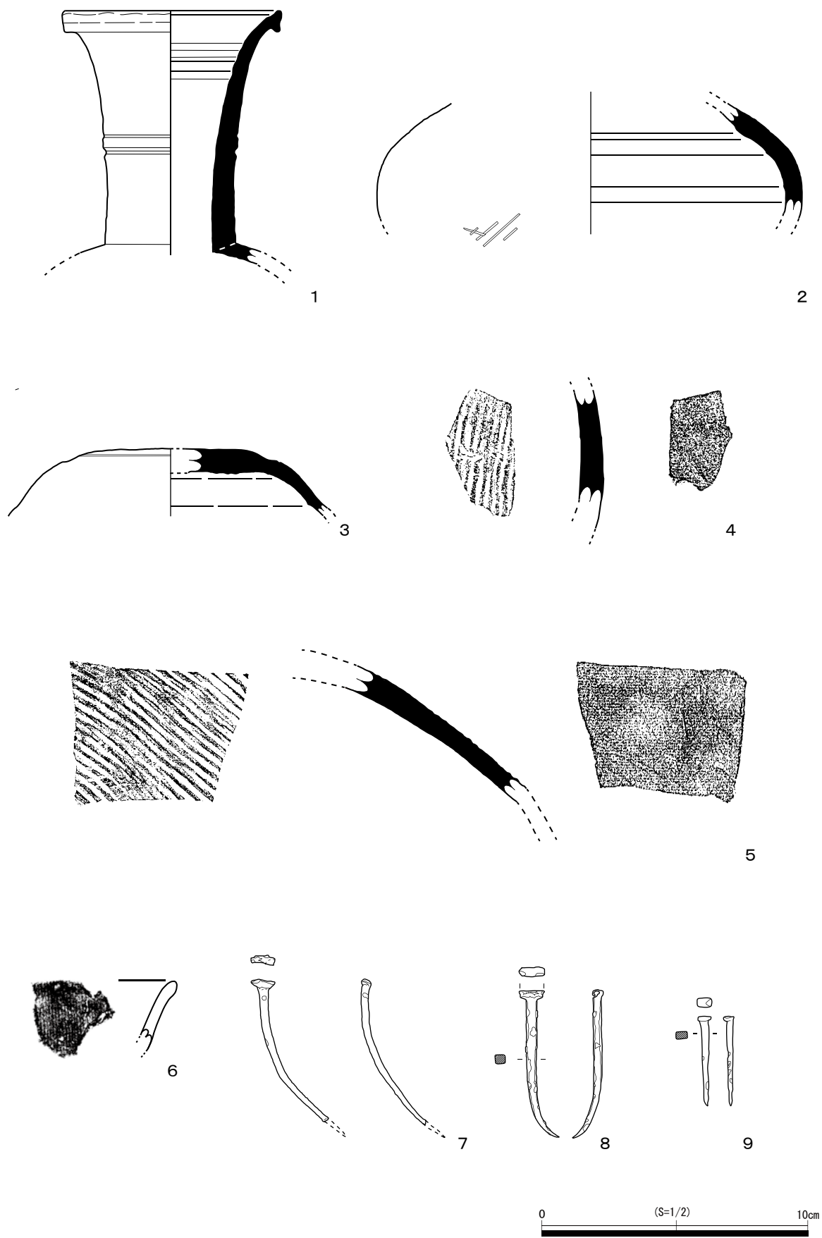
第11图 F 9号墳出土遺物実測図
