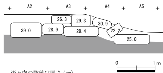
第9図 F9号墳石室側石模式図
