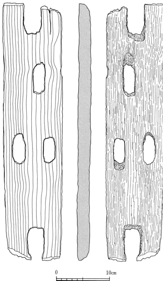
図23 平久保地区13号トレンチ出土木製品(1:4)
